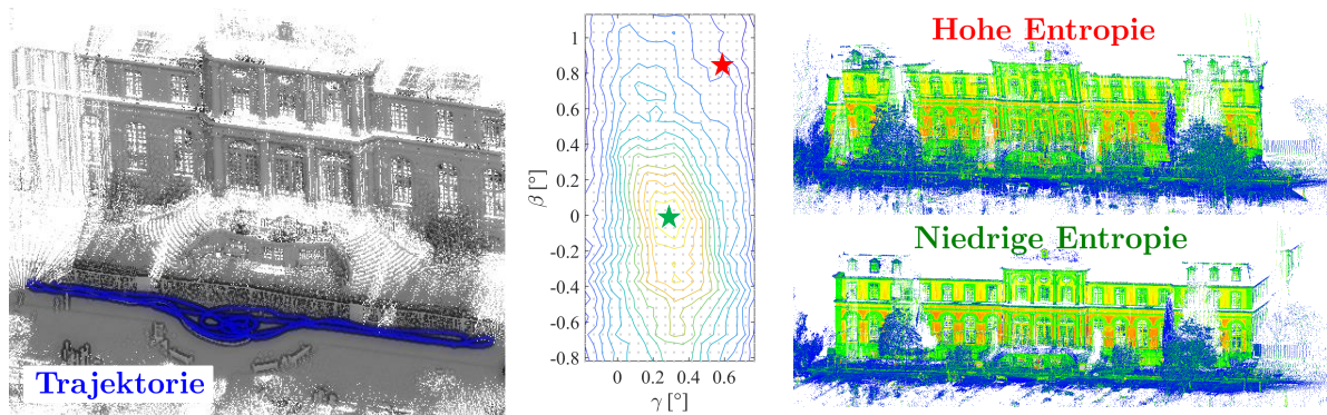
Abbildung 6.5: Entropiebasierte Kalibrierung zwischen einem Profillaserscanner und einer GNSS/IMU-Einheit am Poppelsdorfer Schloss in Bonn. Links: Kalibriermessung, Mitte: Niveaulinien der entropiebasierten Zielfunktion der Kalibrierung (nur Boresight-Winkel \beta und \gamma sind dargestellt), Rechts: Punktwolken mit hoher und niedriger Entropie, berechnet mit optimalen (grün) bzw. suboptimalen Kalibrierparametern (rot) [Janßen, 2017].
