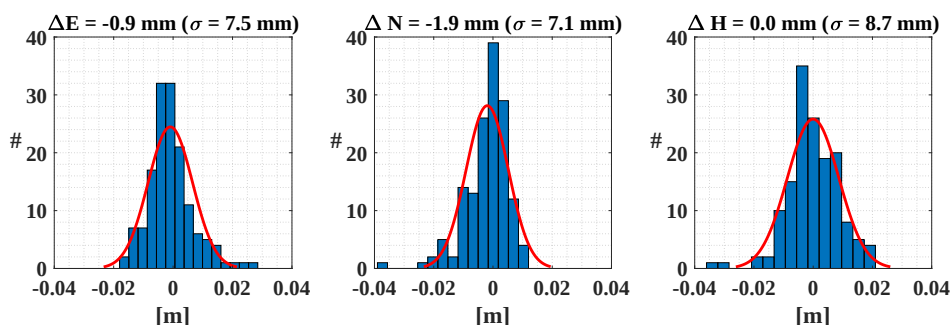
Abbildung 5.23: Ergebnisse der punktbasierten Evaluierung des Mobile Mapping Systems am Campus Klein-Altendorf für Ost-, Nord- und Höhenkomponente basierend auf 148 Scans von Kontrollpunkten aus dem Referenzfestpunktfeld (Abbildung aus Heinz et al. [2020b], modifiziert).
