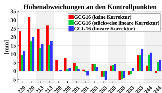
Abbildung 5.22: Signalisierung und Aufnahme eines Kontrollpunktes mit dem Mobile Mapping System (oben). Ergebnisse der punktbasierten Evaluierung der Höhenkomponente mit und ohne Korrekturfunktion für das Quasigeoidmodell GCG16 (unten) (Abbildung aus Heinz et al. [2020a], modifiziert).
