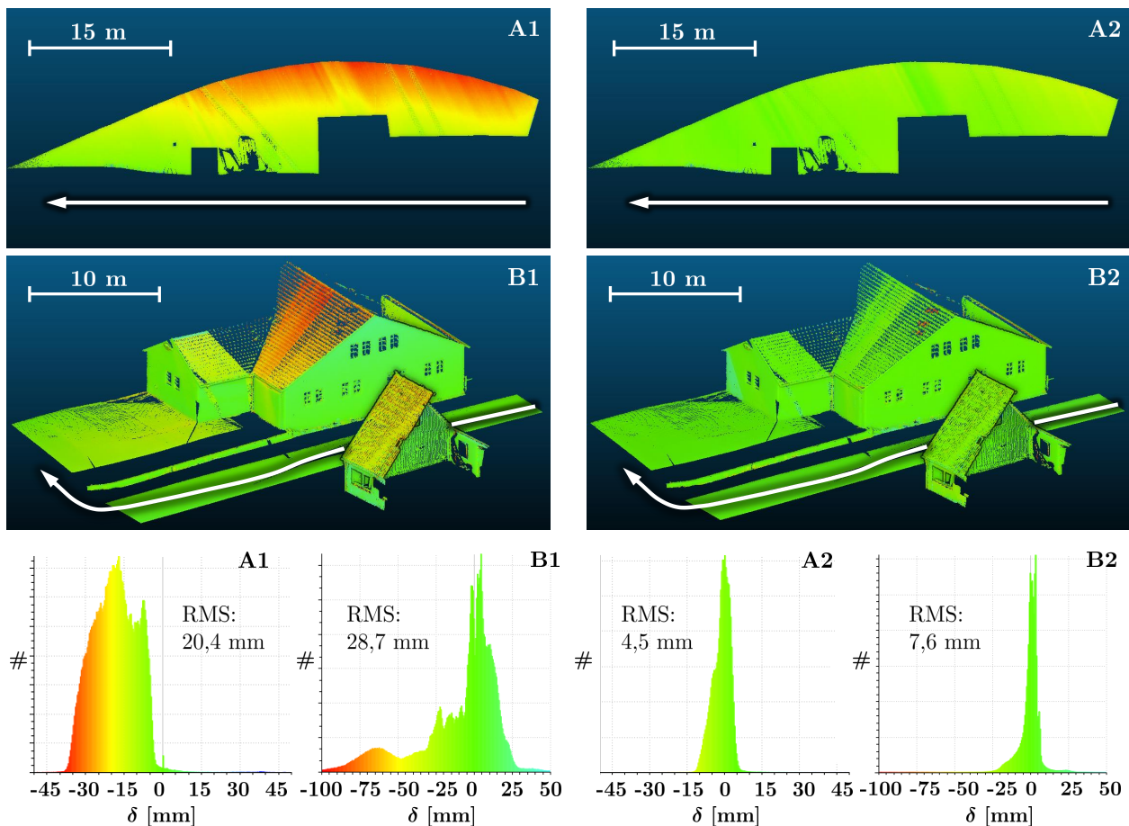
Abbildung 5.26: M3C2-Punktwolkenvergleiche zwischen einer TLS-Referenzpunktwolke und Punktwolken des fahrzeuggetragenen Mobile Mapping Systems. Die Punktwolken des mobilen Systems wurden mithilfe einer Näherungskalibrierung aus der Konstruktionszeichnung des Systems (A1 und B1) und mithilfe der ebenenbasierten Kalibrierung aus Abschnitt 5.4.3 (A2 und B2) berechnet (Abbildung aus Heinz et al. [2020b], modifiziert).
