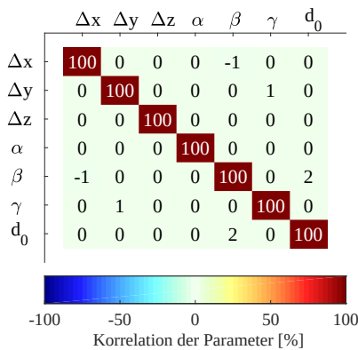
Abbildung 5.14: Parameterkorrelationen für 0° Scannerneigung.
