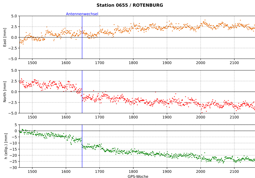
Abbildung 4.3: Koordinatenzeitreihe der GNSS-Referenzstation Rotenburg (0655)
