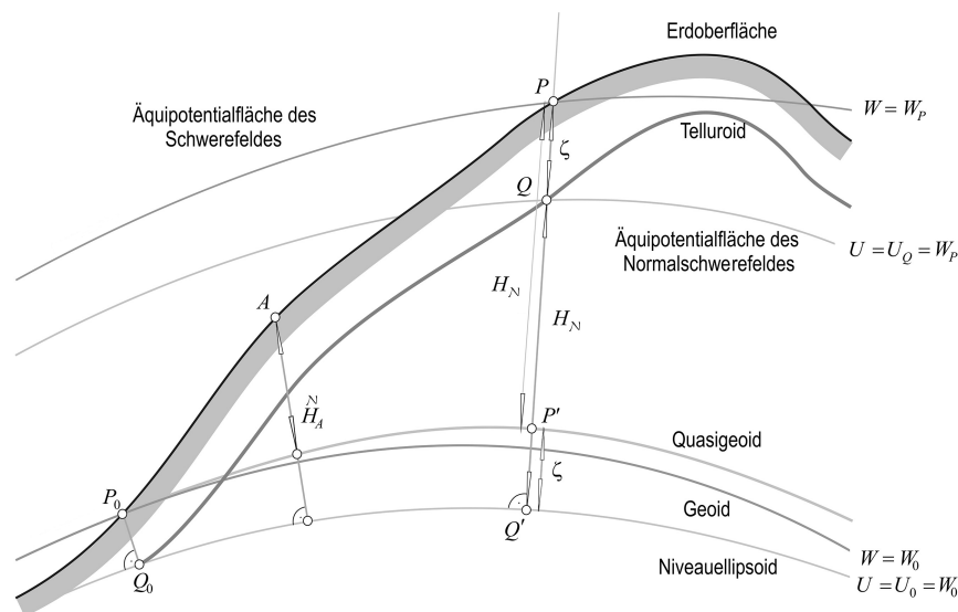
Abbildung 2.2: Normalhöhe H_N , Telluroid und Quasigeoid (vgl. Ilk, 2021)
