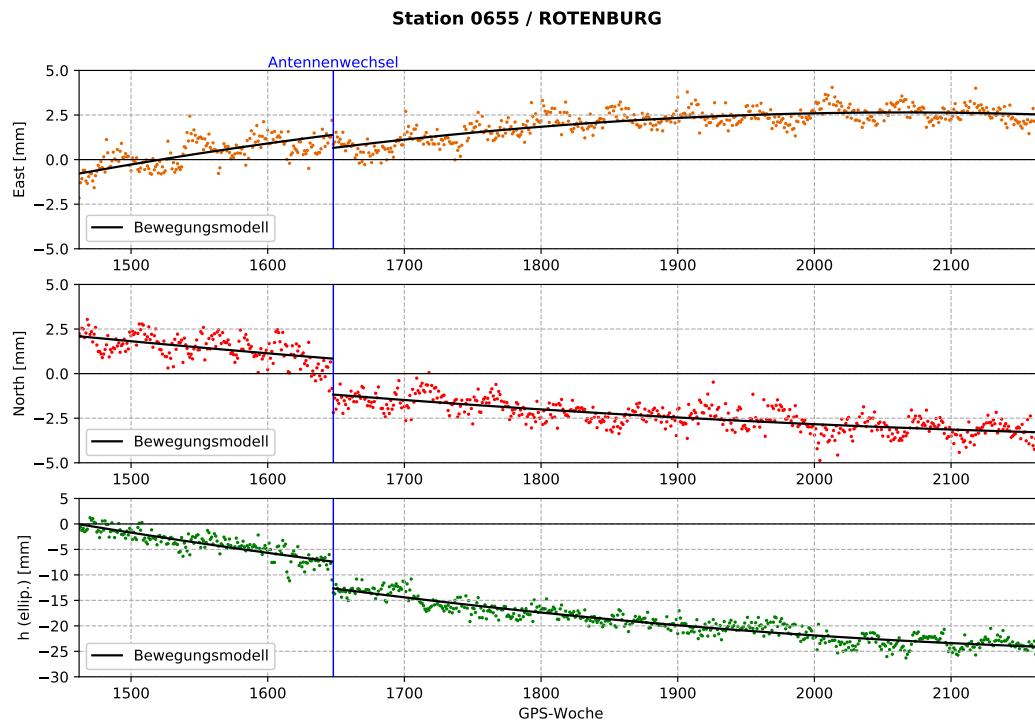
Abbildung 4.5: Zeitpolynome für die Koordinatenzeitreihe der Referenzstation Rotenburg (0655)
