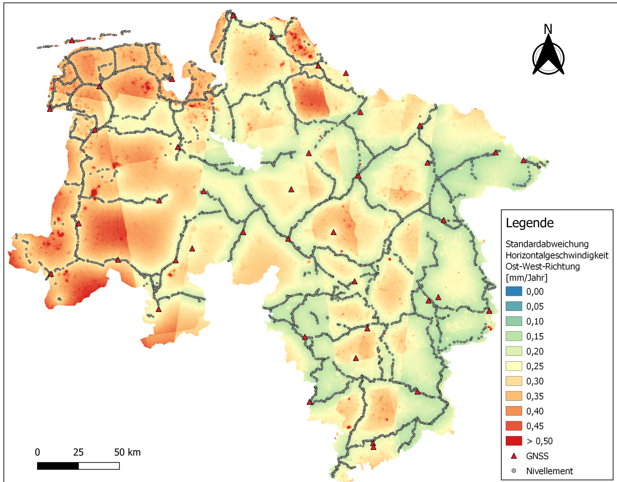
Abbildung 6.13: Standardabweichungen zu den modellierten Horizontalbewegungen
