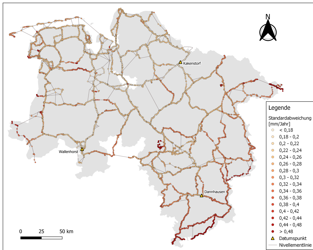
Abbildung A.6: Standardabweichungen der Vertikalgeschwindigkeiten im niedersächsischen Nivellementnetz unter Verwendung einer Teilspurminimierung mit drei Datumspunkten
