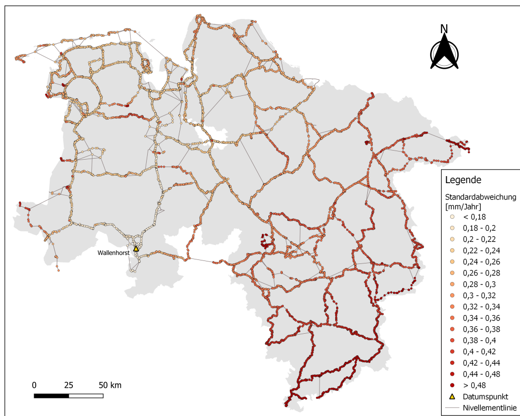
Abbildung A.8: Standardabweichungen der Vertikalgeschwindigkeiten im niedersächsischen Nivellementnetz durch Lagerung auf die UF Wallenhorst
