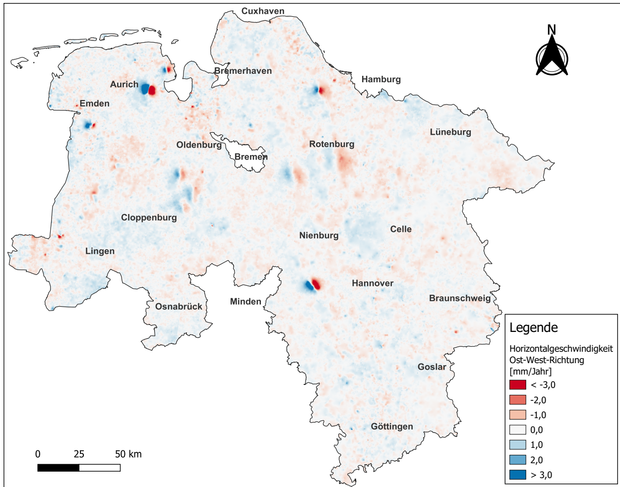
Abbildung 6.12: Niedersächsisches Bodenbewegungsmodell - Horizontalbewegungen
