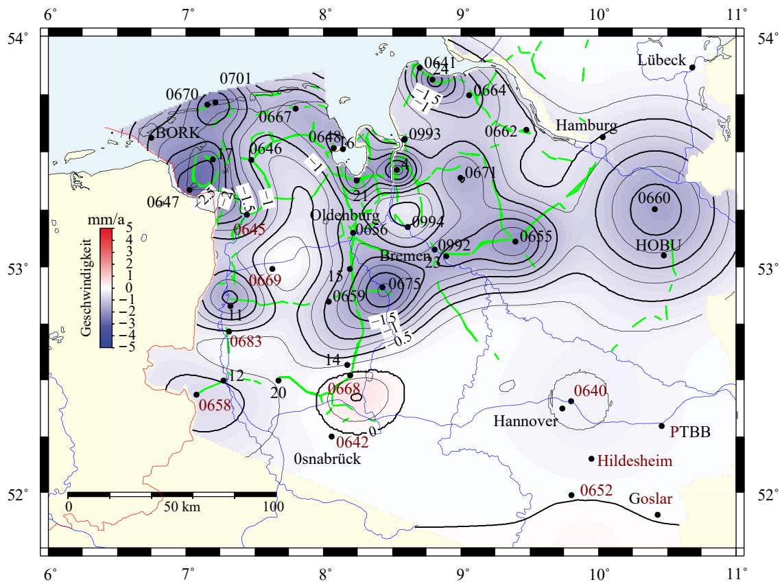
Abbildung 2.4: Geschwindigkeitsfeld als Ergebnis der Kombination aus Nivellement- und GPS-Daten des IKÜS-Projektes (Wanninger u. a., 2009)
