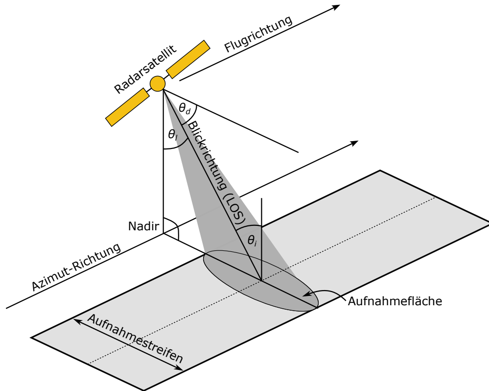
Abbildung 2.6: Aufnahmegeometrie eines Radarsystems (vgl. Woodhouse, 2006, S. 266)
