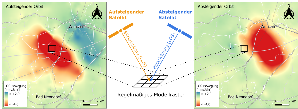
Abbildung 6.9: Aufnahmegeometrie von auf- und absteigenden Radarsatelliten
