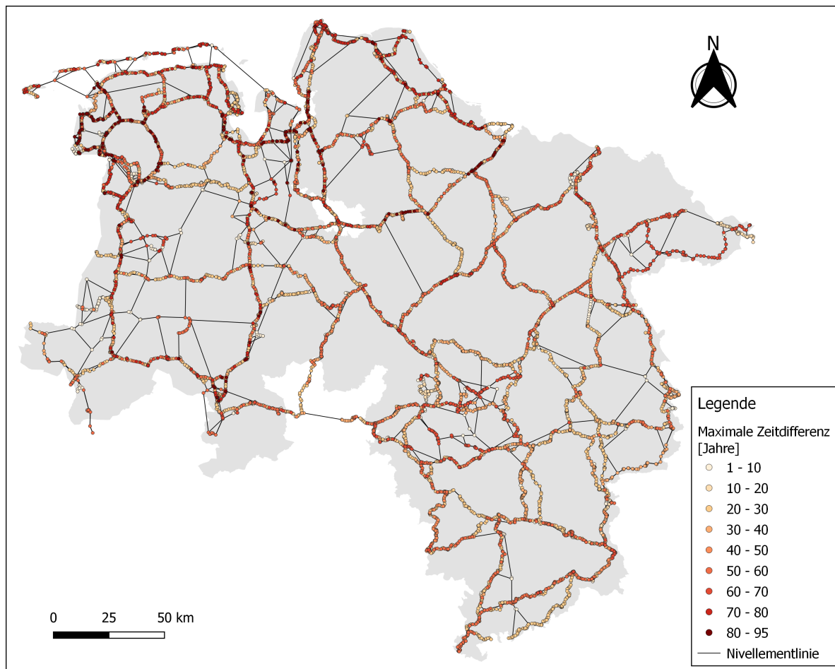
Abbildung 4.18: Aufbereitetes Nivellementnetz als Datengrundlage für die kinematische Höhenausgleichung
