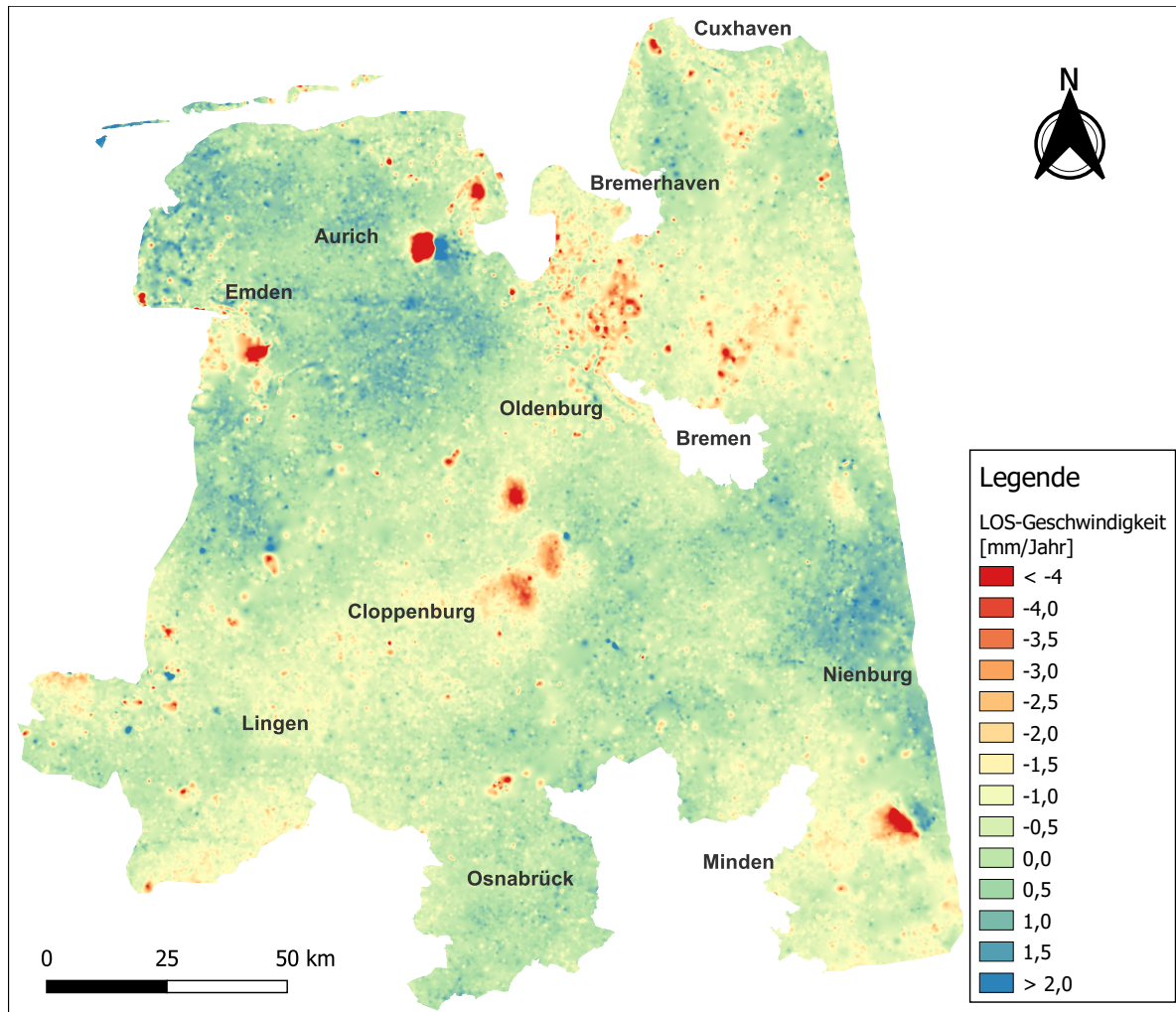
Abbildung 5.4: Unkalibriertes Bewegungsmodell für den SAR-Stack 015_01 aus der MBA
