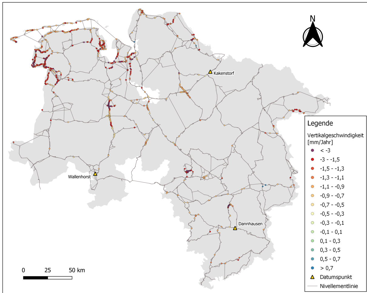
Abbildung 4.21: Signifikante Vertikalgeschwindigkeiten im niedersächsischen Nivellementnetz mit 1% Irrtumswahrscheinlichkeit
