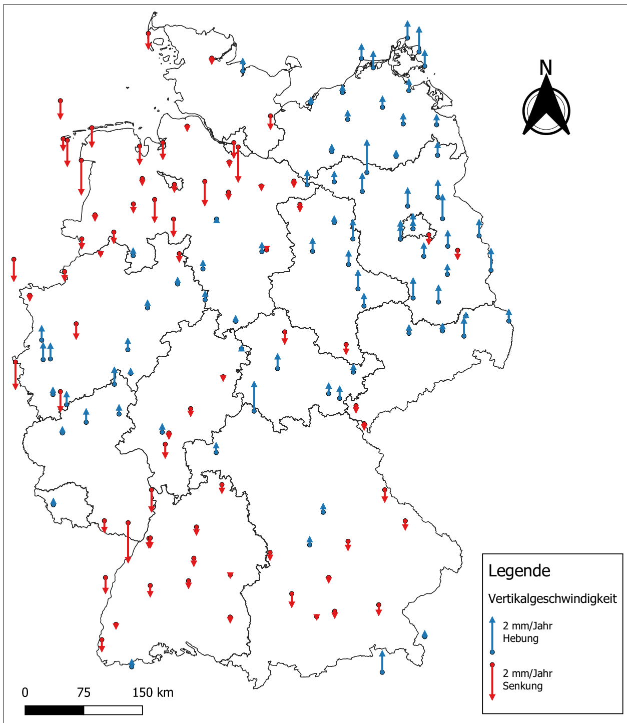
Abbildung A.3: Signifikante Vertikalgeschwindigkeiten der GNSS-Referenzstationen mit 1% Irrtumswahrscheinlichkeit
