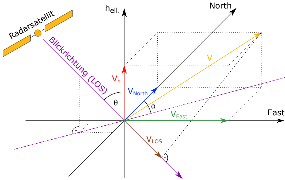
Abbildung 6.1: Projektion einer 3D-Bewegung auf die LOS-Richtung (vgl. Yin, 2020, S. 43)
