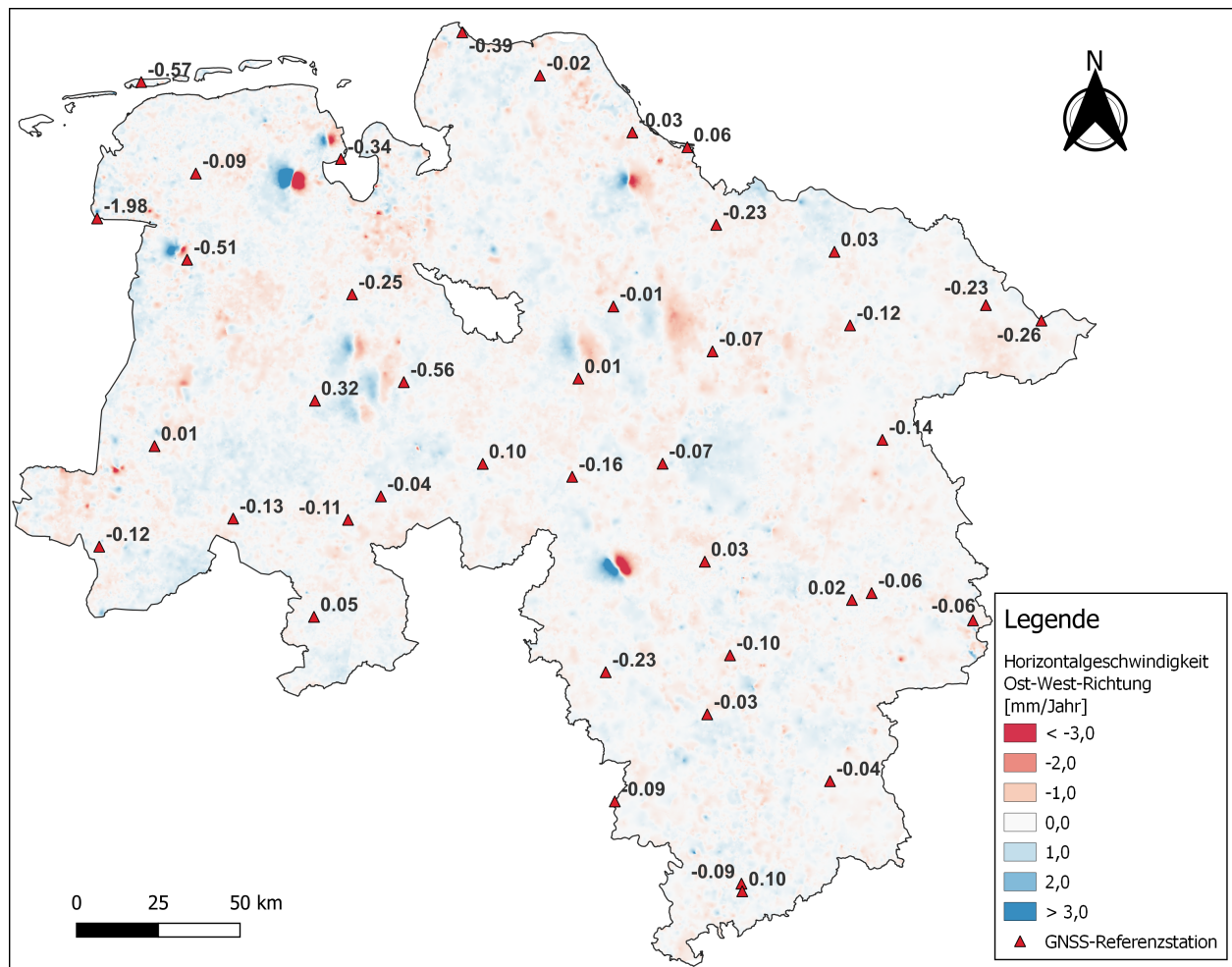
Abbildung 6.17: Differenzen zwischen modellierten Horizontalbewegungen und Verschiebungen der GNSS-Referenzstationen
