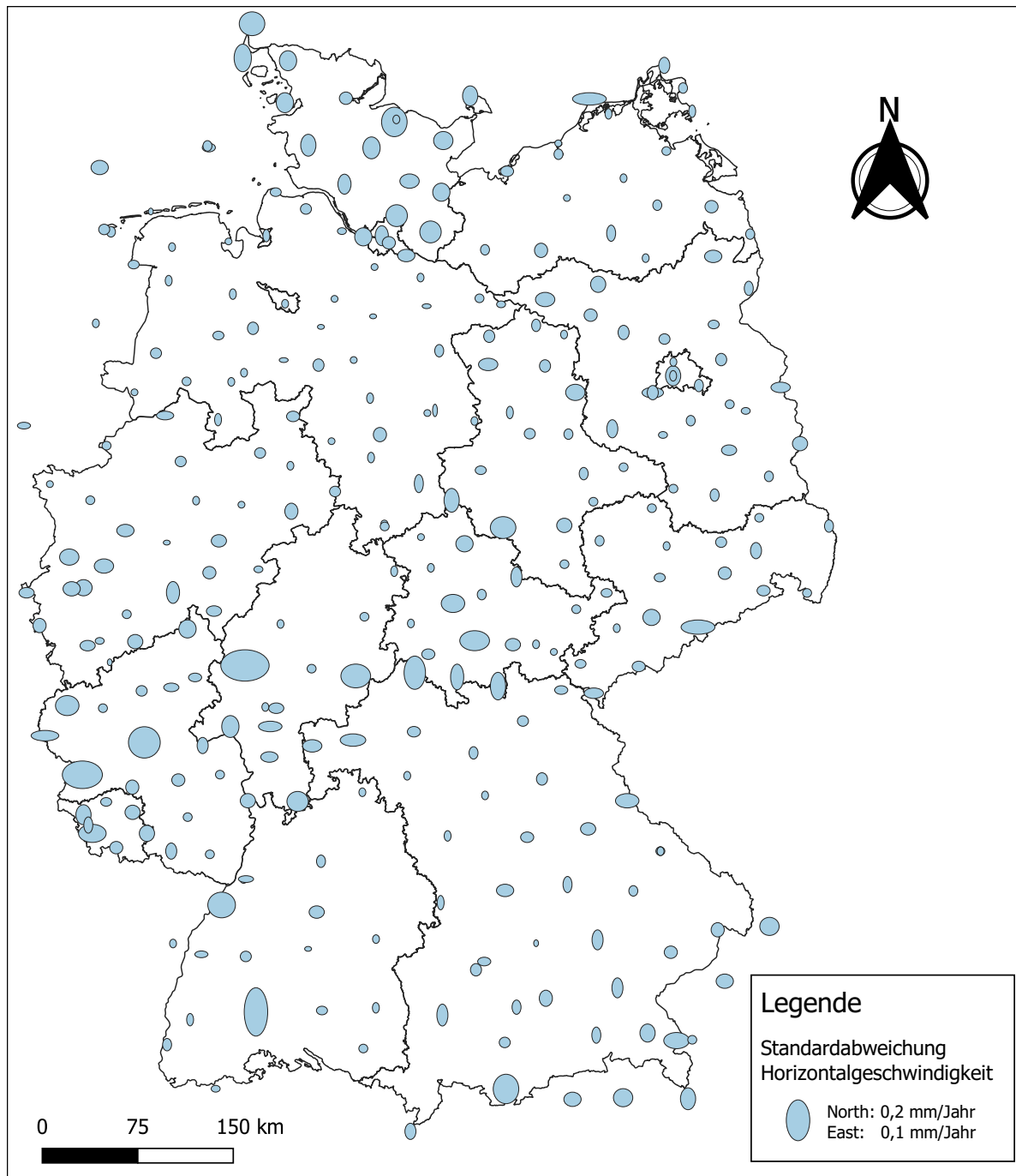
Abbildung 4.10: Standardabweichungen von den Horizontalgeschwindigkeiten der analysierten GNSS-Referenzstationen
