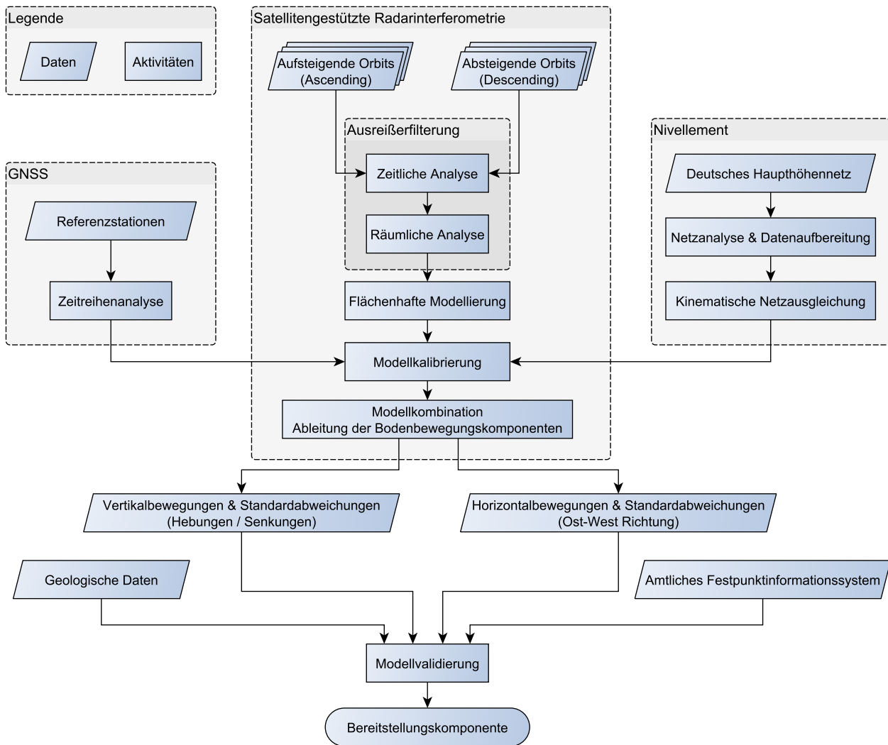
Abbildung 2.7: Prozesskette zur flächenhaften Modellierung von Bodenbewegungen
