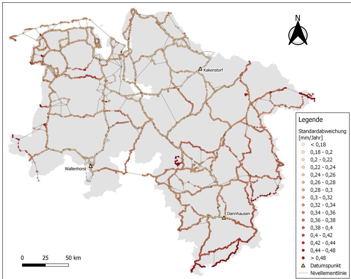
Abbildung 4.20: Standardabweichungen der Vertikalgeschwindigkeiten im niedersächsischen Nivellementnetz
