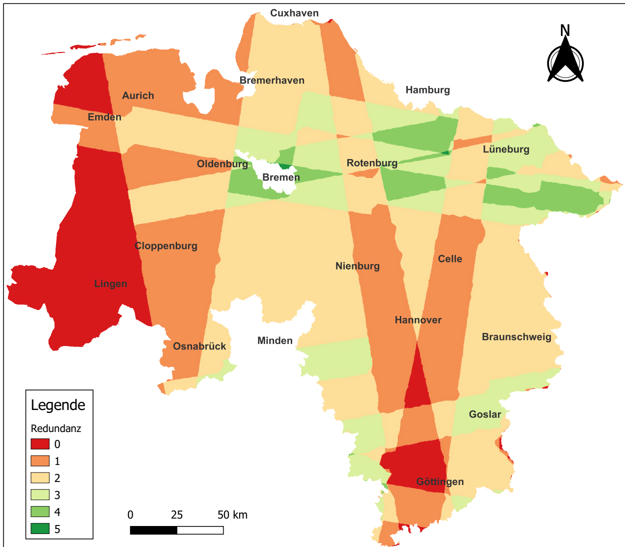
Abbildung C.1: Redundanz im Ausgleichsprozess zur Bestimmung der Vertikal- und Horizontalbewegungen
