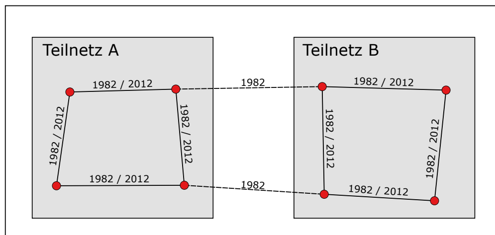
Abbildung 4.17: Wiederholt beobachtetes Nivellementnetz mit Konfigurationsdefekt in der kinematischen Höhenausgleichung
