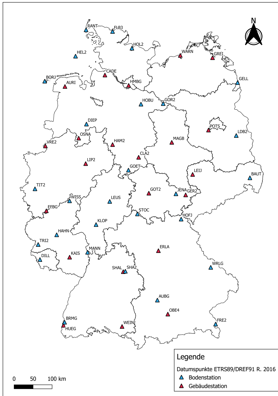
Abbildung A.1: Datumsstationen zur Transformation zwischen ITRF2014 und ETRS89/DREF91 (Realisierung 2016) (Stand: 11.07.2021)
