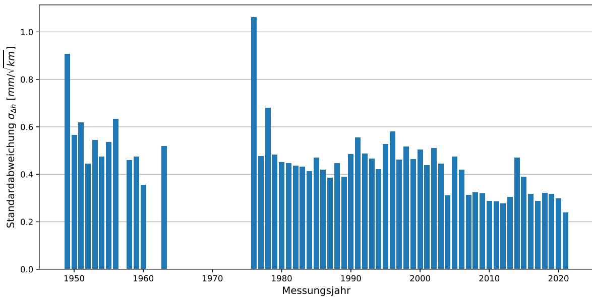
Abbildung 4.15: Zeitliche Verteilung der Standardabweichungen des Doppelnivellements
