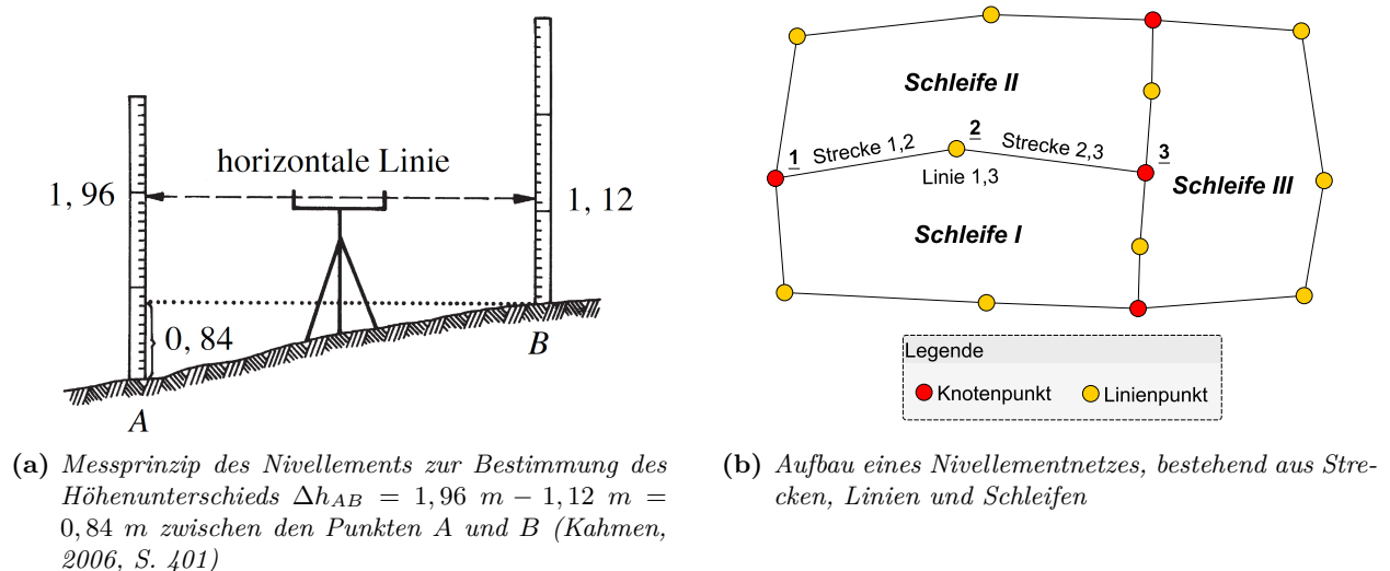
Abbildung 2.5: Grundprinzip des geometrischen Nivellements
