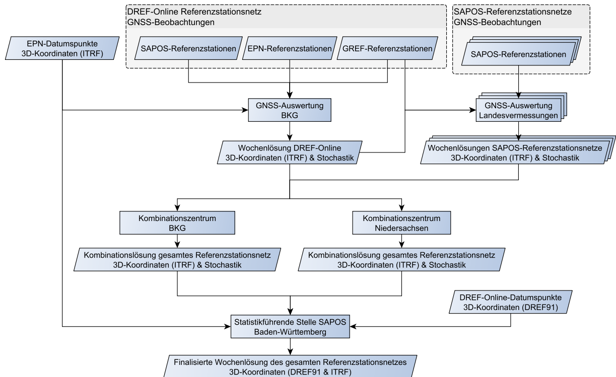
Abbildung 4.1: Prozesskette zur GNSS-Prozessierung des bundesweiten Referenzstationsnetzes
