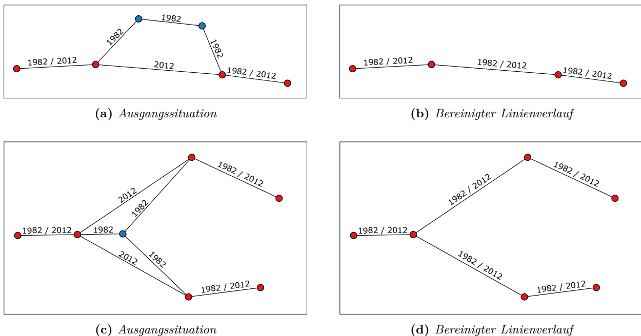
Abbildung 4.16: Zusammenfassung einfach gemessener Nivellementstrecken zwischen wiederholt beobachteten HFPs
