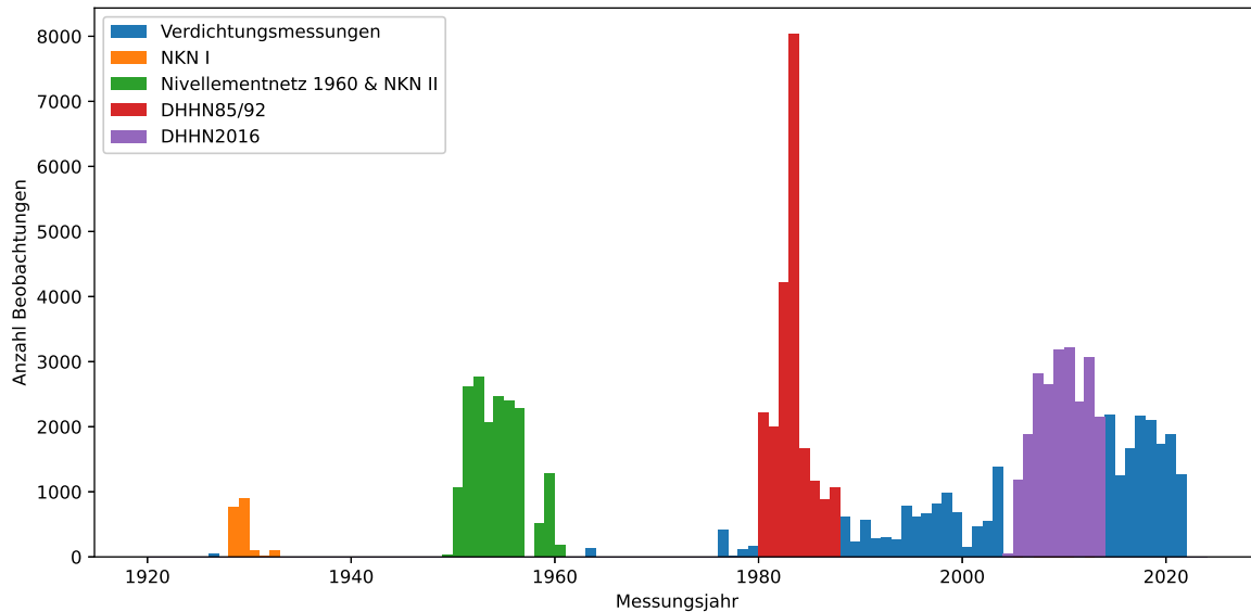
Abbildung 4.14: Zeitliche Verteilung der nivellierten Höhenunterschiede
