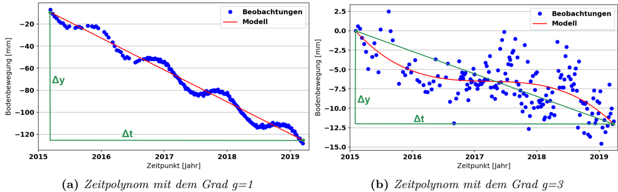
Abbildung 4.30: Bewegungstrends aus verschiedenen Zeitpolynomen (Koppmann, 2020, S. 47)
