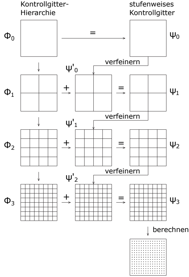
Abbildung 3.4: Schematische Darstellung des optimierten MBA-Algorithmus unter Verwendung einer B-Spline Verfeinerung (Nuckelt, 2007, S. 17)
