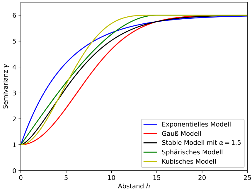
Abbildung 3.7: Verläufe unterschiedlicher theoretischer Variogrammfunktionen
