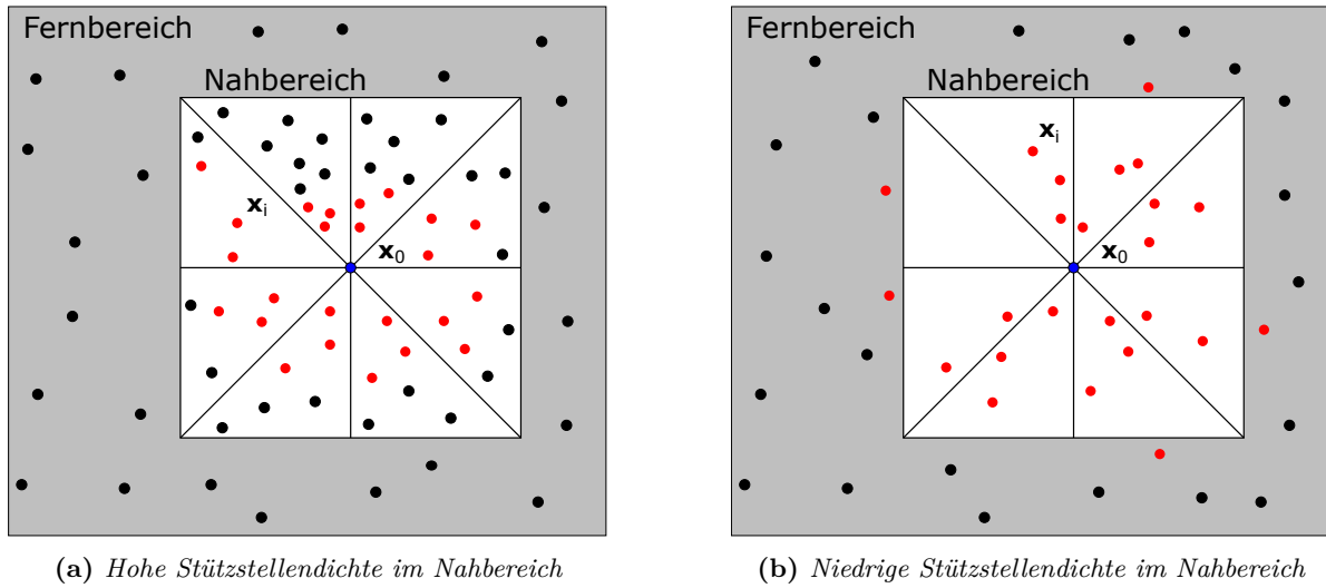
Abbildung 3.8: Stützstellenauswahl zur lokalen Kriging-Approximation
