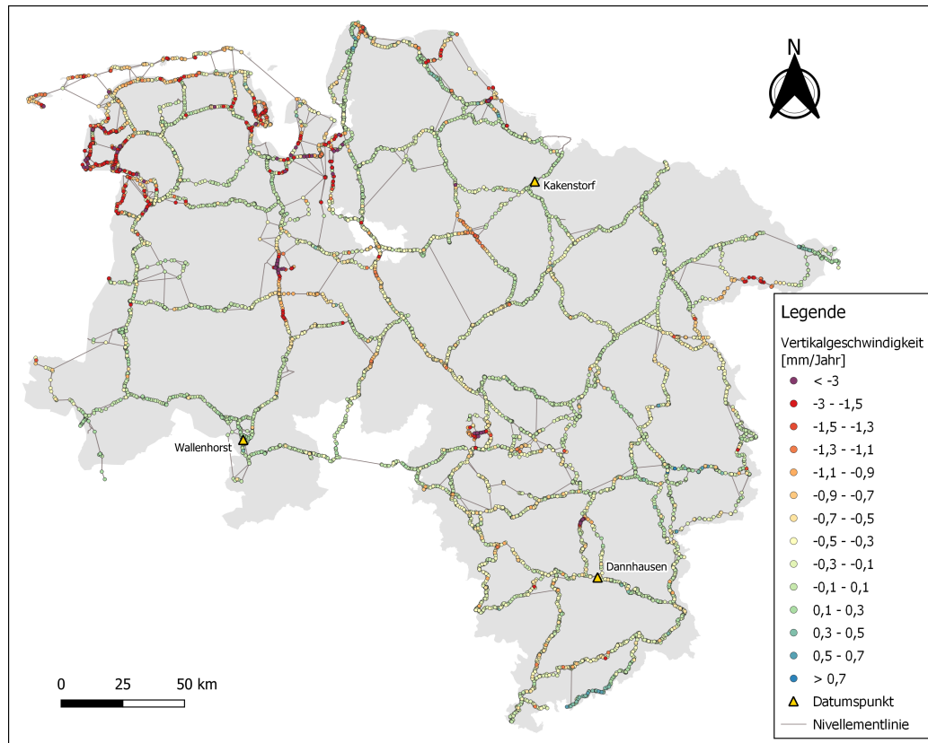
Abbildung A.5: Vertikalgeschwindigkeiten im niedersächsischen Nivellementnetz unter Verwendung einer Teilspurminimierung mit drei Datumspunkten
