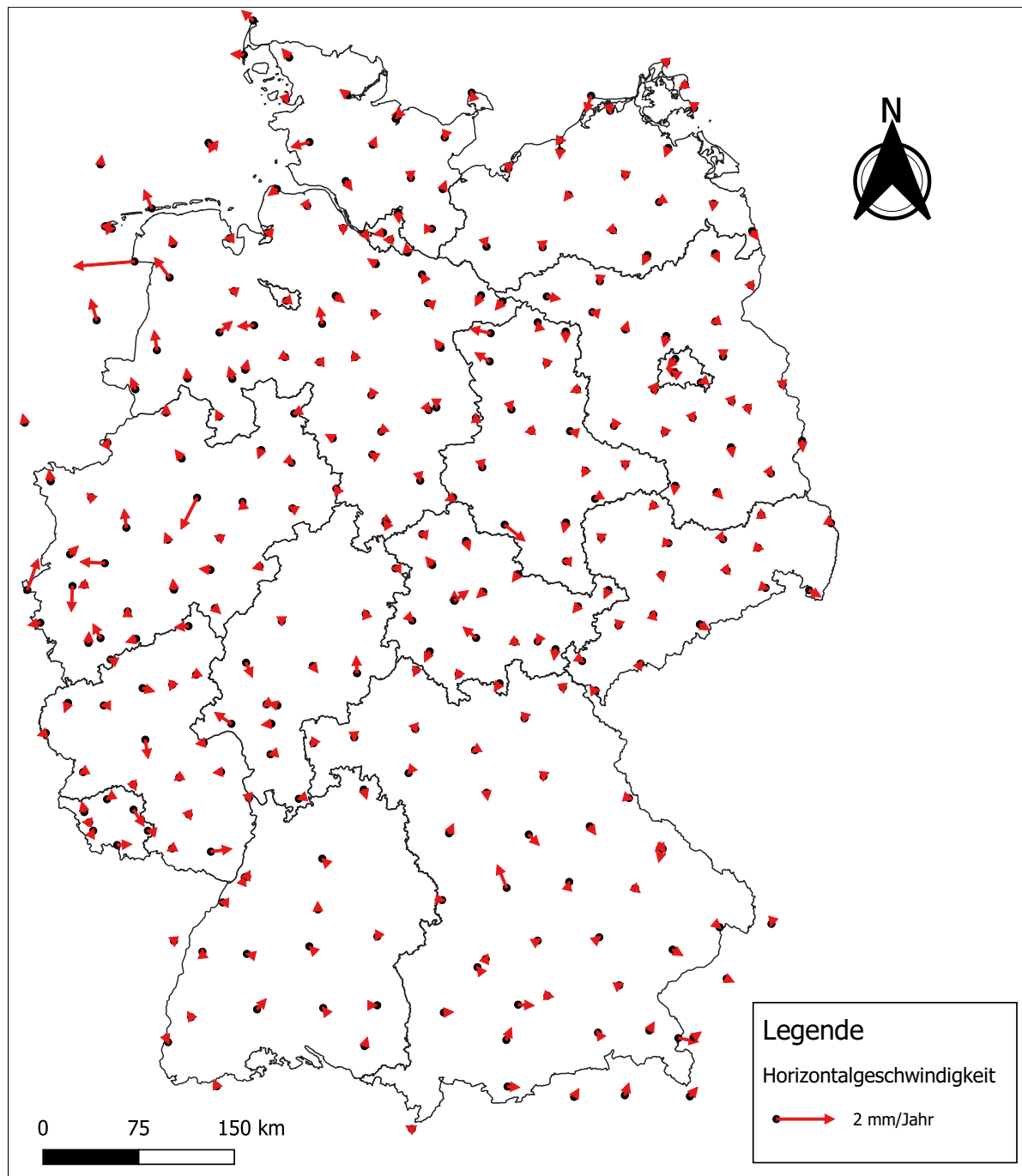
Abbildung 4.9: Horizontalgeschwindigkeiten der analysierten GNSS-Referenzstationen
