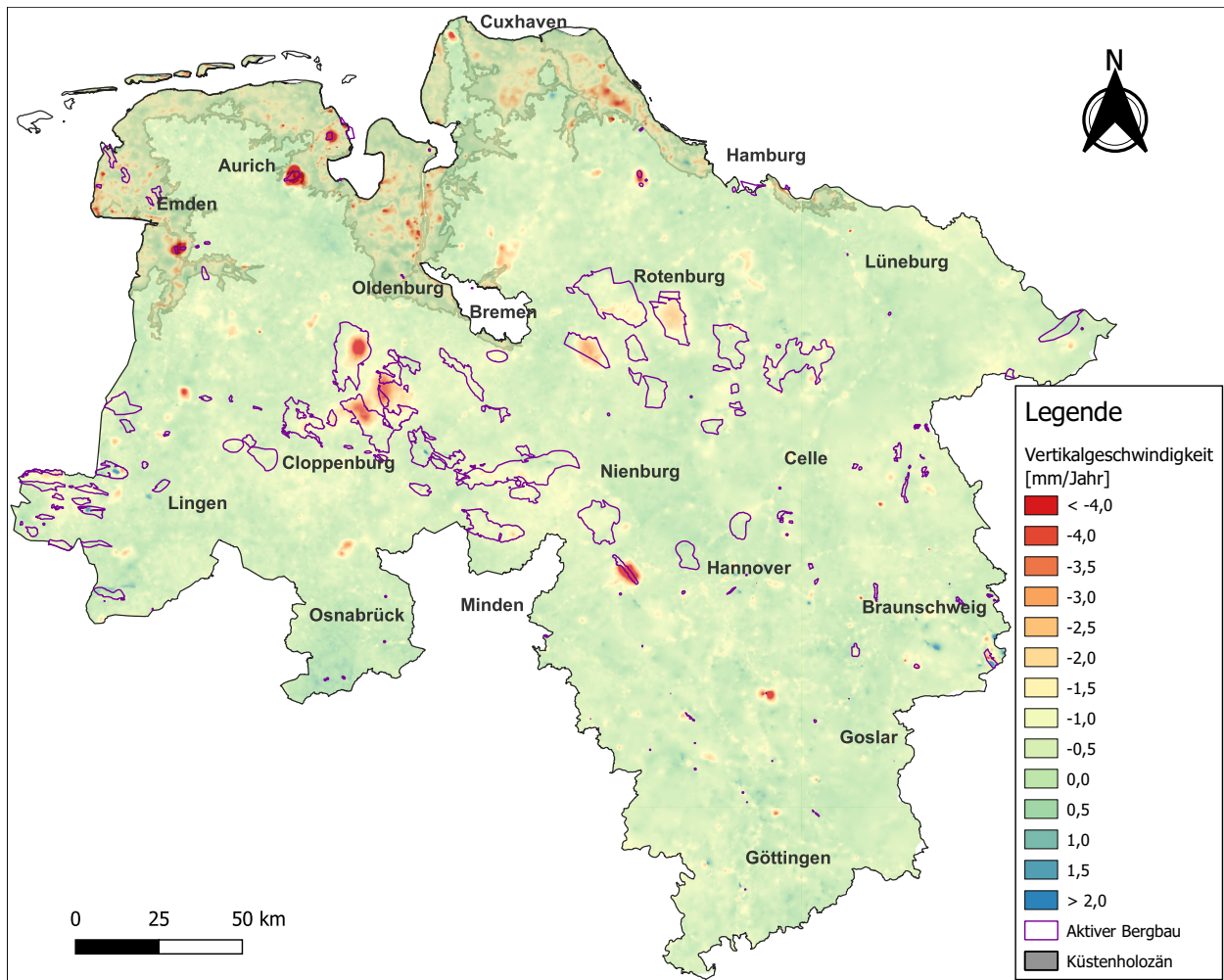
Abbildung 6.14: Modellierte Vertikalbewegungen im Zusammenhang mit geologischen Fachdaten (vgl. NIBIS® Kartenserver, 2021a,b)
