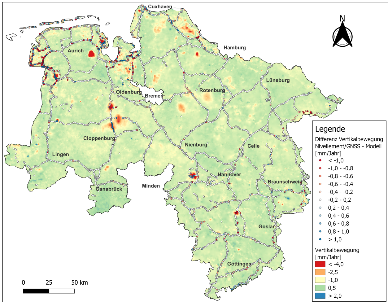
Abbildung 6.15: Differenzen zwischen modellierten Vertikalbewegungen und Höhenänderungen aus Nivellement und GNSS
