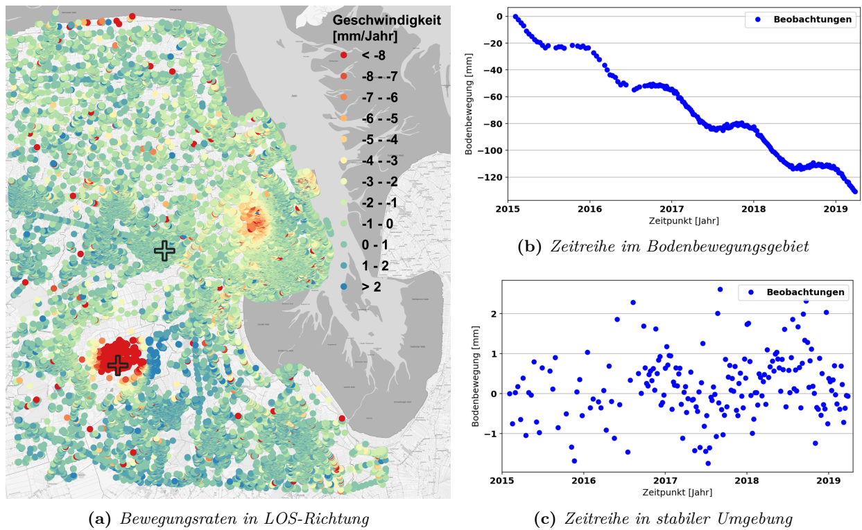
Abbildung 4.27: PSI-Daten für das exemplarische Gebiet Wilhelmshaven (Koppmann, 2020, S.34)
