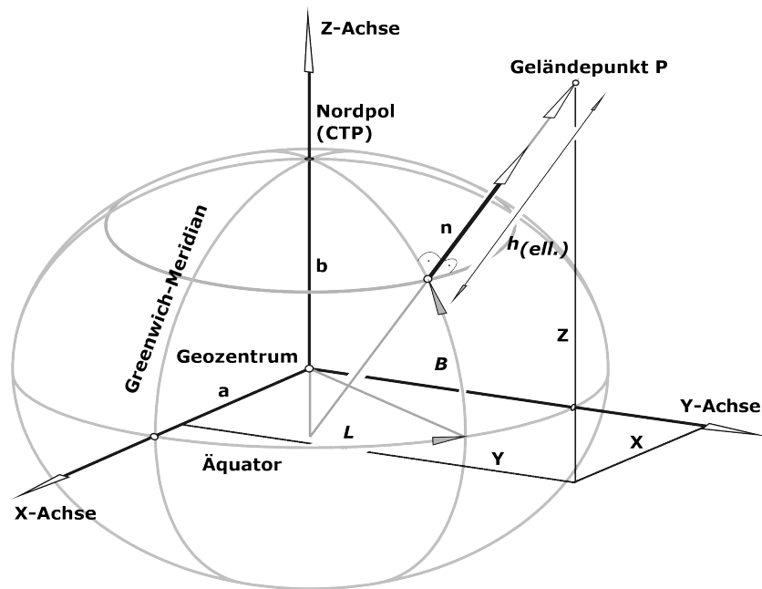
Abbildung 2.1: Beschreibung der geometrischen 3D-Position eines Geländepunktes mittels ellipsoidischer und kartesischer Koordinaten (vgl. Ilk, 2021)
