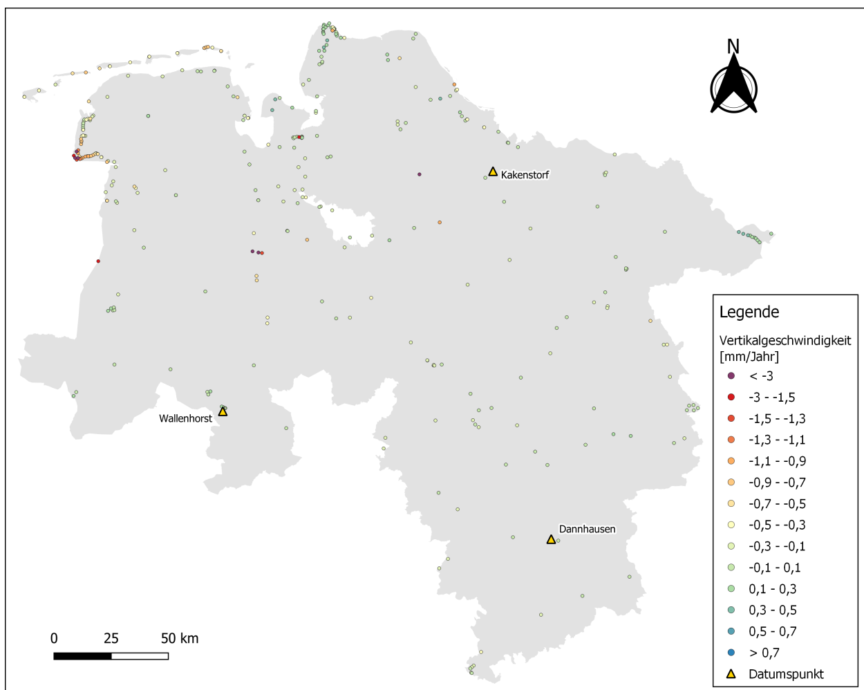
Abbildung 4.24: Vertikalgeschwindigkeiten von UFs und tief gegründeten RFs
