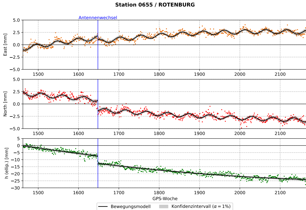
Abbildung 4.7: Vollständiges Bewegungsmodell der Referenzstation Rotenburg (0655)
