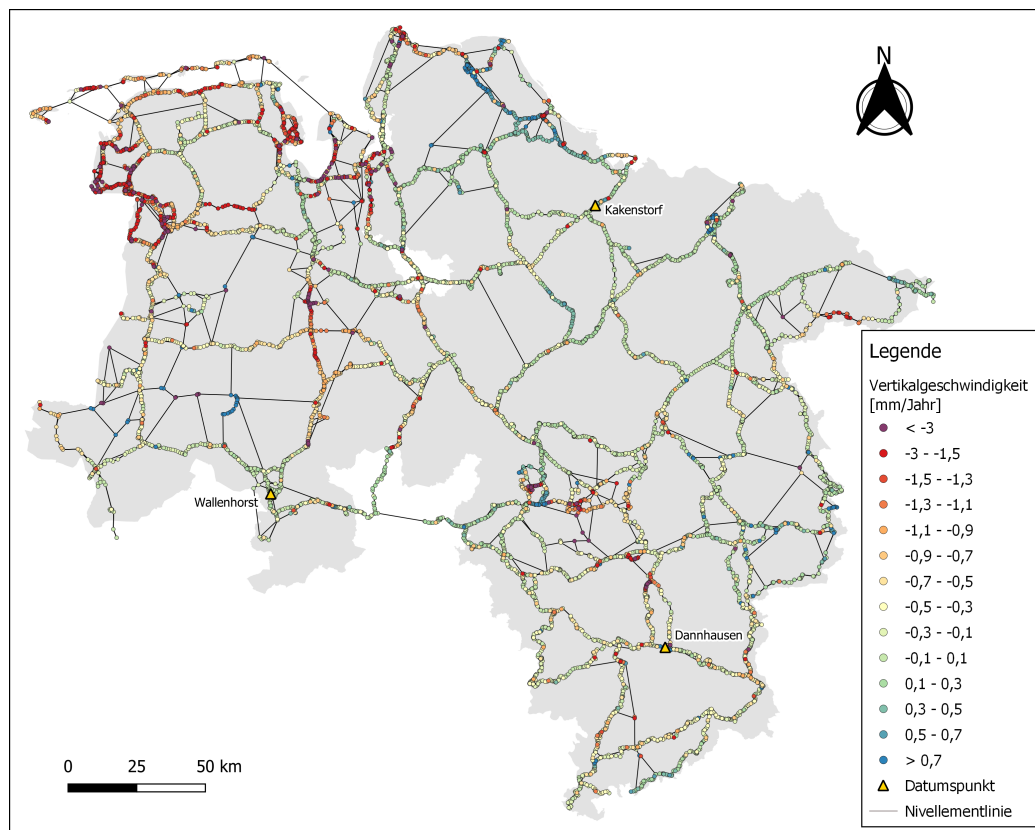
Abbildung A.4: Vertikalgeschwindigkeiten im niedersächsischen Nivellementnetz ohne detaillierte Datenaufbereitung und Entfernung grober Ausreißer
