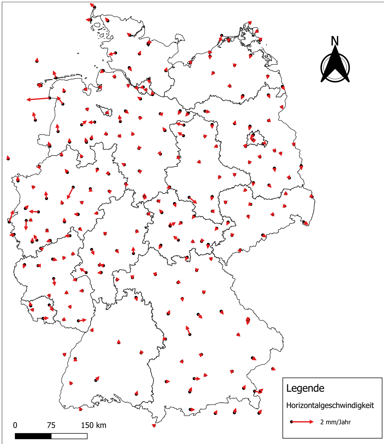
Abbildung A.2: Signifikante Horizontalgeschwindigkeiten der GNSS-Referenzstationen mit 1% Irrtumswahrscheinlichkeit
