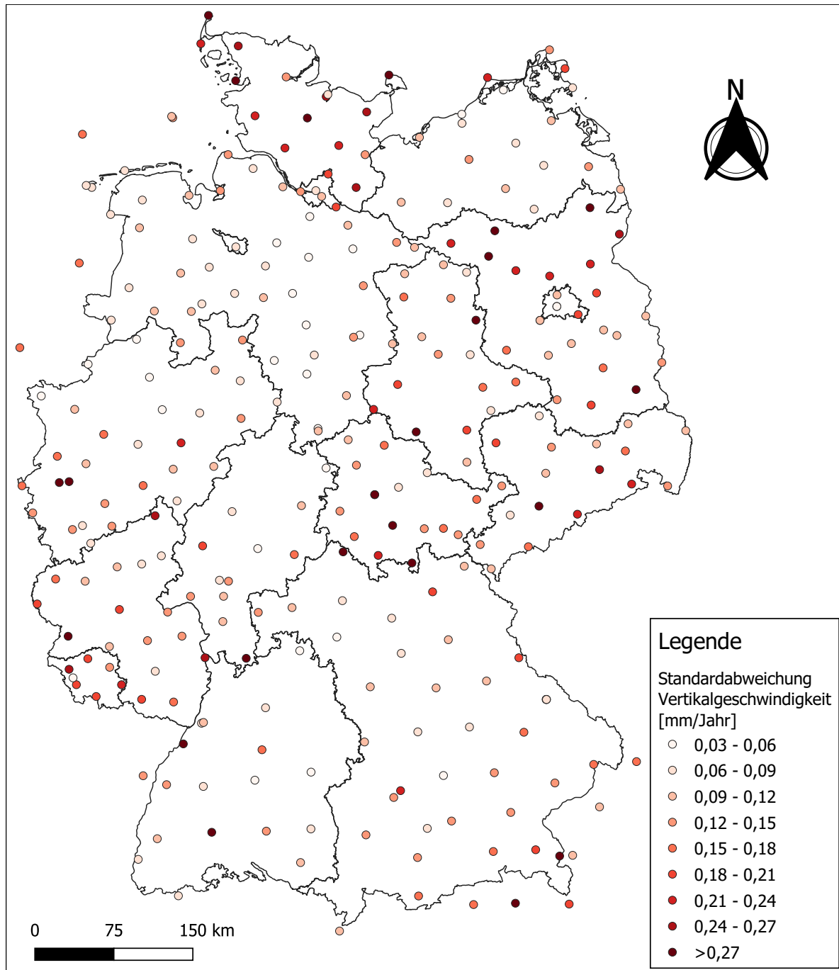
Abbildung 4.12: Standardabweichungen von den Vertikalgeschwindigkeiten der analysierten GNSS-Referenzstationen
