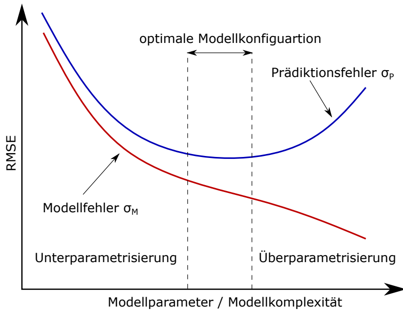
Abbildung 3.9: Verläufe des Prädiktions- und Modellfehlers in Abhängigkeit zur Modellkomplexität (vgl. Esbensen und Geladi, 2010)
