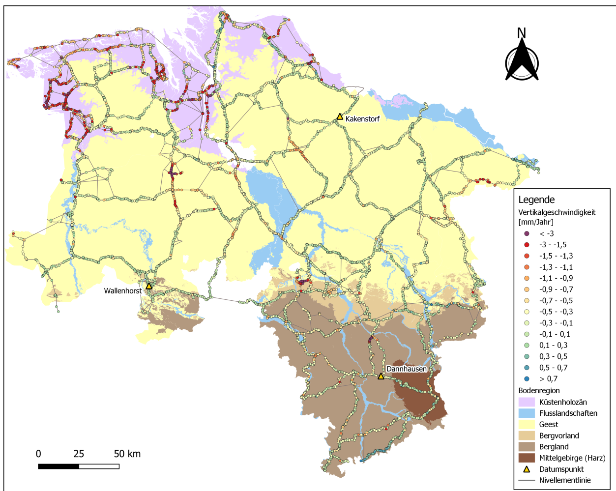
Abbildung 4.22: Vertikalgeschwindigkeiten in Zusammenhang mit geologischen Bodenregionen (vgl. NIBIS® Kartenserver, 2021b)
