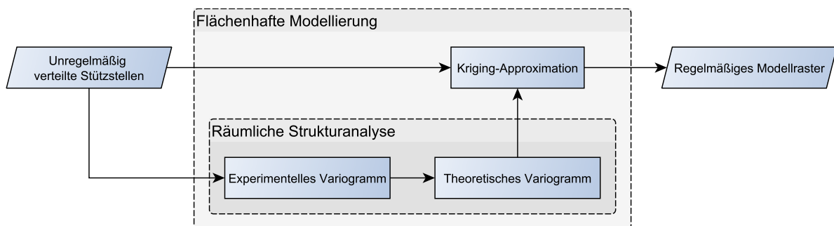
Abbildung 3.5: Ablauf einer geostatistischen Modellierung eines flächenhaften Prozesses
