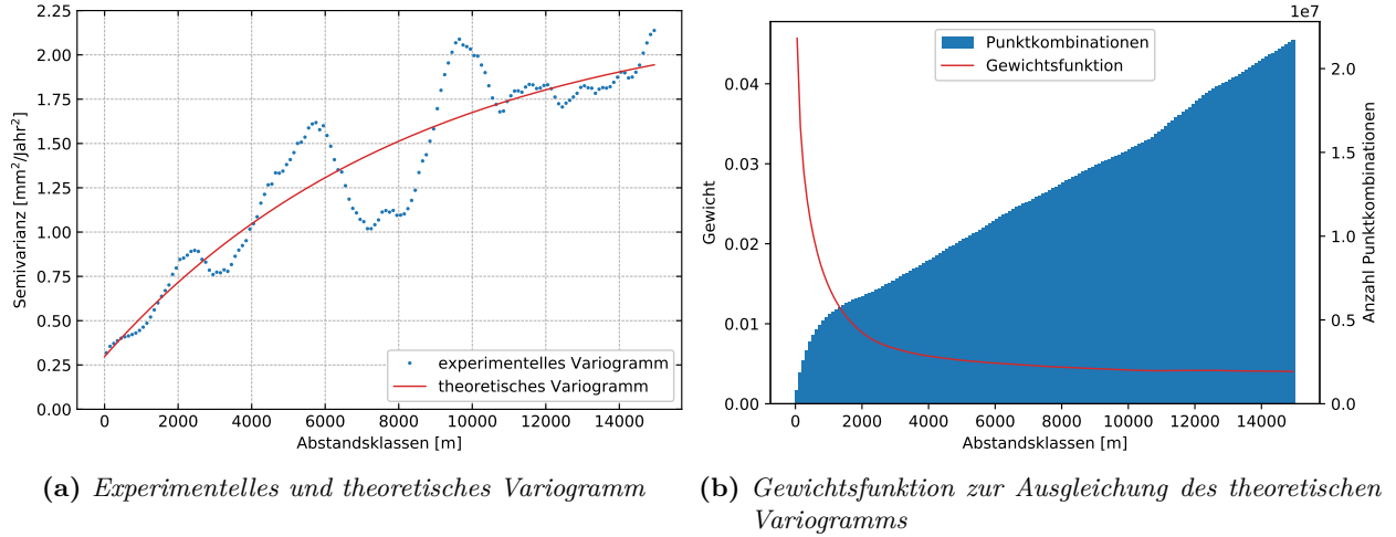
Abbildung 5.6: Räumliche Strukturanalyse für den exemplarischen SAR-Stack 015_01
