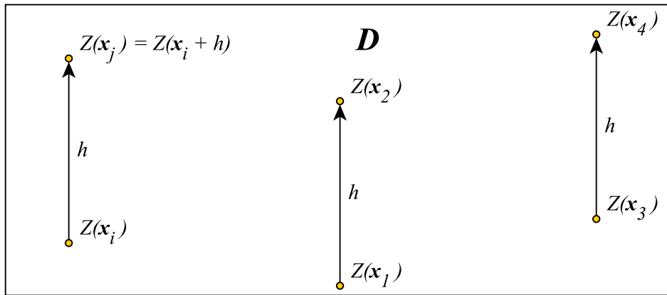
Abbildung 2.8: Untersuchungsgebiet D mit den darin befindlichen ortsabhängigen Zufallsvariablen Z(\mathbf{x}_i) (vgl. Montero u. a., 2015, S. 14)
