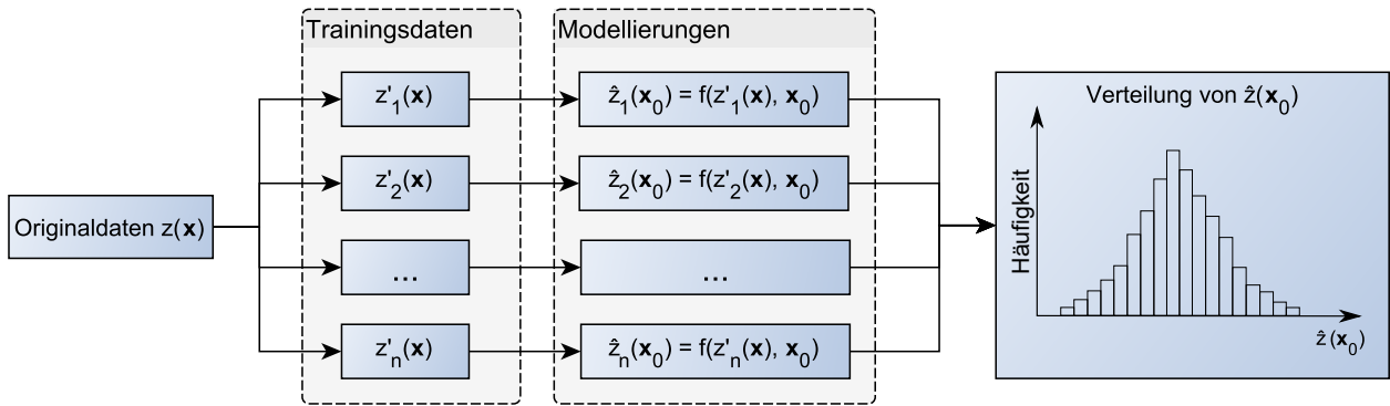
Abbildung 3.10: Allgemeiner Ablauf von Resampling-Verfahren
