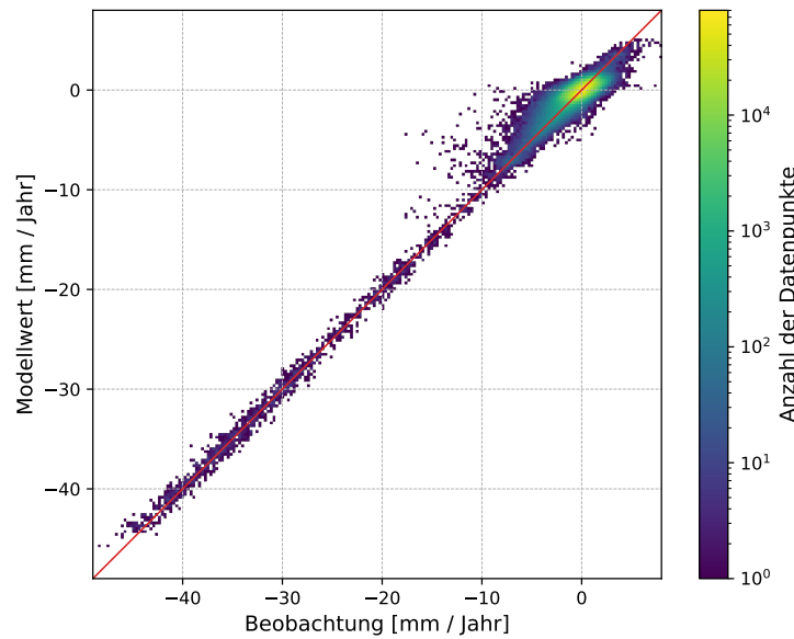
Abbildung 5.8: Vergleich zwischen Beobachtungen und Modellwerten aus Ordinary Kriging
