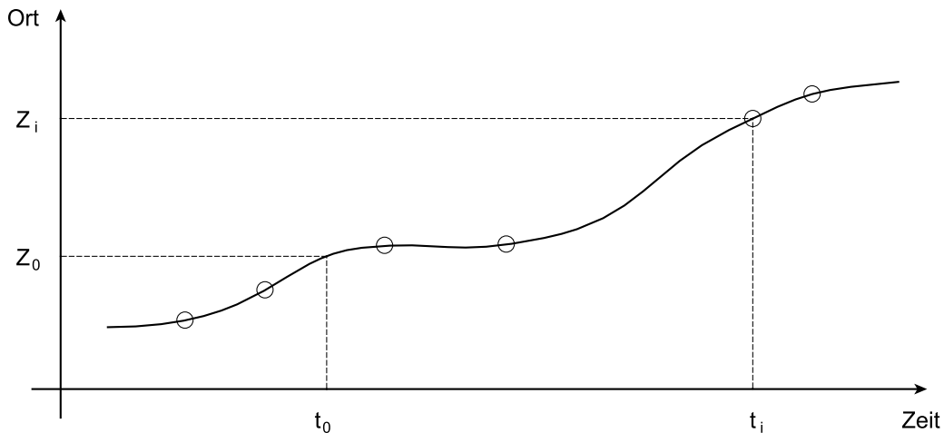
Abbildung 3.1: Ortsänderung eines Objektpunktes im Ablauf der Zeit (vgl. Zippelt, 1988, S. 19)
