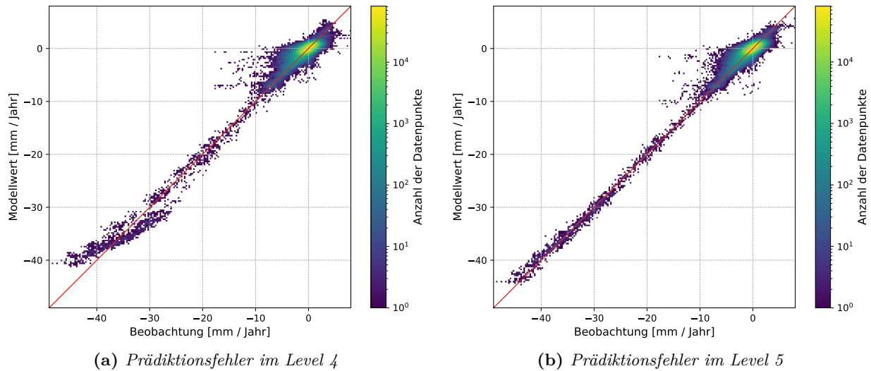
Abbildung 5.3: Vergleich zwischen Beobachtungen und Modellwerten unterschiedlicher MBA
