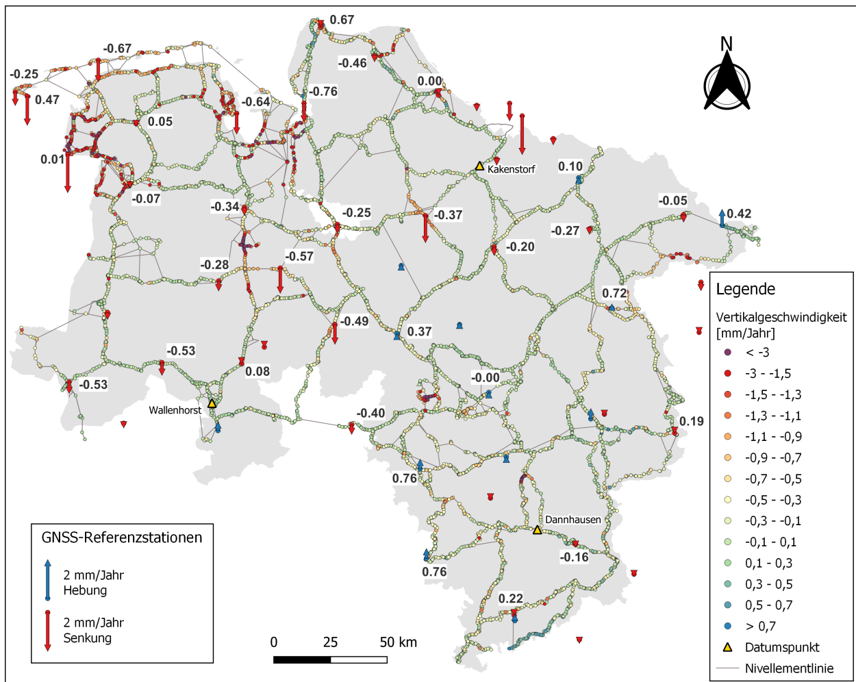
Abbildung 4.25: Differenzen zwischen den finalen Vertikalgeschwindigkeiten aus Nivellement und GNSS-Daten
