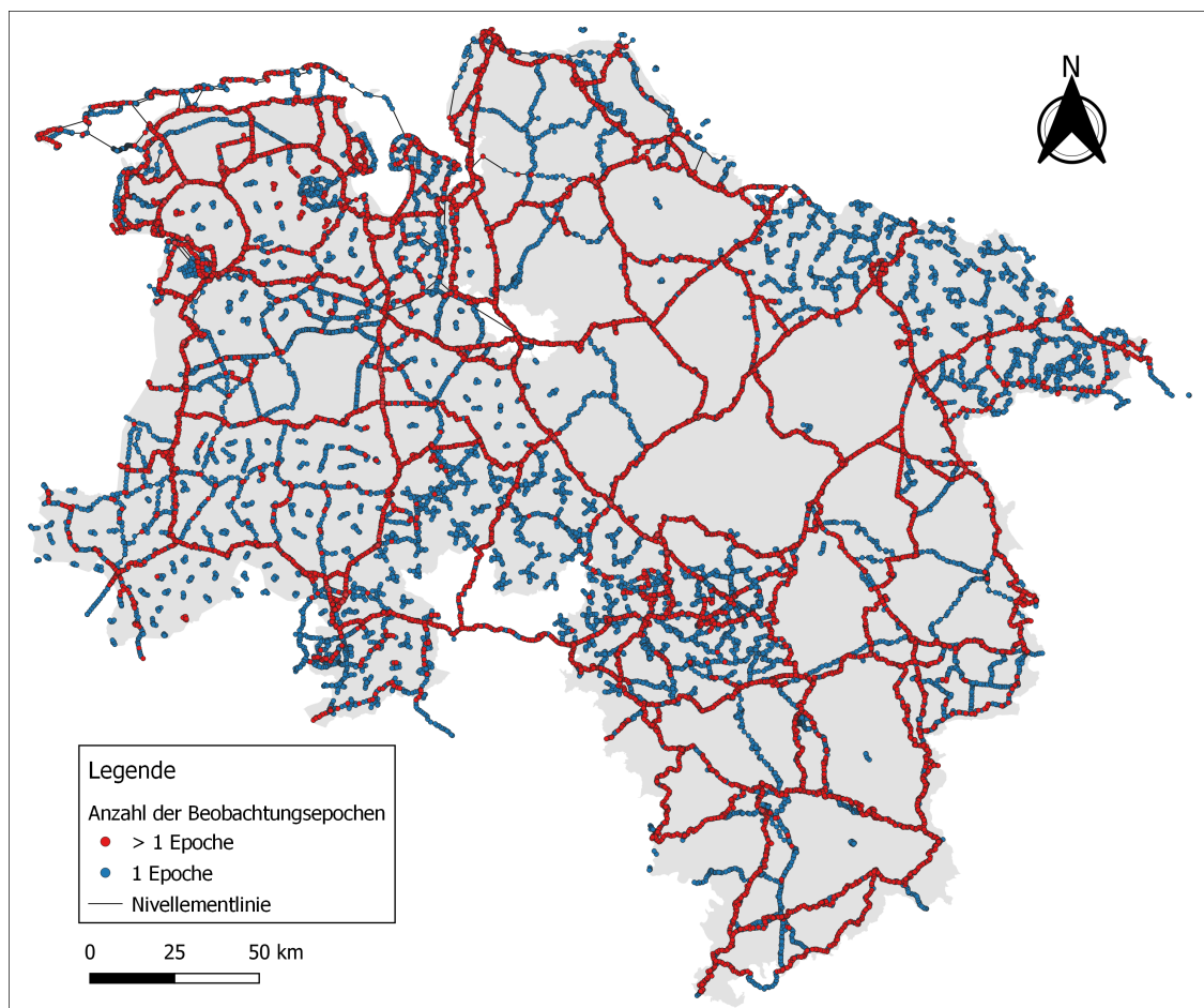
Abbildung 4.13: Nivellementnetz als Datengrundlage zur Ableitung von Vertikalbewegungen
