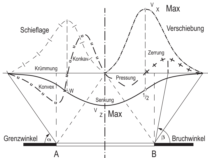
Abbildung 2.3: Elemente der Bodenbewegung über einer Abbaufläche (Kratzsch, 2013)
