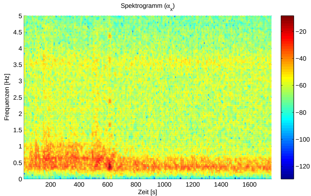
Abb. 3.24: Spektrogramm (Power Spectral Density) für \Delta\omega_{x,MRU}^{B,N}
