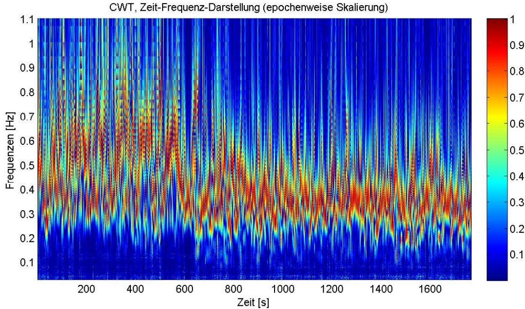
Abb. 3.25: Zeit-Frequenzdarstellung der CWT (frequenzweise Skalierung) für \Delta\omega_{x,MRU}^{B,N} im Frequenzbereich 0,1 – 1,1 Hz
