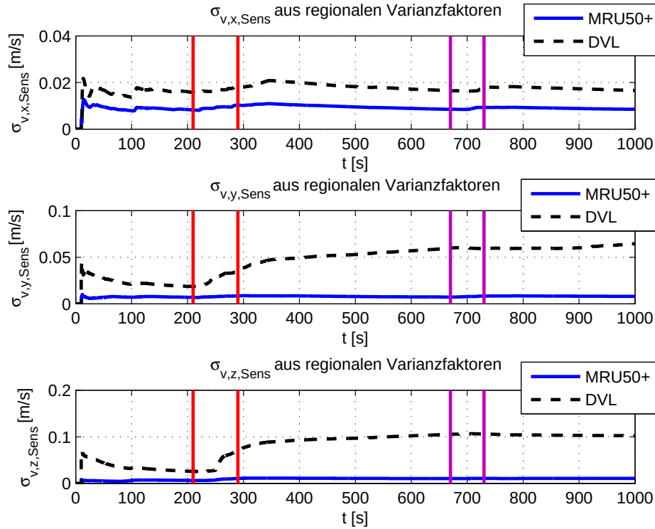
Abb. 5.8: Geschätzte regionale Varianzkomponenten für l_{v,MRU,k+1} und l_{v,DVL,k+1} bei einer Messfahrt mit zwei Wenden
