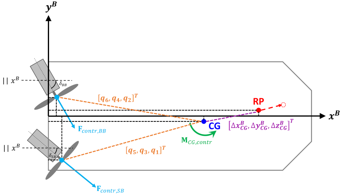
Abb. 4.3: Einfluss eines am Massenschwerpunkt CG wirksamen Drehmoments M_{CG,contr} , resultierend aus den Kraftvektoren F_{contr,SB} und F_{contr,BB} (zwei Propeller), auf das Bewegungsverhalten am Referenzpunkt RP
