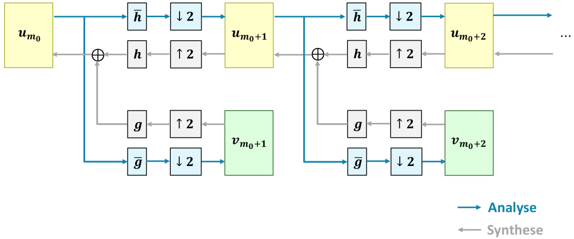
Abb. 3.10: Schnelle Wavelet-Transformation - Analyse und Synthese durch Filterung des Signals (nach Bani 2005; Mallat 2009)
