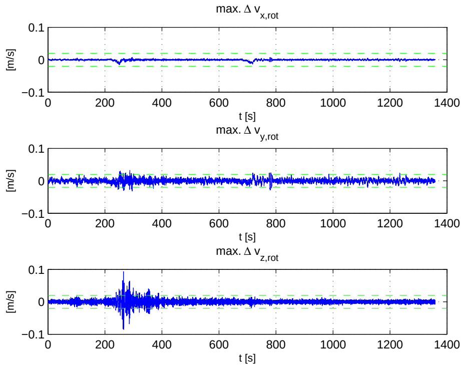
Abb. 5.5: Einfluss von \Delta v_{Rot}^B auf \bar{v}_{k+1}^B für \Delta p_{CG}^B = [15, 48 \text{ m } 3, 87 \text{ m } 1 \text{ m}]^T im Vergleich zur Messgenauigkeit (grüne Linie)
