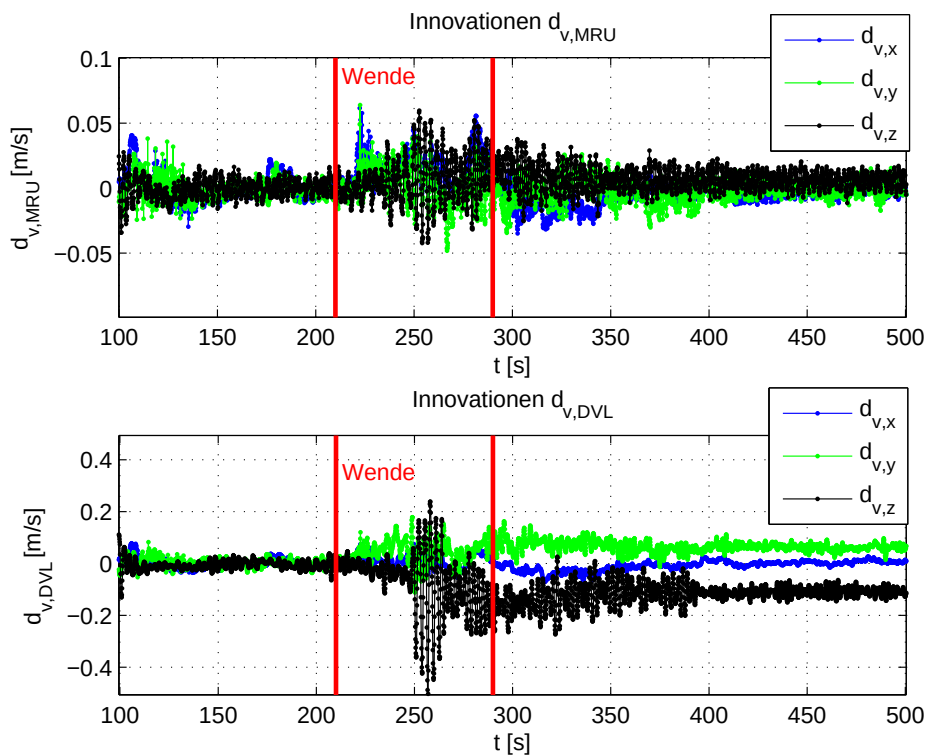
Abb. 5.7: Innovationen bzgl. l_{v,MRU,k+1} und l_{v,DVL,k+1} mit auftauchendem Offset
