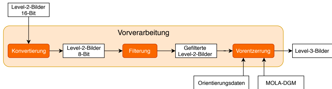
Abbildung 3.3. Ablauf der Vorverarbeitung unterteilt in drei Schritte
