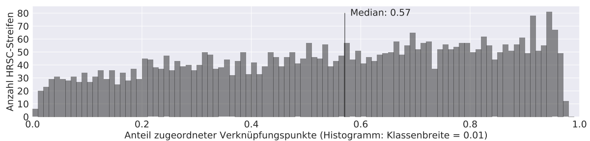
Abbildung 4.17. Zuordnungsquote bei der Verknüpfungspunktbestimmung (Verknüpfungspunkte / Kandidatenpunkte); Histogramm über alle 4 322 HRSC-Streifen; Median: 57 %
