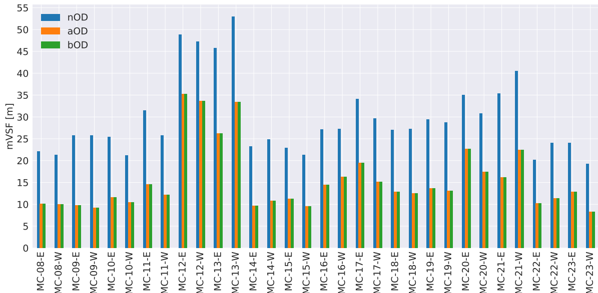
Abbildung 4.51. Mittlerer Vorwärtsschnittfehler (mVSF) für 32 Halbkachelblöcke; blau: nominelle Orientierungsdaten (nOD); orange: ausgeglichenen Orientierungsdaten (aOD); grün: blockausgeglichene Orientierungsdaten)
