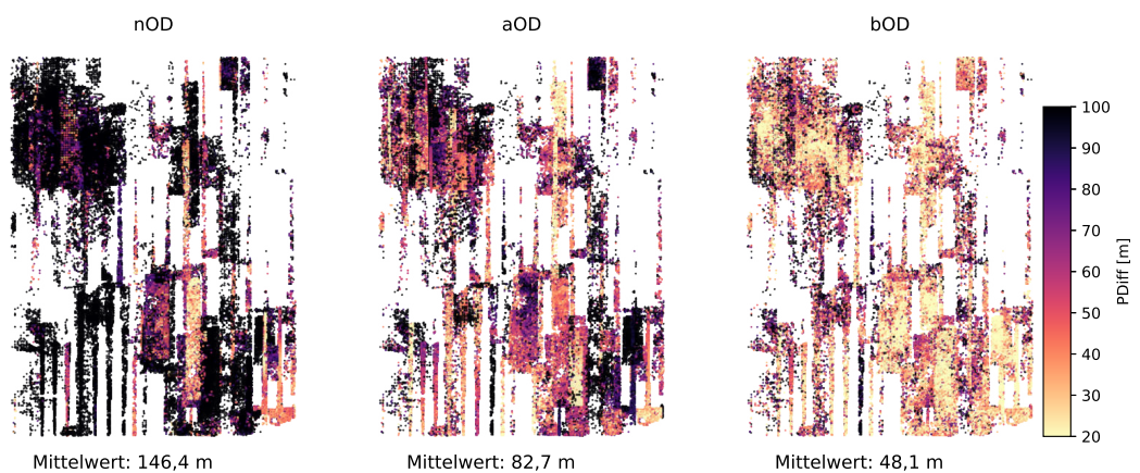
Abbildung 4.45. Distanz zwischen Punkten benachbarter Streifen (PDiff) aus der Evaluierung der HRSC-Objektpunkte mit unterschiedlichen Orientierungsdaten (nOD, aOD und bOD)
