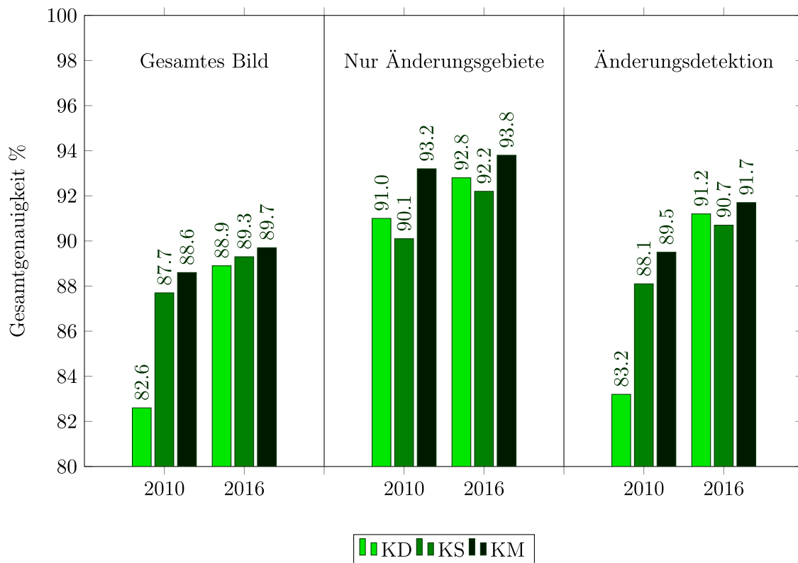
Abbildung 61: Gesamtgenauigkeit [%]. Datensatz: Hameln , Multitemporal, Karte: 1955.
