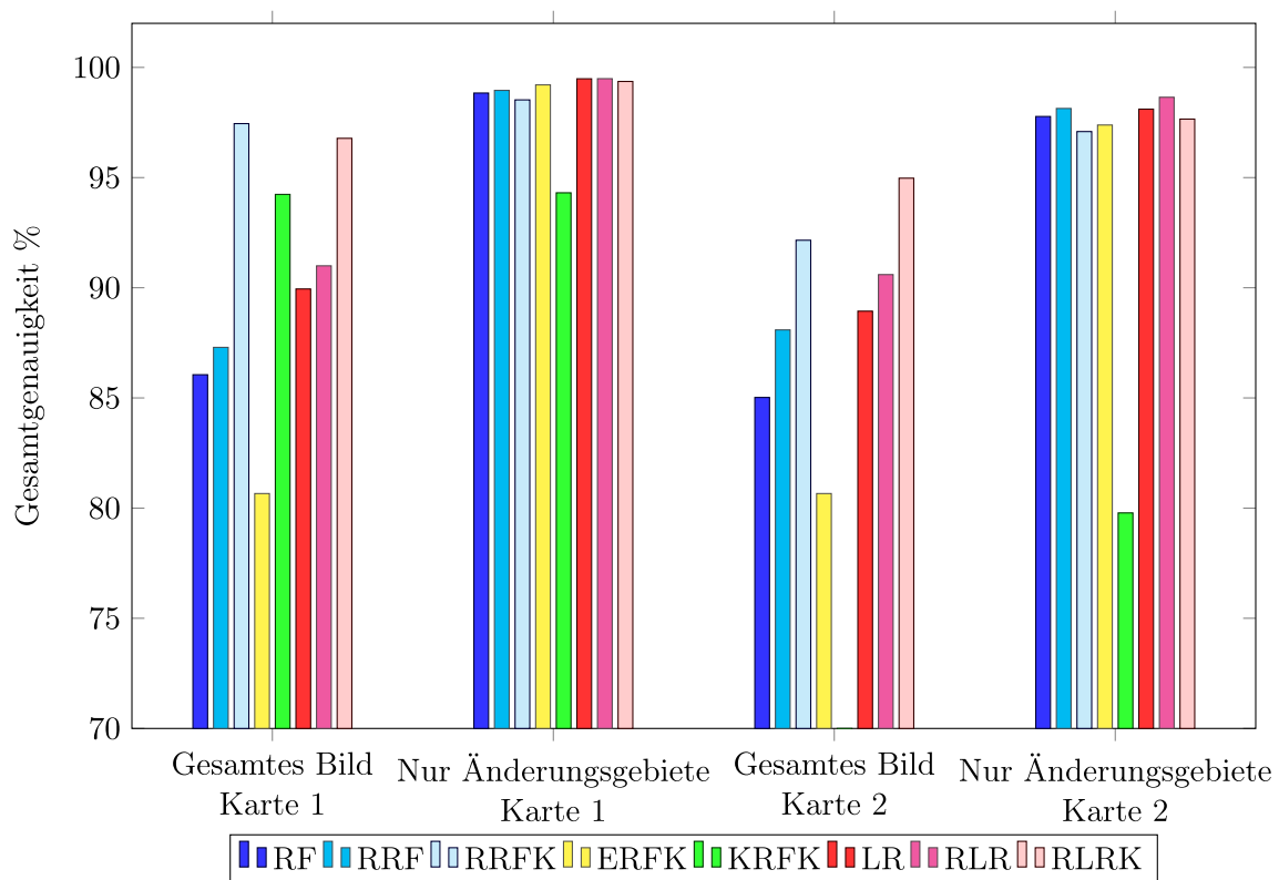
Abbildung 58: Gesamtgenauigkeit [%]. Datensatz: Husum .
