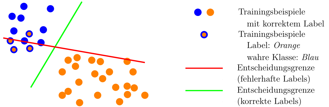
Abbildung 7: Beispiel für die Auswirkung von fehlerhaften Trainingsbeispielen auf die Klassifikation von zwei Klassen ( Blau und Orange ) in einem zweidimensionalen Merkmalsraum. Die rote Entscheidungsgrenze erreicht einen höheren Informationszuwachs als die grüne Entscheidungsgrenze. Die grüne Entscheidungsgrenze trennt die wahren Labels jedoch besser.
