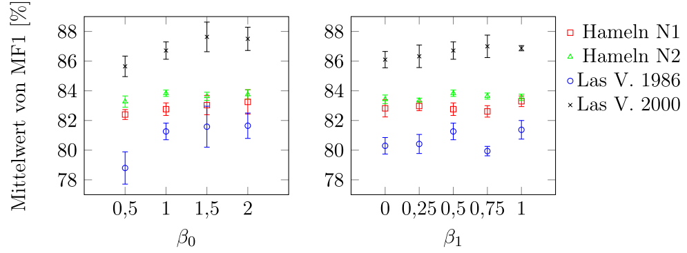
Abbildung 29: Mittelwert von MF1 [%] abhängig von je einem Parameter ( \beta_0 , \beta_1 ) des kontrastsensitiven Potts-Modells.
