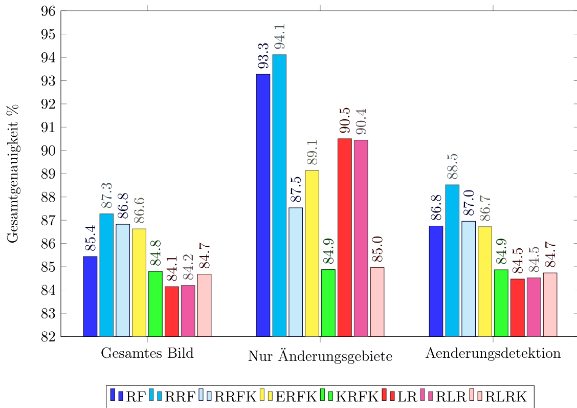
Abbildung 35: Gesamtgenauigkeit [%]. Datensatz: Hameln (N2).
