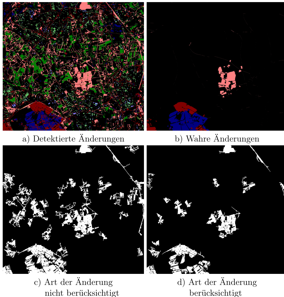
Abbildung 11: Vergleich des Änderungsbildes B abhängig davon, ob die Art der Änderung bei der Bestimmung des Änderungsbildes B berücksichtigt wurde.
