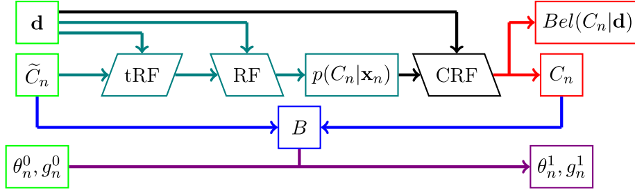
Abbildung 5: Initialisierungsprozess für den RRFK basierend auf dem RF. Rechteckige Boxen: Variablen. Parallelogramme: Prozesse. Parallelogramm mit spitzem Winkel oben rechts: Trainingsprozess. Die Farben in der Abbildung werden im Text aufgegriffen.
