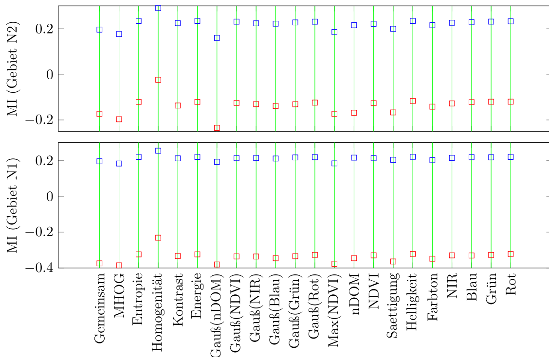
Abbildung 21: MI für die erste Iteration. Oben - MI für Gebiet N2 des Datensatzes Hameln . Unten - MI für Gebiet N1 des Datensatzes Hameln . X-Achse: nicht verwendetes Merkmal. Rot: Verwendung der veralteten Karte. Blau: Verwendung der Referenz.
