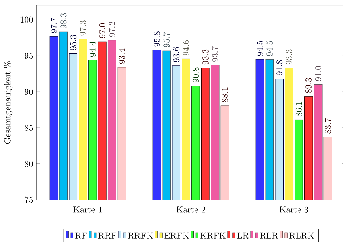
Abbildung 52: Gesamtgenauigkeit [%]. Datensatz: Vaihingen . Grundlage: Nur Änderungsgebiete.
