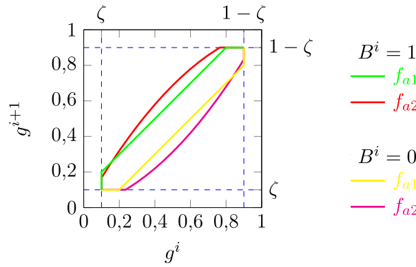
Abbildung 12: Zwei Aktualisierungsfunktionen f_{a1} und f_{a2} der Änderungswahrscheinlichkeit g .
