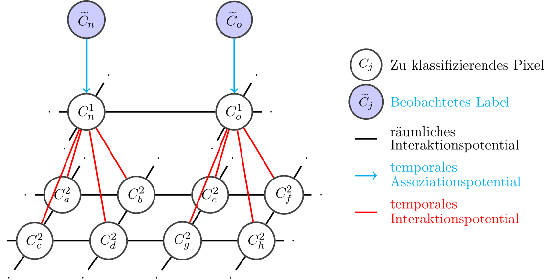
Abbildung 15: Graphenstruktur des CRF für die Klassifikation von zwei Bildern aus unterschiedlichen Zeitpunkten unter Berücksichtigung der Labels einer veralteten Karte. Die Auflösung des Bildes zum Zeitpunkt z = 2 ist doppelt so hoch wie die des Bildes aus z = 1 . Die Daten \mathbf{d}^1 und \mathbf{d}^2 sind nicht abgebildet.
