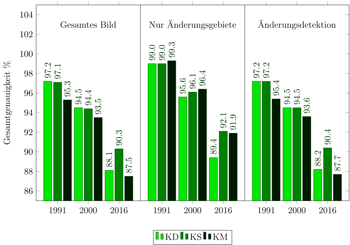
Abbildung 63: Gesamtgenauigkeit [%]. Datensatz: Las Vegas, Multitemporal, Karte: 1986.
