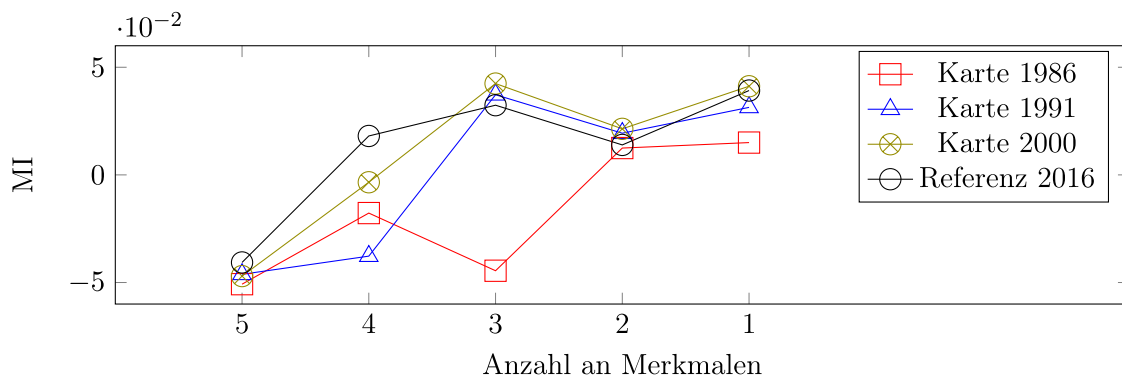
Abbildung 23: MI von Las Vegas abhängig von der Anzahl an verbleibenden Merkmalen.
