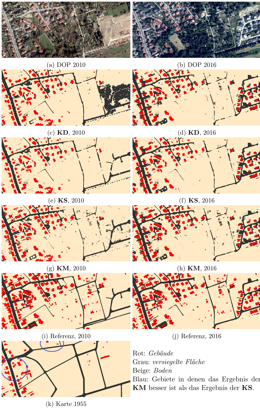
Abbildung 62: Ausschnitt aus dem Gebiet NA des Datensatzes Hameln , in dem sich auch Gebiet N1 befindet, für welchen eine Referenz vorliegt.
