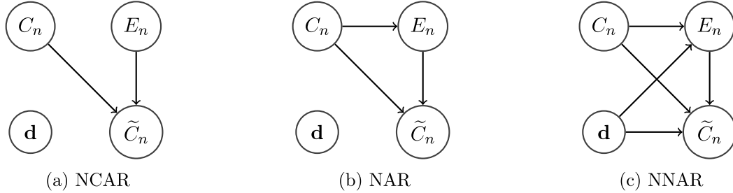
Abbildung 1: Statistische Zusammenhänge zwischen den Daten \mathbf{d} , dem wahren Label C_n , dem Auftreten eines Fehlers E_n und dem potentiell fehlerhaften Label \tilde{C}_n an einem Primitiv n für die drei Modelle Noise Completely At Random (NCAR), Noise At Random (NAR) und Noise Not At Random (NNAR). Der Zusammenhang zwischen den Daten \mathbf{d} und dem wahren Label C_n ist für eine bessere Übersicht nicht dargestellt [Frénay und Verleysen, 2014].
