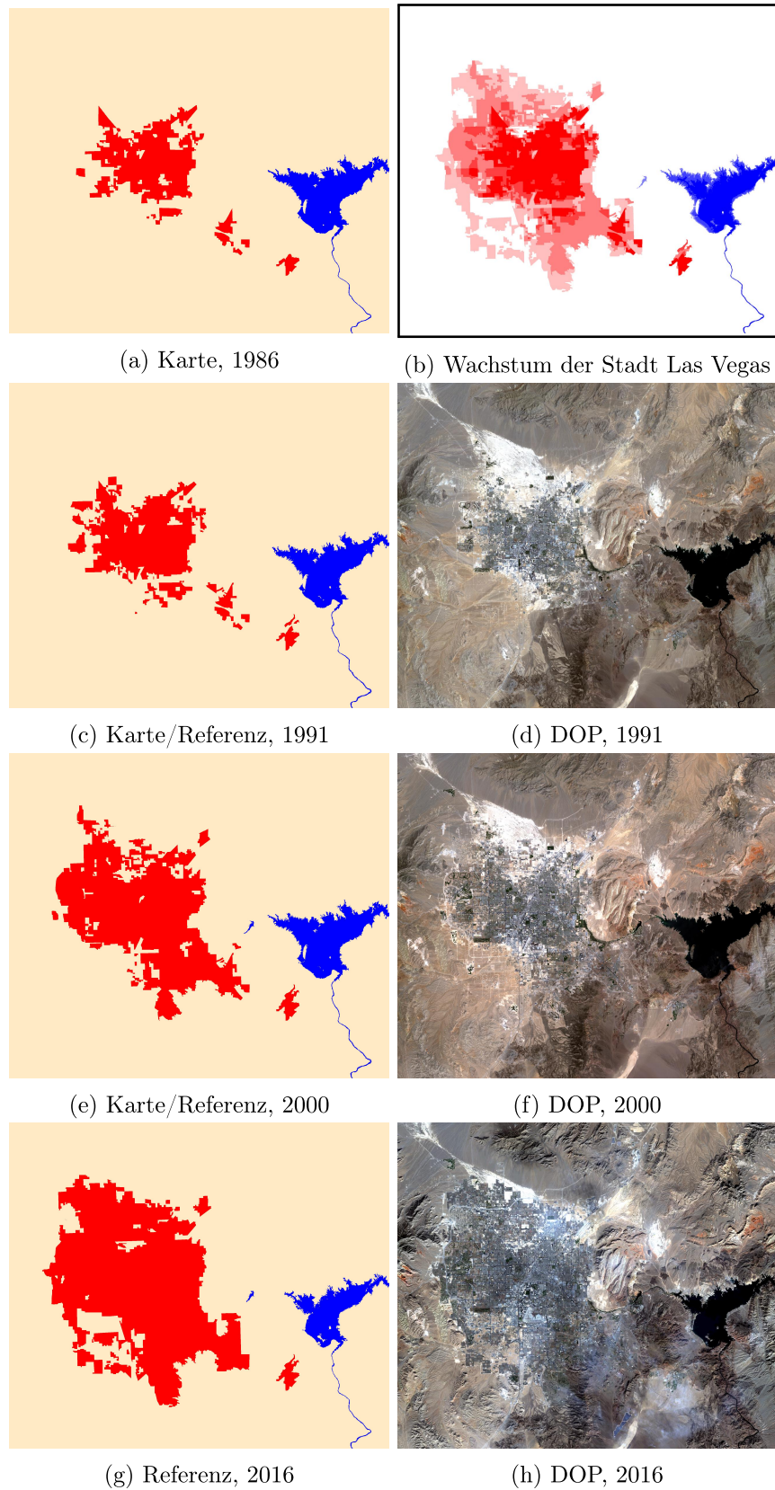
Abbildung A.3: DOPs, Referenzen und Karte des Datensatzes Las Vegas .
