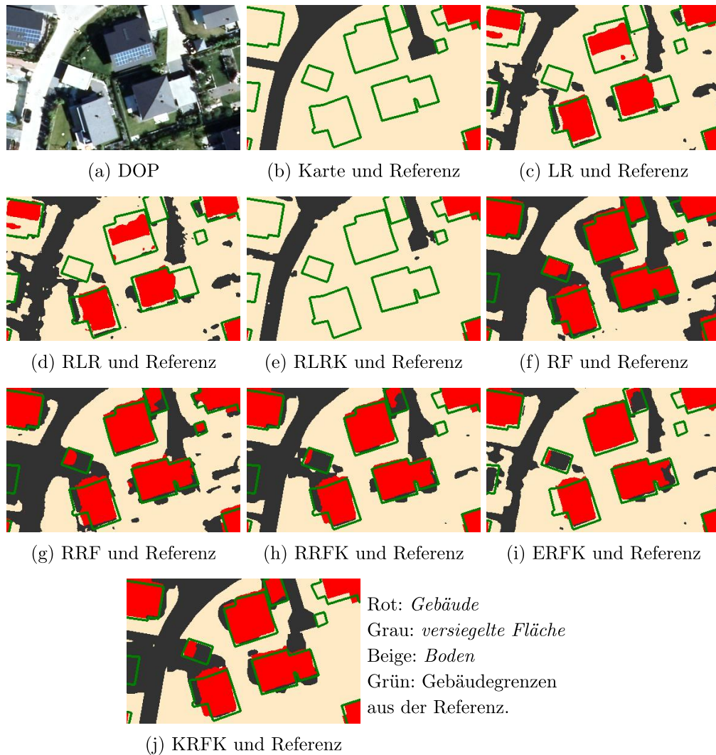
Abbildung 37: Ausschnitt aus Gebiet N1 des Datensatzes Hameln mit neuen Gebäuden.
