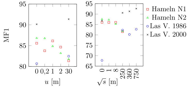
Abbildung 33: MF1 [%] abhängig von den Parametern u (minimale Breite der Segmente) und s (minimale Größe der Segmente).
