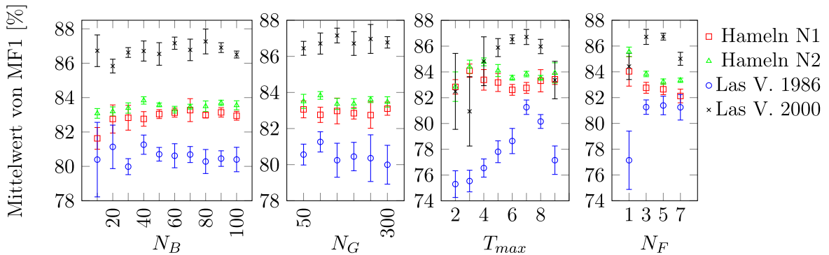
Abbildung 28: Mittelwert von MF1 [%] abhängig von je einem Parameter ( N_B , N_G , T_{max} , N_F ) des Random Forest.
