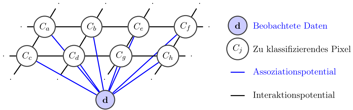
Abbildung 4: Graphenstruktur des klassischen CRF für die Klassifikation eines Bildes aus einem Zeitpunkt nach [Förstner, 2013].
