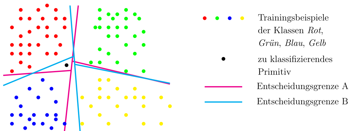
Abbildung 3: Zwei mögliche Aufteilungen eines 2D Merkmalsraumes mit Hilfe des CART Algorithmus (A und B) in die Klassen Rot , Grün , Blau und Gelb . Das unklassifizierte Primitiv (schwarzer Punkt) wird, abhängig von dem gewählten Baum, entweder der Klasse Rot oder Blau zugeordnet.
