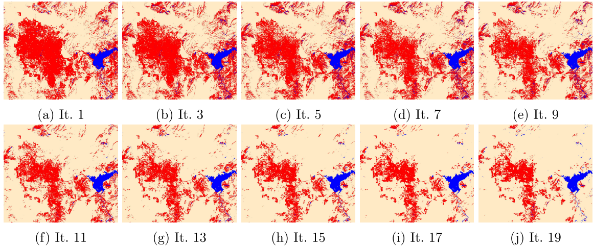
Abbildung 32: Klassifikationsergebnis des Datensatzes Las Vegas abhängig von der Anzahl der Iterationen (Abkürzung für Iteration: It.). Die Karte stammt aus 1986. Rot: Bebauung . Blau: Wasser . Beige: Boden .
