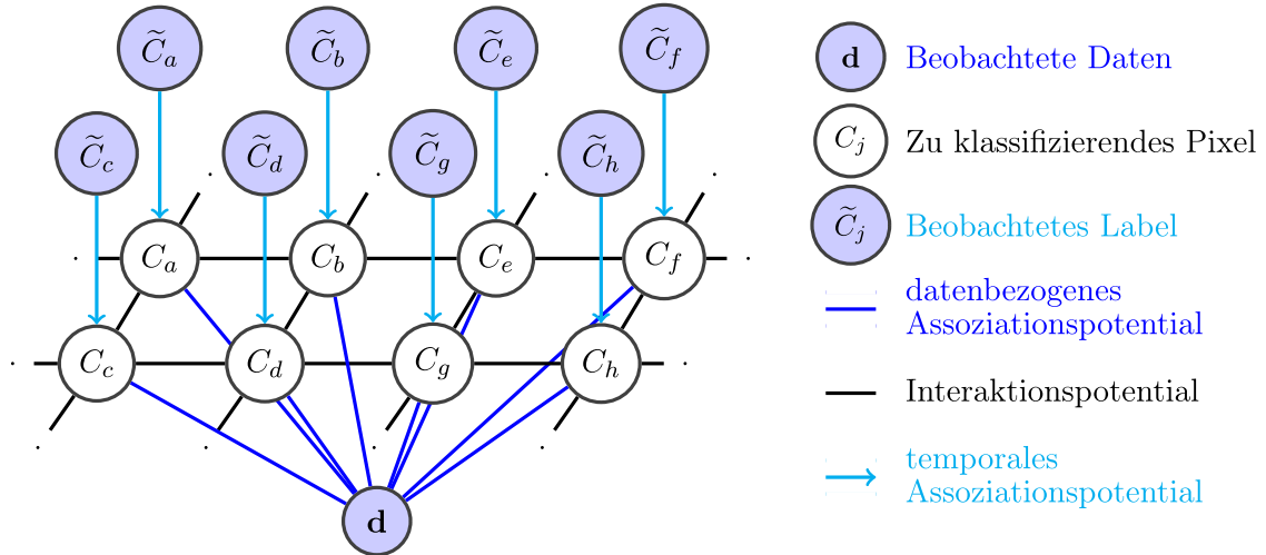
Abbildung 9: Graphenstruktur des CRF für die Klassifikation eines Bildes aus einem Zeitpunkt unter Berücksichtigung der Labels einer veralteten Karte.
