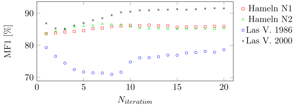
Abbildung 30: MF1 [%] abhängig von der Anzahl der Iterationen des iterativen Klassifikationsprozesses.
