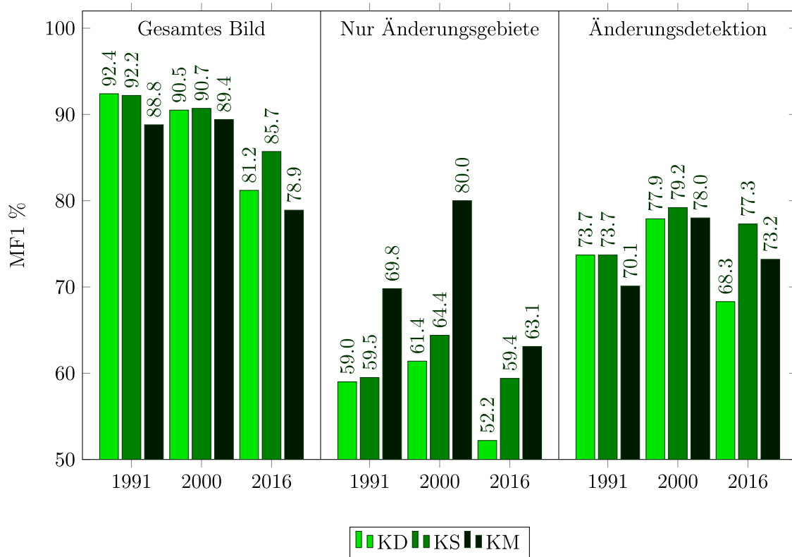
Abbildung 64: MF1 [%]. Datensatz: Las Vegas , Multitemporal, Karte: 1986.
