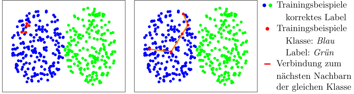
Abbildung 20: Trainingsbeispiele mit fehlerhaftem Label, die im Merkmalsraum Ballungen bilden (links) und zufälliges Auftreten fehlerhafter Labels (rechts). Die orangefarbenen Linien zeigen für jedes fehlerhaft gelabelte Trainingsbeispiel den nächsten Nachbarn der gleichen Klasse. Bilden die fehlerhaften Trainingsbeispiele Ballungen, ist auch bei diesen Trainingsbeispielen diese Distanz relativ klein und somit die orangefarbene Linie sehr kurz.
