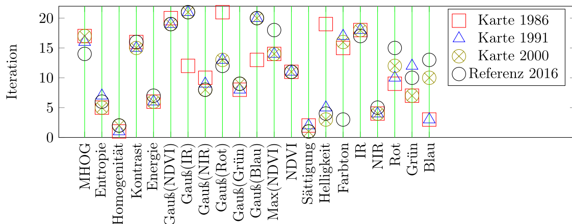
Abbildung 24: Iteration, in dem Merkmal aus der Liste entfernt wurde. Ein hoher Wert deutet auf ein wichtiges Merkmal hin. Datensatz: Las Vegas .
