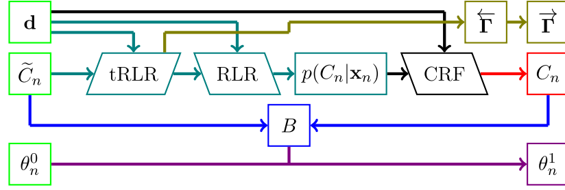
Abbildung 13: Initialisierungsprozess für die RLRL basierend auf der RLR. Rechteckige Boxen: Variablen. Parallelogramme: Prozesse. Parallelogramm mit spitzem Winkel oben rechts: Trainingsprozess. Die Farben in der Abbildung werden im Text aufgegriffen.
