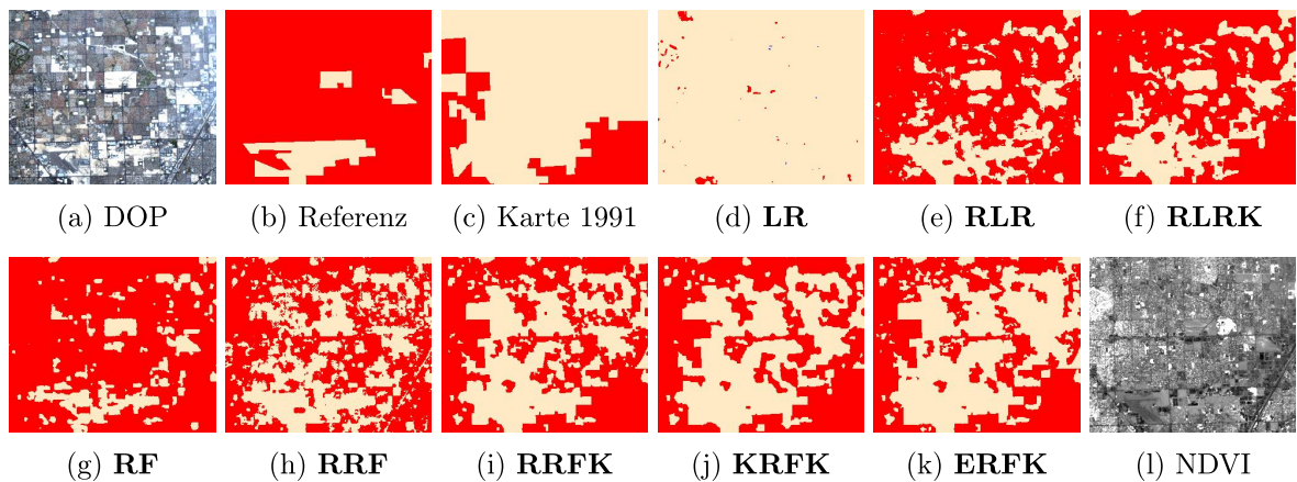
Abbildung 47: Ausschnitt aus dem Datensatz Las Vegas mit einem Neubaugebiet. Karte von 1991. Rot: Bebauung . Blau: Wasser . Beige: Boden .
