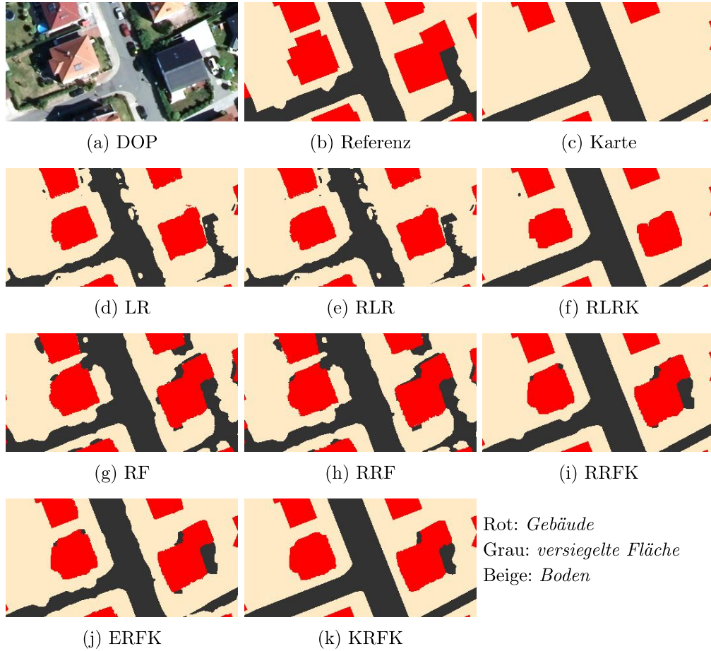
Abbildung 39: DOP und Ergebnisse eines Ausschnittes des Gebietes N2 des Datensatzes Hameln , in dem die zwei neuen Gebäude in Gebiet N2 enthalten sind.
