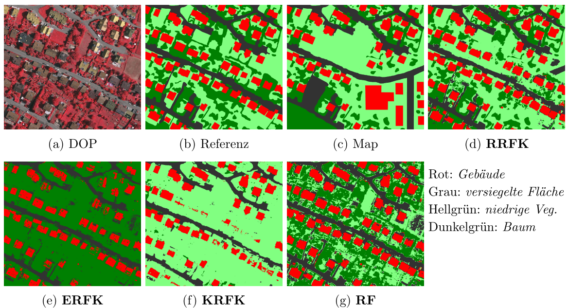
Abbildung 56: Gebiet A13 aus Vaihingen . Karte 3 (28,8% Änderungen).
