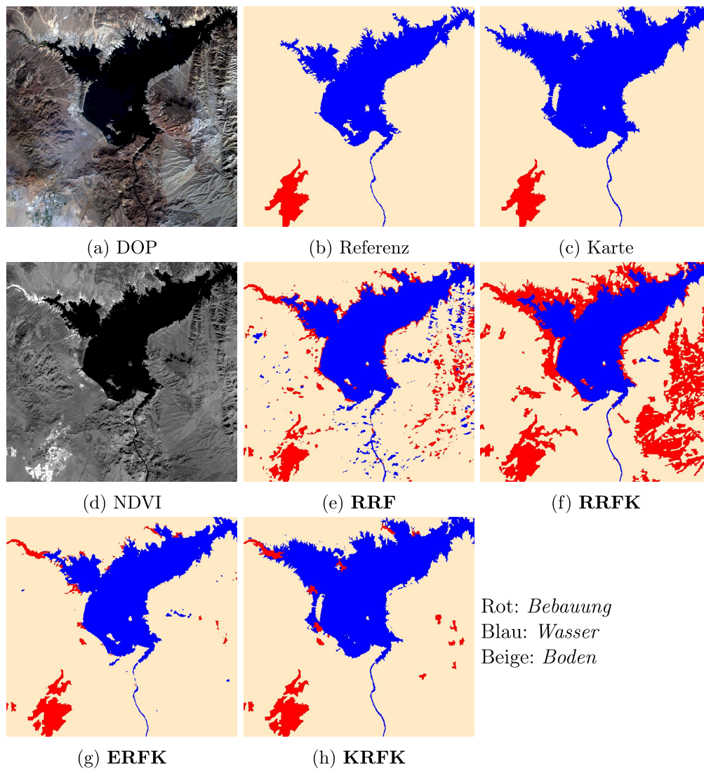
Abbildung 50: Ausschnitt aus Las Vegas mit einem Seegebiet. Karte von 2000.
