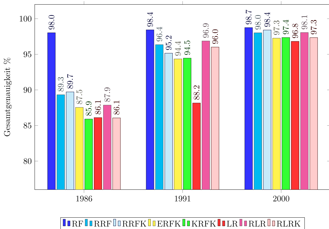
Abbildung 45: Gesamtgenauigkeit [%]. Datensatz: Las Vegas . Grundlage: Nur Änderungsgebiete.
