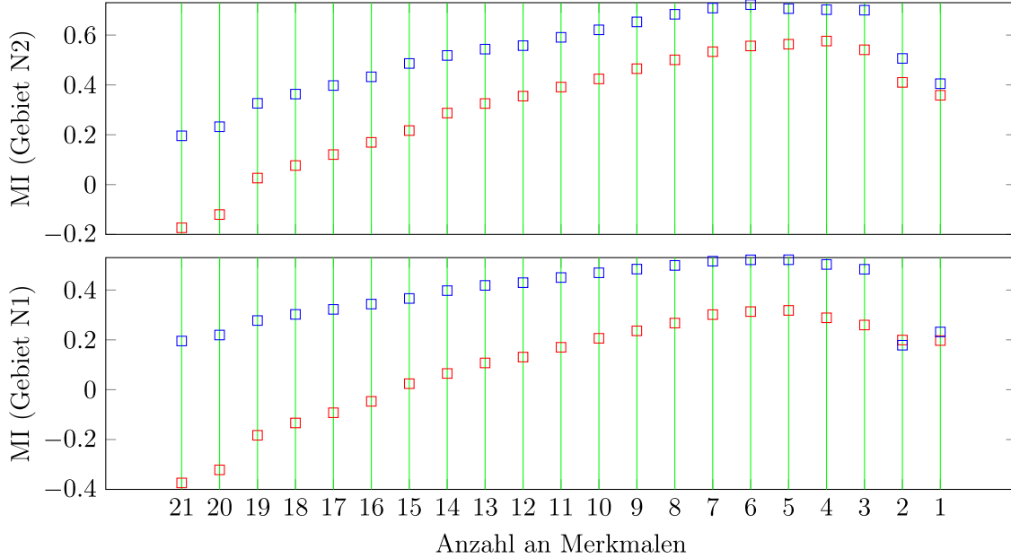
Abbildung 22: MI abhängig von der Anzahl der verbleibenden Merkmale. Oben - MI für Gebiet N2 des Datensatzes Hameln . Unten - MI für Gebiet N1 des Datensatzes Hameln .
