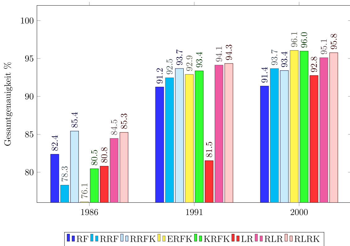
Abbildung 44: Gesamtgenauigkeit [%]. Datensatz: Las Vegas . Grundlage: Gesamtes Bild.
