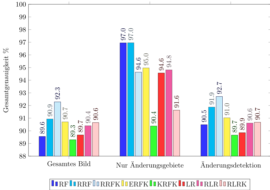
Abbildung 34: Gesamtgenauigkeit [%]. Datensatz: Hameln (N1).
