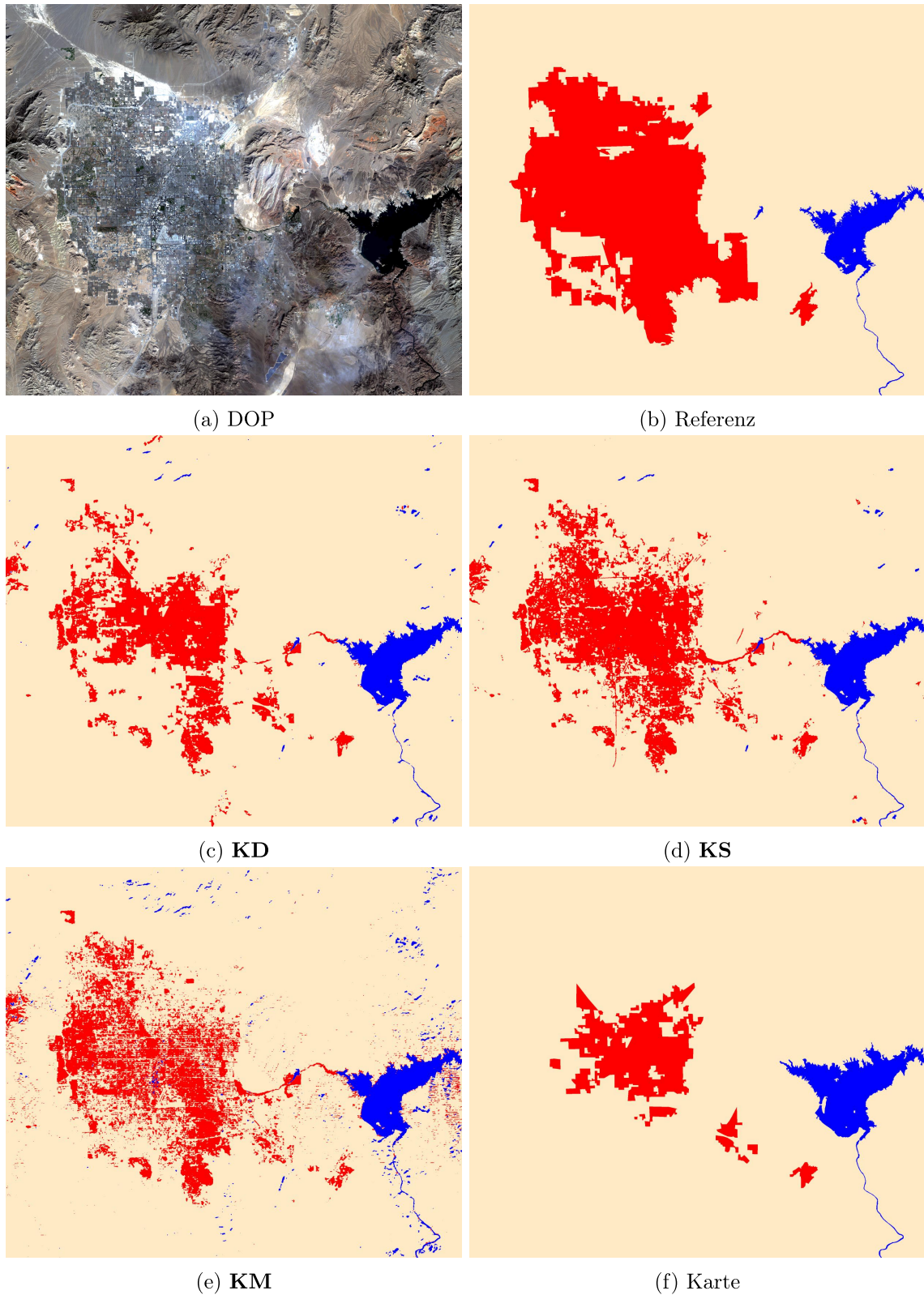
Abbildung 66: DOP, Referenz und Ergebnisse für das Jahr 2016 des Datensatzes Las Vegas und die verwendete Karte aus dem Jahr 1986. Rot: Bebauung . Blau: Wasser . Beige: Boden .
