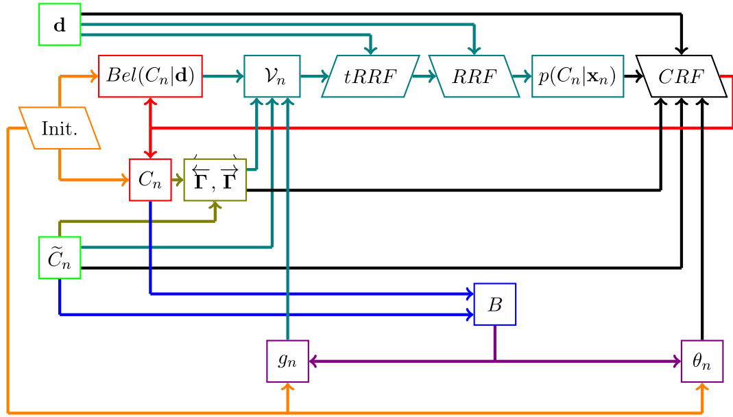
Abbildung 6: Iterativer Prozessablauf des RRFK . Rechteckige Boxen: Variablen. Parallelogramme: Prozesse. Parallelogramm mit spitzen Winkel oben rechts: Trainingsprozess. Init: Initialisierungsprozess. Die Farben in der Abbildung werden im Text aufgegriffen.
