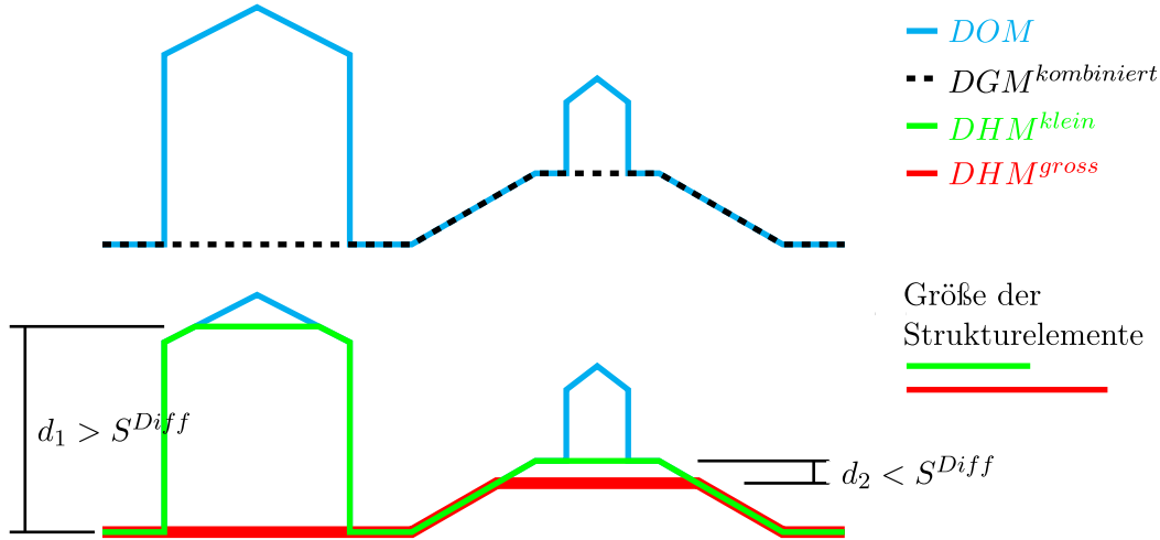
Abbildung 2: Erstellung eines DGMs aus einem DOM mit Hilfe zweier Opening-Operationen mit unterschiedlich großen Strukturelementen.
