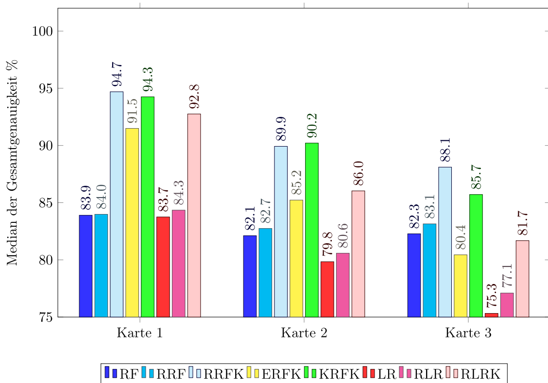
Abbildung 51: Median der Gesamtgenauigkeit über alle Gebiete [%]. Datensatz: Vaihingen . Grundlage: Gesamtes Bild.
