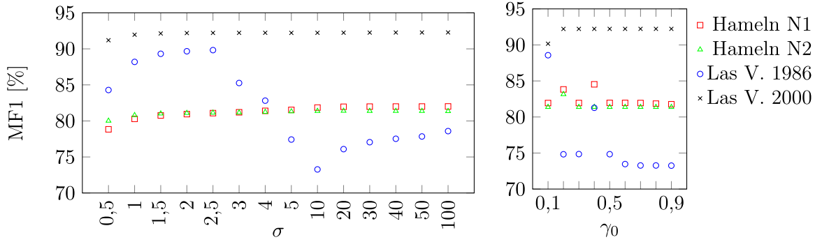
Abbildung 26: MF1 [%] abhängig von je einem Parameter ( \sigma , \gamma_0 ) der robusten logistischen Regression.
