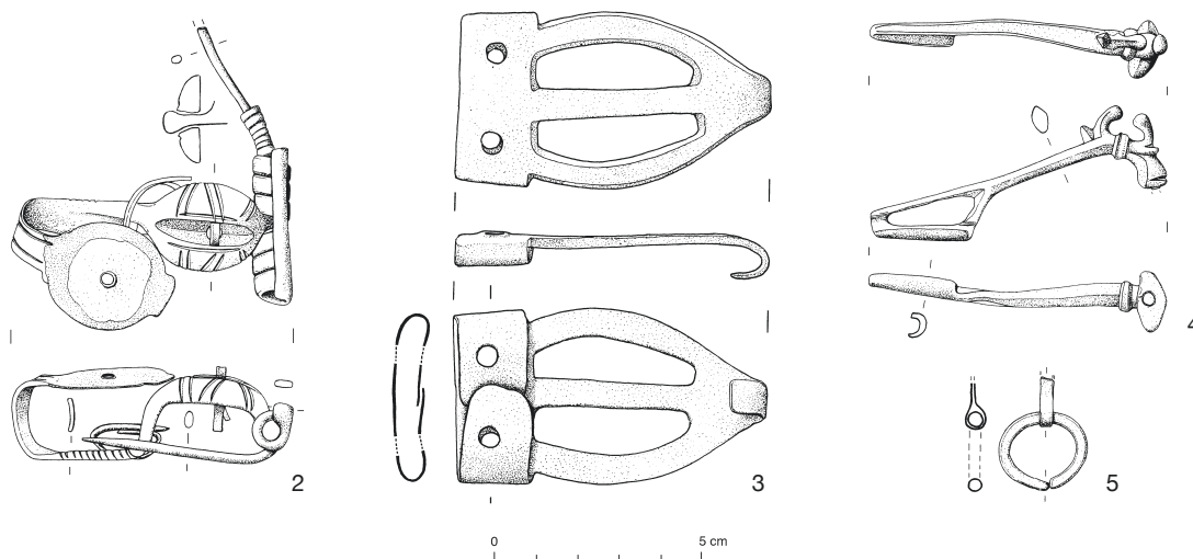
Abb. 4. Ampass-Demlfeld, Sprossengürtelhaken mit eingehängten Fibeln. – Bronze. – 2–5 M. 1:2.
