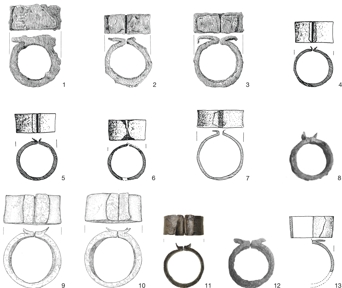
Abb. 8. Stockringe. 1–3 Faggen-Kiahbichl. – 4–8 Volders-Himmelreich. – 9–10 Gurgltal (zwischen Strad und Nassereith). 11 Ehrwald-Loisachtal. – 12 Oberperfuss-Birgl. – 13 Tulfes-Burkt. Vgl. Tab. 1 . – Eisen. – M. 1:4.
