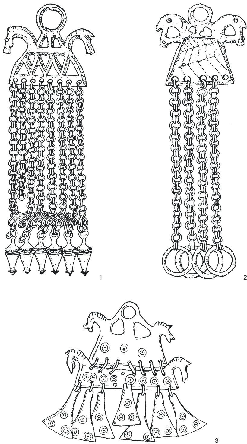
Abb. 3. Anthropomorphe Darstellungen mit antithetischen Pferdeprotomen aus dem Liburnisch-Japodischen Raum; alle aus Bronze: 1–2 Jezerine; 3 Vinica. – M. 2:3.
