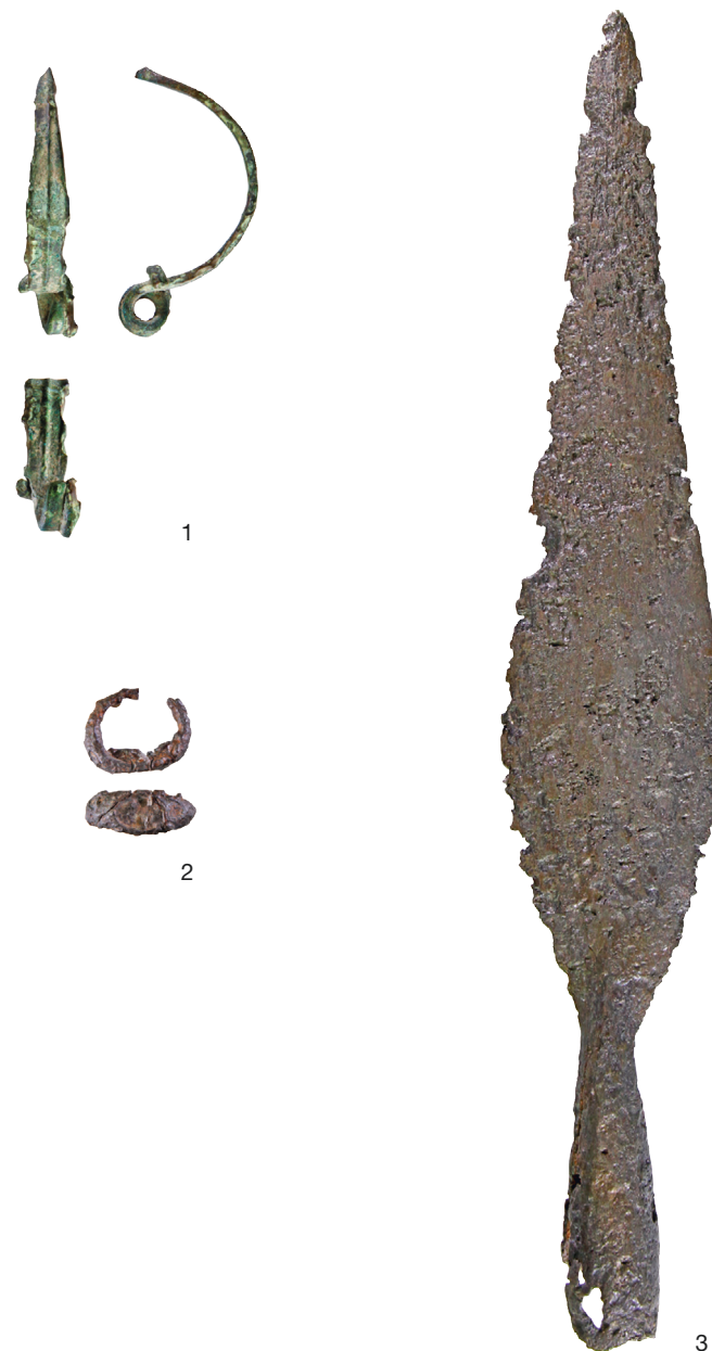
Abb. 5. Ehrwald (Tirol). Funde aus dem 1954 entdeckten Grab. – 1 M. 2:3; 2–3 M. 1:2.
