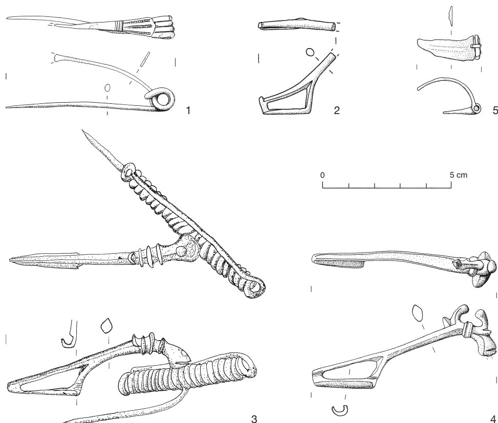
Abb. 2. Ampass-Demlfeld, Fibelfunde des 1. Jahrhunderts v. Chr. – Bronze. – M. 2:3.
