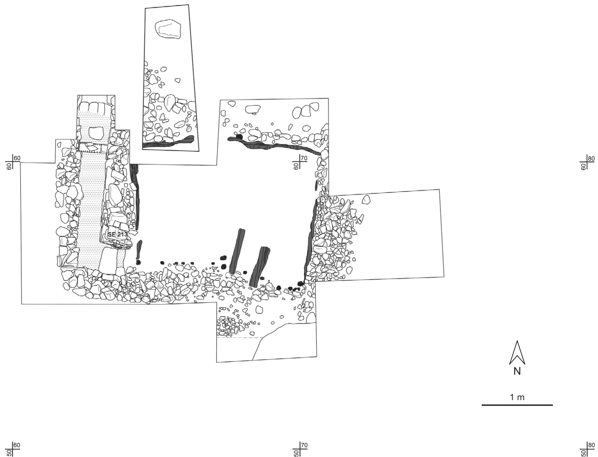
Abb. 7. Stams. Haus 3, zweidimensionale photogrammetrische Aufnahme. An der hangseitigen Rückwand wurden in knappem Abstand vertikale Bauhölzer gesetzt, die eine Bretterwand stützten.
