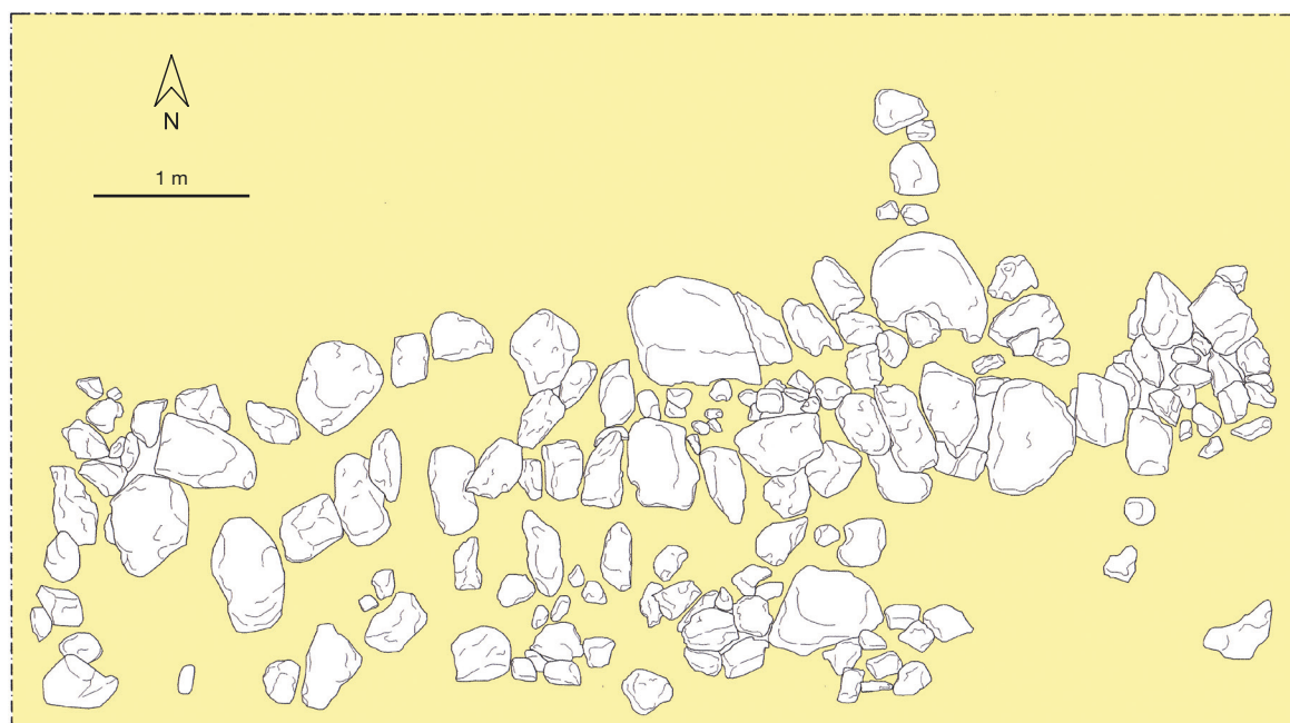
Abb. 4. Stams. Schnitt I, steingerechte Aufnahme der bogigen Terrassierungsmauern. Am rechten Ende der Mauern befindet sich das noch mit Steinen verfüllte Pfostenloch eines mutmaßlichen Tropaions.
