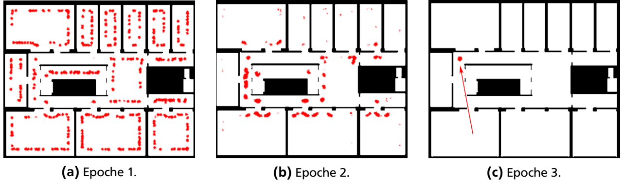
Abbildung 2.4.: Drei Epochen einer Partikelfilterzustandsschätzung im Gebäude B auf dem Campus der Hochschule Karlsruhe (HSKA).
