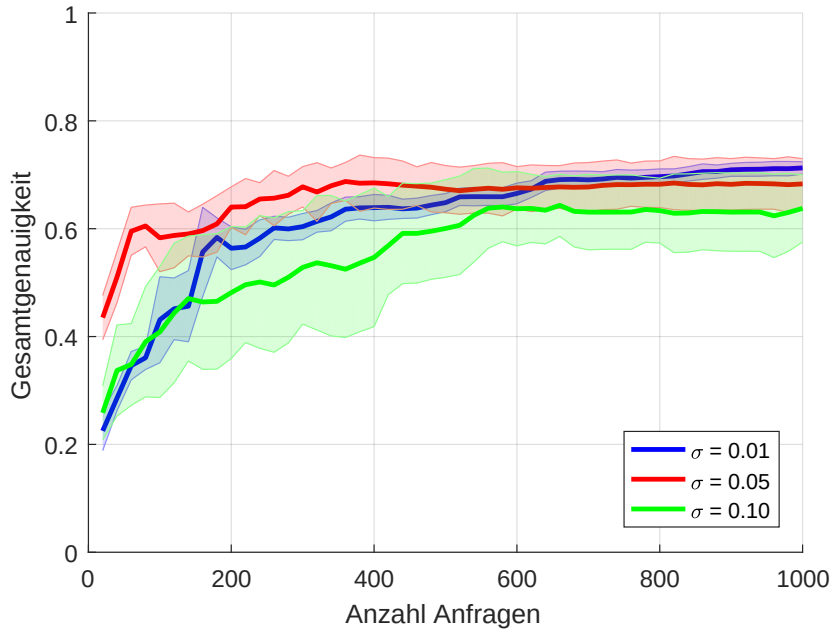
Abbildung 6.5: Der Parameter \sigma steuert die Größe des Einflussbereichs der einzelnen Repräsentantenvektoren (Abbildung nach [Wuttke et al., 2018] auf dem Datensatz Vaihingen). Kleine Werte bedeuten einen kleinen Einflussbereich während des Trainings. Dies führt zu langsamerer Exploration, weshalb die blaue Kurve zu Beginn schlechter ist als die rote Kurve. Große Werte führen dazu, dass jeder Repräsentantenvektor viele andere beeinflusst. Dies führt zu verringerter Spezialisierung und ist der Grund dafür, dass die rote Kurve am Ende schlechter ist als die blaue Kurve. Im Extremfall beeinflussen sich alle Repräsentantenvektoren gegenseitig, so dass alle gleichberechtigt sind. Das Lernen ähnelt in diesem Fall dem passiven Lernen, da dort die Auswahl der Trainingsbeispiele gleichverteilt stattfindet. Dies zeigt sich darin, dass die grüne Lernkurve am schlechtesten ist.
