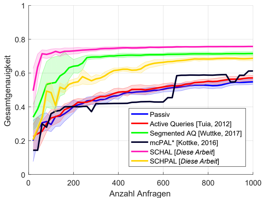
Abbildung 6.10: Vergleich der vorgestellten Methode, in den Varianten mit und ohne Berücksichtigung der lokalen Dichte (SCHPAL und SCHAL) auf dem Vaihingen-Datensatz (Abbildung nach [Wuttke et al., 2018]). Ebenso sind andere Methoden aus dem Stand der Wissenschaft dargestellt. Die durchgezogenen Linien sind die Mittelwerte von zehn Wiederholungen des Experimentes und die schattierten Flächen sind die zugehörigen Standardabweichungen. Die in dieser Arbeit vorgestellte SCHAL-Methode ist in ihrer Version ohne die Berücksichtigung der lokalen Dichte sowohl in maximal erreichter Gesamtgenauigkeit als auch in der Lernrate deutlich besser als die anderen Methoden.
