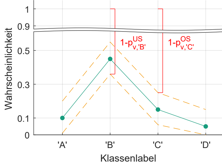
Abbildung 4.6: Beispielfähige Verteilung der Klassenlabel für einen Knoten (Abbildung nach [Wuttke et al., 2018]). Der relative Anteil p_{v,w} ist in grün und die Unsicherheitsschranken p_{v,w}^{US} und p_{v,w}^{OS} sind in orange dargestellt. Klassenlabel B ist akzeptabel , da der maximale Klassifikationsfehler für Klassenlabel B ( 1 - p_{v,B}^{US} = 0,64 ) kleiner ist als der doppelte minimale Klassifikationsfehler für Klassenlabel C ( 2 \cdot (1 - p_{v,C}^{OS}) = 1,5 ).
