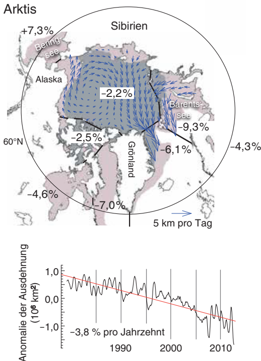
Abb. 6. Mittleres Zirkulationsmuster von Meereis und die dekadischen Trends (%) der jährlichen Anomalien der Meereisausdehnung (d.h. nach Entfernung des Jahresgangs) in verschiedenen Regionen der Arktis. Pfeile zeigen die mittlere Richtung und Geschwindigkeit der Eisdrift an. Die mittlere Meereisbedeckung, beruhend auf Satellitenbeobachtungen, in maximaler (minimaler) Ausdehnung im Zeitraum von 1979 bis 2012 ist in Orange (Grau) schattiert. – IPCC (2014a), Abb. FAQ 4.1 (Abbildung 1).
