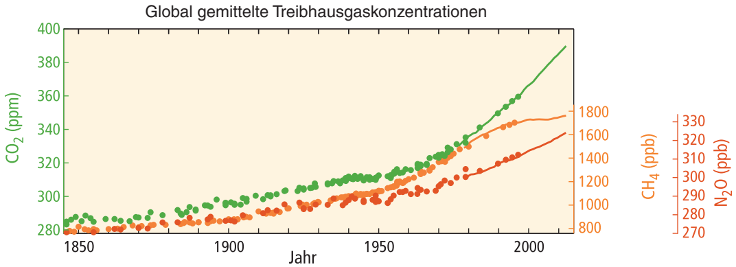
Abb. 7. Atmosphärische Konzentrationen der Treibhausgase Kohlendioxid ( \text{CO}_2 , grün), Methan ( \text{CH}_4 , orange) und Lachgas ( \text{N}_2\text{O} , rot), ermittelt aus Eisbohrkerndaten (Punkte) und aus direkten atmosphärischen Messungen (Linien). – IPCC (2014b), Abb. SPM.1c.
