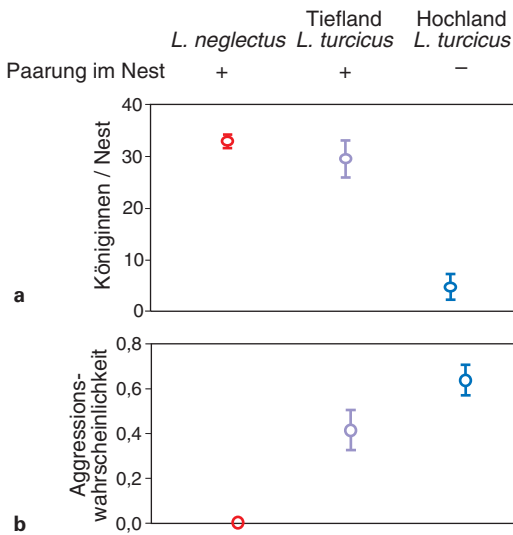
Abb. 6. Invasive Parameter bei Lasius neglectus und L. turcicus (Tieflandform und Hochlandform): a , Paarungsverhalten und Königinenzahl ( n = 18, 12, 13 Populationen, Anova p < 0,001 ); b , Aggression zwischen den Nestern einer Kolonie ( n = 17, 12, 13 Populationen, Anova p < 0,001 ). – Nach Daten aus Cremer et al. (2008).
