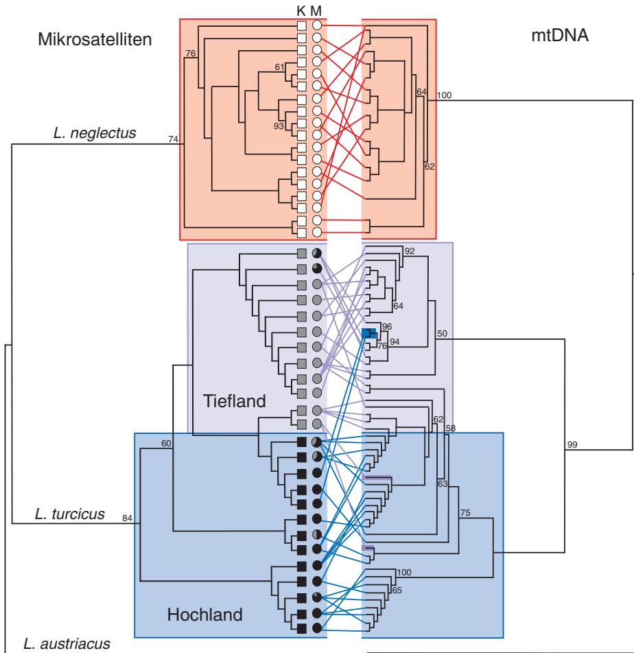
Abb. 3. Phylogenetischer Stammbaum von Lasius neglectus (pink) und L. turcicus (purple: Tieflandform; blue: Hochlandform); links: basierend auf Mikrosatelliten, rechts: basierend auf mitochondrialer DNA (mtDNA; Cytochrom-Oxidase-I); K (Vierecke Mitte): kutikuläre Kohlenwasserstoffe, s. Abb. 4; M (Kreise Mitte): morphometrische Parameter, s. Abb. 5. – © Cremer et al. (2008), CC-BY-2.0.
