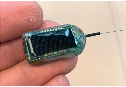
Abb. 12. Am MPI für Ornithologie entwickelter Miniatursender aus dem ICARUS-System (< 5 Gramm).
