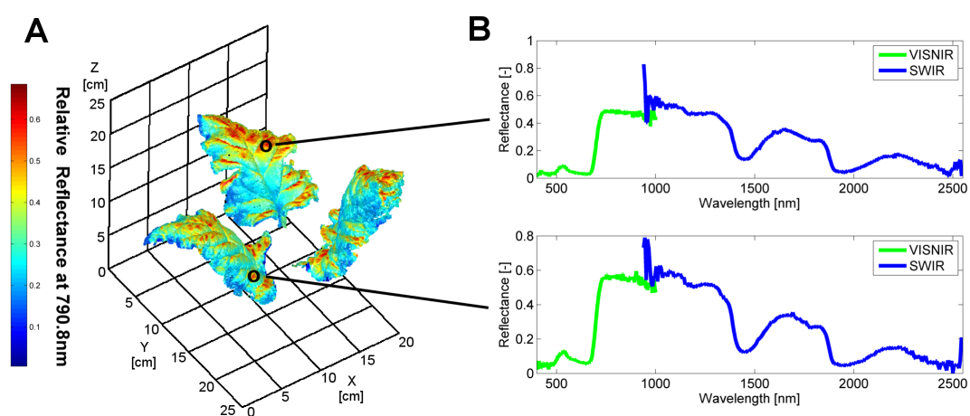
Abbildung 8.3 Beispiel der Fusion einer 3D-Punktwolke einer Rübenpflanze mit hyperspektralen Daten (A). Dabei ist an jedem Oberflächenpunkt der hyperspektrale Messwerte abgreifbar (B) [Behmann et al., 2015b].
