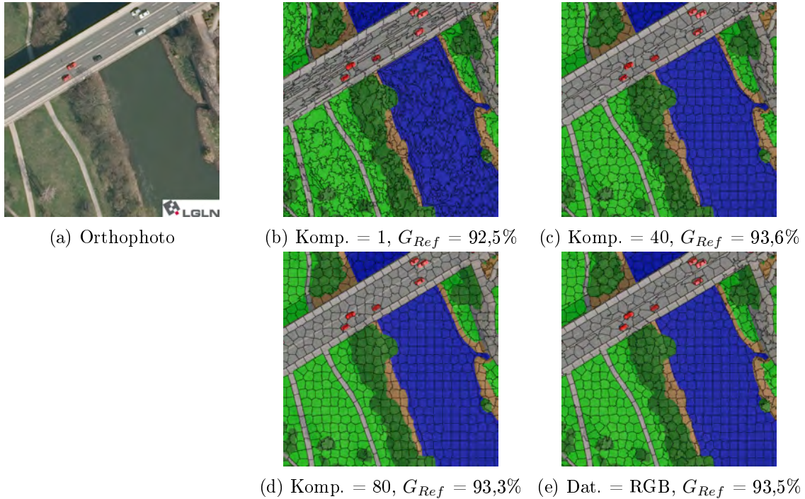
Abbildung 5.2.: Orthophoto einer Szene im Testgebiet Hameln (a), überlagert mit den Ergebnissen der Superspikelsegmentierung für eine Größe von 400 Pixeln und die Kompaktheitsparameter (Komp.) 1 (b), 40 (c) und 80 (d) unter Verwendung der sekundären Bildinformationen als Eingangsdaten sowie für eine Kompaktheit von 20 bei Verwendung der primären Bildinformation (Dat. = RGB) als Eingangsdaten (e). Die Grenzen der segmentierten Superspiksel sind jeweils den pixelbasierten Referenzdaten überlagert. Die Farben markieren die Zugehörigkeit zur Bodenbedeckungsklasse: Geb. (orange), Vers. (grau), Bod. (braun), Gras (hellgrün), Baum (dunkelgrün), Was. (blau), Fhgz. (rot) und Sonst. (rosa). G_{Ref} : Gesamtgenauigkeit abgeleitet aus pixelweisen Vergleich der Referenzlabels pro Superspiksel zu den pixelbasierten Referenzdaten.
