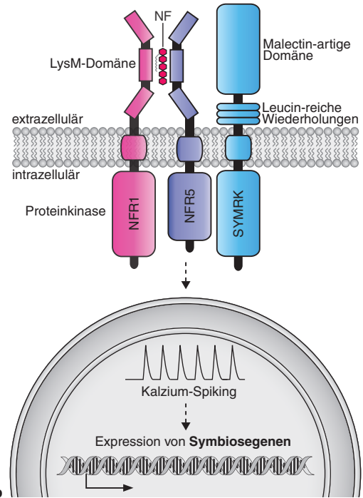
Abb. 5. Rezeptorkomplexbildung und spezifische Antwort der Pflanzenzelle in Abhängigkeit von den Signalmolekülen: schematische Darstellung des Chitin-Rezeptorkomplexes in Reis ( a ) und des Nod-Faktor-Rezeptorkomplexes in Lotus ( b ). Erläuterungen s. Text. – Grafik: Martina Ried.
