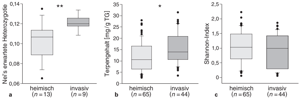
Abb. 6. Tanacetum vulgare (Rainfarn): a , Genetische Diversität [angegeben als Index »Nei's erwartete Heterozygotie«], basierend auf 95 genetischen Markern, b , Gesamtgehalt an Terpenen [in mg/g TG], basierend auf 84 Komponenten und c , chemische Diversität [Shannon-Index] in Blättern von Populationen aus Europa (heimische Vorkommen, 13 Populationen, 65 Individuen) und Nordamerika (invasive Vorkommen, 9 Populationen, 44 Individuen), nach Anzucht unter standardisierten Bedingungen. Die Boxplots zeigen die Mediane, 10-, 25-, 75- und 90-Perzentile und die Punkte die Ausreißer; *: P < 0,05 ; **: P < 0,01 nach Mann-Whitney U-Test. – a, c, nach Wolf et al. (2012), mit Erlaubnis von Elsevier; b, nach Wolf et al. (2011), mit Erlaubnis von Springer.
