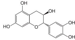
Abb. 1. Strukturformel von (–)-Catechin (Flavan-3-ol).
