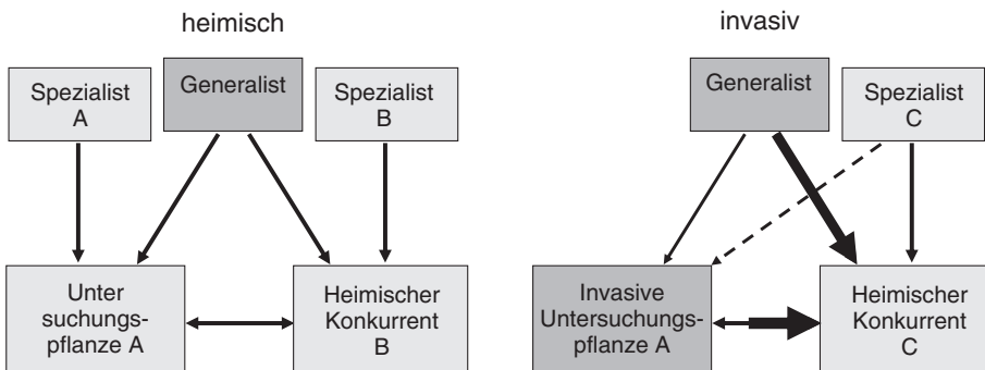
Abb. 2. Schematische Darstellung zur Enemy-release-Hypothese; Erläuterungen s. Text.
