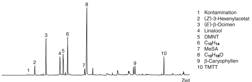
Abb. 2. Gaschromatogramm des Duftes eines Blattes von Phaseolus lunatus , nach Befall mit Spodoptera (Lepidoptera); DMNT: 4,8-Dimethyl-1,3(E),7-nonatrien, MeSA: Methylsalicylat, TMTT: 4,8,12-Trimethyltrideca-1,3,7,11-tetraen.
