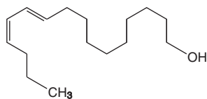
Abb. 2. Strukturformel von Bombykol ([10E,12Z]-10, 12-Hexadecadien-1-ol).
