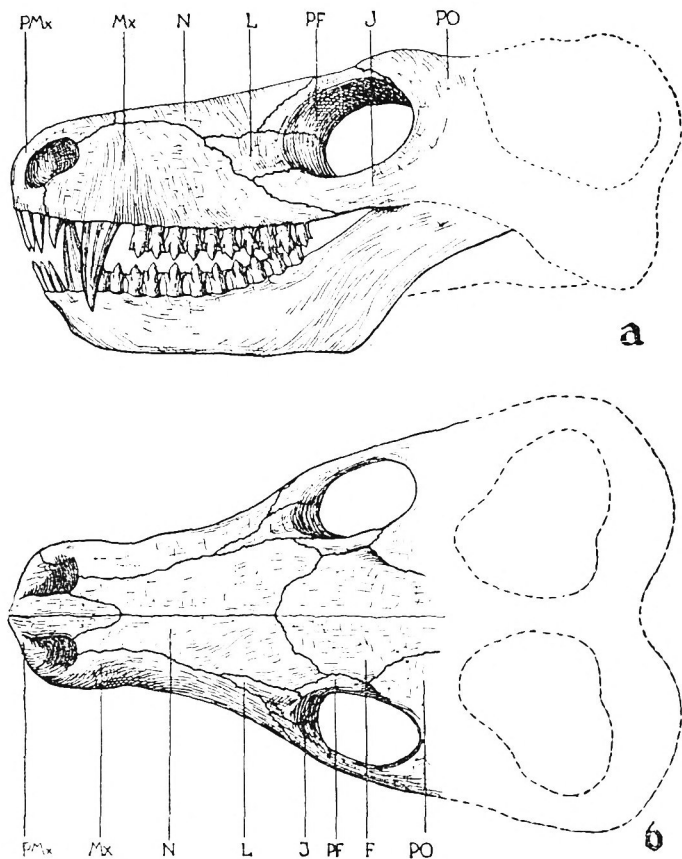
Fig. 2. Tribolodon freerensis Seeley. Rekonstruktionsversuch des Kopfes a) Seitenansicht, b) Oberseite. Natürl. Größe. — F Frontale. J Jugale. L Lacrimale. Mx Maxillare. N Nasale. PF Praefrontale. PMx Prae- maxillare. PO Postorbitale.
