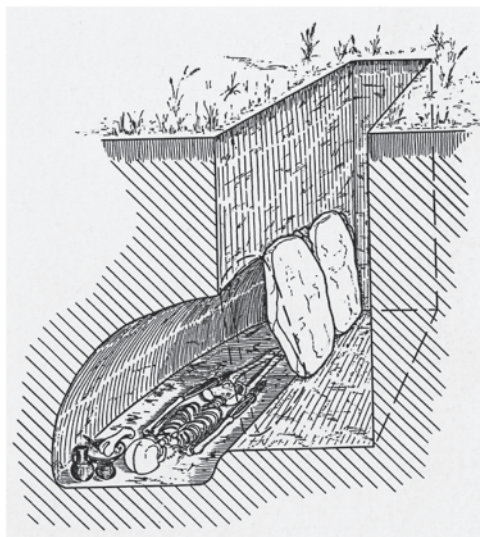
Tafel 17. 1-2 Katakombengrab mit querliegendem Dromos (T-förmig), 3 Nischengrab, 4 Erdgrab. 1-3 Axonometrie.
