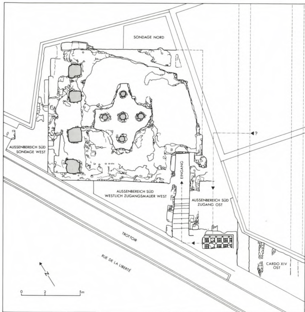
Abb. 2. Karthago, Kobbat Bent el Rey. Schematischer Übersichtsplan: Aufsicht auf die Kobbat Bent el Rey mit Oberlichtern (gerastert) und Bezeichnung der Sondagenbereiche. M. 1:200.
