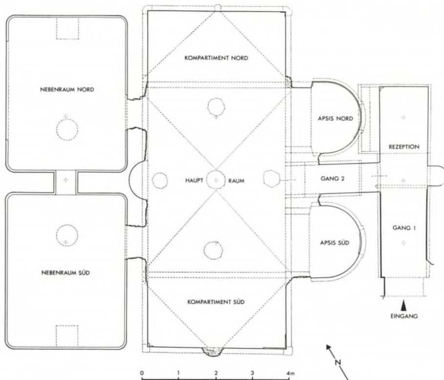
Abb. 3. Karthago, Kobbat Bent el Rey. Grundriß der unterirdischen Anlage mit Angabe der Oberlichter (nach Storz [Anm. 4] 49 Abb. 6). M. 1:100.
