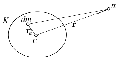
Abb. 10.1 Gravitationsfeld eines Kontinuums
