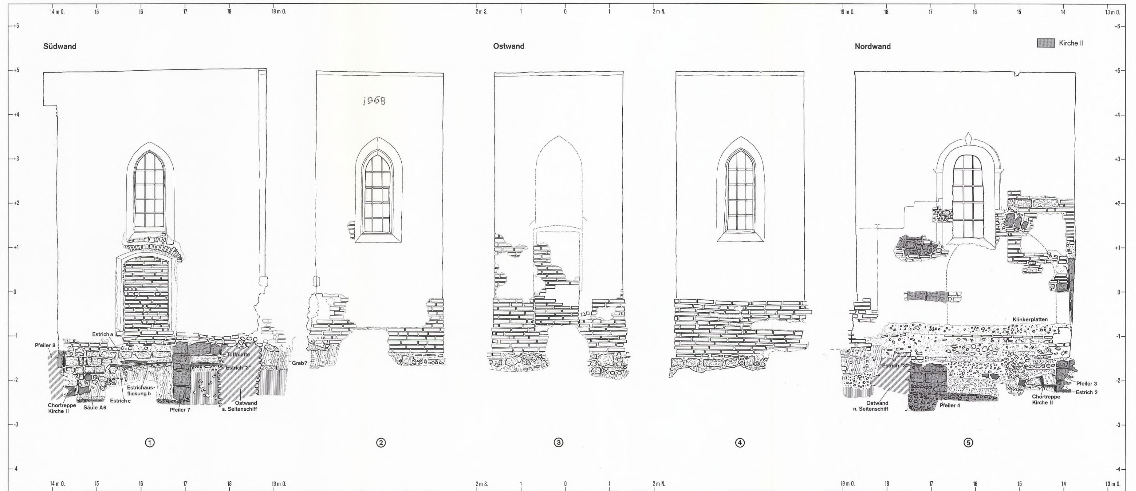
Sandau, Stadt Landsberg a. L., St. Benedikt. Wände des Chores der Kirche IV, Außenseiten. M. 1:50.
