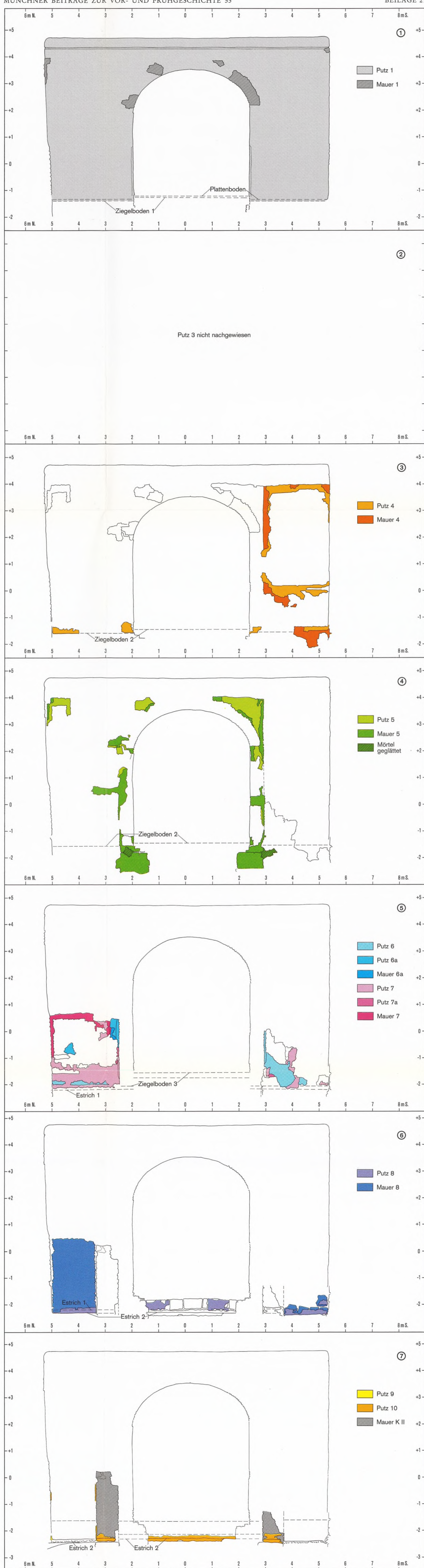
Sandau, Stadt Landsberg a. L., St. Benedikt. Langhausostwand, Abfolge der Mauerputze auf der Innenseite. M. 1:75.
