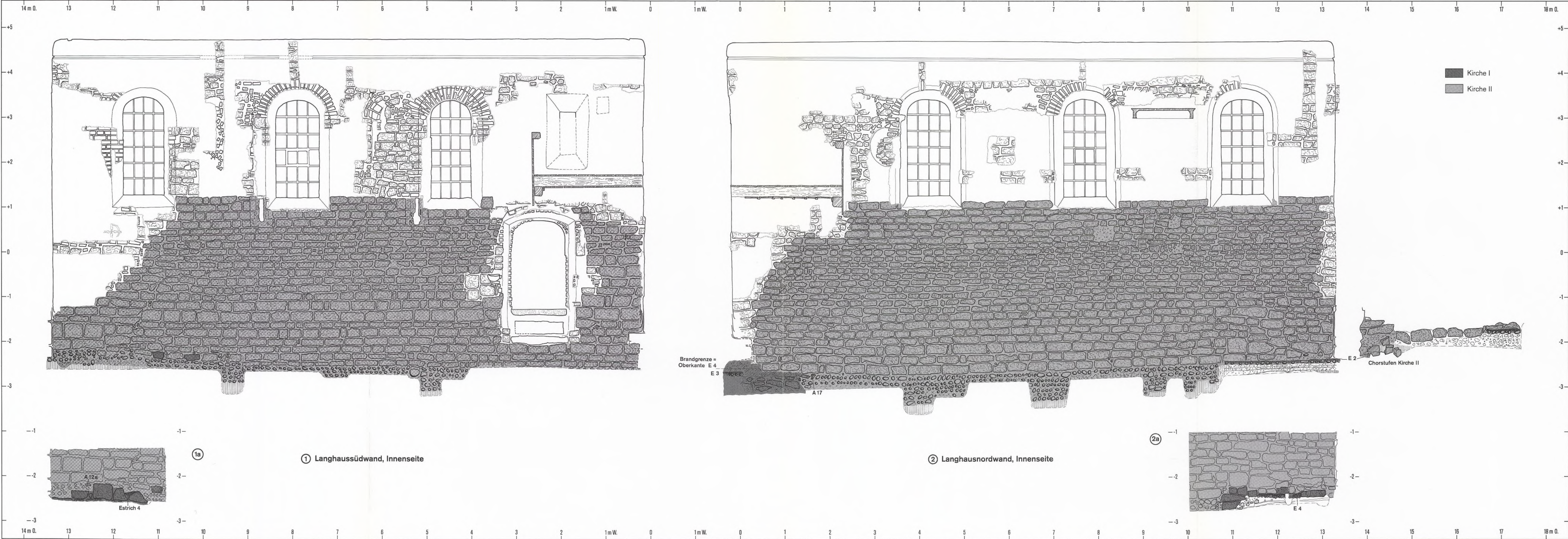
Sandau, Stadt Landsberg a. L., St. Benedikt. 1 Langhaussüdwand, Innenseite; 2 Langhausnordwand, Innenseite. M. 1:50.
