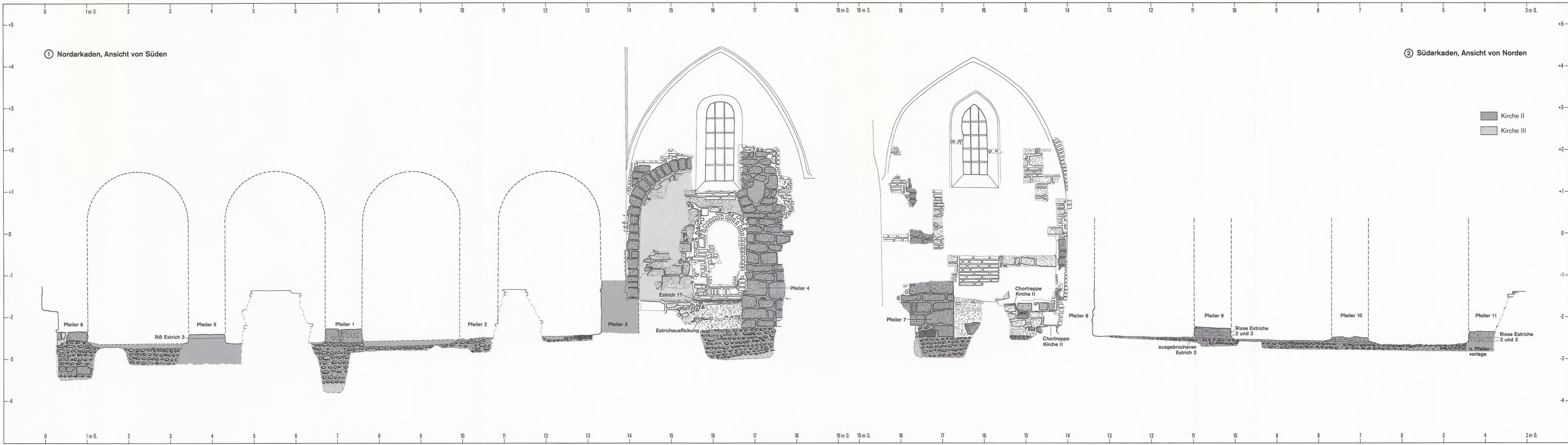
Sandau, Stadt Landsberg a. L., St. Benedikt. Arkaturen der Kirche II. 1 Nordarkaden, Ansicht von Süden; 2 Südarkaden, Ansicht von Norden. M. 1:50.
