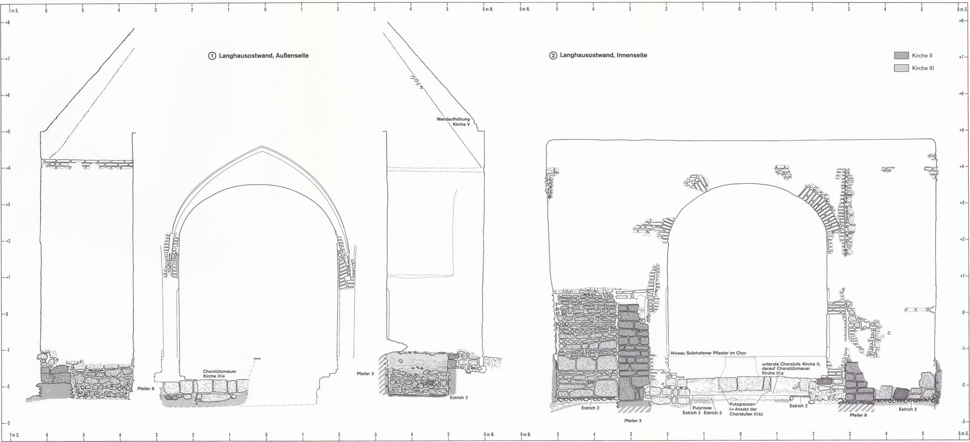
Sandau, Stadt Landsberg a. L., St. Benedikt. Langhausostwand. 1 Außenseite; 2 Innenseite. M. 1:50.
