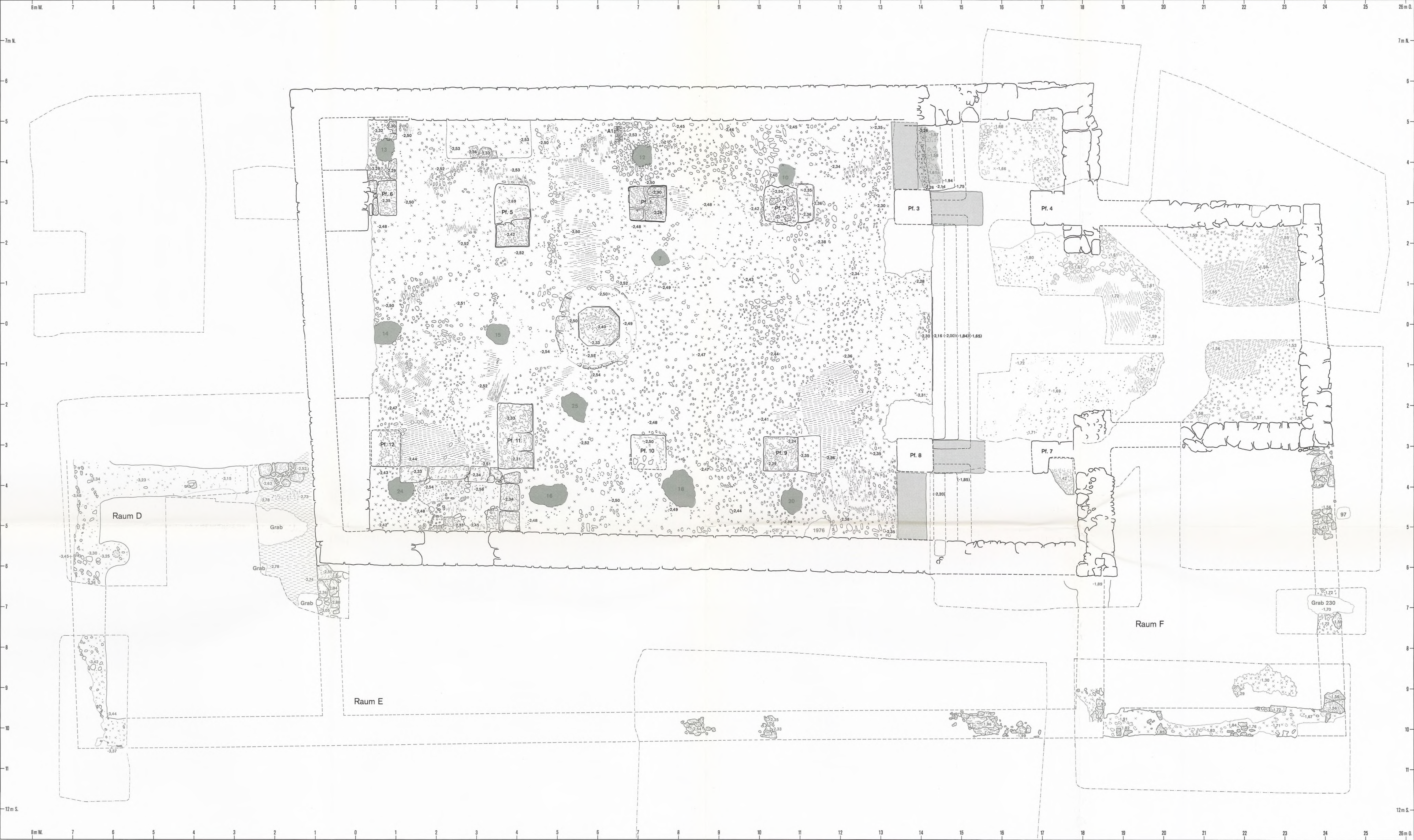
Sandau, Stadt Landsberg a. L., St. Benedikt. Grundriß der Kirchen IIa und III. M. 1:50.
