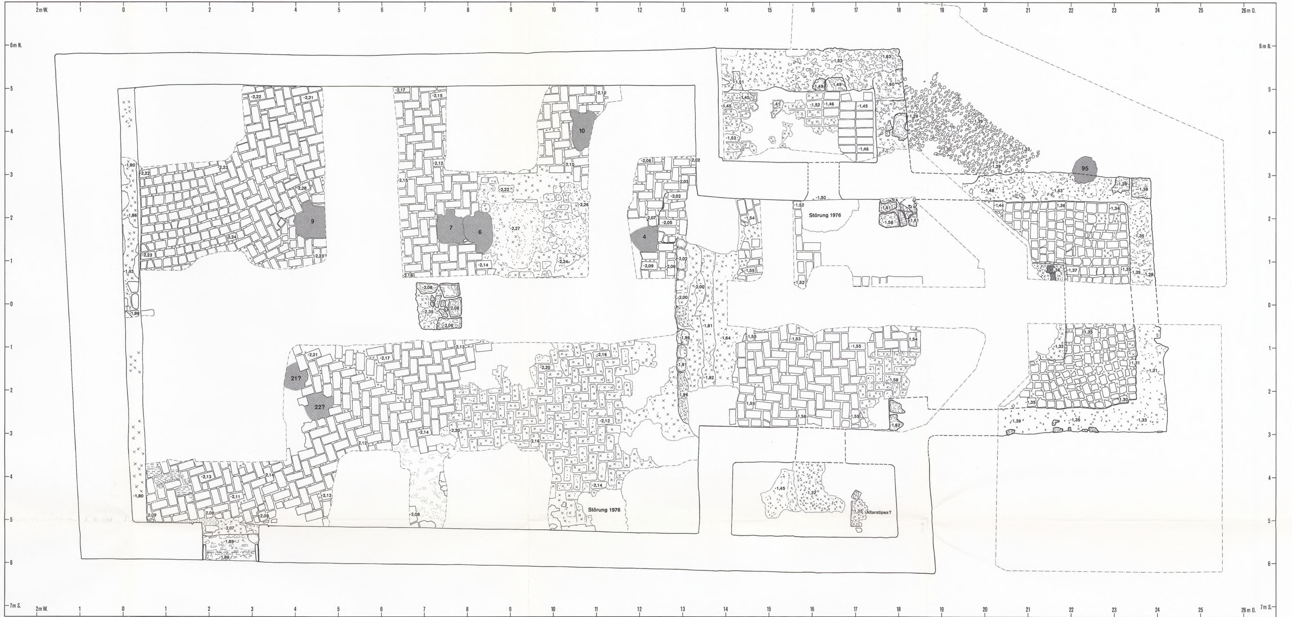
Sandau, Stadt Landsberg a. L., St. Benedikt. Grundriß der Kirche IIIc. M. 1:50.
