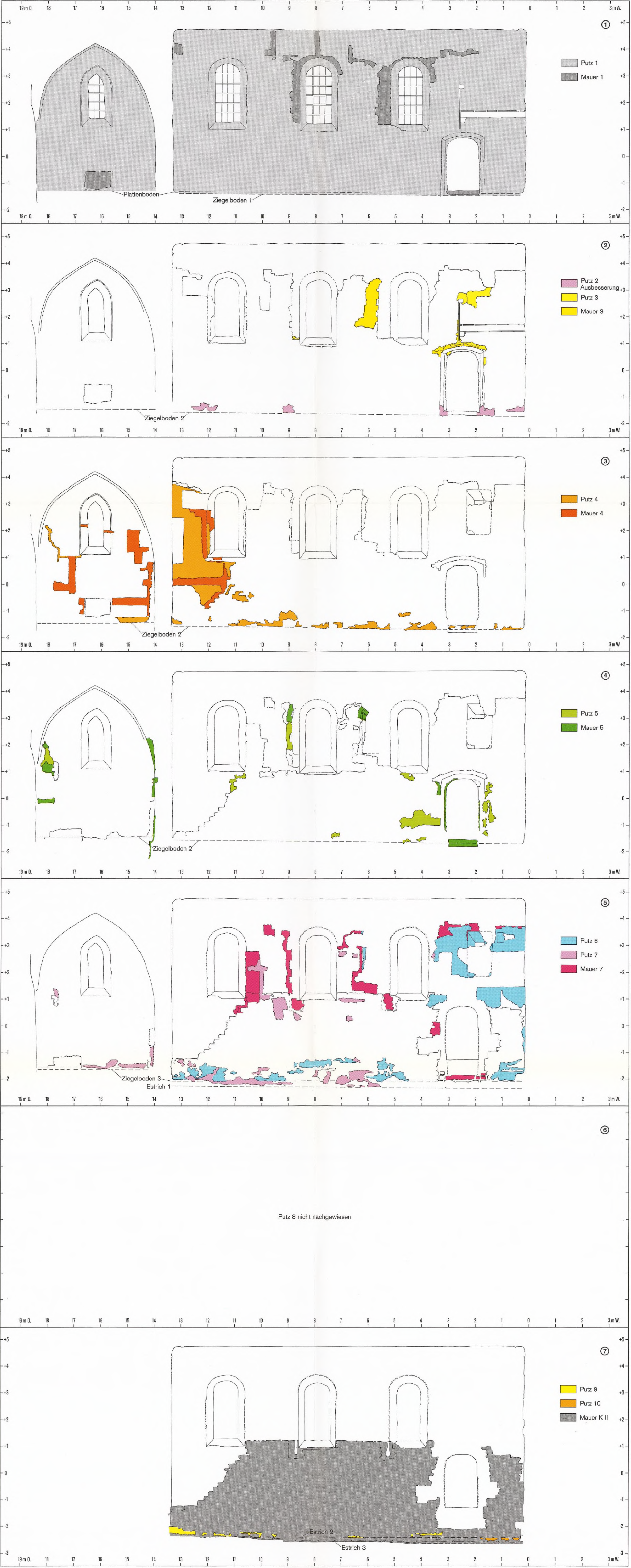
Sandau, Stadt Landsberg a. L., St. Benedikt. Langhaus- und Chorsüdwall, Abfolge der Mauerputze auf der Innenseite. M. 1:75.
