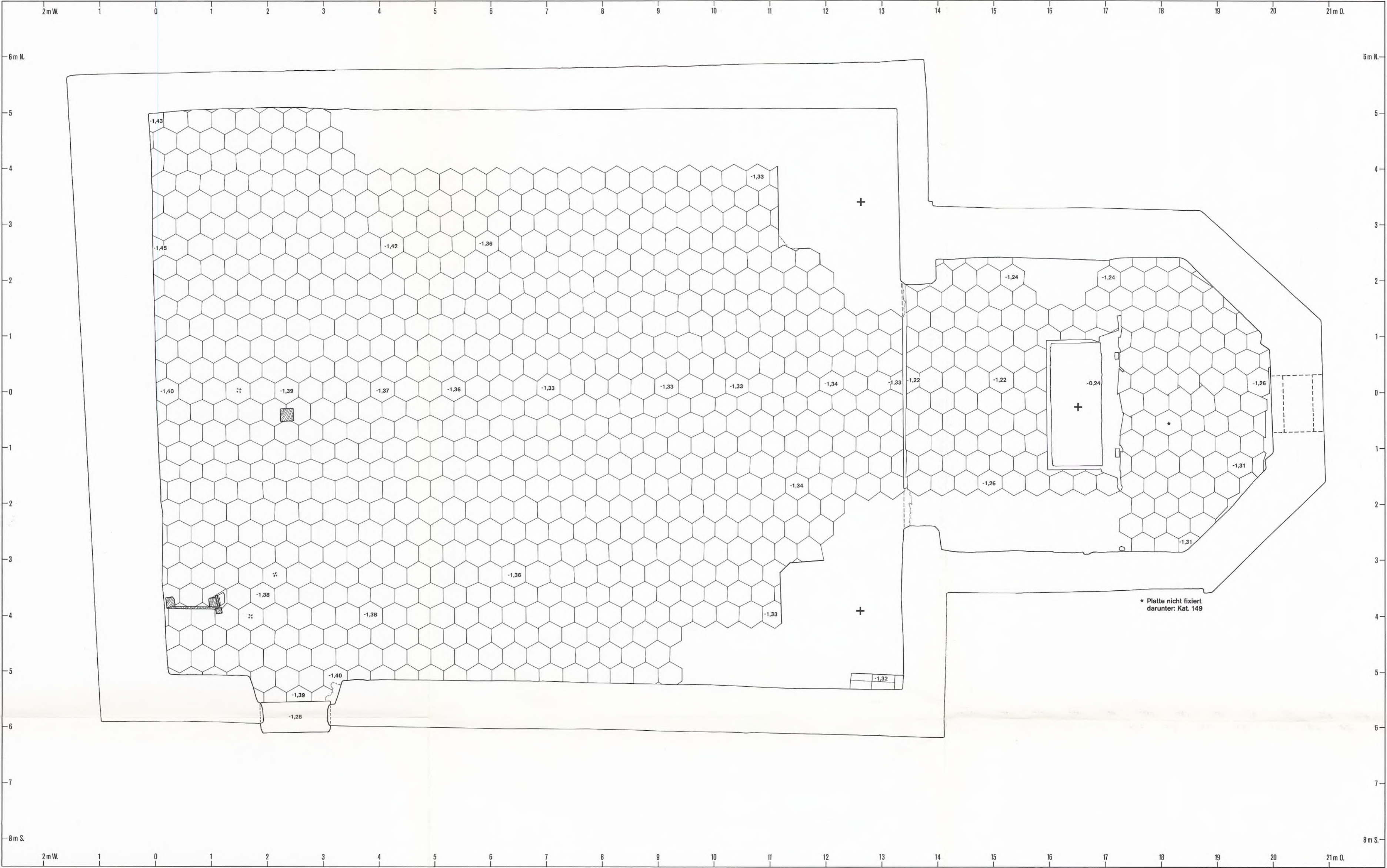
Sandau, Stadt Landsberg a. L., St. Benedikt. Grundriß der Kirche Va. M. 1:50.
