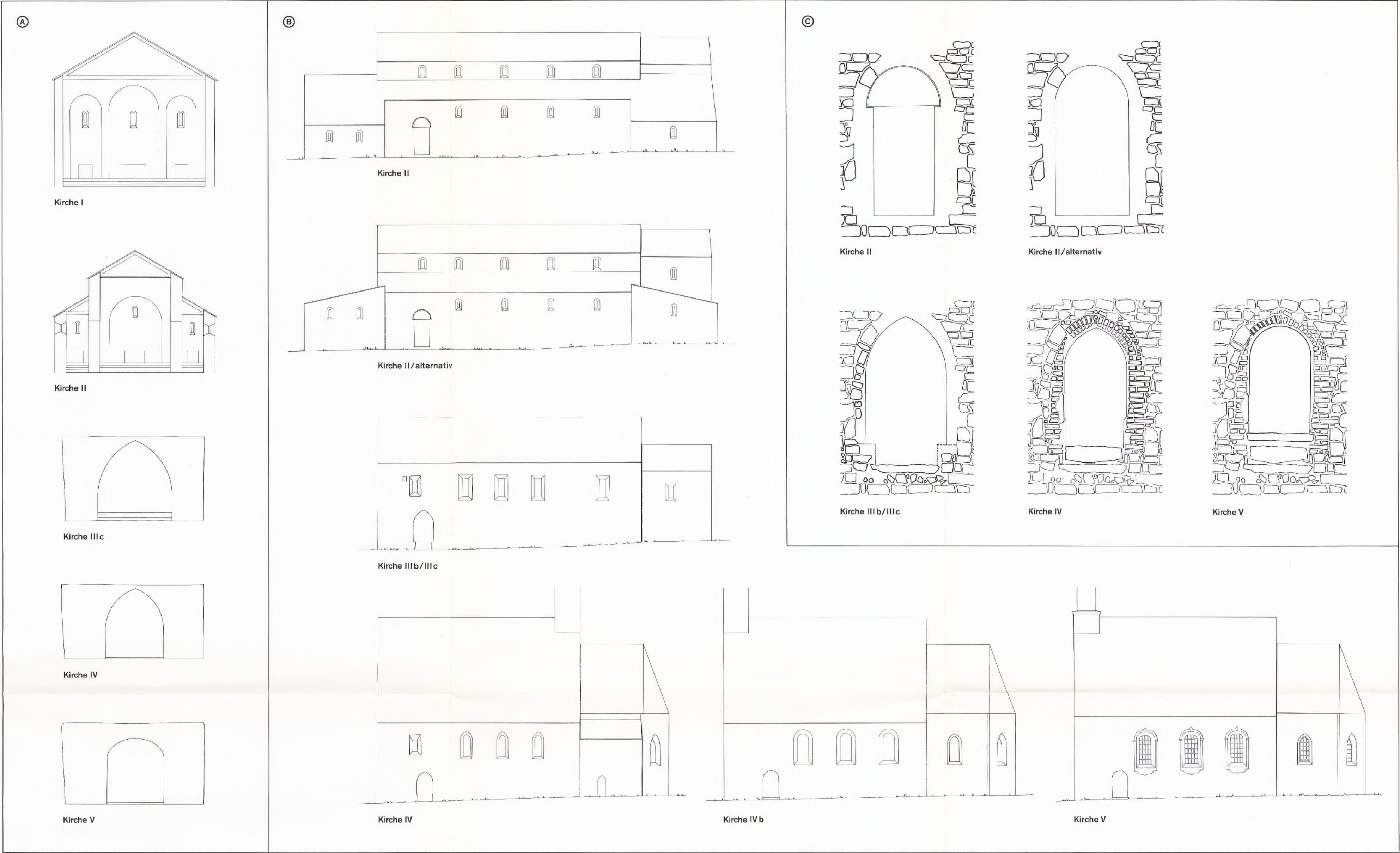
Sandau, St. Benedikt. Rekonstruktionsskizzen. A Schnitt am Choransatz bzw. Triumphbögen; B Aufriß und Befensterung der Südwand; C Türbogen. A u. B M. 1:200; C M. 1:50.
