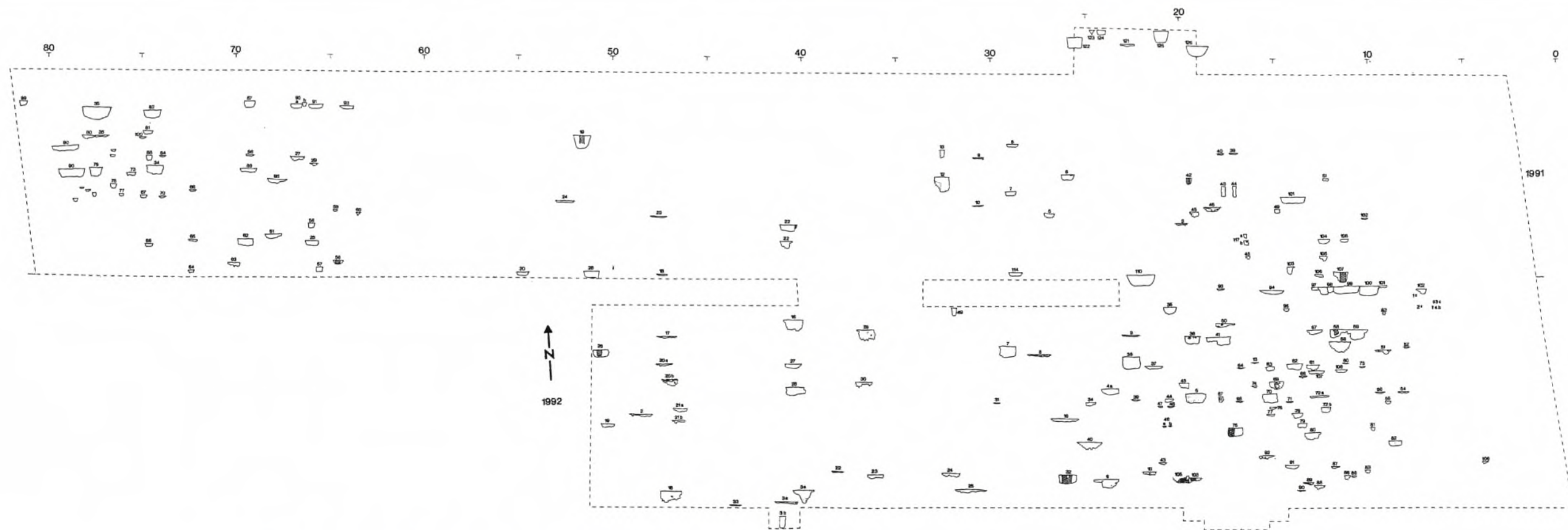
Karlburg – villa. A Plan der Grabungsflächen 1991 und 1992 mit Eintrag der Befunde aus den Plana 1–4 (vgl. Taf. 27–32). – B Pfostenschnittplan der Grabungsflächen 1991 und 1992.
