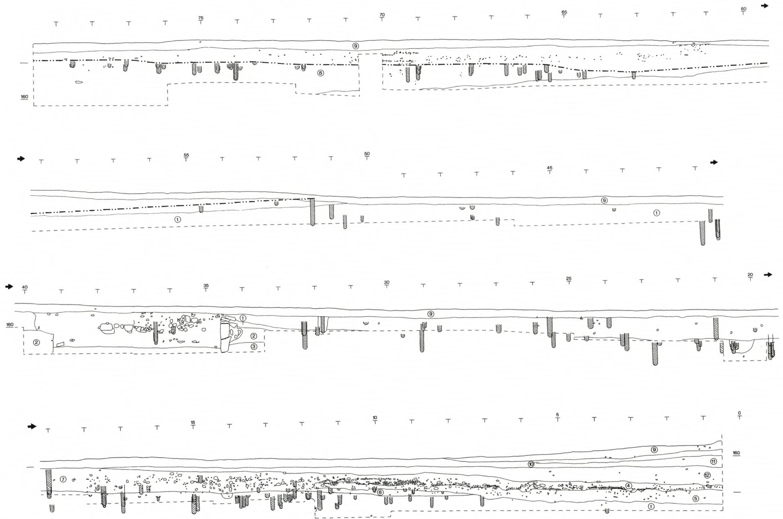
Karlburg – villa. Grabungen 1991 und 1992. Zusammengesetztes Profil aus Nordprofil 1992 (bis m 51) und Südprofil 1991 (bis m 79,7) mit schematischer Eintragung der Pfostengruben aus dem Planum (vgl. Beil. 5). Strich-Doppelpunkt-Linie: Mainseitenarm nach Aufgabe der Siedlung.
