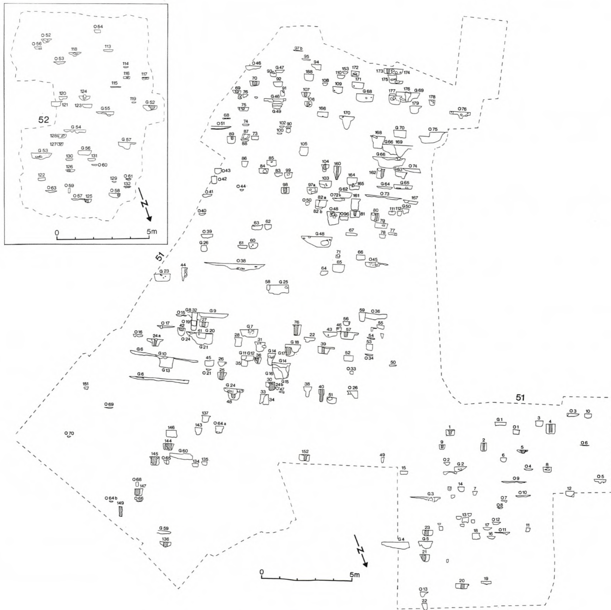
Roßtal. Schnittplan von Pfosten, Gruben (G) und Objekten (O) in den Flächen 51 und 52 (vgl. Beil. 14).
