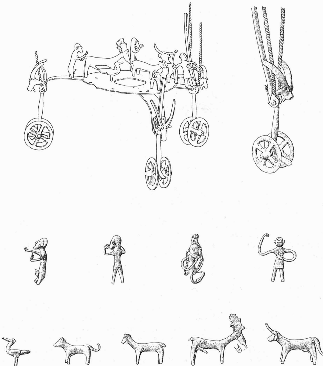
Abb. 13. Lucera, Prov. Foggia, Apulien, Grabfund. Teile eines Kesselwagens. Bronze, oben links M. 1: 4, sonst M. 1: 3. Nach E. Woytowitsch Anm. 44.
