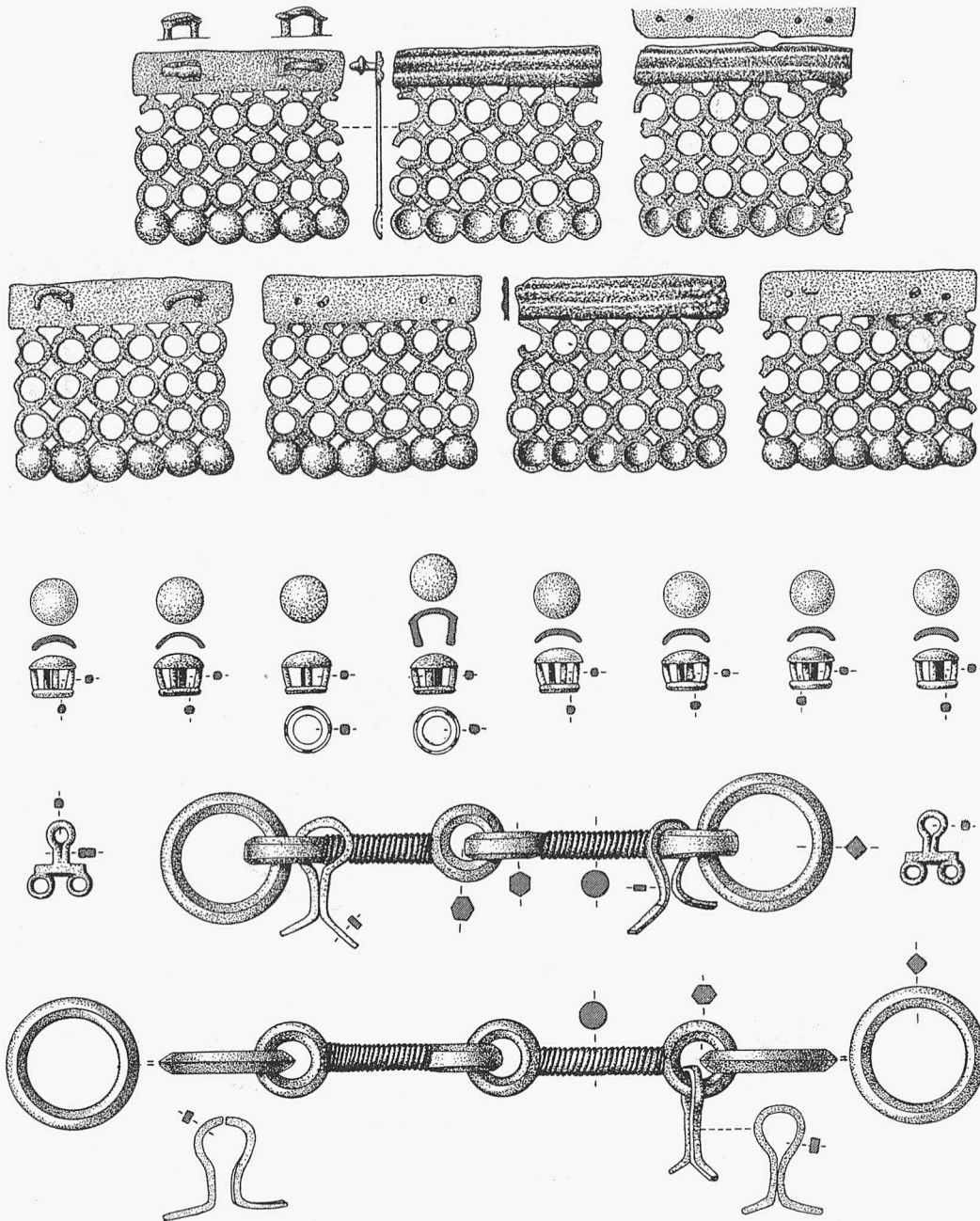
Abb. 81. Großbeibstadt, Unterfranken, Grab. Jochzubehör und Zaumzeug. Bronze, M. 1: 2. Nach G. Kossack Anm. 259. Zugehörig Abb. 80.82.
