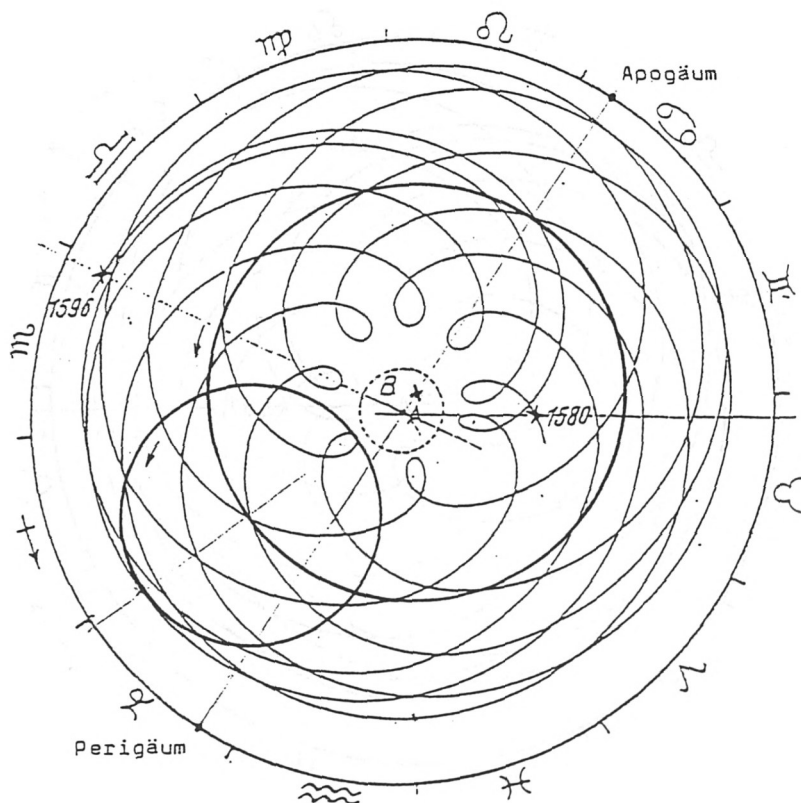
Bild 3: Marsbahn nach Art des Ptolemäus, gezeichnet von J. Kepler (1609) mit Deferent (Radius R ) und Epizykel ( r ) r/R = 0,685 nach Ptolemäus (Almagest 10,8) Apogäum des Mars: Krebs 25^{\circ} 30' (Almagest 10,5) synodische Umlaufzeit T_{\text{syn}} = 779,95 \text{ d} = 2,135 \text{ a}
