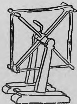
Abb. 2. Piemontesische Drehhaspel
