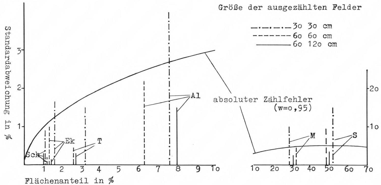
Abb. 16. a) Beeinflussung der Streuung durch die Größe der Stichproben-Felder und durch die Meßpunktezah: Standardabweichung einiger Fossilgruppen bei verschiedenen großen Meßfeldern und konstanter Punktezah ( n = 400 ).
