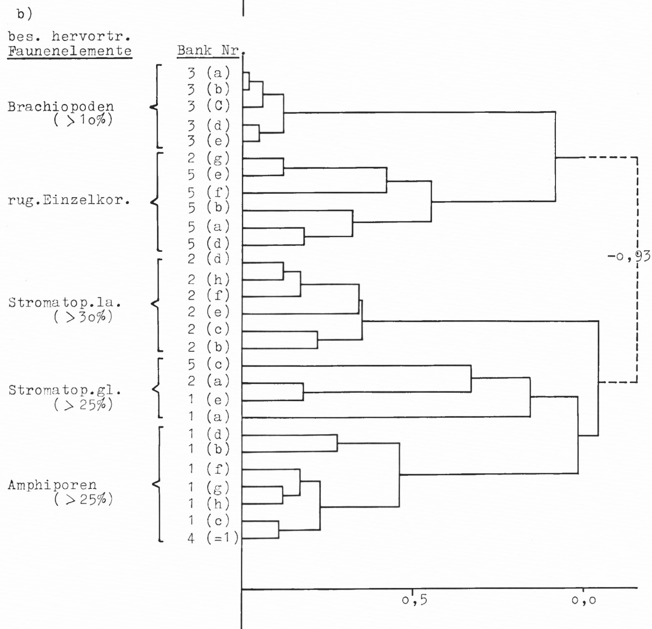
Abb. 27. Clusterdiagramme der Fauna und Schichten im Profil 28, Steinbruch Steltenberg in Hohenlimburg, berechnet aufgrund von standardisierten i-Zahlen unter Verwendung von \cos \Phi -Koeffizienten. a) R-Technik, b) Q-Technik.
