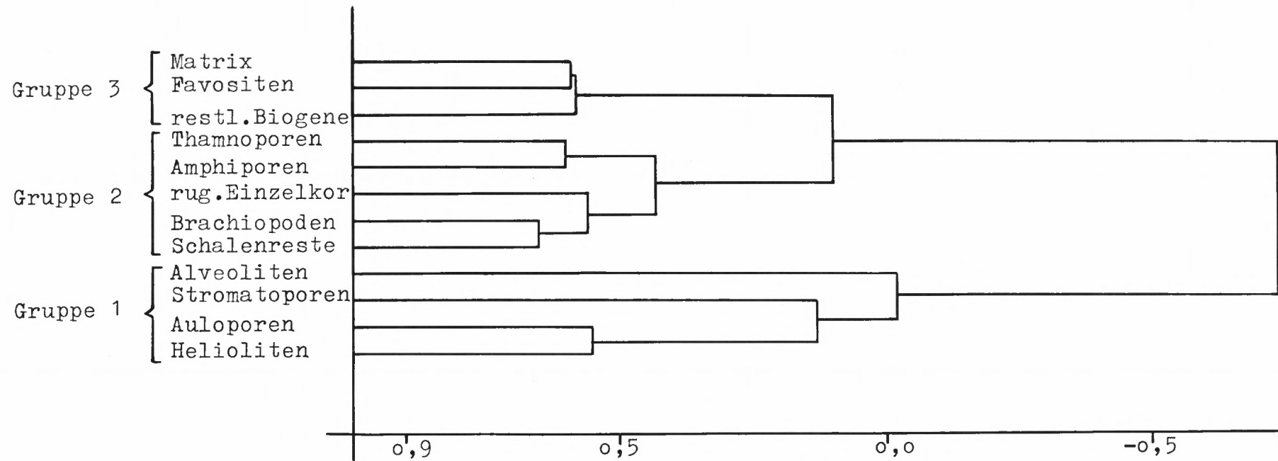
Abb. 19. Cluster-Diagramme der Faunenelemente auf der Schichtfläche in Letmathe. Berechnung aufgrund der Prozentwerte von 14 Großfeldern (60 × 60 cm) unter Verwendung der Korrelationskoeffizienten-Matrix, R-Technik.
