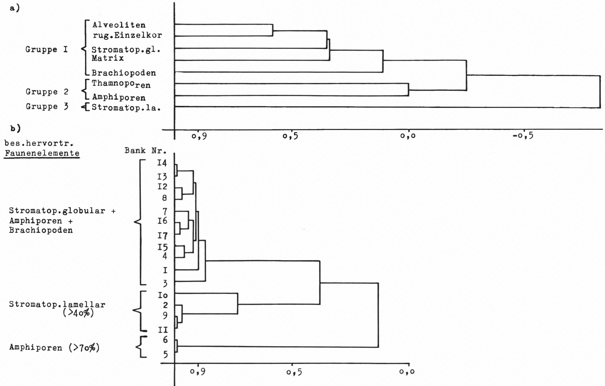
Abb. 28. Clusterdiagramme der Faunenelemente und der Bänke im Profil 17 im Steinbruch Steltenberg, Hohenlimburg. Unveränderte Urmatrix, Korrelationskoeffizienten. a) R-Technik, b) Q-Technik.
