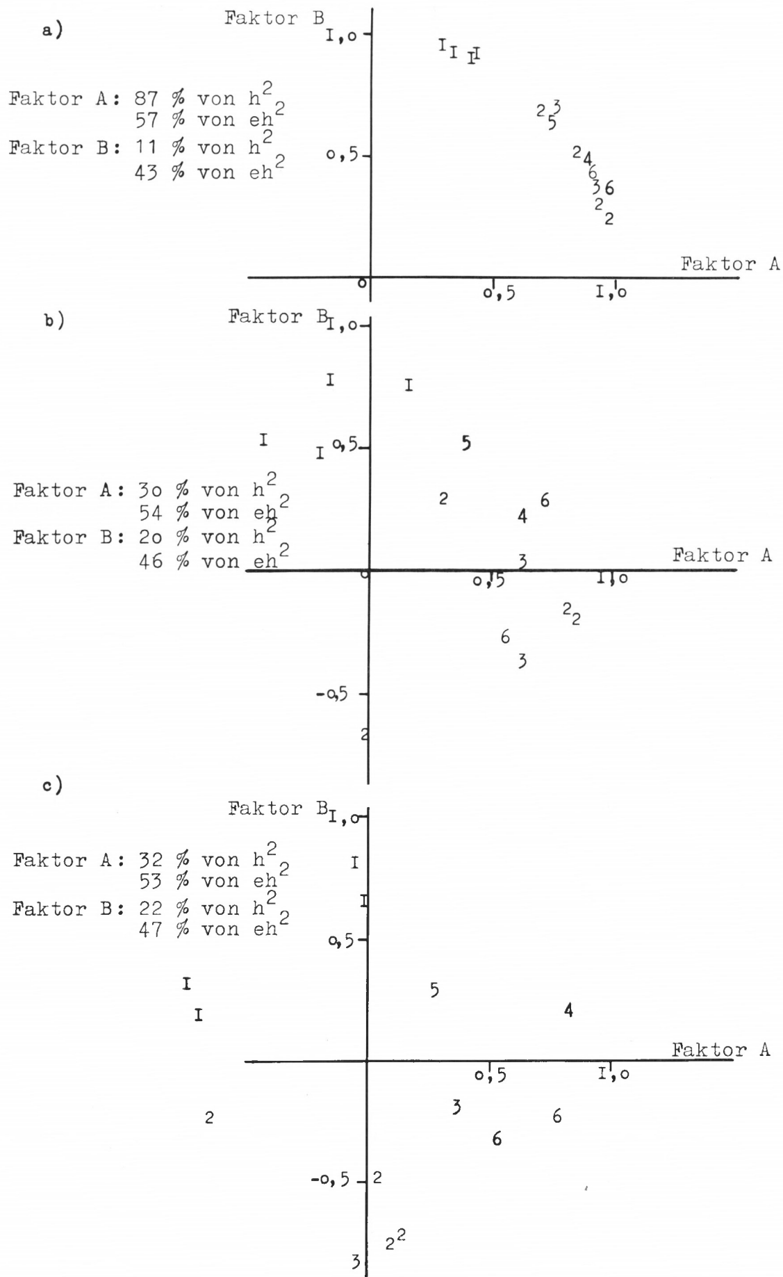
Abb. 20. Rotierte Faktorendiagramme für 14 Großfelder aus 6 Testbereichen der Schichtfläche Letmathe, Q-Technik. Vergleich der Faktorenanalyse (berechnet aus der Korrelationskoeffizienten-Matrix) bei Veränderung der Ausgangsdaten (Prozentwerte der Punktauszahlung von 14 Großfeldern): a) bei unveränderten Daten, b) bei normierten Daten und c) bei standardisierten Daten.
