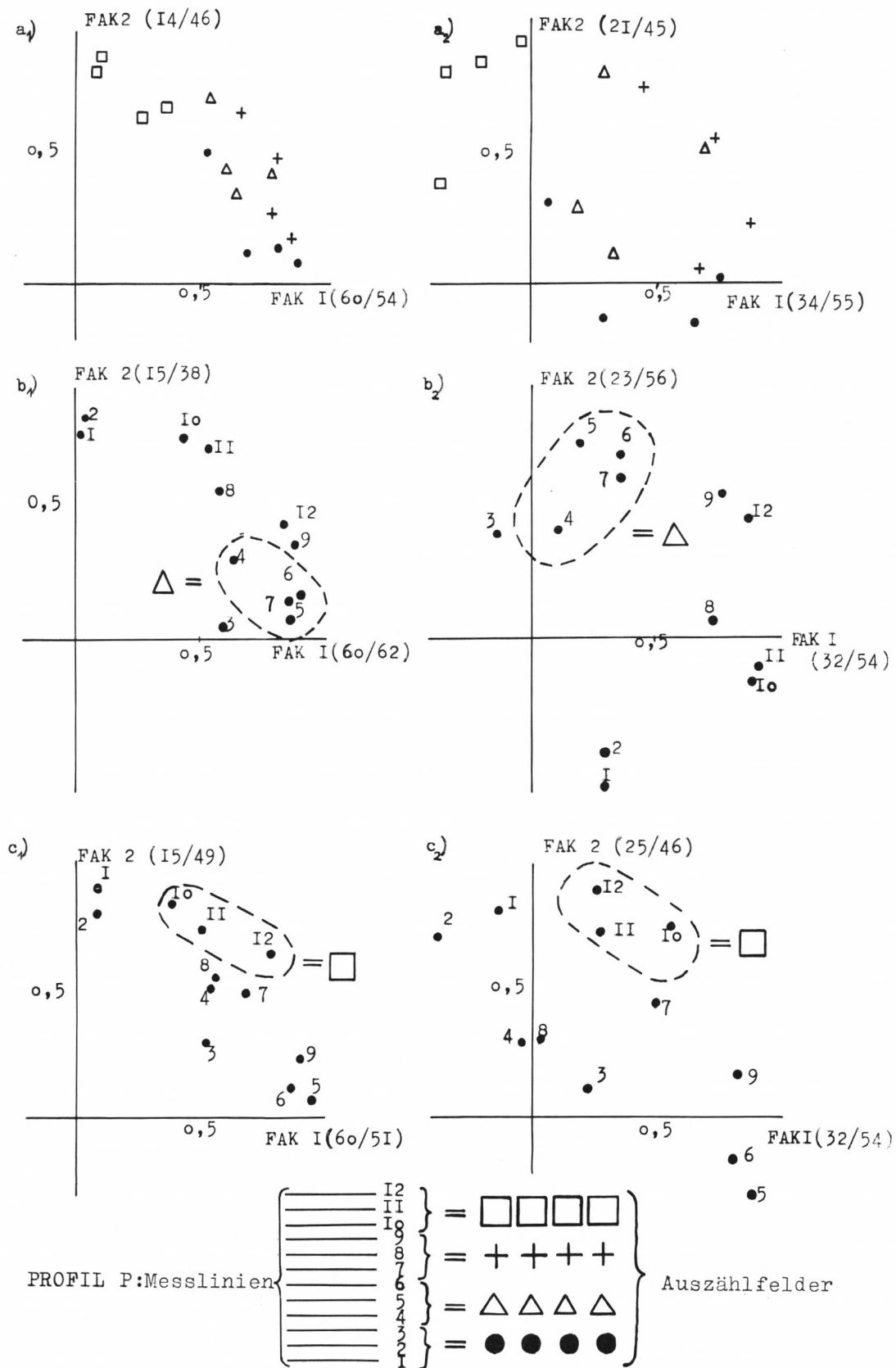
Abb. 23. Vergleich der Meßverfahren, dargestellt durch rotierte Faktorendiagramme (Q-Technik) der Auszähleinheiten im Profil P, östlichster Steinbruch S der Lenne in Letmathe. Es wurden nur 2 Faktoren extrahiert. Die Skizze an der Basis der Abbildung zeigt die Anordnung der Meßlinien bzw. der Auszählfelder (30 × 30 cm). Die Berechnung der Faktorenmatrix erfolgte in der linken Diagrammreihe unter Verwendung der cos-Φ-Koeffizienten, in der rechten Diagrammreihe mit Hilfe des Korrelationskoeffizienten. Als Ausgangsdaten dienten bei a) die normierten Prozentwerte der Punktauszahlung (400 Punkte pro Feld), bei b) die normierten Prozentwerte der Linearzählung und bei c) die normierten i-Zahlen der Linearzählung. In den Diagrammen gibt die erste Zahl hinter den Faktoren den Anteil des Faktors an der Gesamtkommunalität an, die zweite Zahl den Anteil an der von den beiden Faktoren erfaßten Kommunalität.
