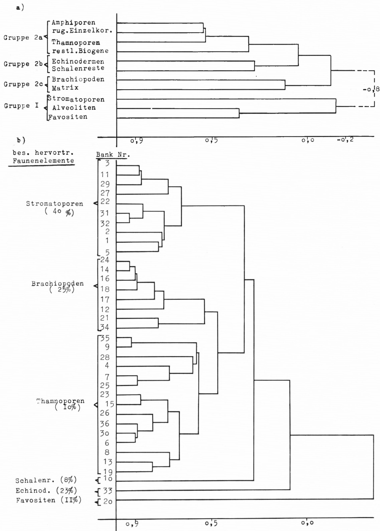
Abb. 24. Clusterdiagramm von Fauna und Bänken im Profil 36, Steinbruch Letmathe, errechnet aus den Prozentwerten unter Verwendung der Korrelationskoeffizienten. Die Auszählung der Bänke erfolgte nach der Linearzählmethode. a) R-Technik; zwei miteinander negativ korrelierte Großgruppen stehen einander gegenüber, die Lebensformtypen entsprechen (massive, großwüchsige Kolonien; zylindrische, kleine Formen, schalentragende Organismen und Matrix). b) Q-Technik; Clusterung nach 6 Gruppen, die monomikten Assoziationen (Brachiopoden; Thamnoporen) und heteromikten Assoziationen (Stromatoporen) entsprechen, siehe Seite 54.
