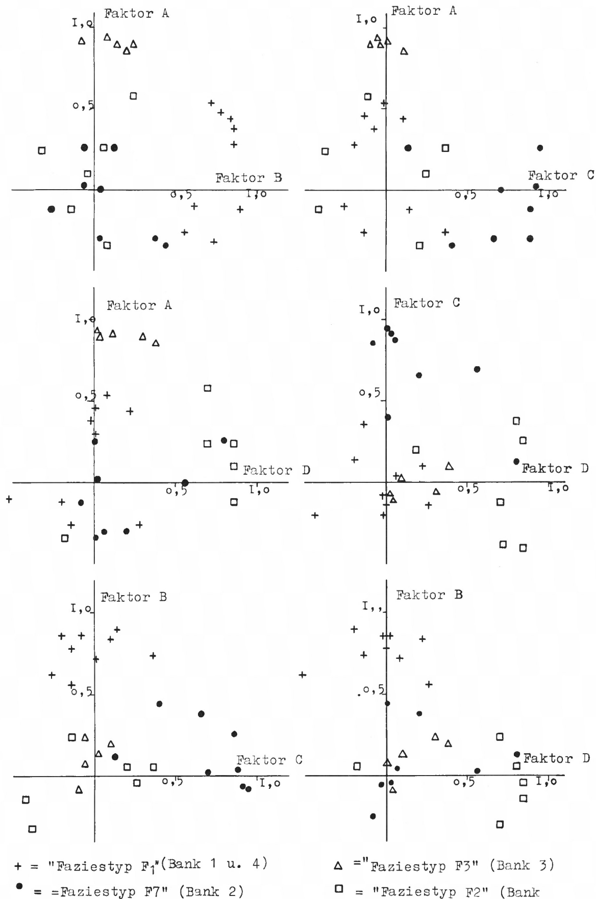
Abb. 26. Rotierte Faktorendiagramme (Korrelationskoeffizienten, normierte Daten) der Faunenelemente im Profil 28 im Steinbruch Steltenberg, Hohenlimburg. Für die Faktoren ergeben sich folgende Anteile an der Gesamtkommunalität in Prozentwerten (in Klammern ist der Anteil an eh^2 (=rotierter Anteil von h^2 ) angeführt): Faktor A 30 (28), Faktor B 11 (27), Faktor C 20 (23) und Faktor D 11 (21). Faziestypen (Geländean-sprachen): F 1 = Biomikrit mit sehr zahlreichen Amphiporen und sehr wenigen anderen Faunenelemen-ten; F 2 = Biomikrit reichem Faunenspektrum, bestehend aus Stromatoporen, Alveoliten, rugosen Einzel-korallen und Thamnoporen u. a.; F 3 = Brachiopoden-Biomikrit; F 7 = Mikrit mit globularen und la-mellaren Stromatoporen in Lebensstellung.
