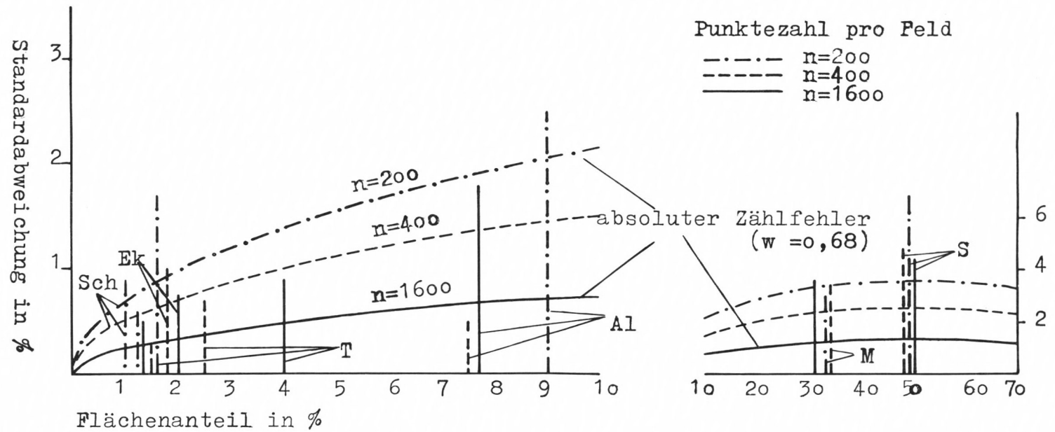
Abb. 16. b) Beeinflussung der Streuung durch die Größe der Stichproben-Felder und durch die Meßpunktezah: Standardabweichung bei konstanter Meßfeldgröße (60 × 60 cm), aber unterschiedlicher Punktezah. Al = Alveoliten, EK = Einzelkorallen, M = Matrix (mikritische Grundmasse mit Feinbiodebitrus), S = Stromatoporen, SCH = Schalen-Reste (meist Brachiopoden), T = Thamnoporen.
