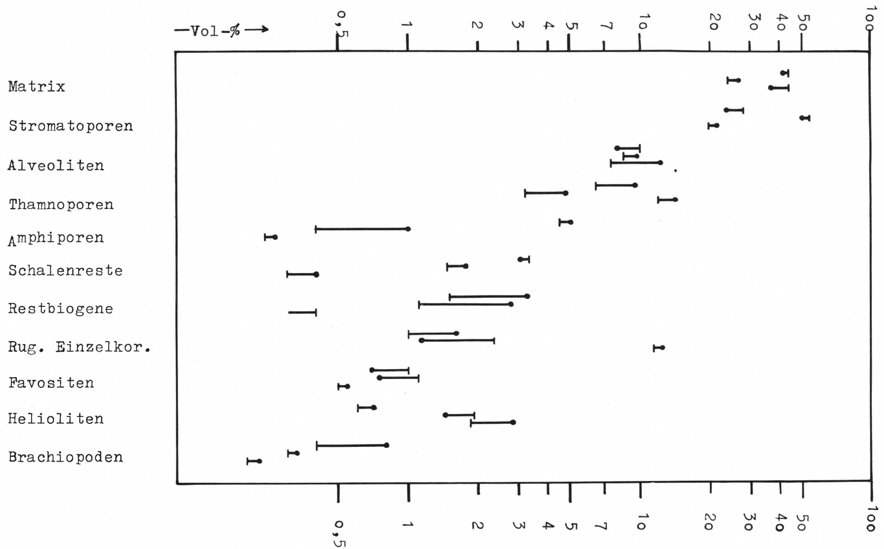
Abb. 17. Abweichungen der Mittelwerte bei Punktauszählung (angedeutet durch Punkt) und Linearmeßmethode (dargestellt durch Querstrich [-]) in 3 Testbereichen. Für jede Komponente gilt: linke Eintragung = Testfeld 2 auf der Schichtfläche in Letmathe, mittlere Eintragung = Testfeld 1 auf der Schichtfläche in Letmathe, rechte Eintragung = Profil P in Letmathe. Die Punktzählmethode liefert genauere Werte.
