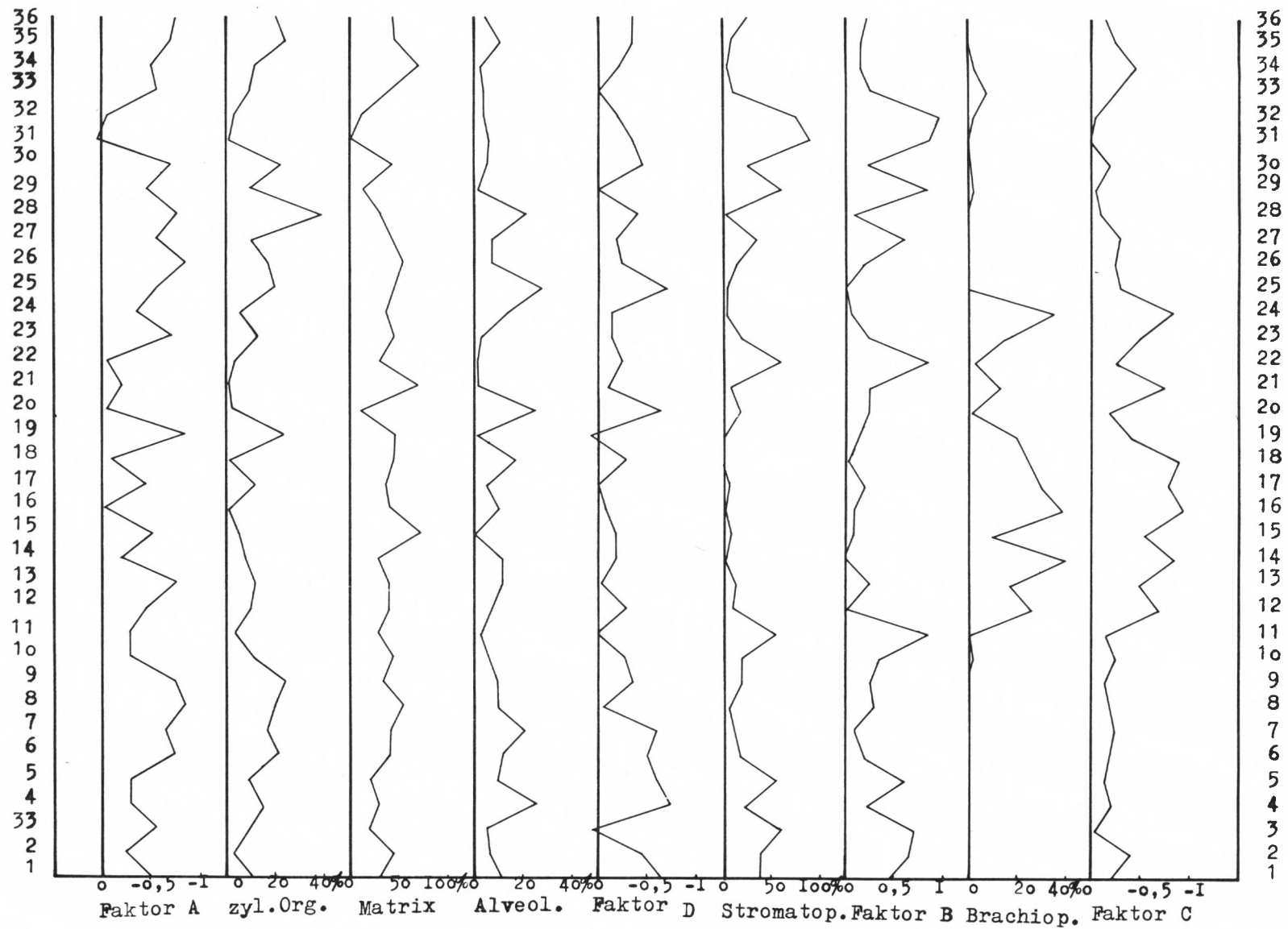
Abb. 25. Faktorenanalyse (Q-Technik) des Profils 36, Letmathe. Säulendiagramme zeigen die Verteilung der Faktorenladungen, der Faunenelemente und der Matrix. Die Kurven bringen die direkte Bindung der Faktoren an einzelne Faunenelemente in den 36 untersuchten Bänken zum Ausdruck. Faktorenanalyse unter Verwendung von normierten Daten und \cos\Phi -Koeffizienten.
