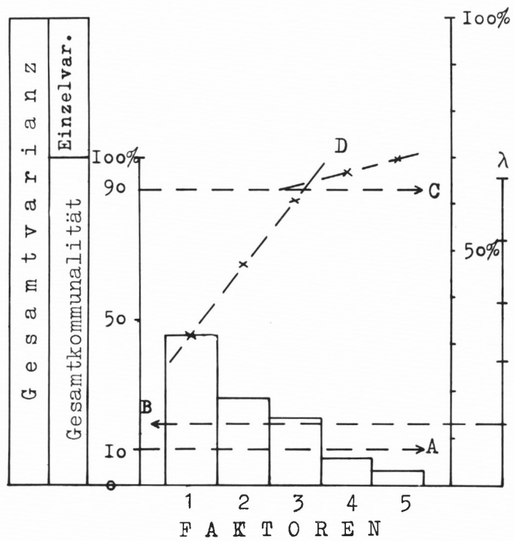
Abb. 18. Bestimmung der Zahl der zu extrahierenden Faktoren am Beispiel des Profils P im östlichsten Steinbruch S der Lenne in Letmathe.
