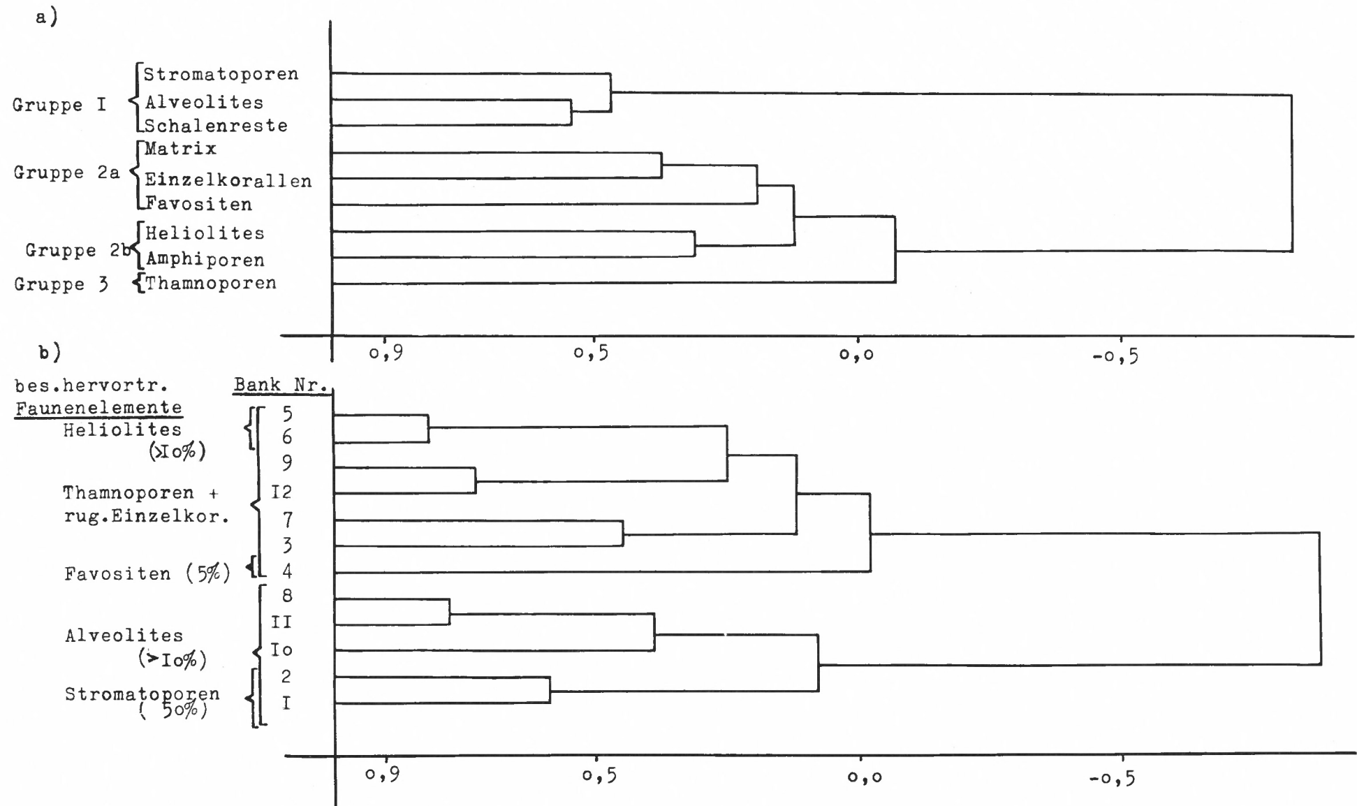
Abb. 22. Clusterdiagramm von Fauna und Bänken des Profils P, östlichster Steinbruch S der Lenne, berechnet aus der Korrelationsmatrix. Ausgangsdaten sind die standardisierten Prozentwerte der Linearauszählung. a) R-Technik, b) Q-Technik.
