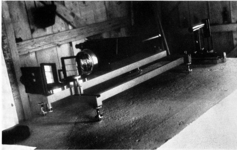
Fig. 10. Lichtquelle und Meßfernrohr
