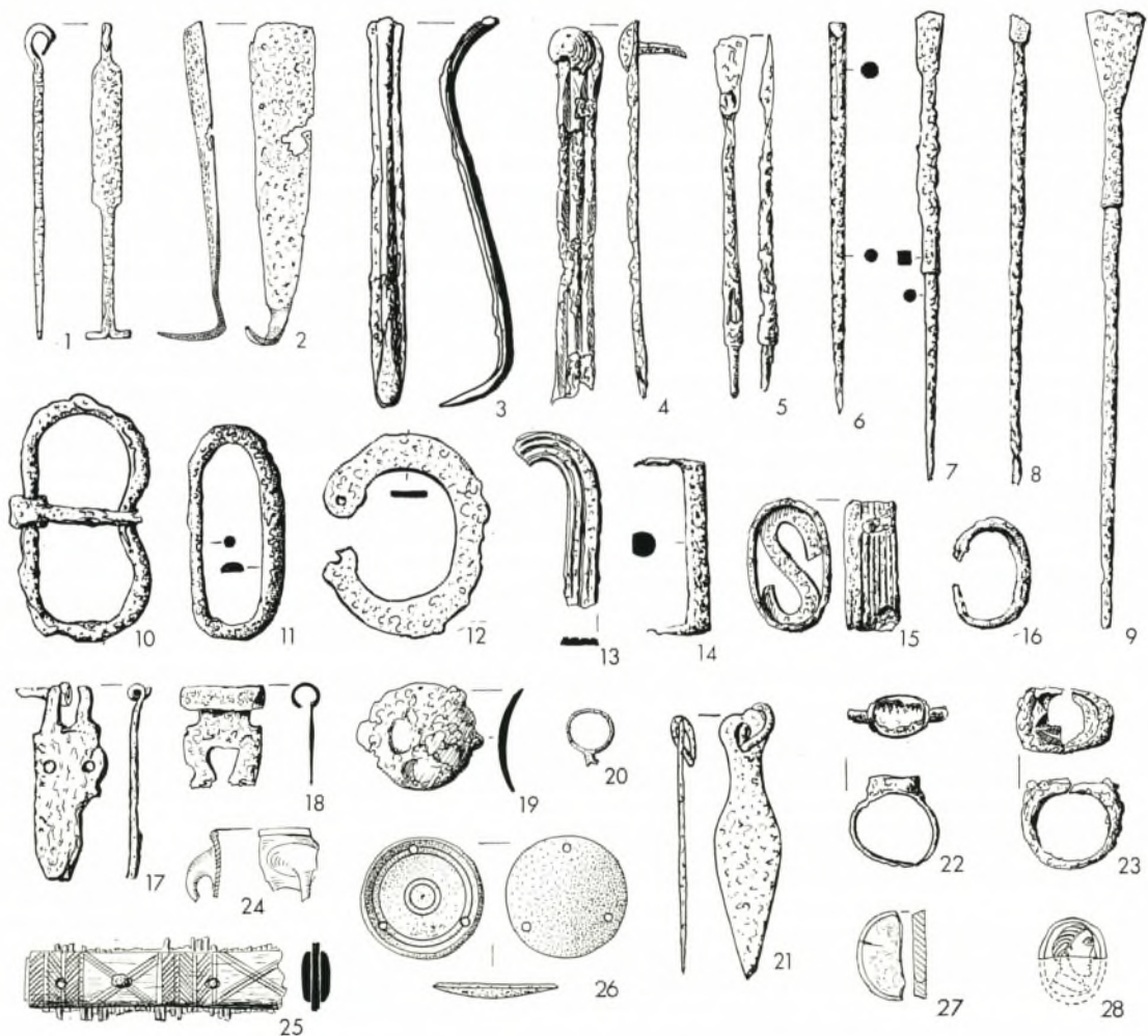
Objekte aus Eisen (1-23), Glas (24, 27-28), Knochen (25) und Bronze (26). M. 2:3. 1-2, 5-9 vgl. S. 191; 3-4, 15 vgl. S. 193; 10-14, 16-23 vgl. S. 187; 24 vgl. S. 179; 25 vgl. S. 182; 26 vgl. S. 186; 27-28 vgl. Taf. 53, 10-11 u. S. 283 f.
