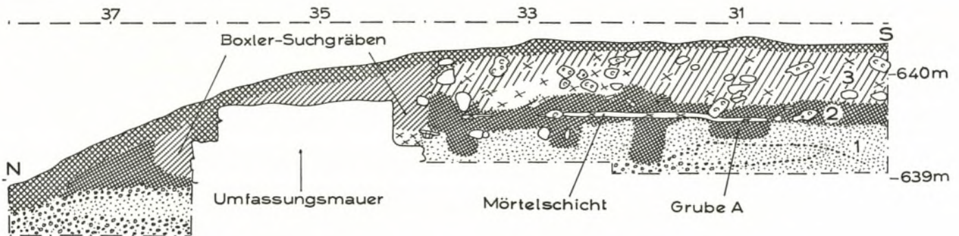
Abb. 16. Schnitt k. Ostprofil. In Grube A Münze Diocletian M 94. M. 1:50.
