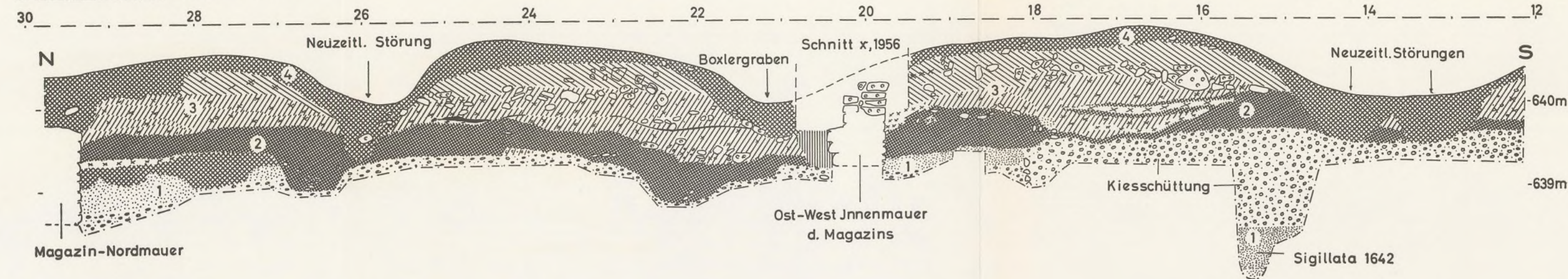
Schnitt mm, ll, ee, Ostprofil 1:50
