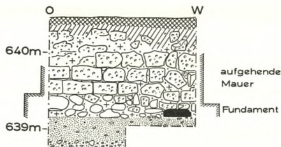
Abb. 18. Schnitt h. Außenansicht der Umfassungsmauer. M. 1: 50.
