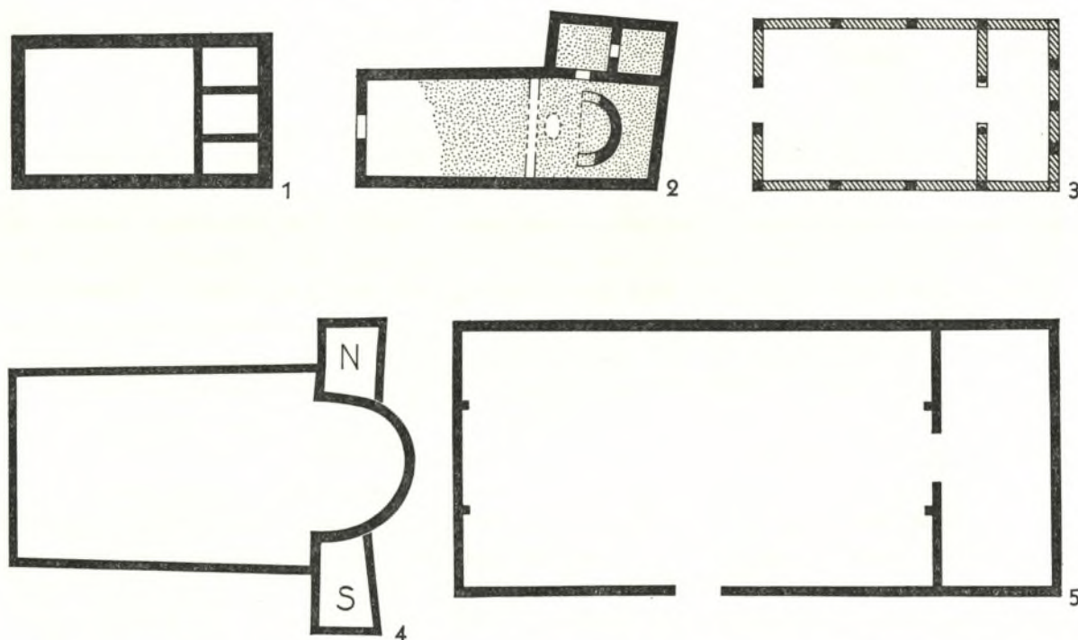
Abb. 73. 1 Lorenzberg, 2 Lauriacum (nach R. Noll), 3 Henchir el Atech (nach H. Lehner), 4 Kaiseraugst (nach R. Laur-Belart), 5 Kékkút (nach Arch. Ért. 45, 1931, 32 Abb. 20) M. 1:400.
