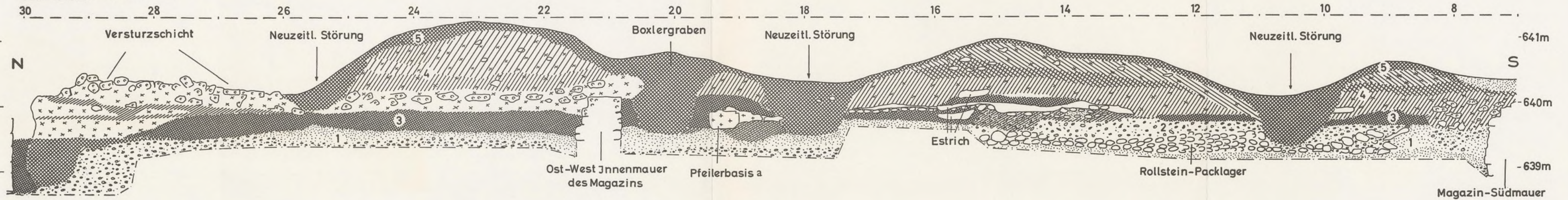
Schnitt gg, Ostprofil 1:50
