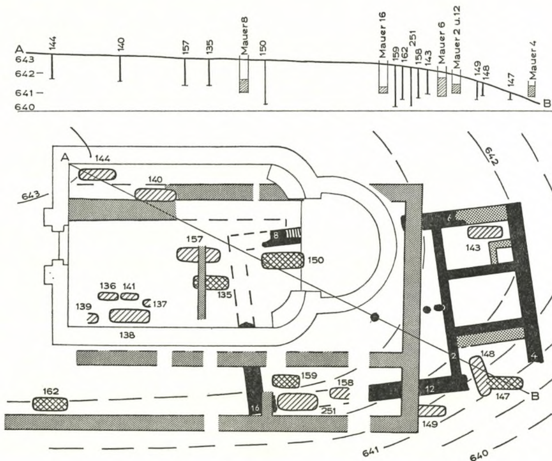
Abb. 72. Orientierung und Tiefe von Mauern und Gräbern im Bereich der Lorenzkapelle. M. 1:200. Beigabeführende Gräber kreuzschraffiert. Linie A–B Projektionsebene der heutigen Oberfläche zwischen A und B.
