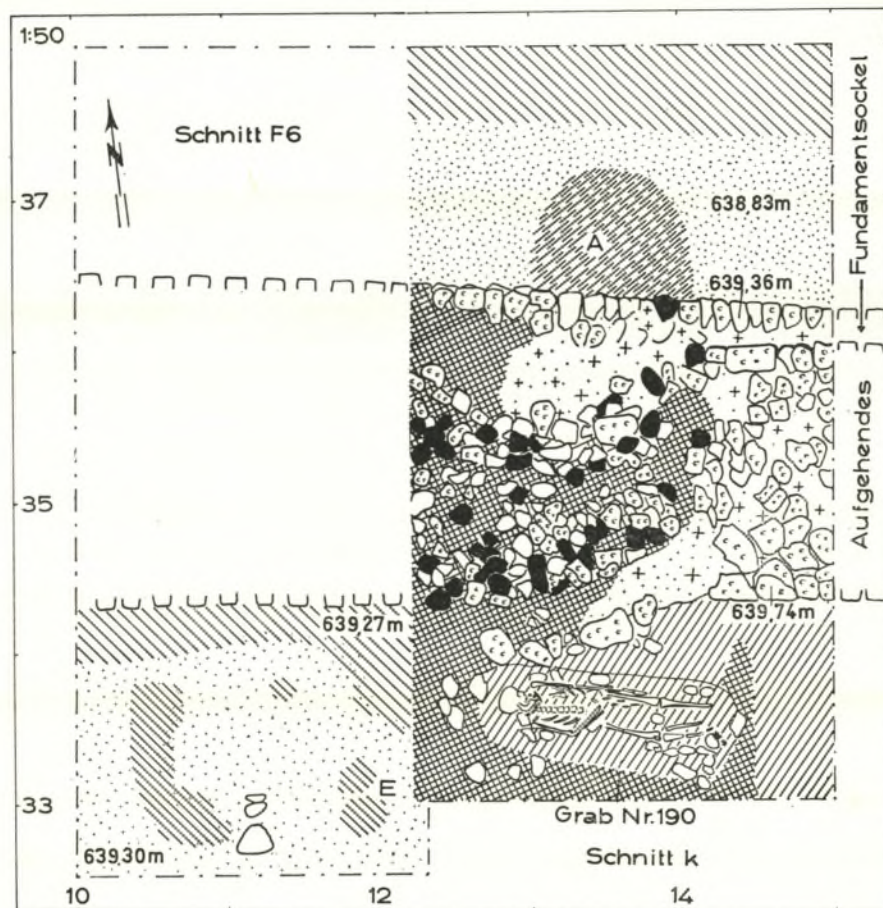
Abb. 14. Schnitt k und F 6. Planum mit Umfassungsmauer (schwarz: verbrannte Tuffsteine). M. 1:50.
