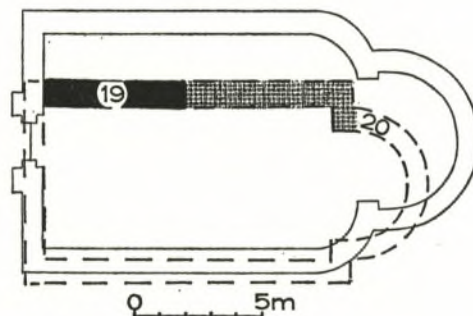
Abb. 75. Bau III. M. 1:300.
