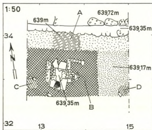
Abb. 15. Schnitt k. Planum mit frühromischer Grube (A), Herdstelle (B) und Pfosten (C–D). M. 1:50.
