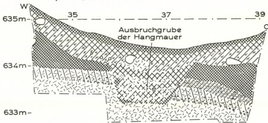
Schnitt H 2, Nordprofil 1:50
