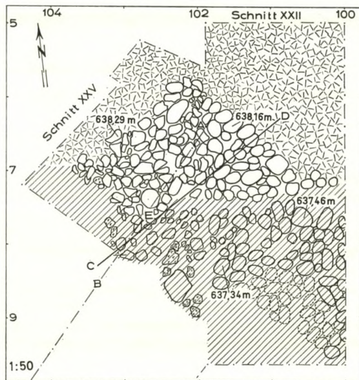
Abb. 5. Schnitt XXII/XXV. Südliche Torwange der Umfassungsmauer. M. 1:50.
