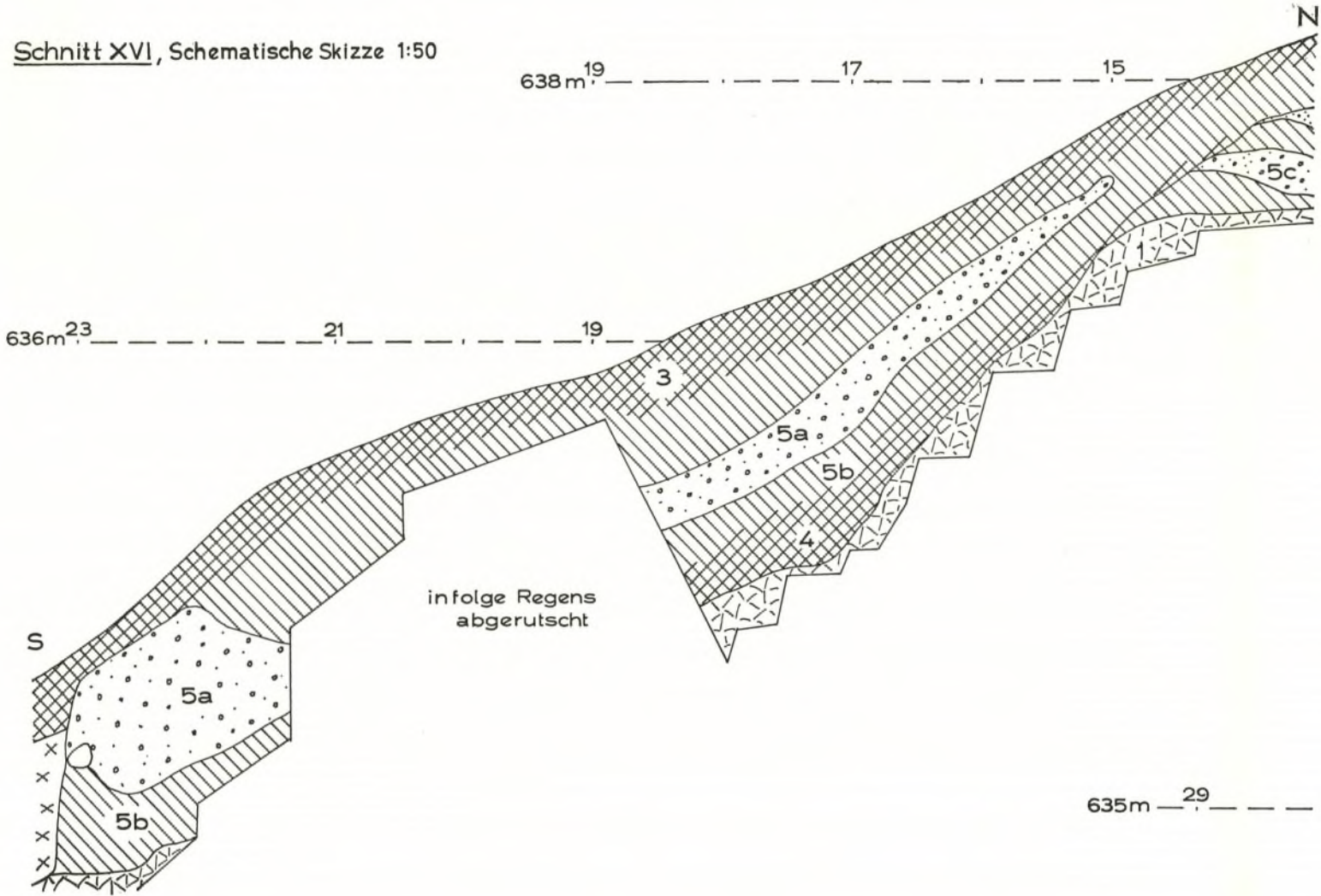
Schnitt XVI, Westprofil 1:50
