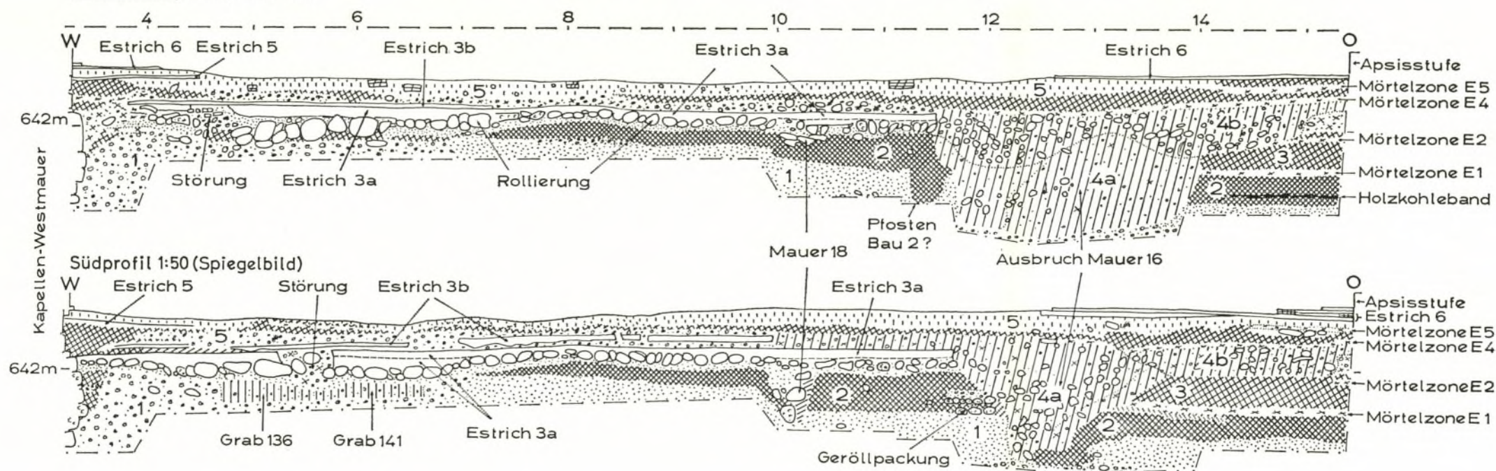
Schnitt K1, Nordprofil 1:50
