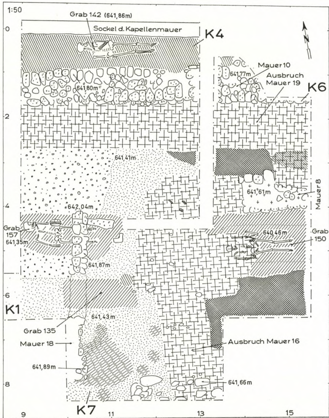
Abb. 63. Schnitt K 1, 4, 6, 7. Planum. M. 1:50.
