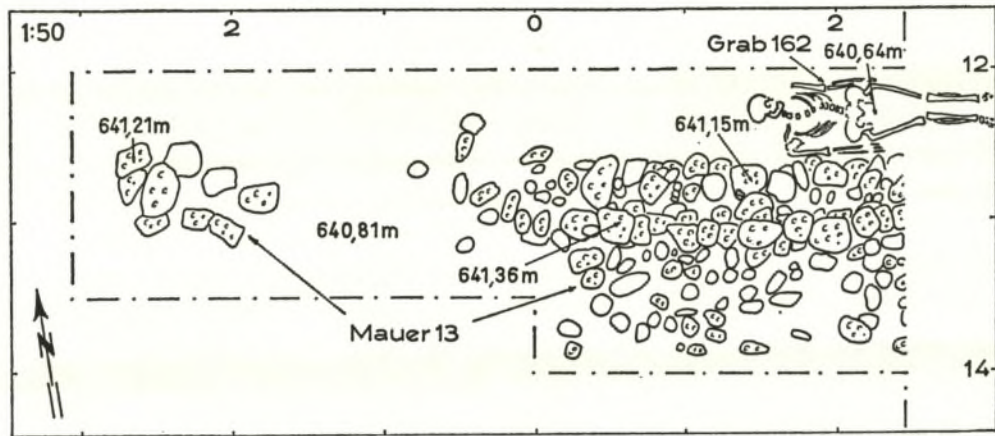
Abb. 69. Schnitt K 10, Erweiterung. Planum. M. 1:50.
