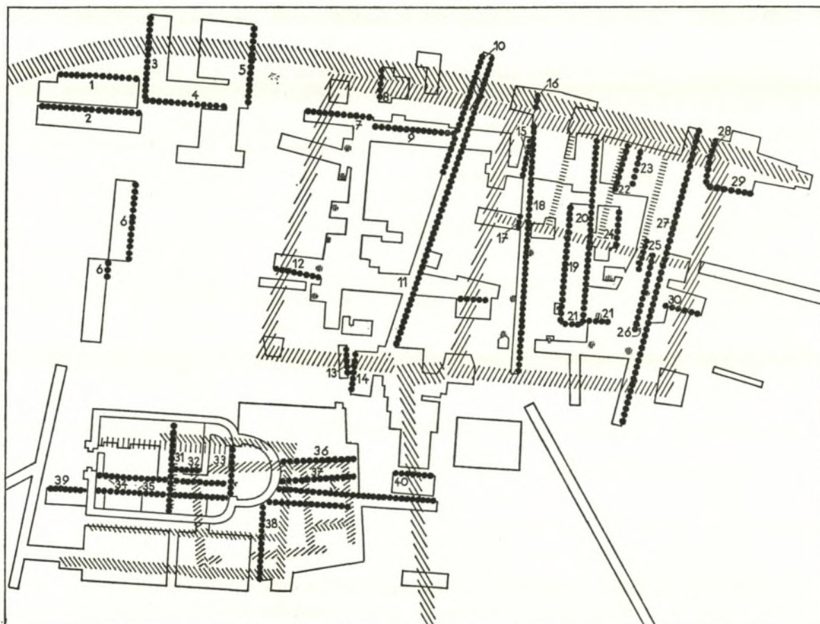
Abb. 23. Übersichtsplan der abgebildeten Profile im Bereich von Kirche und Magazingebäude. M. 1 : 500.
