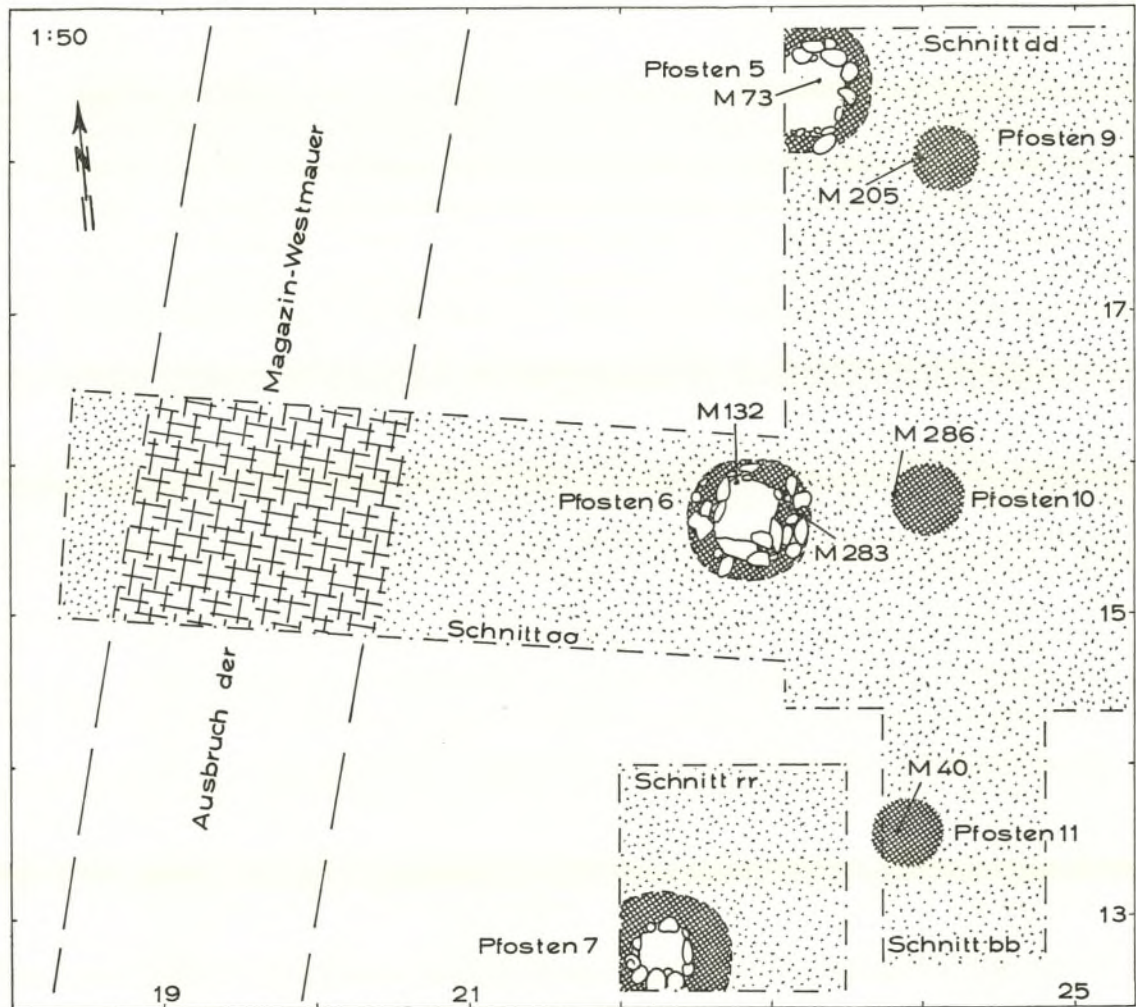
Abb. 36. Schnitt aa/bb/oo/rr. Planum mit Pfosten 5–7 und 9–11 in Raum A (Hof). M. 1:50.
