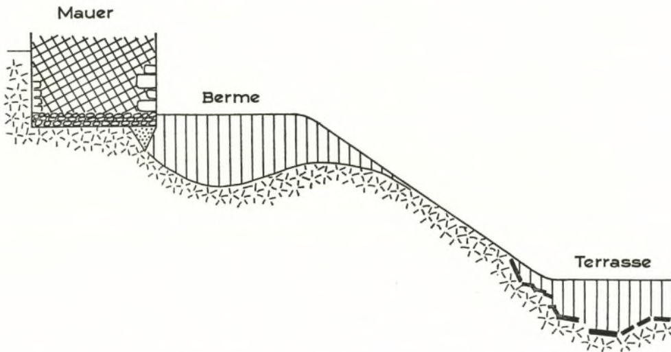
Abb. 22. Schematische Rekonstruktion von Umfassungsmauer und Berme nach Schnitt XXVI (vgl. Texttaf. B). M. 1: 100.
