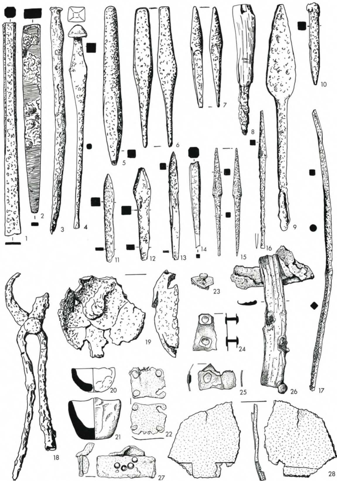
Werkzeug und Geräte aus Eisen (1–19), Gußtiegel aus Ton (20–21) und Bleche aus Bronze (22–28). M. 1:2. 1–19 vgl. S. 190 f.; 20–21 vgl. S. 174; 22–28 vgl. S. 186.
