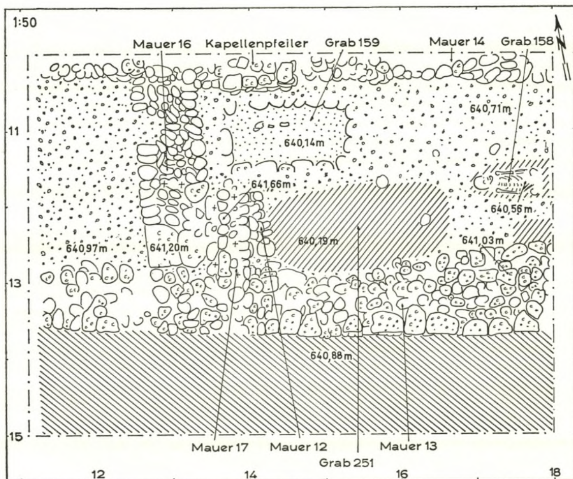
Abb. 61. Schnitt K 8. Planum. M. 1:50.
