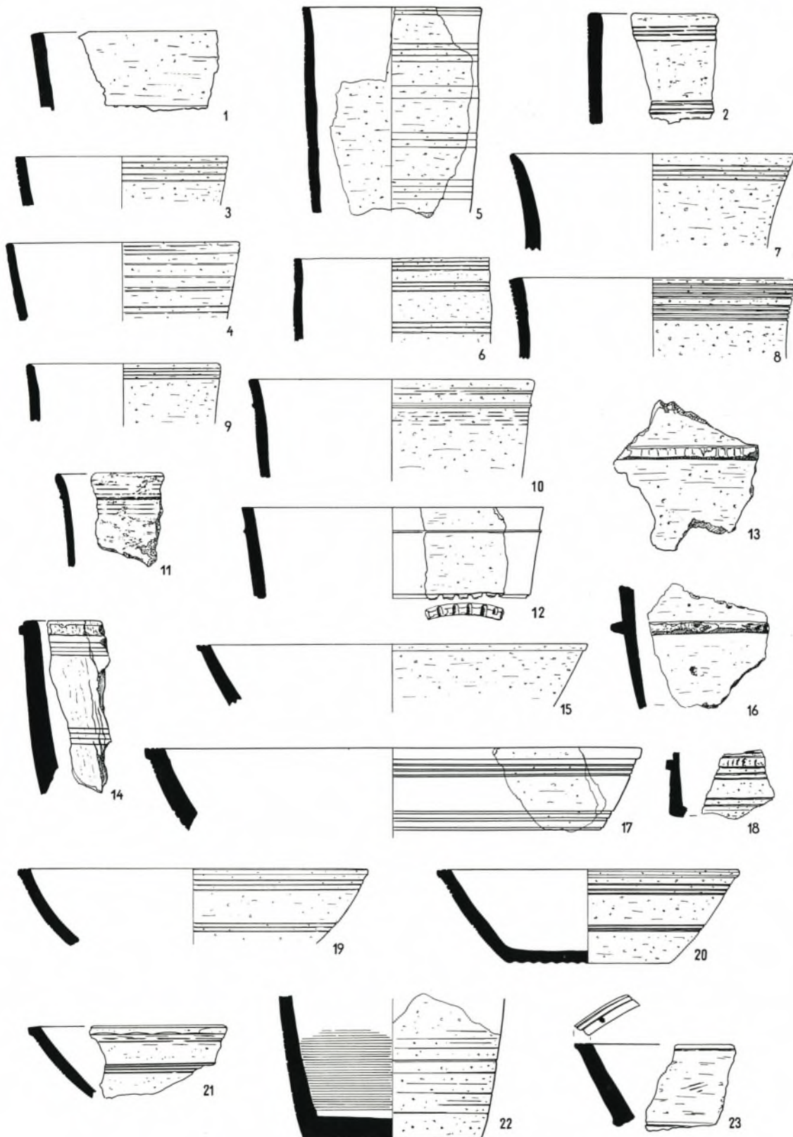
Becher und Schalen aus Lavez. M. 1:3. Vgl. S. 176 f.
