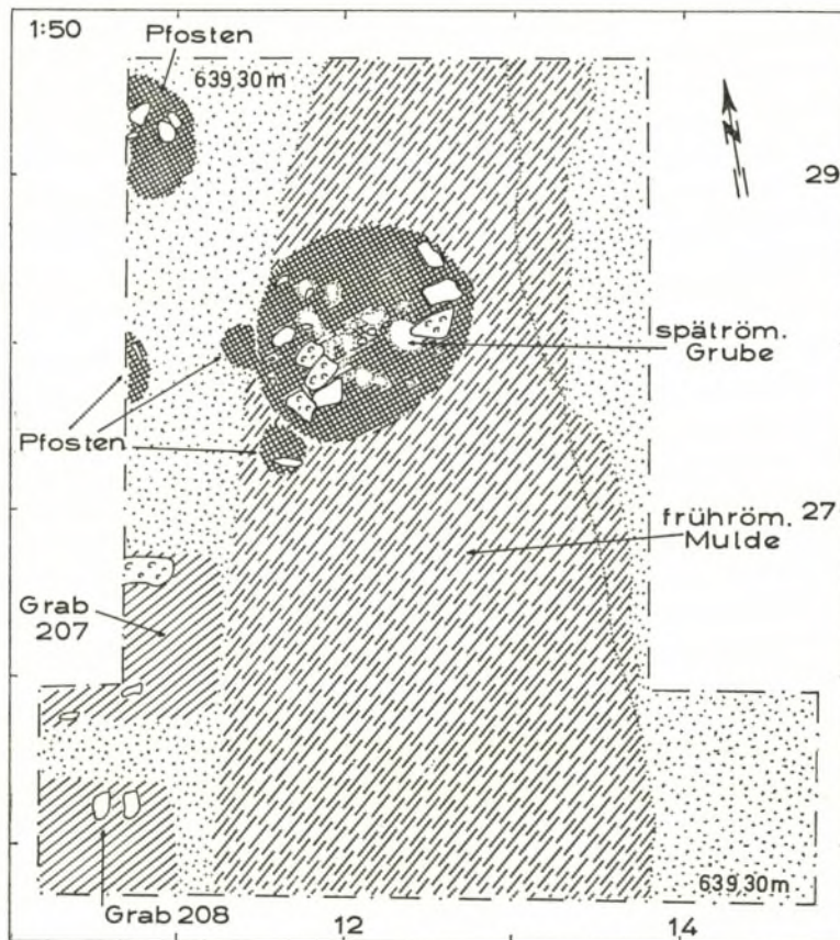
Abb. 51. Fläche F 4. Planum. M. 1:50.
