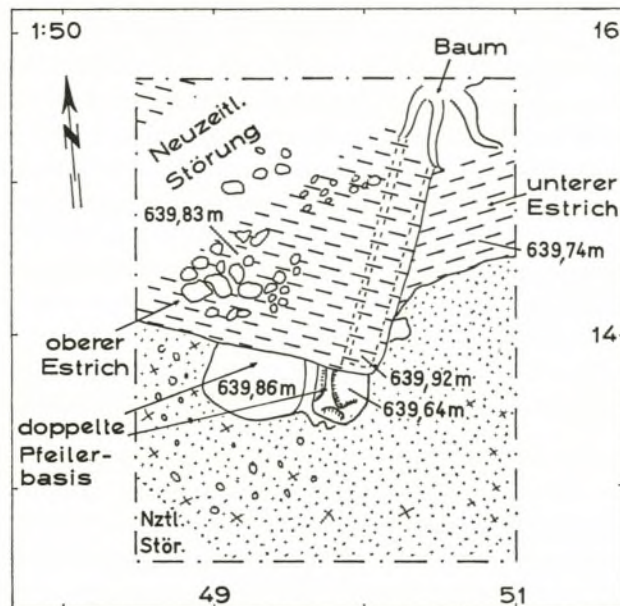
Abb. 43. Fläche nn. Planum mit Pfeilerbasis g und Estrichüberschneidung. M. 1:50.
