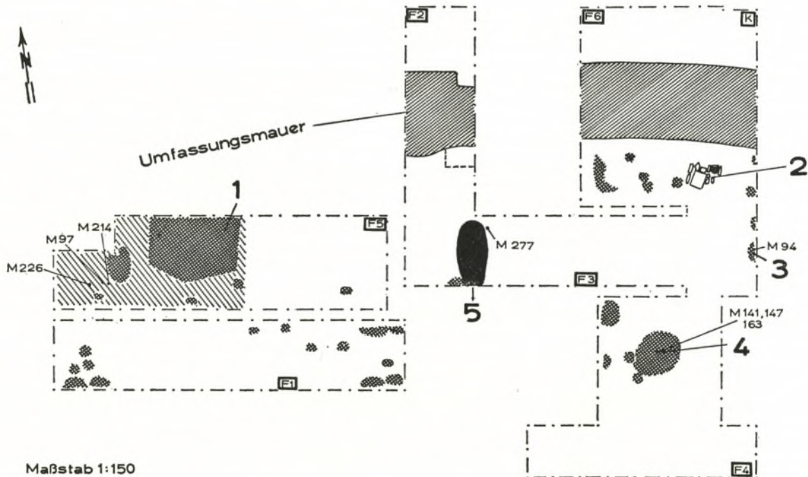
Abb. 52. Spätromische Siedlungsspuren westlich des Magazingebäudes. 1 Haus mit Grube und Herdstelle, 2 Herdstelle, 3 Grube, 4 Grube, 5 Feuerstelle. M. 1:150.
