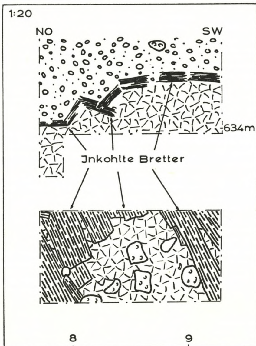
Abb. 4. Schnitt XXVI. Bretterlagen im Profil und Planum zwischen 7,70 m und 9,30 m SW. M. 1: 20.
