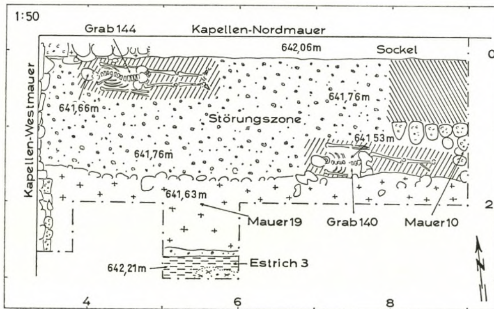
Abb. 66. Schnitt K 3. Planum. M. 1:50.
