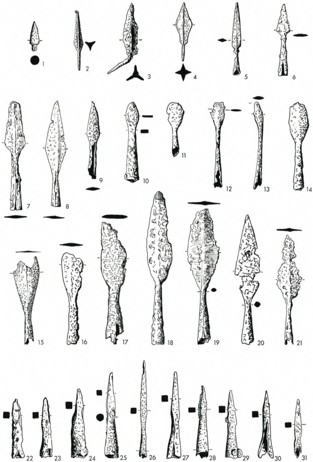
Pfeilspitzen aus Eisen. M. 1:2. Vgl. S. 188 f.
