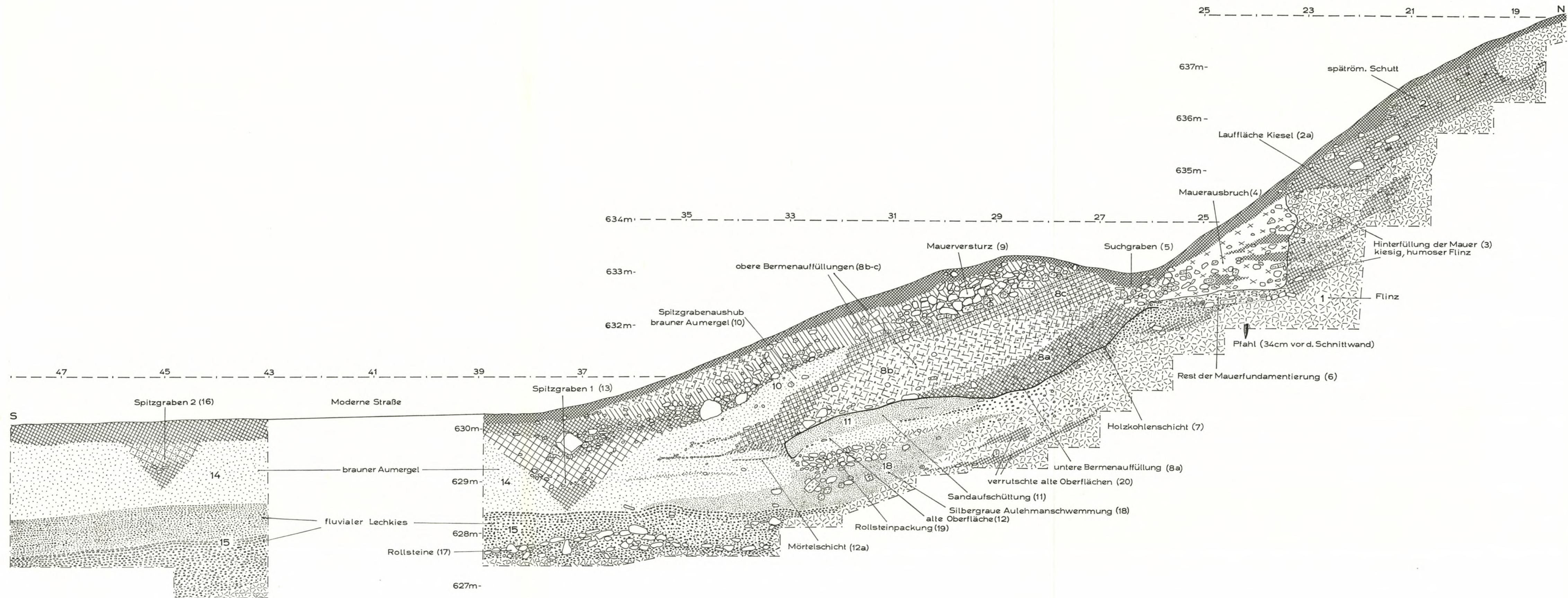
Schnitt I, Westprofil. M. 1:50.
