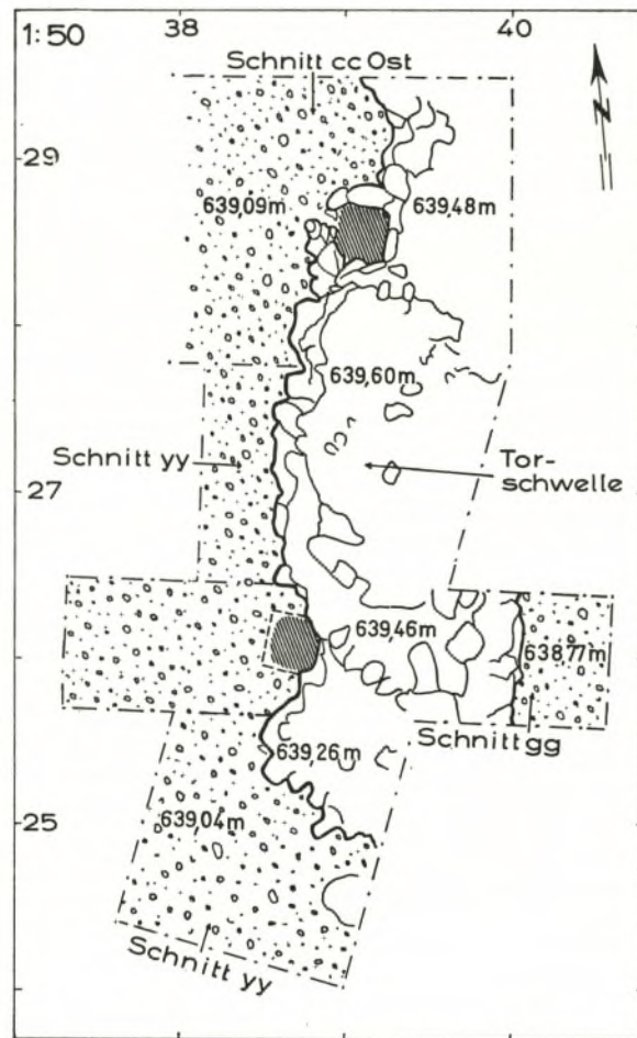
Abb. 32. Schnitt cc/gg/yy. Planum mit Türpfosten 14 und 15 und Schwelle. M. 1:50.
