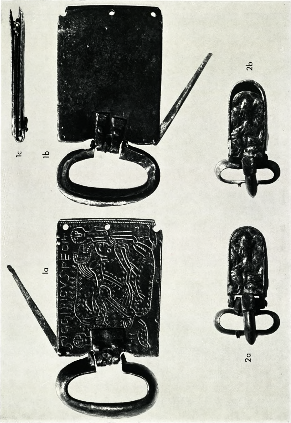
Verschließbare Reliquiarschnallen von Gondorf (1) und von Prizzi in Sizilien (2). Messing bzw. Bronze. M. 1 : 1.
