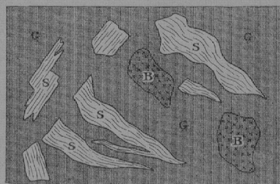
Gneisseinschlüsse (S) und basische Ausscheidungen (B), im Granit (G), am Habachkees. Maassstab ca. 1:15.
