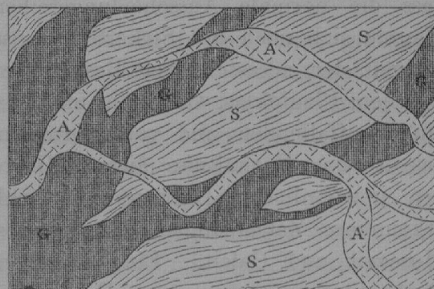
Apophysen von Centralgranit (G) und Gänge von Aplit (A) in Amphibolit (S). Weisseneck im obersten Hollersbachthal. Maassstab ca. 1:30.
