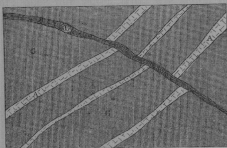
Ein Zug paralleler Gänge von Aplit (A), verworfen von einem schmalen basischen Gang (L). Im Granit (G), am Untersulzbachkees. Maassstab ca. 1:35.
