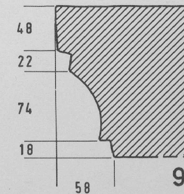
FRAUENCHIEMSEE, TORBAU Kämpferprofile der Arkaden und Durchgänge Stand 1962. Maße in Millimeter M. 1 : 4
