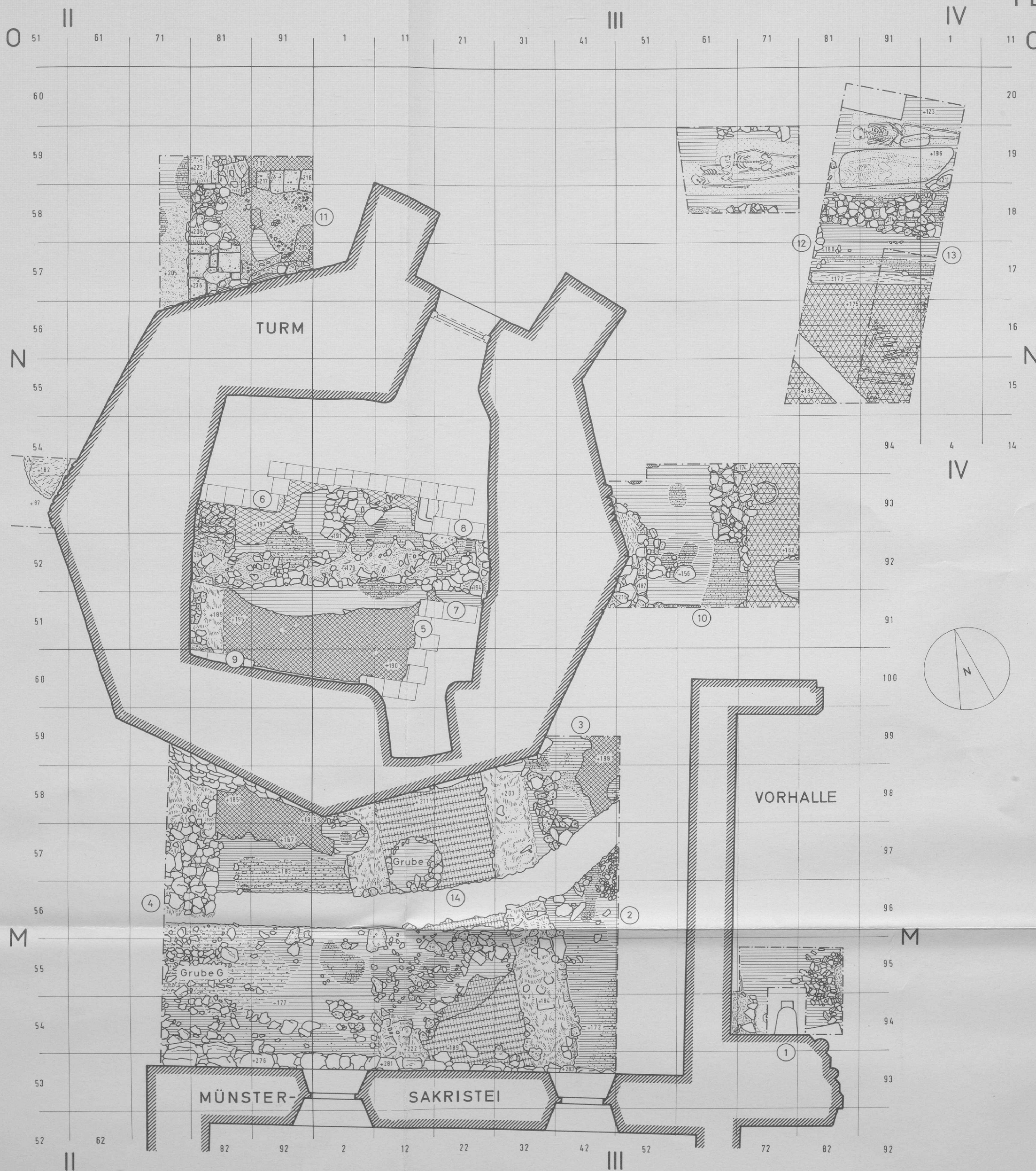
FRAUENCHIEMSEE, SAKRISTEI-TURM Schnitte im Turm und um den Turm Stand 1961 - 1963
