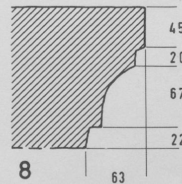
FRAUENCHIEMSEE, TORBAU Kämpferprofile der Arkaden und Durchgänge Stand 1962. Maße in Millimeter M. 1 : 4
