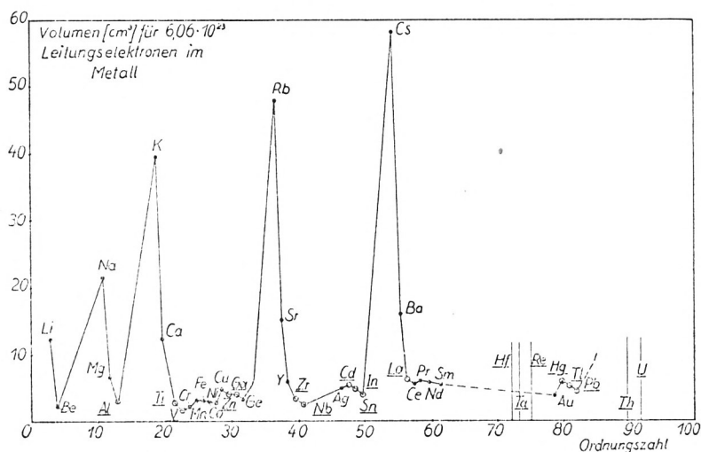
Abb. 2. Supraleiter (unterstrichen) und Volumen für Leitungselektronen.
