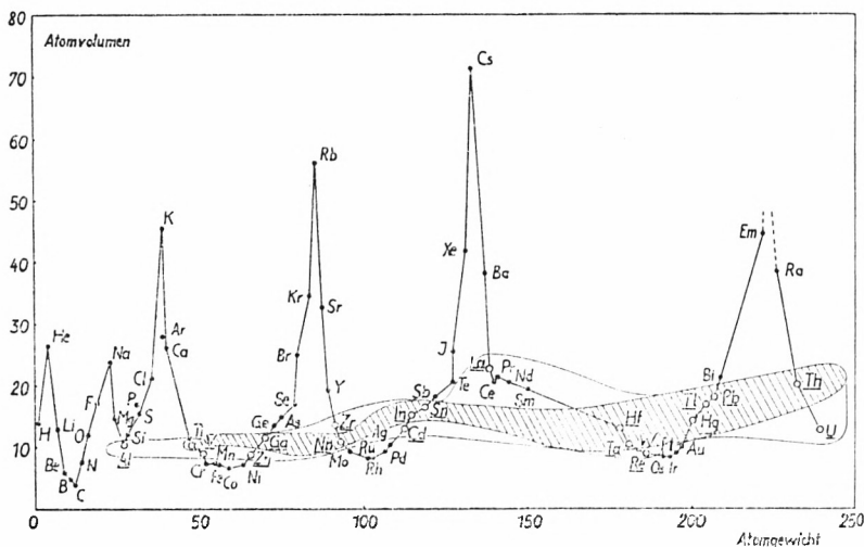
Abb. 1. Supraleiter (unterstrichen) und Atomvolumen.
