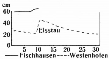
Fig. 3 Vergleich der Wasserstände von Fischhausen und Westenhofen, Januar 1914
