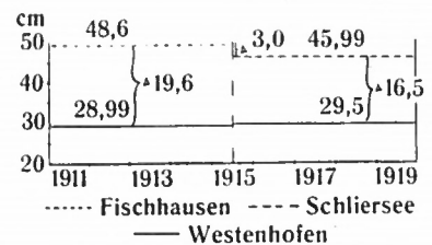
Fig. 8 P.N.-Bestimmung des Pegels Fischhausen
