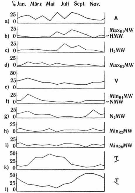
Fig. 2. Würmsee (1908-1950, ohne 1945)
