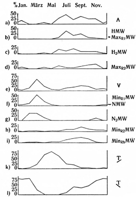
Fig. 2. Walchenseestaubecken (1924-1950)
