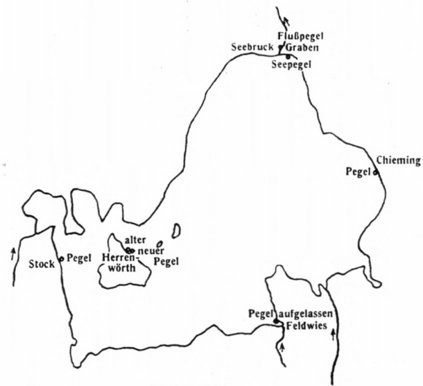
Fig. 3. Chiemsee
