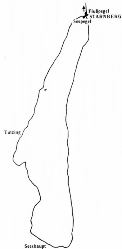
Fig. 2. Würmsee
