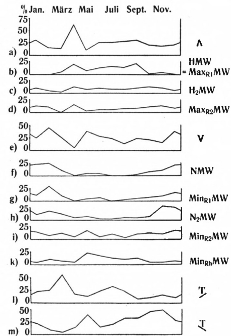
Fig. 3. Schliersee (1912-1950)
