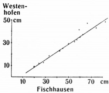
Fig. 2 Bezugslinie der Wasserstände von Fischhausen und Westenhofen
