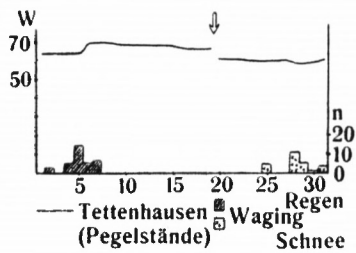
Fig. 1 Niederschlag und Wasserstand am Waginger See im Dezember 1938
