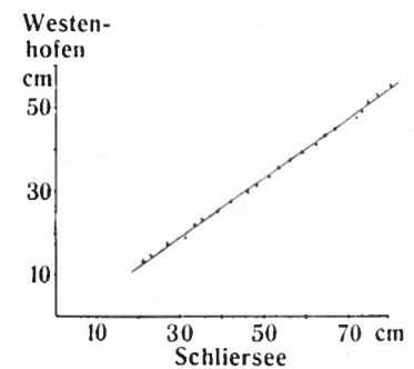
Fig. 6 Bezugslinie der Wasserstände von Schliersee und Westenhofen
