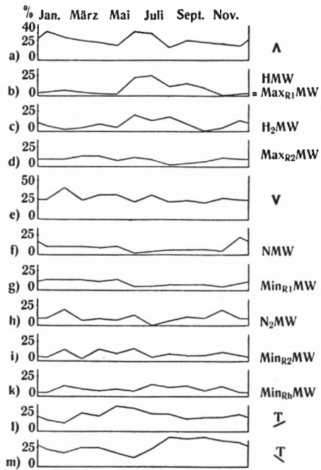
Fig. 3. Simssee (1907-1950)
