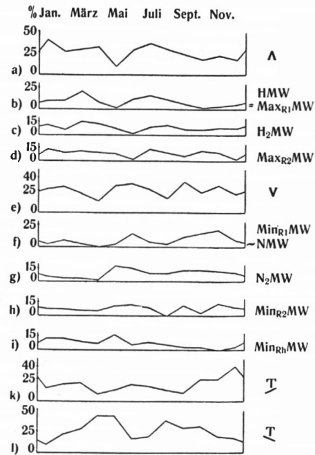
Fig. 4. Waginger See (1901-1950)
