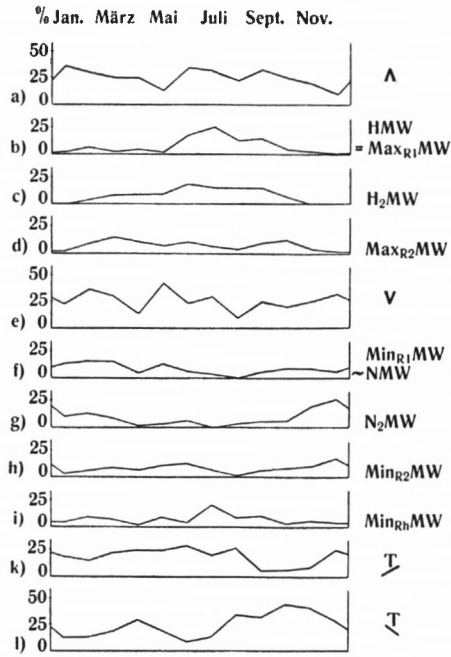
Fig. 1. Staffelsee (1909-1950)
