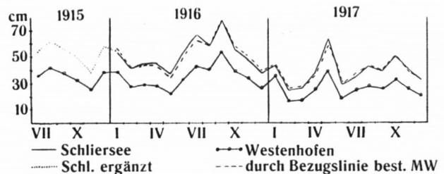
Fig. 7. Vergleich von Bezugswerten und reellen Monats- mittelwerten von Schliersee und Westenhofen, 1915-1917
