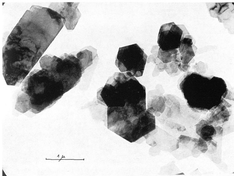
1. Elektronenmikroskopisches Bild eines technisch verwerteten Kaolins, das die (pseudo)hexagonalen Blättchen des Kaolinites zeigt.
