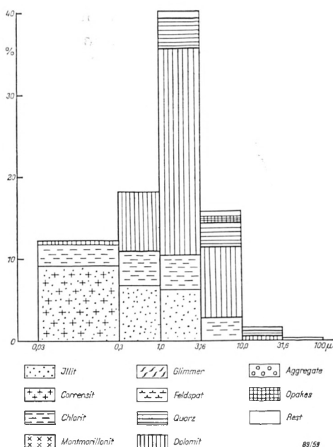
Abb. 6. Kornverteilung und Mineralgehalt einer Tonprobe aus dem Gipskeuper. („Irex“-Bohrung bei Kulmbach in 145–148 m Tiefe nach H. H. Schmitz, Geol. Jahrb. 77, 1959, 88).
