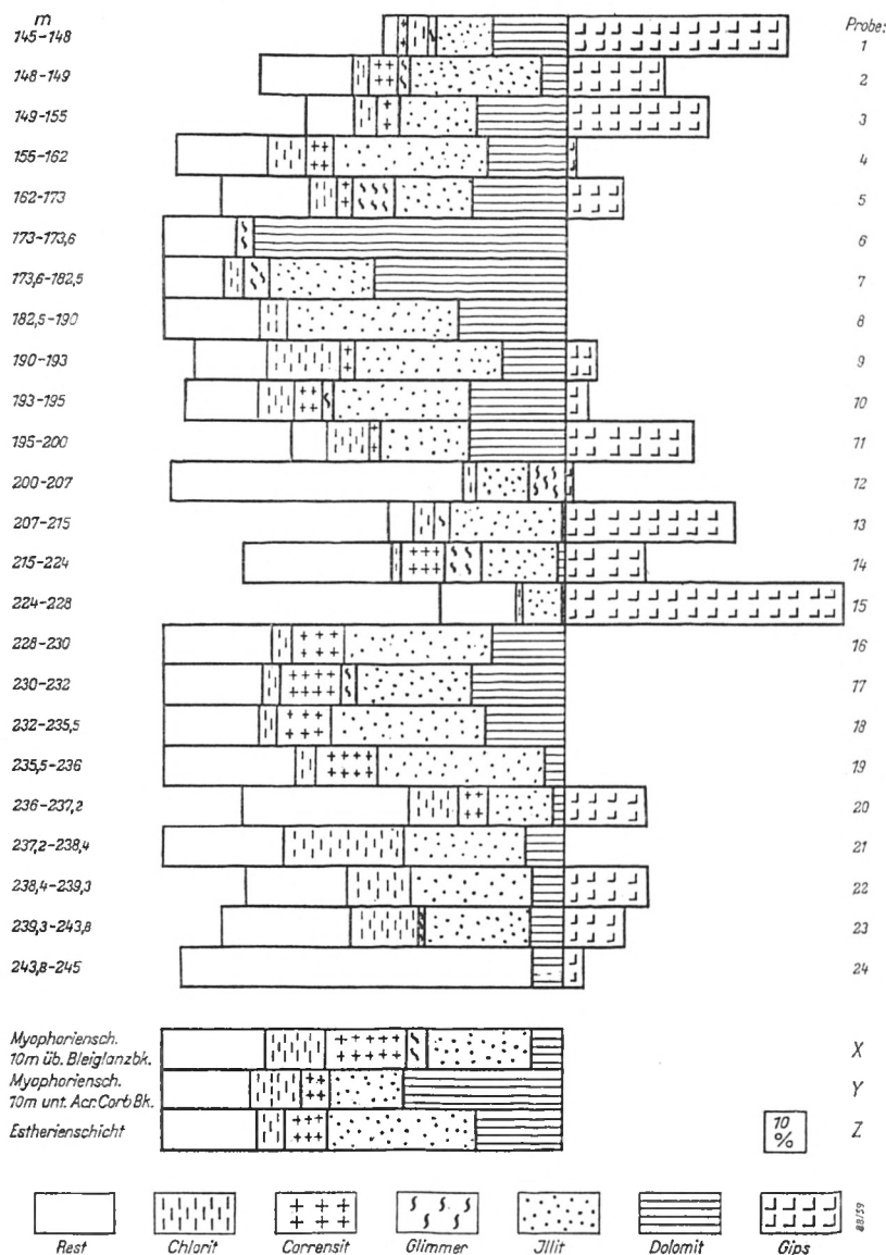
Abb. 7. Die mittlere Verteilung der Minerale in den Proben des Gipskeupers der „Irex“-Bohrung von 145-245 m Tiefe nach H. H. Schmitz
