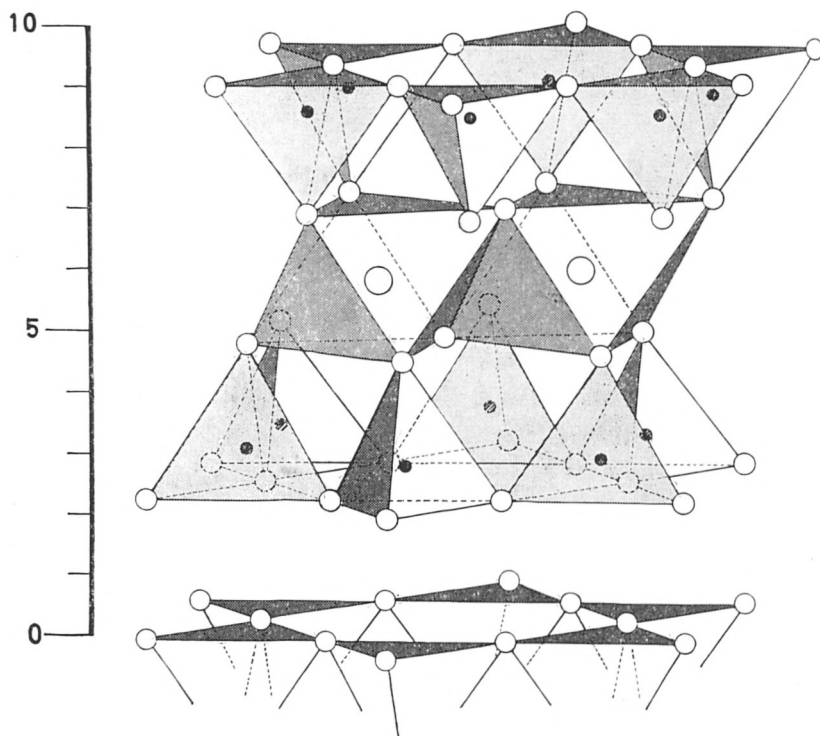
Abb. 3. Darstellung des Elementarbereiches des Montmorillonites.
