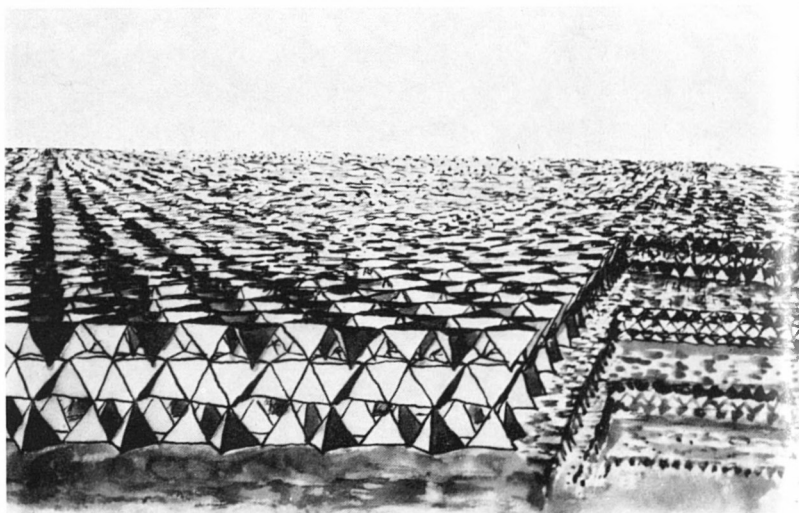
2. Übersichtsbild der Kristallstruktur des Montmorillonites nach einer Zeichnung von W. Forkel. Dargestellt ist eine Folge von Schichten; jedes Schichtpaket besteht aus einer Oktaederschicht, die beiderseitig von Tetraederschichten umgeben ist. Der Aufbau der Tetraeder und Oktaeder entspricht weitgehend demjenigen des Kaolinites.
