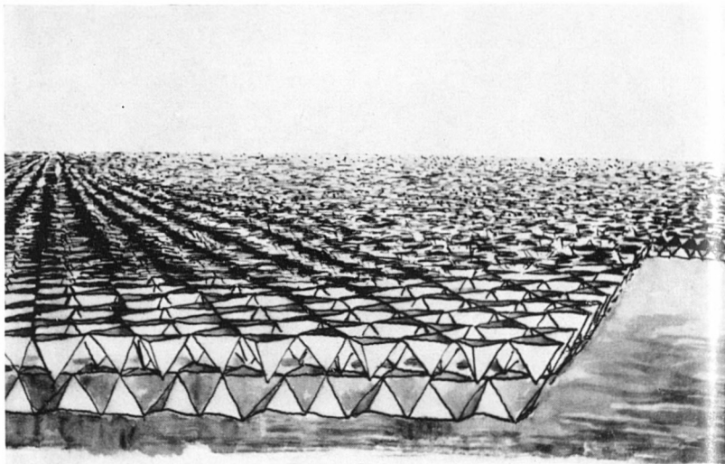
1. Übersichtsbild der Kristallstruktur des Kaolinites nach einer Zeichnung von W. Forkel. Dargestellt ist ein Schichtpaket mit einer „Tetraederschicht“ (oben) und einer „Oktaederschicht“ (unten). Im Inneren eines Tetraeders ist ein Silizium-Atom zu denken, an den Ecken der Tetraeder sitzen Sauerstoff-Atome; in jedem Oktaeder wird ein Aluminium-Atom von Sauerstoff-Atomen und Hydroxyl-(=OH)-Gruppen oktaedrisch umgeben.
