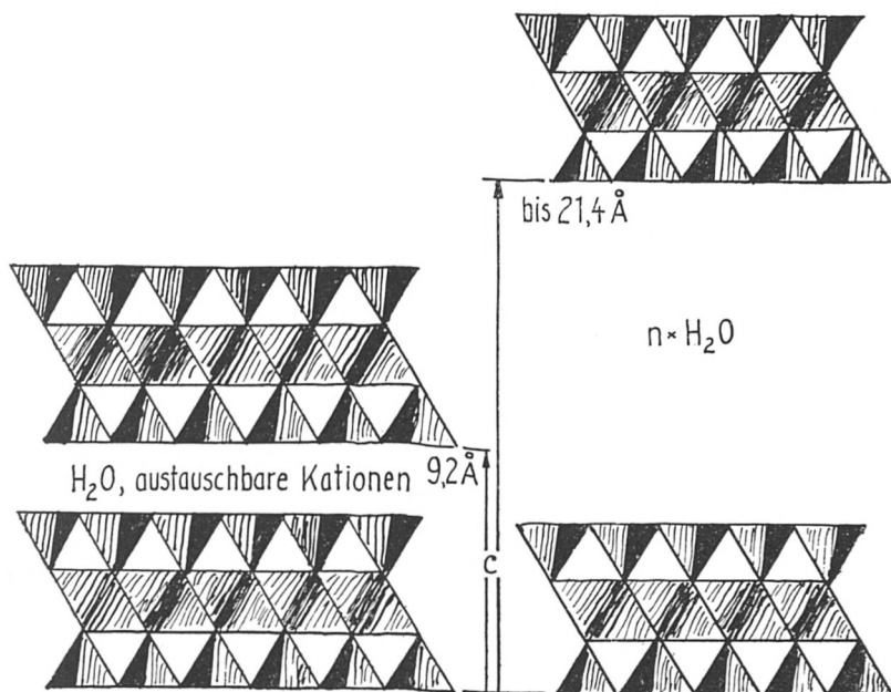
Abb. 4. Der schematische Aufbau des Montmorillonites ist in zwei verschiedenen Stadien der Quellung dargestellt, links mit einem Minimalabstand der Schichten, rechts bei stärkster Quellung. Zwischen den Schichten sind eingebaute Wassermoleküle zu denken.
