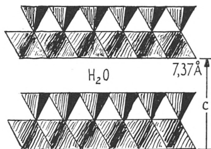
Abb. 2. Die Aufeinanderfolge von Kaoliniteschichten ist im Querschnitt senkrecht zur Schicht schematisch dargestellt.
