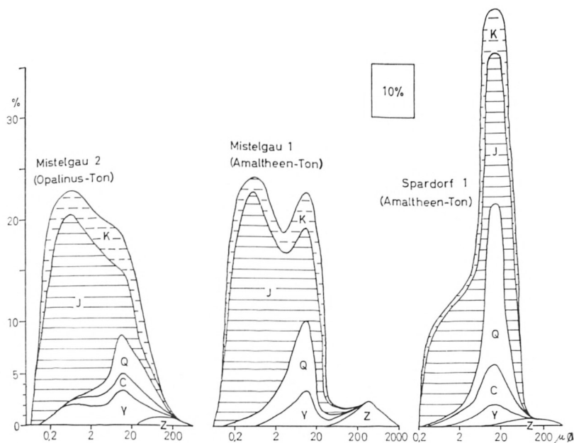
Abb. 9. Kornaufbau und Mineralbestand repräsentativer Proben aus dem Opalinuston und Amaltheenton Frankens nach H. H. Krumm.
