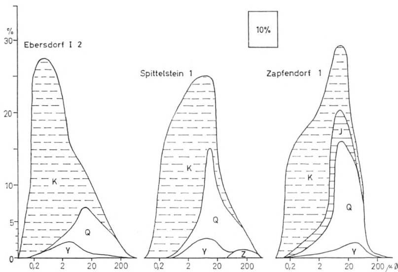
Abb. 8. Kornaufbau und Mineralbestand repräsentativer Proben aus den Rät-Lias-Übergangsschichten Frankens nach H. H. Krumm. K = Kaolin-Gruppe, I = Glimmerartige Minerale; Q = Quarz, Y = Rest (Gips, seltene Feldspatreste, Schwerminerale, Fossilreste, organische Substanzen und opake Minerale).
