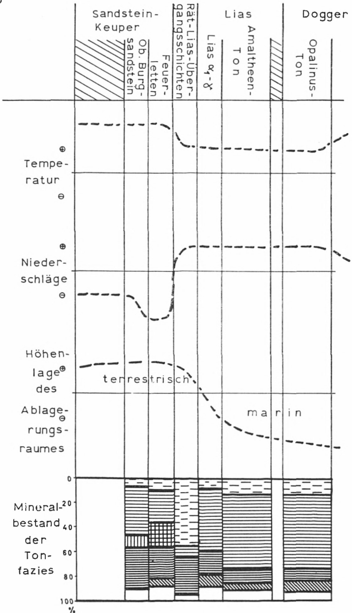
Abb. 10. Gemeinsame Darstellung über die Beziehungen von Klima, Ablagerungsraum und Mineralbestand in den untersuchten Schichten vom Sandsteinkeuper bis zum Opalinuston in Franken nach H. H. Krumm. Horizontal gestrichelt: Kaolingruppe; weit schraffiert: Glimmerartige Minerale; eng schraffiert: Quarz, vertikal schraffiert: Montmoriningruppe; quadriert: Illit-Montmorillonit; schräg schraffiert: Karbonate; weiß: Rest.
