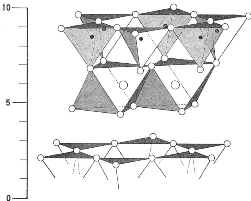
Abb. 1. Darstellung eines kleineren Bereiches der Kristallstruktur des Kaolinites bei stärkerer Vergrößerung gegenüber Abb. 3. Die Kenntnis dieser sogenannten Elementarzelle genügt, um den gesamten Aufbau der Kristalle zu verstehen. Die Kreise stellen die Schwerpunkte der einzelnen Atome dar. 1 \text{ \AA} = 10^{-8} \text{ cm.}
