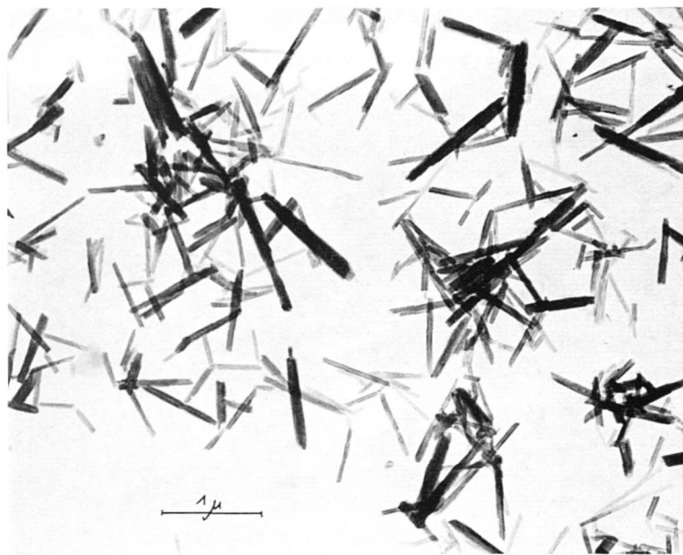
2. Elektronenmikroskopisches Bild eines Tones mit Halloysit von Djebel Debar mit Röllchen-Textur der einzelnen Kristalle.
