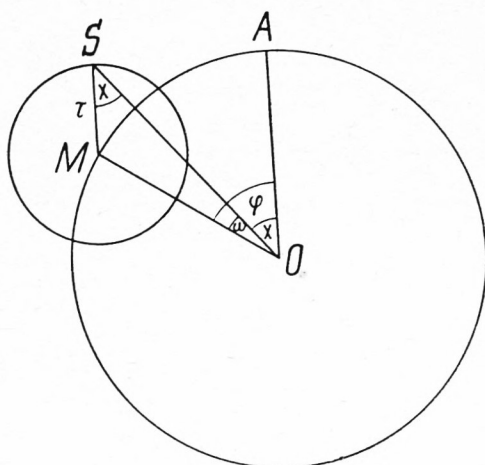
Fig. 1. Epizykel
