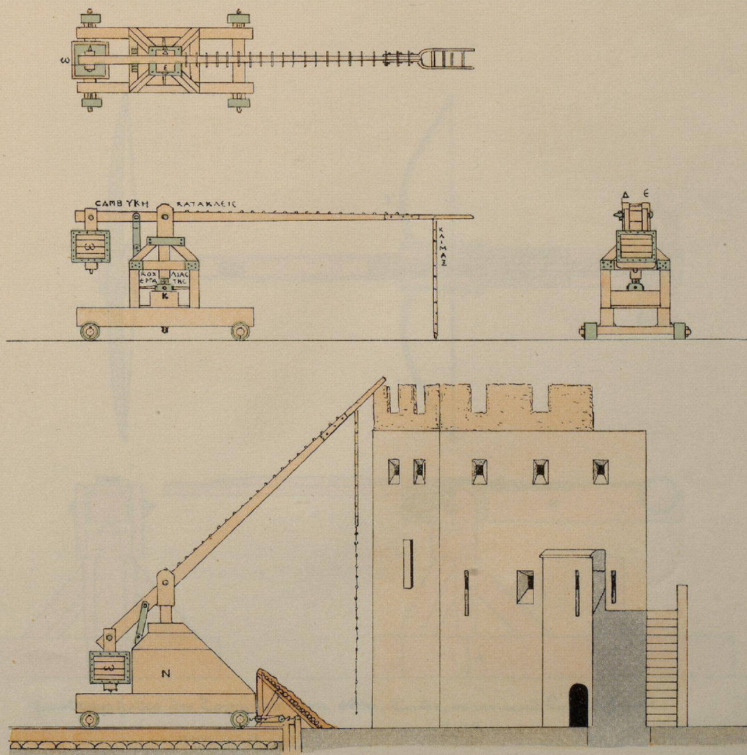
Belagerungsleiter 'CAMBYKH'
