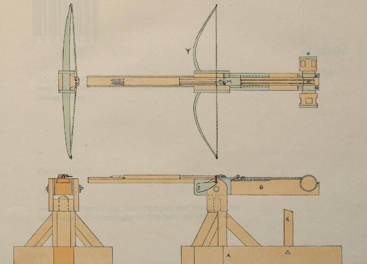
Gastraphetes des Zopyros von oben, links, vorn und Querschnitt
