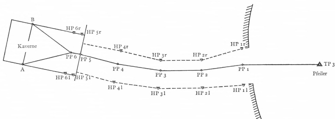
Figur 11. Anordnung der Polygonpunkte und Höhenfestpunkte im Zugangsstollen und in der Kaverne
