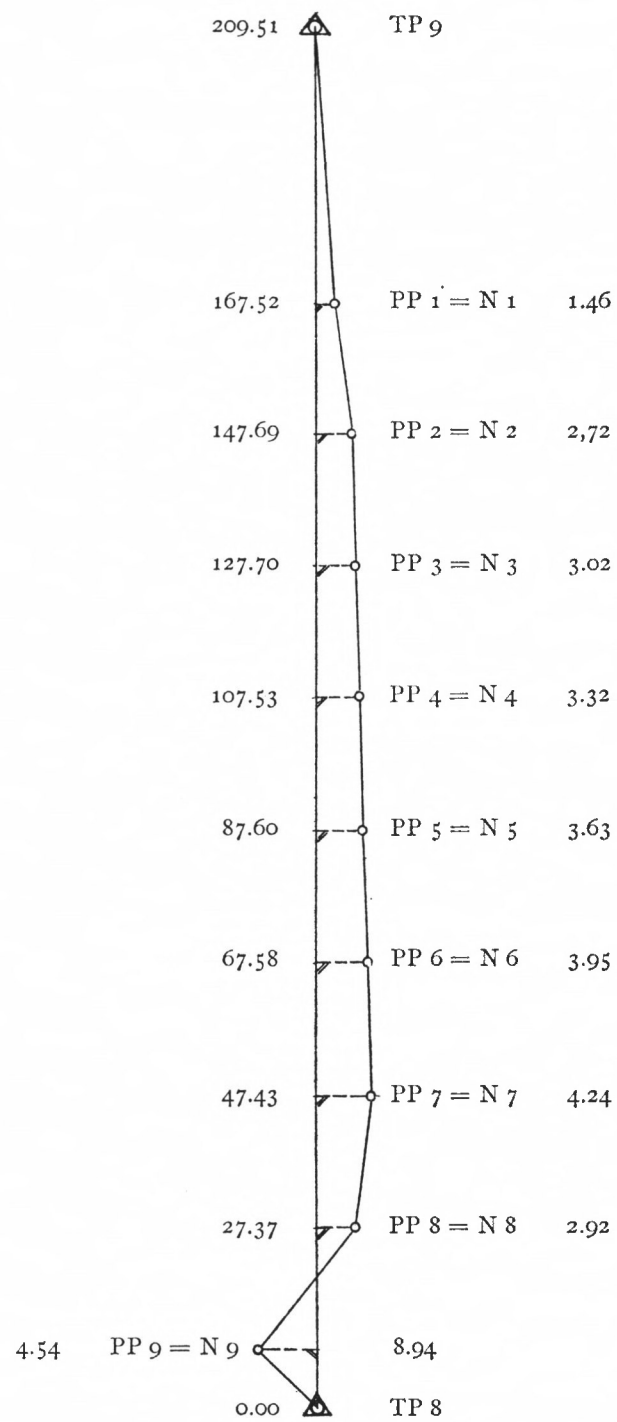
Figur 10. Skizze des Polygonzuges auf der Dammkrone
