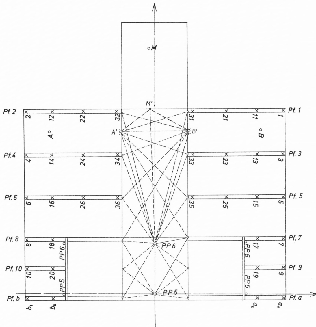
Figur 12. Anordnung der Zielmarken in der Kaverne
