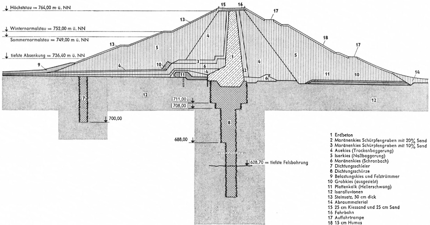
Figur 4. Querschnitt Staudamm in Dammitte
