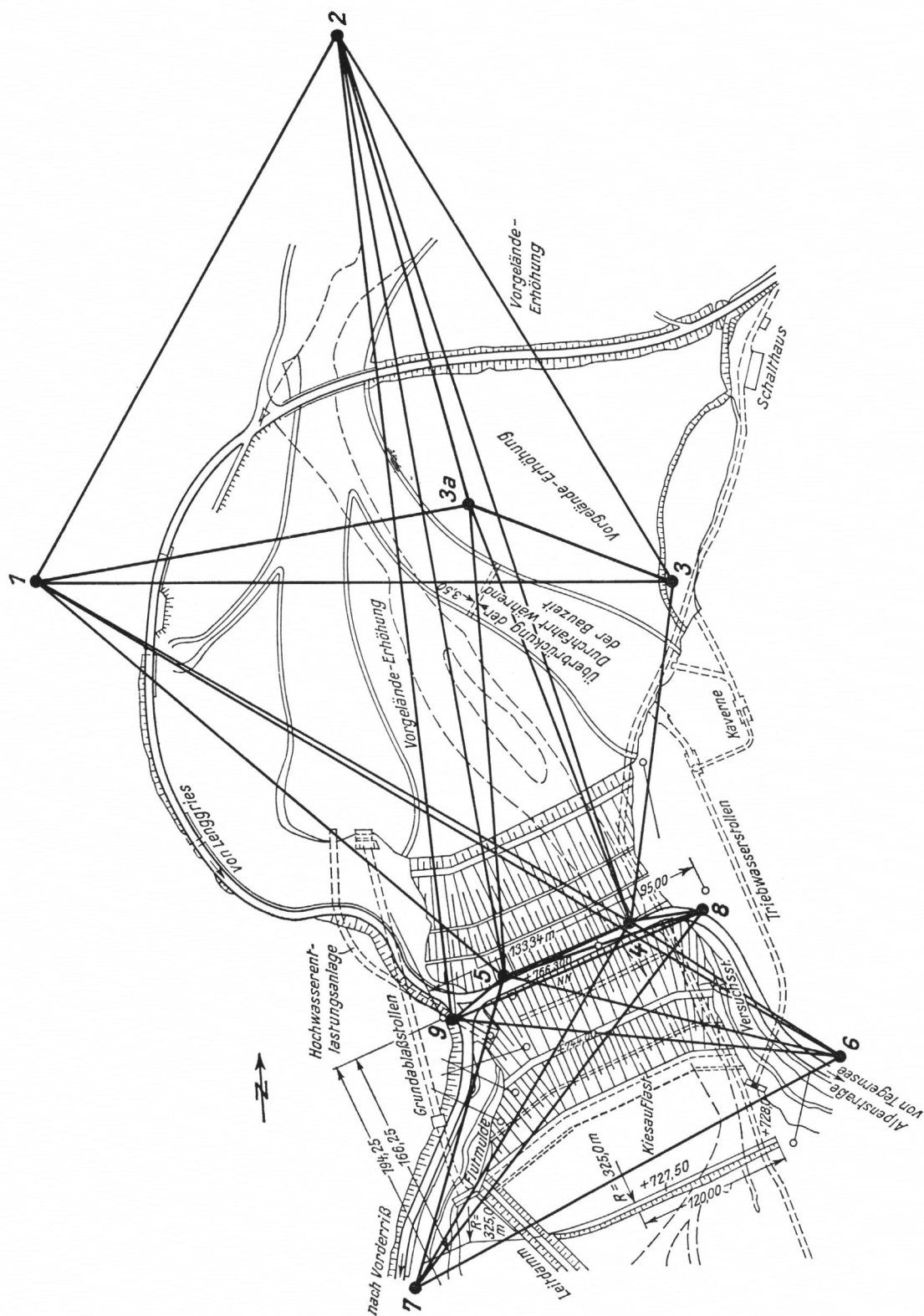
Figur 9b. Dreiecksnetz mit Lageskizze
