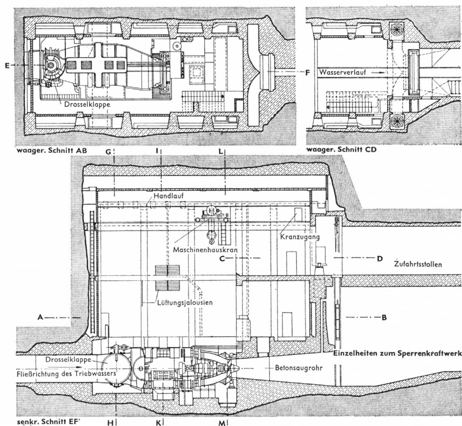
Figur 6a. Schnitte durch die Kaverne
