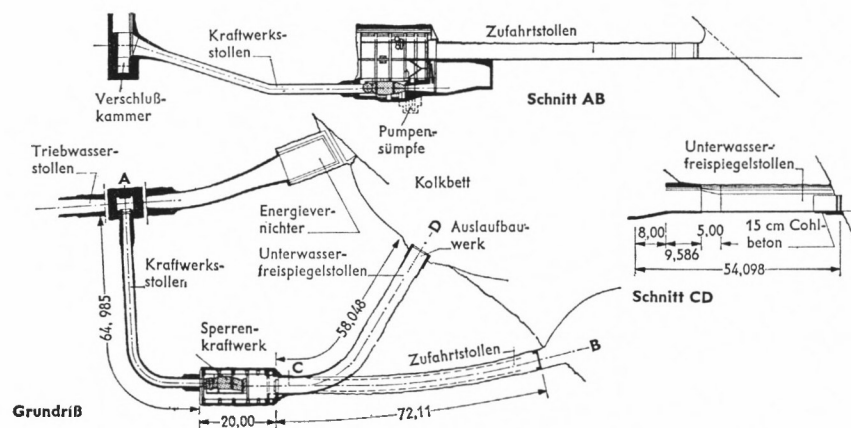
Figur 5. Gesamtübersicht Sperrenkraftwerk
