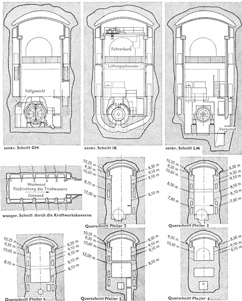
Figur 6b. Schnitte durch die Kaverne
