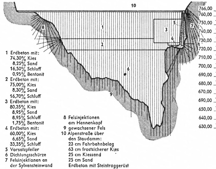
Figur 3. Längsschnitt Staudamm in Längsachse
