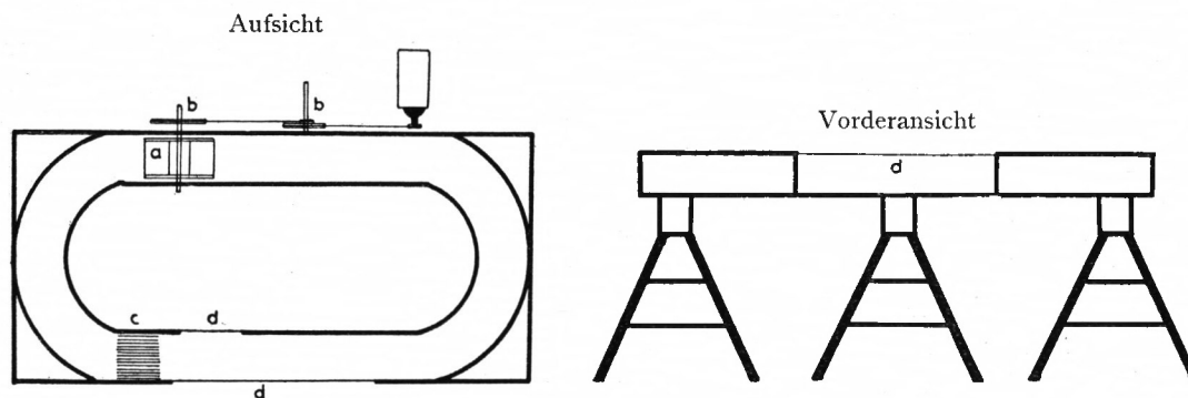
Abb. 1. Strömungsbecken (nähere Erklärung im Text). Zeichenerklärung: a Flügelrad; b Übersetzung; c Gleichrichter; d Glasscheiben.
