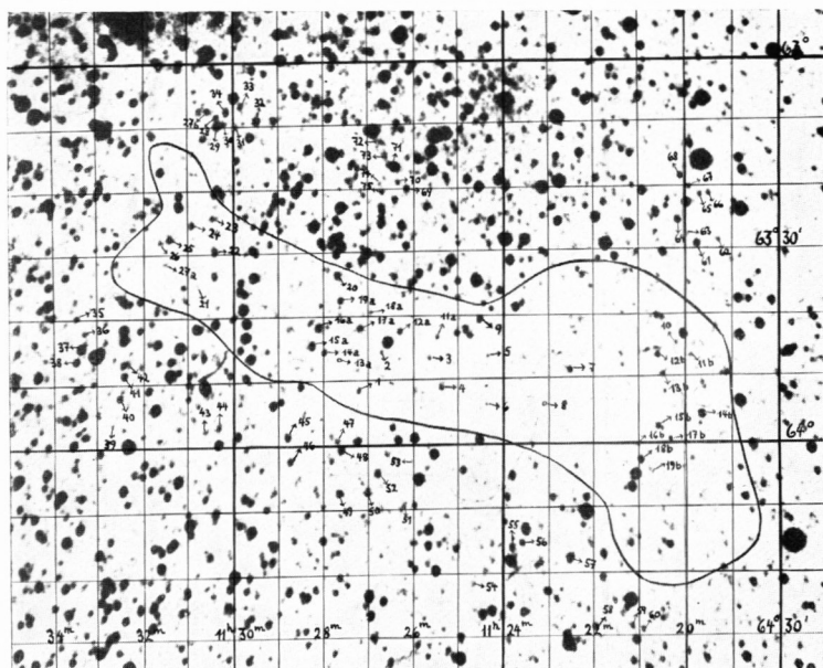
DW VI 11 \alpha_{1875} = 11^h 23,5^m \delta_{1875} = -63^\circ 48' Nr. 310 Vergr. 11×
