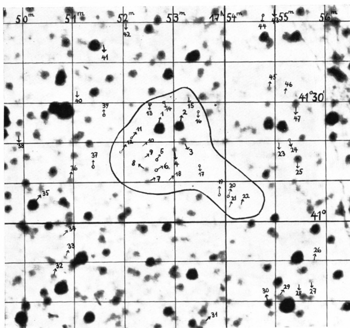
Nr. 327 DW IX 6 \alpha_{1875} = 17^h 53,5^m \delta_{1875} = -41^\circ 18' Vergr. 16×
