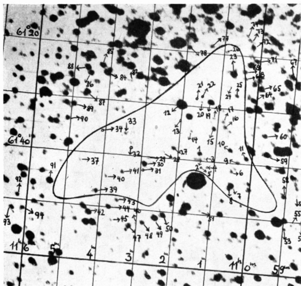
DW VI 8 \alpha_{1875} = 11^h 2,5^m \delta_{1875} = -61^\circ 38' Nr. 308 Vergr. 21×
