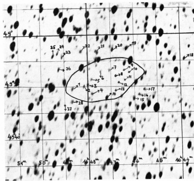
DW VIII 7 \alpha_{1875} = 16^h 47.2^m \delta_{1875} = -49^\circ 17'
