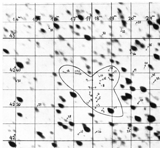
Nr. 328 DW IX 7 \alpha_{1875} = 17^h 18,1^m \delta_{1875} = -42^\circ 28' Vergr. 13×
