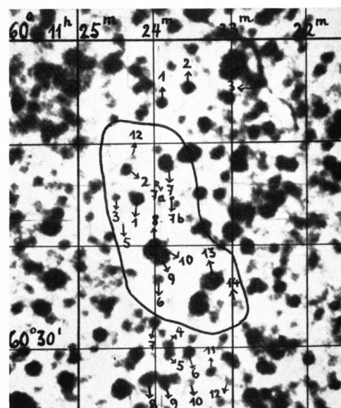
DW VI 7 \alpha_{1875} = 11^h 24^m \delta_{1875} = -60^\circ 16' Nr. 307 Vergr. 28 \times
