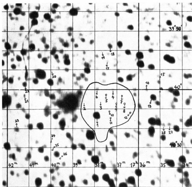
Nr. 325 DW IX 4 \alpha_{1875} = 17^h 37,3^m \delta_{1875} = -40^\circ 9' Vergr. 17×
