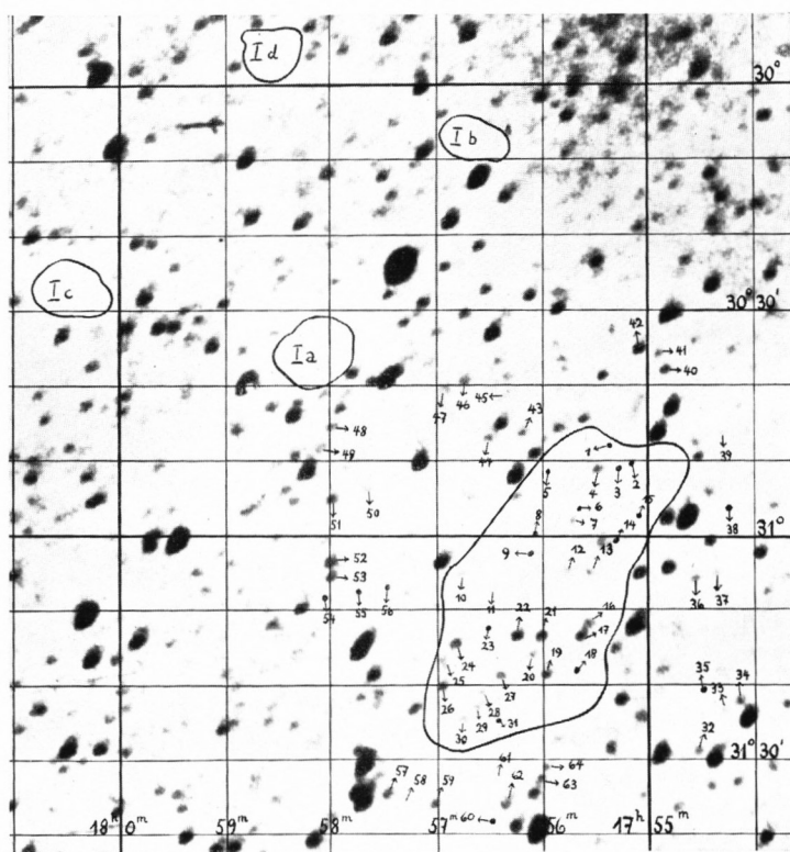
DW IX 1 \alpha_{1875} = 17^h 56^m \delta_{1875} = -31^\circ 9' Nr. 322 Vergr. 14 \times
