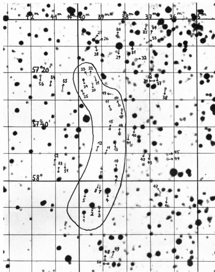
DW VII 3 \alpha_{1875} = 14^h 38,9^m \delta_{1875} = -57^\circ 45' Nr. 315 Vergr. 18×
