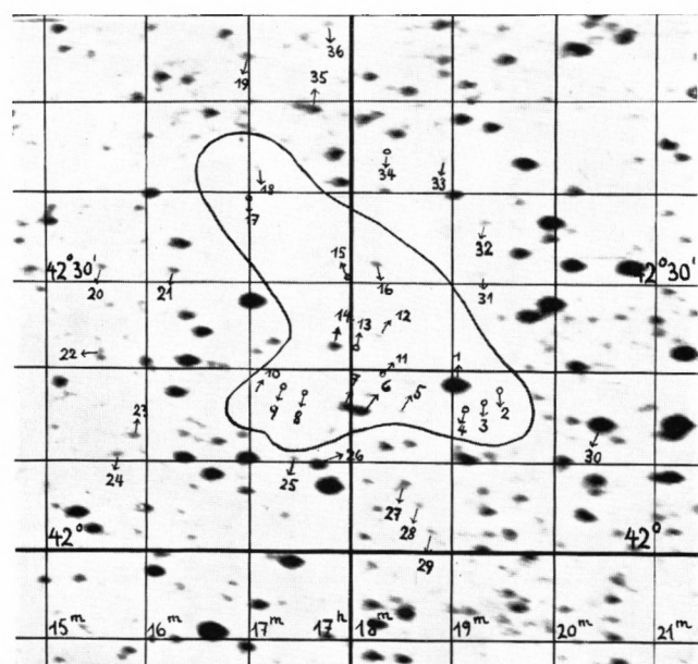
DW VIII 6 \alpha_{1875} = 17^h 18^m \delta_{1875} = -42^\circ 27'
