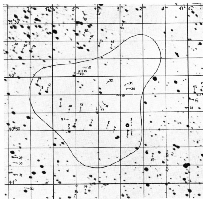
DW VIII 5 \alpha_{1875} = 17^h 4^m \delta_{1875} = -40^\circ 18'
