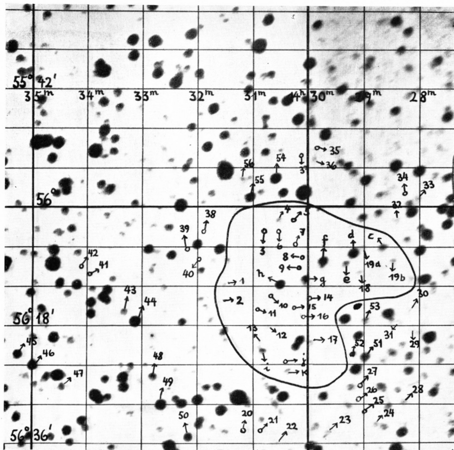
DW VII 2 \alpha_{1875} = 14^h 31^m \delta_{1875} = -56^\circ 13' Nr. 314 Vergr. 24 \times
