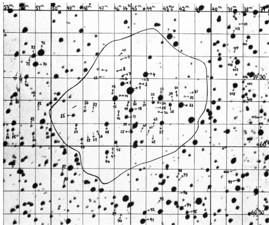
DW VII 1 \alpha_{1875} = 14^h 46^m \delta_{1875} = -59^\circ 42' Nr. 313 Vergr. 15 \times
