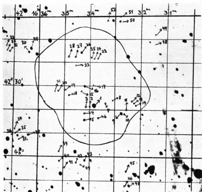
DW VIII 2 \alpha_{1875} = 16^h 34^m \delta_{1875} = -42^\circ 30'
