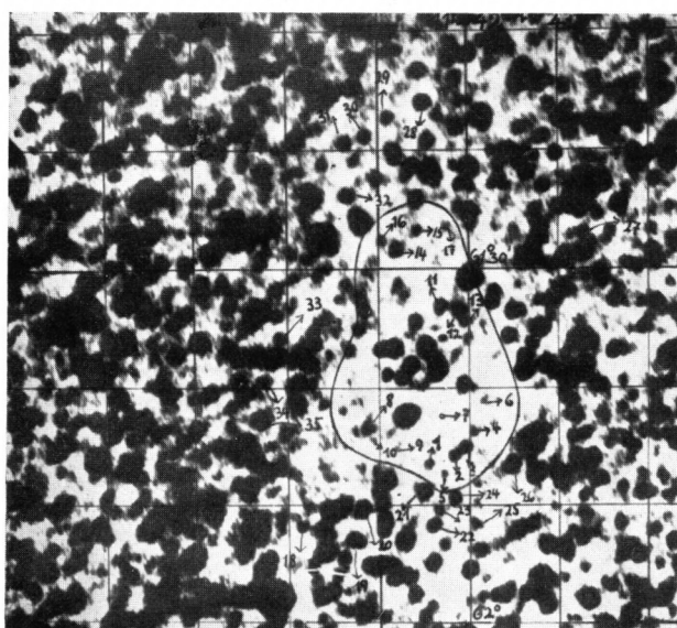
DW VI 6 \alpha_{1875} = 11^h 43,2^m \delta_{1875} = -61^\circ 40' Nr. 306 Vergr. 20 \times
