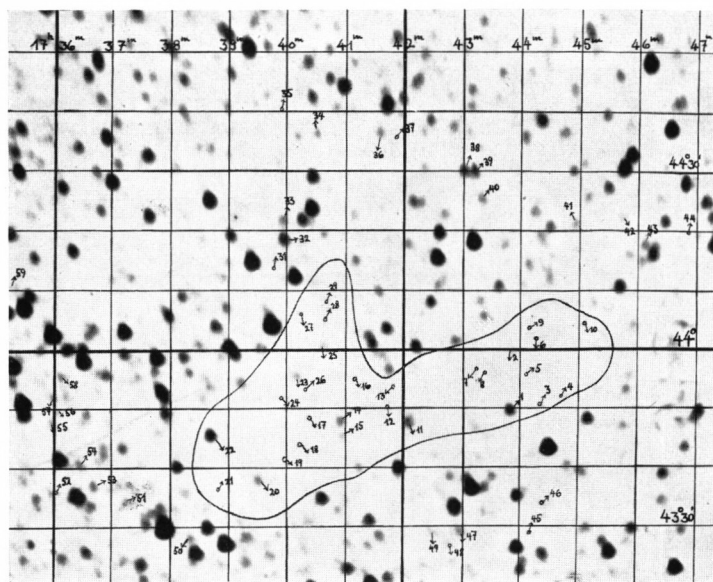
Nr. 326 DW IX 5 \alpha_{1875} = 17^h 41,8^m \delta_{1875} = -43^\circ 51' Vergr. 12×
