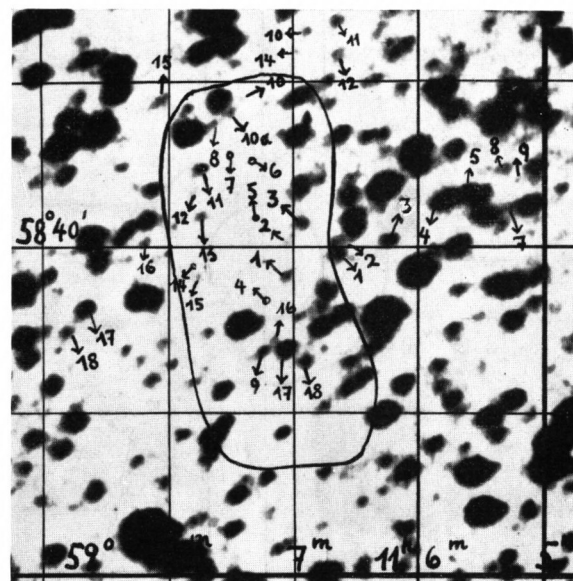
DW VI 5 \alpha_{1875} = 11^h 7,5^m \delta_{1875} = -58^\circ 41' Nr. 305 Vergr. 34 \times
