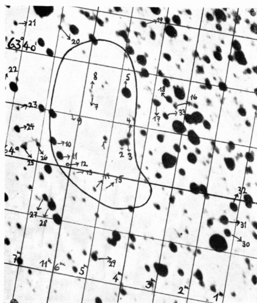
DW VI 10 \alpha_{1875} = 11^h 5,5^m \delta_{1875} = -63^\circ 50' Nr. 309 Vergr. 22×
