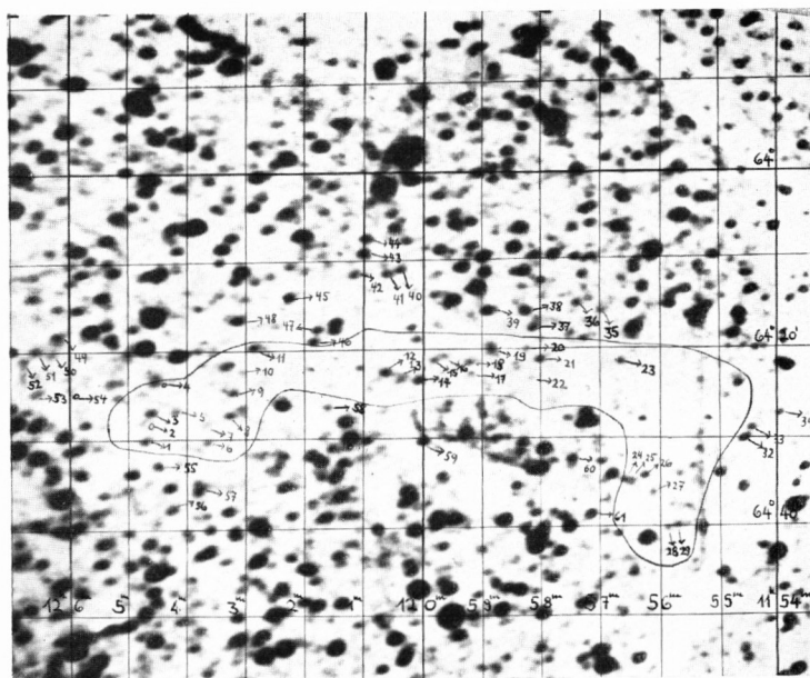
DW VI 12 \alpha_{1875} = 11^h 59^m \delta_{1875} = -64^\circ 22' Nr. 311 Vergr. 17×
