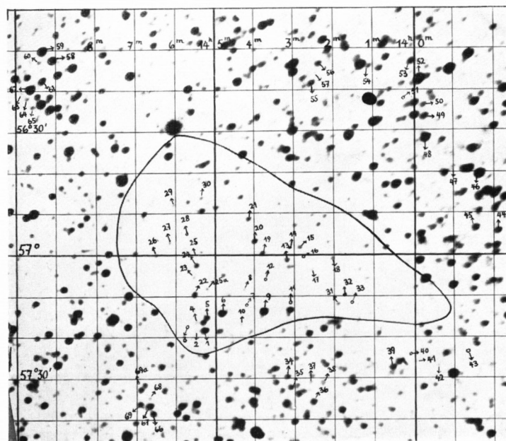
DW VII 3 \alpha_{1875} = 14^h 4^m \delta_{1875} = -56^\circ 57' Nr. 316 Vergr. 12×
