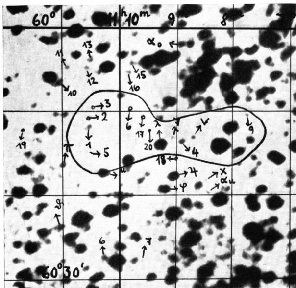
DW VI 4 \alpha_{1875} = 11^h 09^m \delta_{1875} = -60^\circ 14' Nr. 304 Vergr. 33 \times
