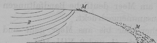
Figur 19. B Bänderung. M Moräne.
