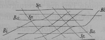
Figur 17. Ba alte Bänder. Bi junge Bänder. Sp Spaltbänder.
