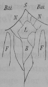
Figur 26. B Bach. F Fels. L Lagune. N Nehrung (Haken).
