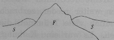
Figur 18. Schmelzkehlen zwischen Felsspitzen F und Schnee S.
