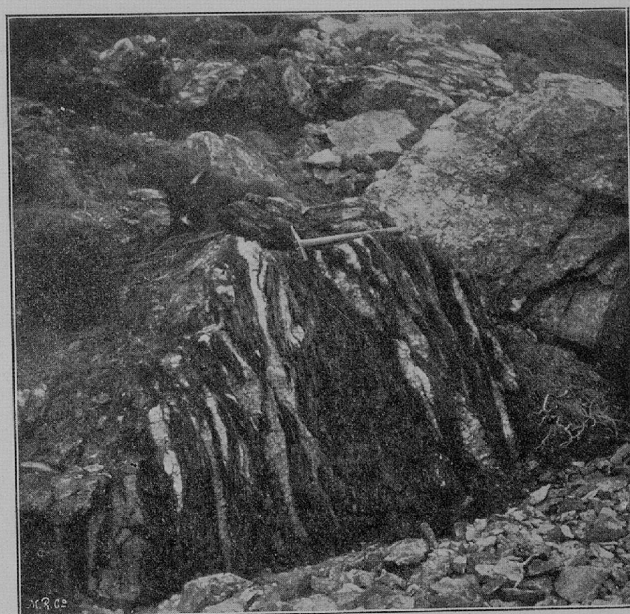
Ebene Schichten mit Quarzlinsen.
