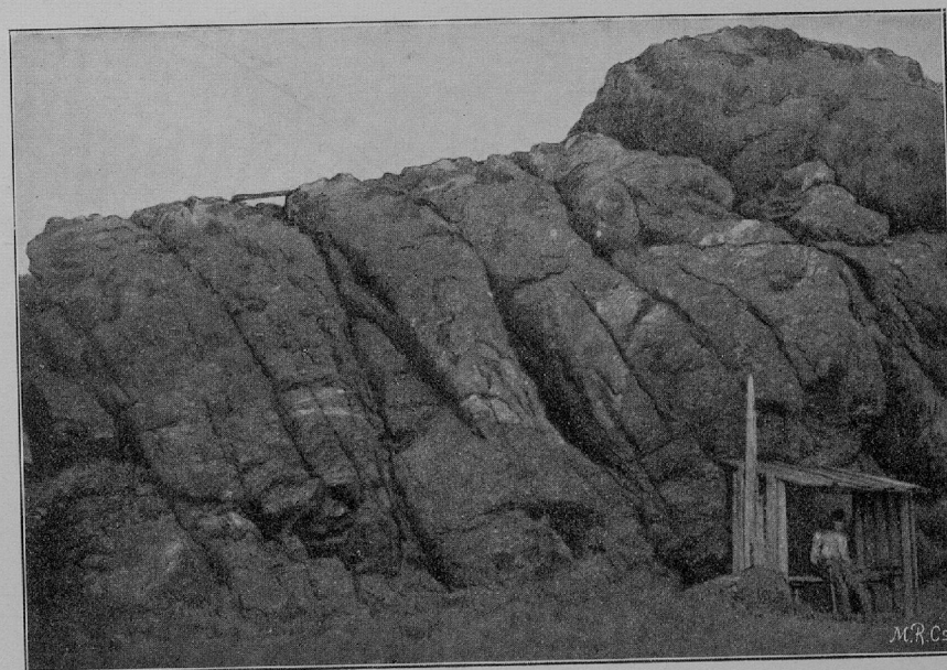
Querspalten am Silberberggipfel.
