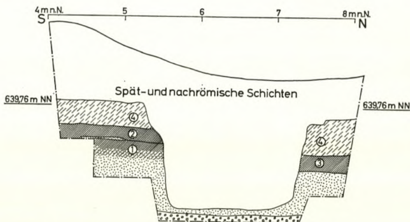
Abb. 12. Westprofil des Schnittes u2. 1 gewachsener Sandboden mit alter Oberfläche. 2.3 frühromische Kulturschicht außerhalb (2) und innerhalb (3) der Grube G9. 4 helle Lehmschicht. M. 1:50.
