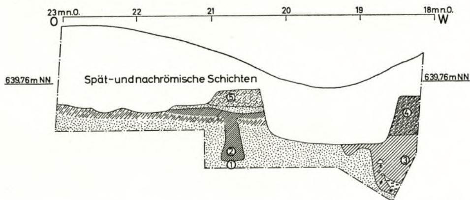
Abb. 14. Südprofil des Schnittes oo. 1 gewachsener Sandboden, alte Oberfläche abgegraben. 2 Gräbchen g 26. 3 Grube unter der spätrömischen Mauer. 4 starke früh-römische Kulturschicht über Grubeneinfüllung. 5 oberste früh-römische Kulturschicht. M. 1:50.
