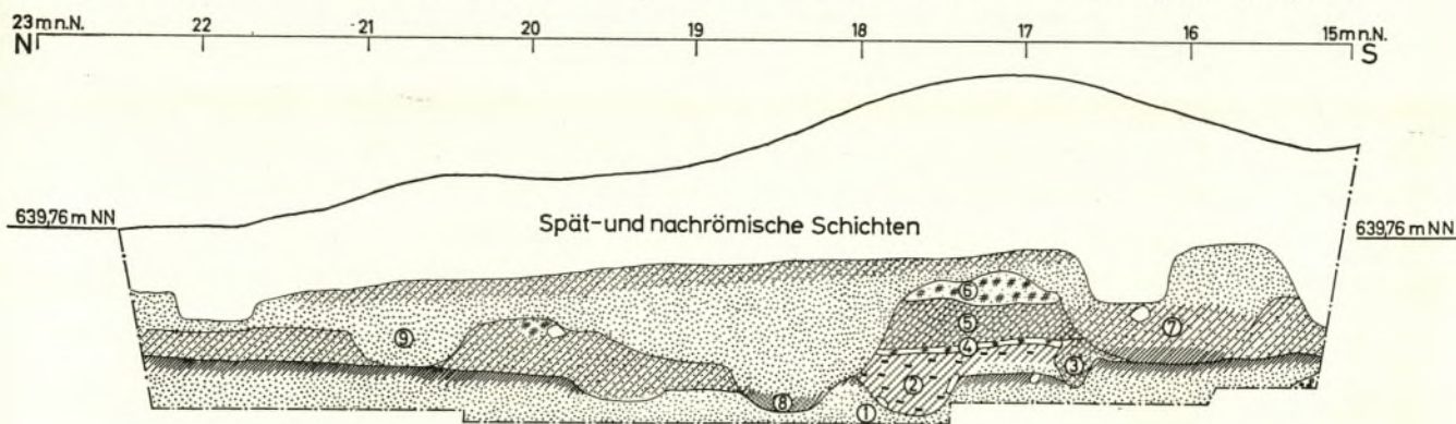
Abb. 4. Ostprofil der Fläche F 7. 1 gewachsener Boden. 2 Grube G 5 (Aschenschicht). 3 Gräbchen g 8. 4 untere Lehmbrandschicht. 5 Kulturschicht zwischen unterer und oberer Lehmbrandschicht. 6 obere Lehmbrandpackung. 7 Gräbchen g 7. 8 „Grube“ G 6. 9 Gräbchen g 10. M. 1:50.
