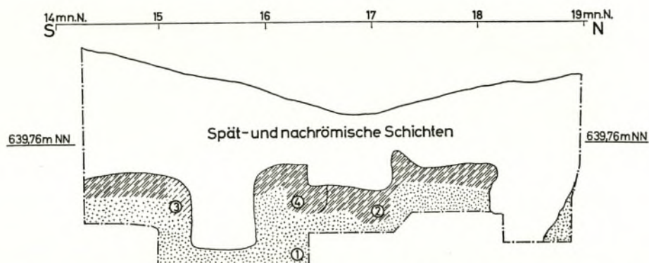
Abb. 15. Westprofil des Schnittes dd. 1 gewachsener Sandboden, alte Oberfläche abgegraben. 2 Gräbchen g 25. 3 Gräbchen g 22. 4 Gräbchen g 24. M. 1:50.
