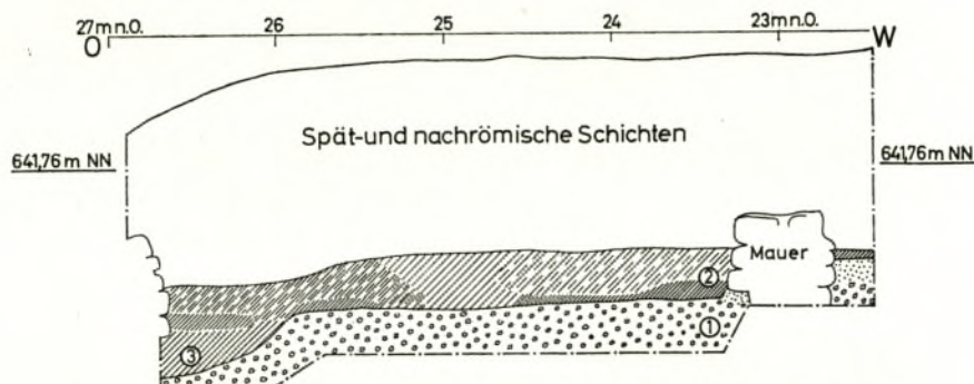
Abb. 7. Südprofil der Fläche K 1 bei 7,50 m n. N. 1 gewachsener Boden. 2 schräg angeschnittenes Gräbchen g 12. 3 Grube G 7. M. 1:50.
