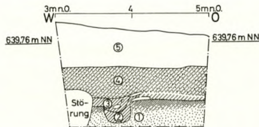
Abb. 5. Nordprofil der Fläche F7. 1 gewachsener Boden. 2 u. 3 Gräben g6. 4 frührömische Auffüllschicht. 5 spät- und nachrömische Schichten. M. 1:50.
