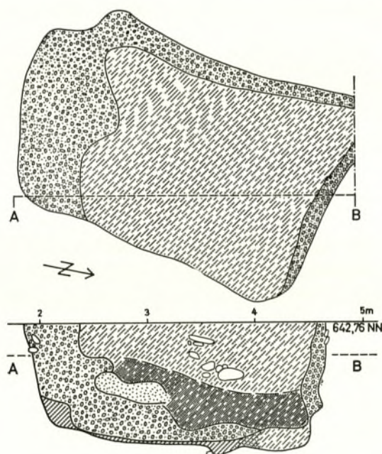
Abb. 22. Schnitte VII und VIIa. Frühromische Kastengrube mit zwei verschiedenen Bauperioden. M. 1:50.
