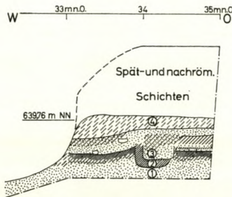
Abb. 10. Nordprofil des Schnittes u4. 1 gewachsener Sandboden mit alter Oberfläche. 2/3 Gräbchen g16/17. 4 frührömische Kulturschicht. M. 1:50.
