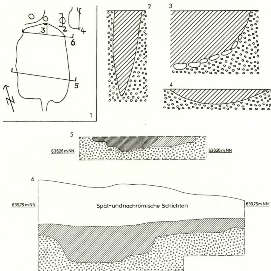
Abb. 21. Schnitt qu. 1 Gruben G 20–G 22 mit Lage der Profile 2–6. 2 Schnitt durch das Pfostenloch an der Nord-Ost-Ecke von G 20. 3 Teilprofil im nördlichen Abschnitt von Grube G 20. 4 Längsschnitt durch Grube G 22. 5.6 Querschnitte durch die Grube G 20. 1 M. 1:100; 2–4 M. 1:20; 5.6 M. 1:50.
