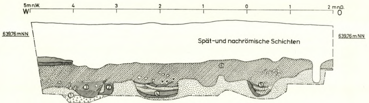
Abb. 1. Nordprofil der Fläche F1. 1 gewachsener Sand- oder Kiesboden. 2 Gräbchen g2. 3 Gräbchen g1. 4 grubenartige Vertiefung. 5 nördliche Erweiterung von Grube G2. 6 homogene frühromische Kulturschicht. M. 1:50.
