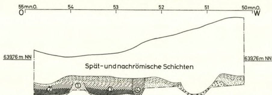
Abb. 17. Südprofil des Schnittes y. 1 gewachsener Boden. 2 Grube G 17. 3 Grube G 18. 4 Gräbchen g 41. M. 1:50.
