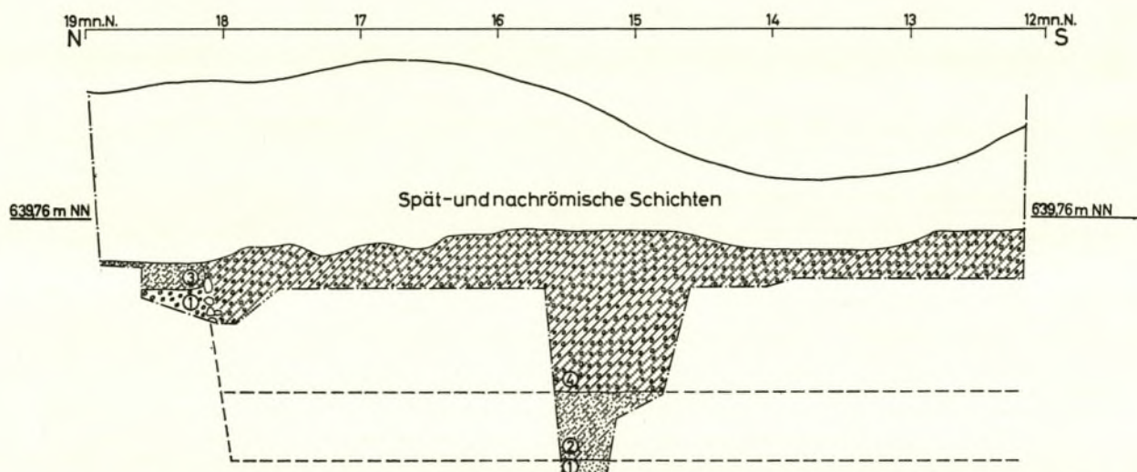
Abb. 19. Ostprofil des Schnittes ee. 1 gewachsener Boden. 2 frühromische Kulturschicht im „Schacht“. 3 frühromische Kulturschicht außerhalb des „Schachtes“. 4 kiesige Auffüllschicht. M. 1:50.
