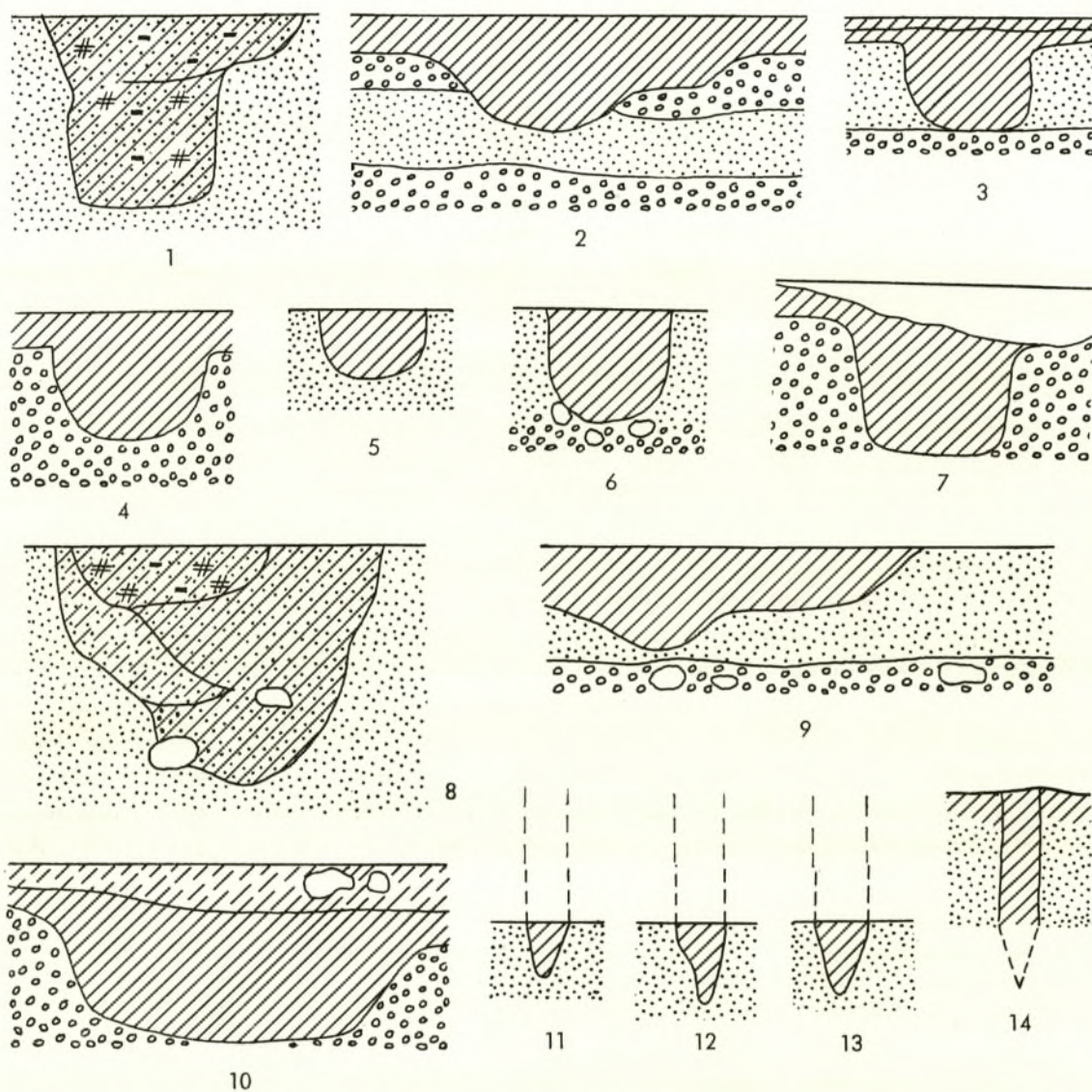
Abb. 2. Profile von Gruben, Gräbchen und Pfostenlöchern. Gräbchen 1: g2; 2: g5; 3: g14; 4: g29; 5: g44; 6: g49; 7: g28. Gruben 8: G2; 9: G4; 10: G14. Pfostenlöcher 11-14: Schnitt uu in Gräbchen g15. M. 1:20.
