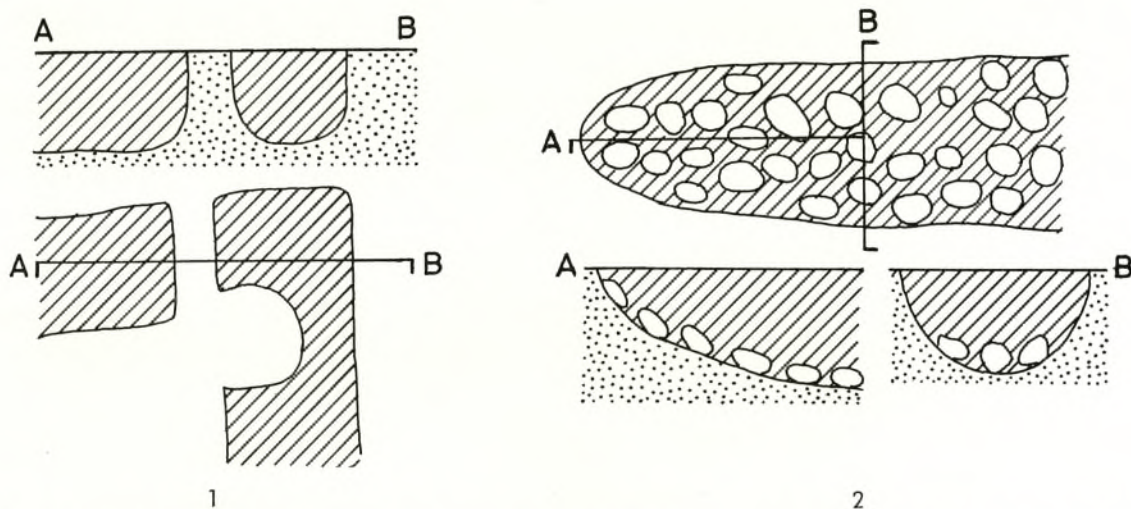
Abb. 18. Schnitt p, Mittelteil. 1 Schnitt durch die Gräbchen g45 und g48. 2 Quer- und Längsschnitt durch Gräbchen g47 M. 1:20.
