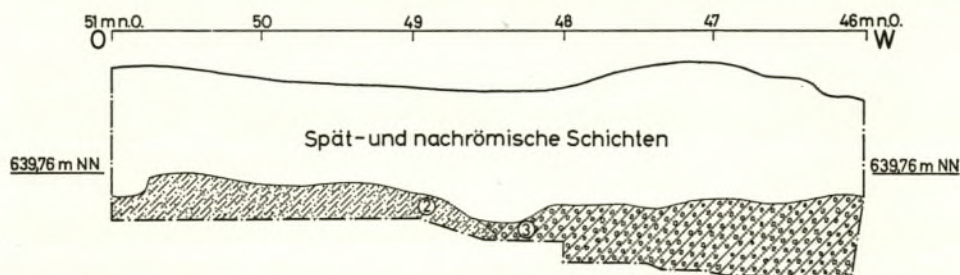
Abb. 20. Südprofil des Schnittes nn/ee. 2 frühromische Kulturschicht außerhalb des „Schachtes“ (vgl. Abb. 19, 3). 3 kiesige Auffüllschicht (vgl. Abb. 19, 4). M. 1:50.
