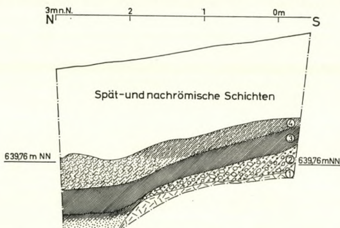
Abb. 8. Ostprofil des Schnittes ww. 1 gewachsene Flinzrippe, die bei 2 m n. N. stark abfällt. 2 gewachsener Kies- bzw. Sandboden. 3 stark verschlickte frühromische Schicht. 4 helle, trockene frühromische Sandschicht. M. 1:50.
