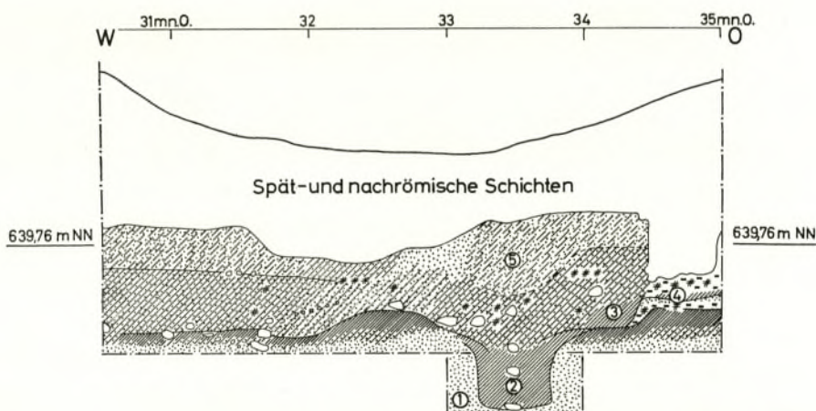
Abb. 9. Nordprofil von Schnitt uu bei 2,50 m n. N. 1 gewachsener Sandboden mit alter Oberfläche. 2 Grube G8. 3 Gräbchen g16/17. 4 mehrere dünne Kulturschichten östl. von g16/17. 5 stark durchwühlte frühromische Kulturschicht. M. 1:50.
