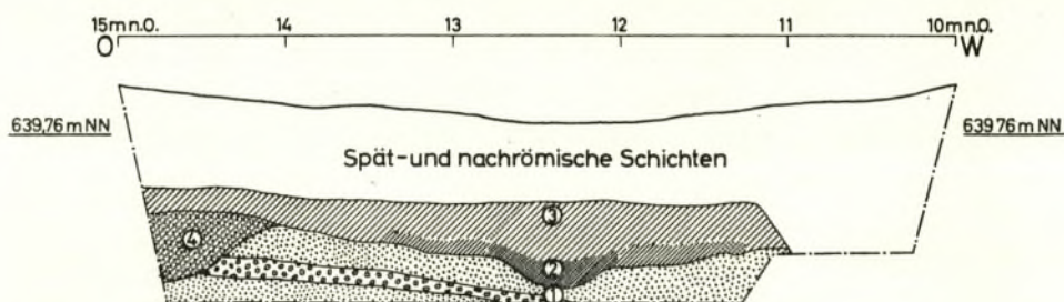
Abb. 3. Südprofil der Fläche F4. 1 gewachsener Boden. 2 Gräbchen g5. 3 muldenförmige Vertiefung G3. 4 Grube mit reinem Flußsand (nur im Profil beobachtet). M. 1:50.
