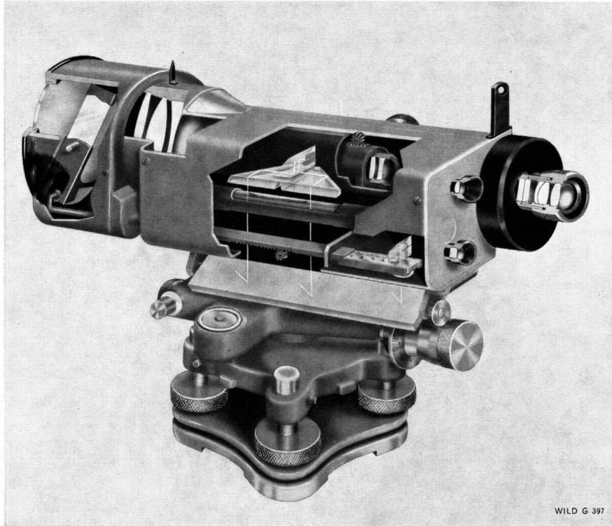
Fig. 1 Wild N3-Präzisionsnivellier im Schnitt
