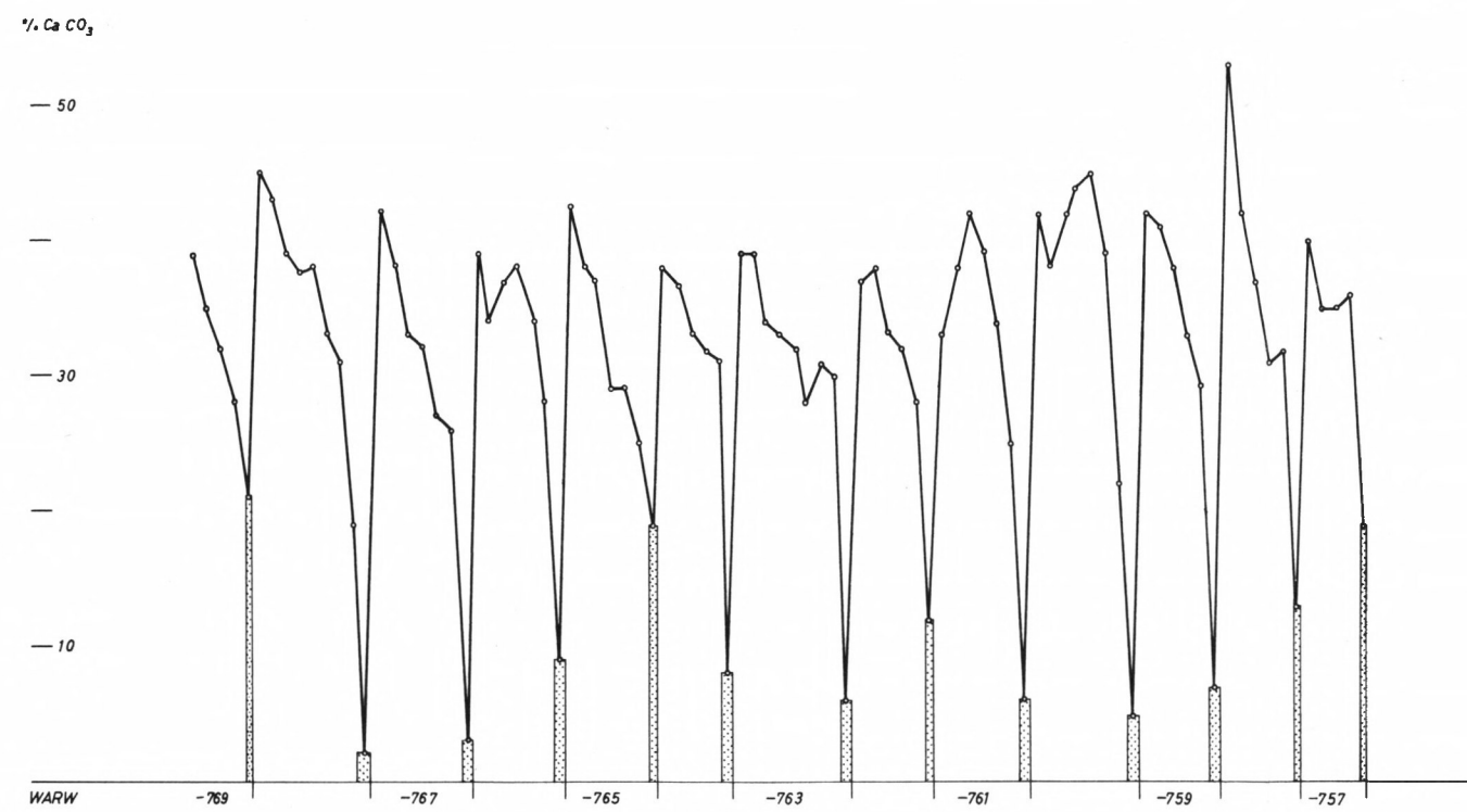
a. \text{Ca CO}_3 -ANTEIL DER WARWEN -769 BIS -757 UPPSALA-REGION NACH ARRHENIUS
