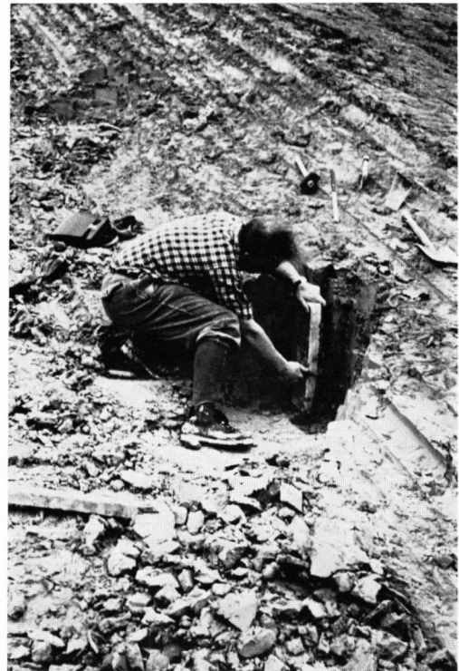
Abb. 2 Herausschneiden eines Entnahmekastens
