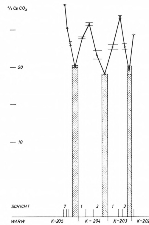
b. \text{Ca CO}_3 -ANTEIL DER WARWEN K-205 BIS K-202 ROSENHEIMER BECKEN WARWENMÄCHTIGKEIT 5-FACH VERGRÖßERT
