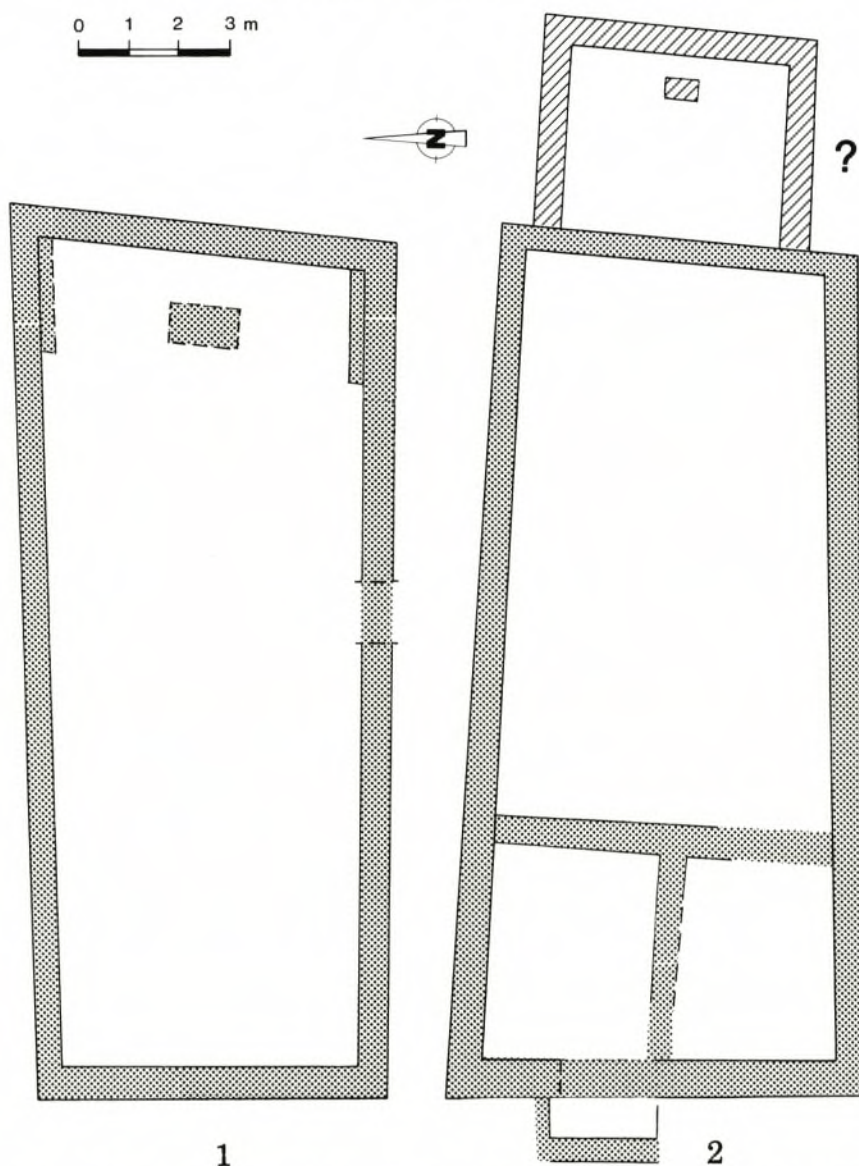
Abb. 20. 1 frühmittelalterliche Kirche auf dem Colle di Zuca, Periode 1; 2 S. Maria Maddalena auf dem Colle Santino, Bau I, Periode 1. M. 1:150.
