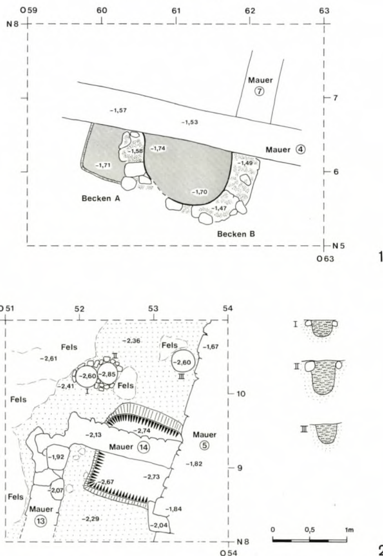
Abb. 10. Römischer Gebäudekomplex A (Periode I): 1 gemörtelte Becken an Mauer 4; 2 Grube mit Pfostenlöchern westlich des Zisternenraumes D. M. 1 : 50.
