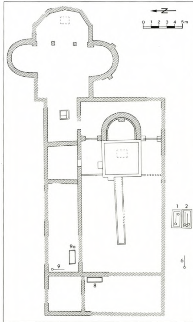
Abb. 61. Invillino: Grundriß der spätantiken Kirchenanlage auf dem Colle di Zuca. M. 1 : 300.
