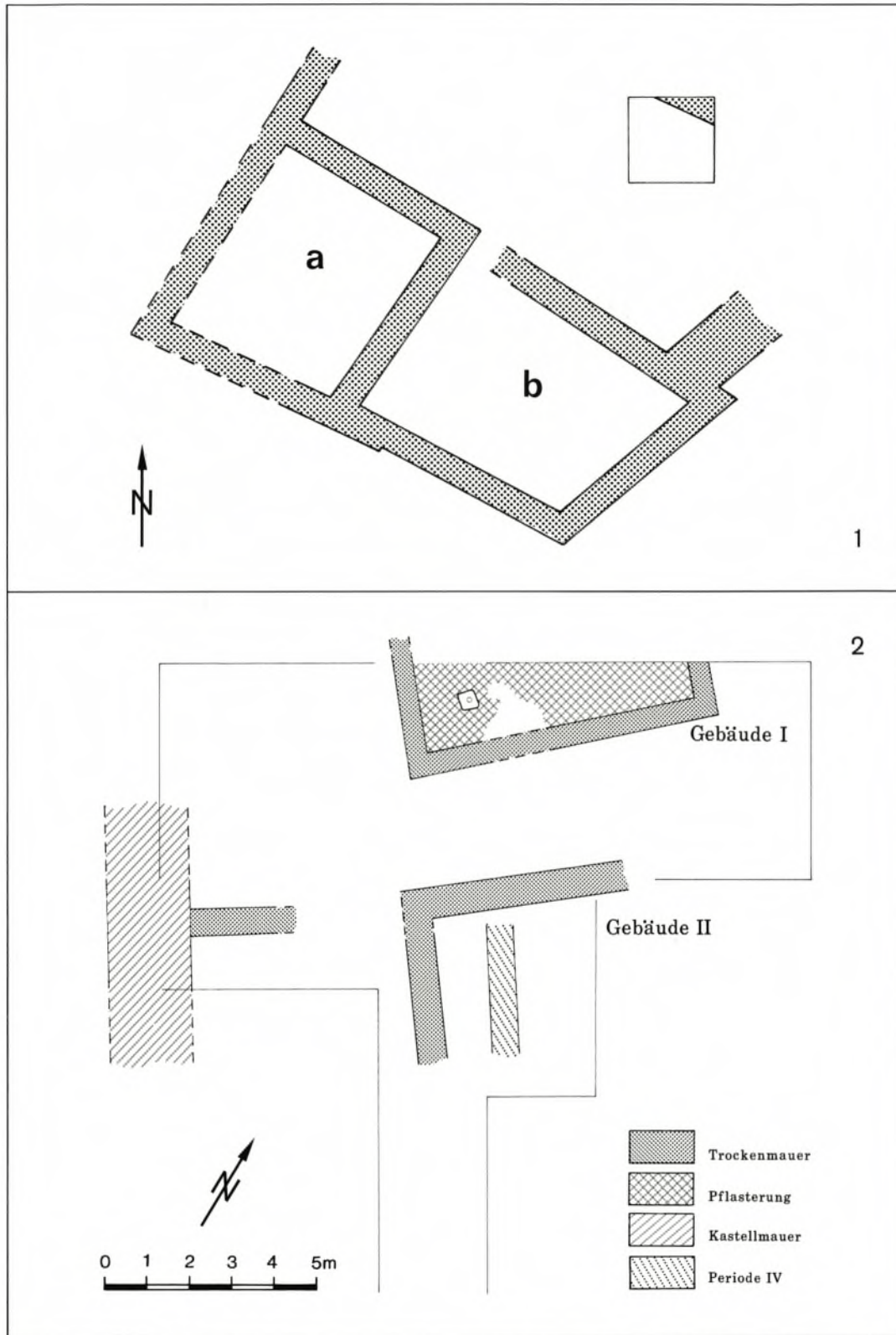
Abb. 55. Holzbauten auf Trockenmauersockeln in Castelseprio (Prov. Varese): 1 italienische Ausgrabung; 2 polnische Ausgrabung (nach Anm. 10). M. 1: 150.
