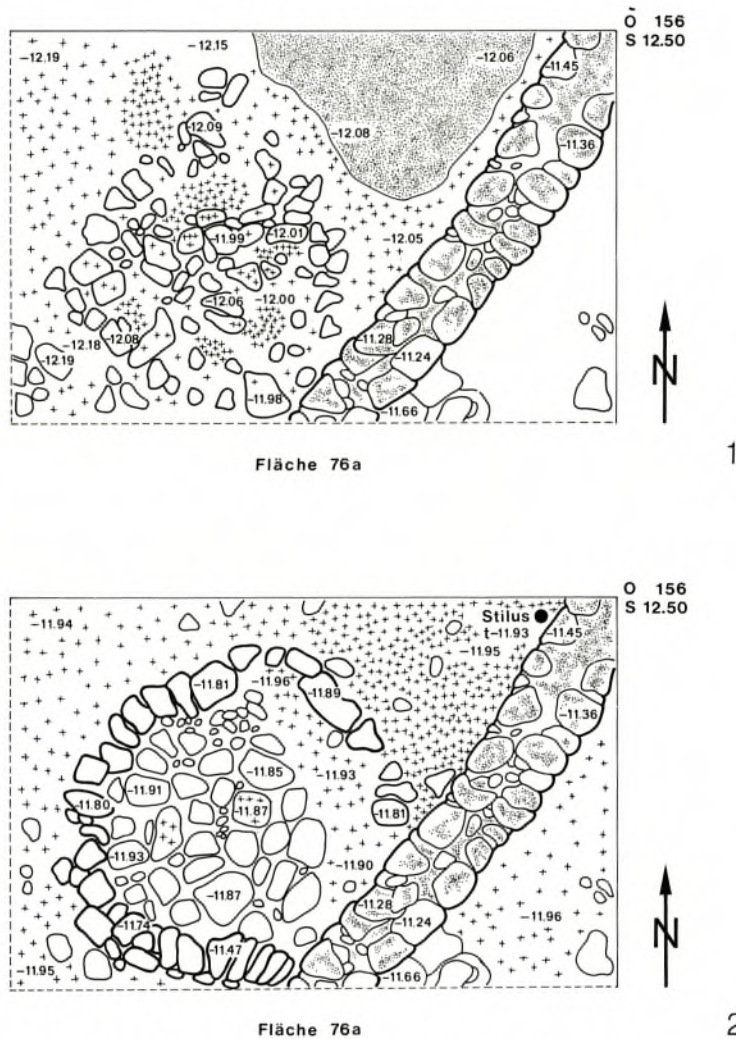
Abb. 16. Älterer (1) und jüngerer (2) ,Ofen' in der großen, runden Zisterne (Beilage 10) mit Holzkohle und Ascheresten (Periode III). M. 1:50.
