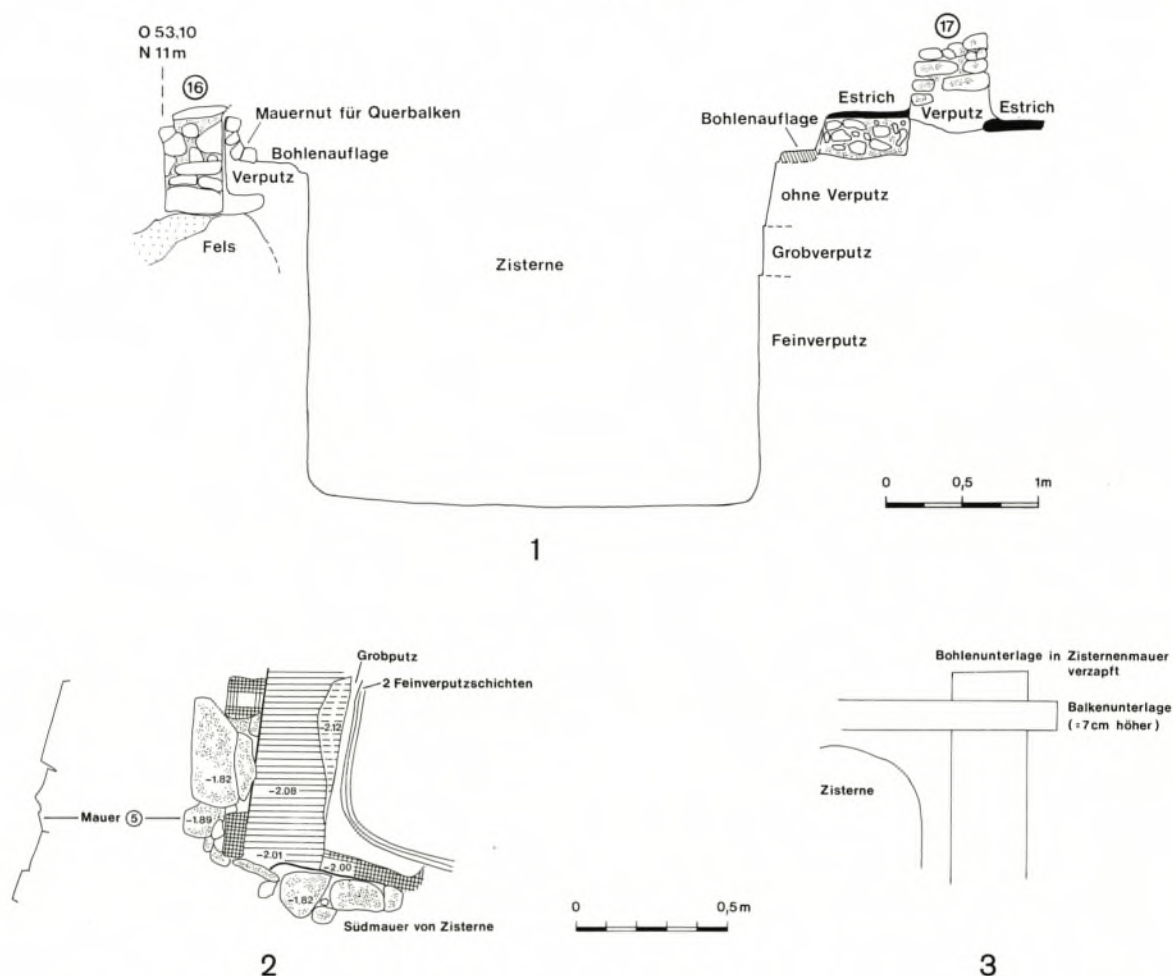
Abb. 11. Römischer Gebäudekomplex A, Zisterne: 1 Querschnitt; 2 Verputzschichten in der Südwestecke; 3 hölzerne Abdeckung. 1 M. 1:50; 2–3 M. 1:25.
