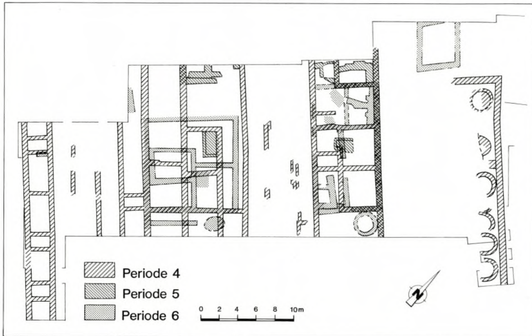
Abb. 56. Carnuntum (Niederösterreich), Nordostbereich des Legionslagers: Periode 4 = vorvalentinianisch, Periode 5 = valentinianisch, Periode 6 = nachvalentinianische Zivilbauten aus Holz auf Trockenmauersockeln (nach Anm. 22). M. 1 : 400.
