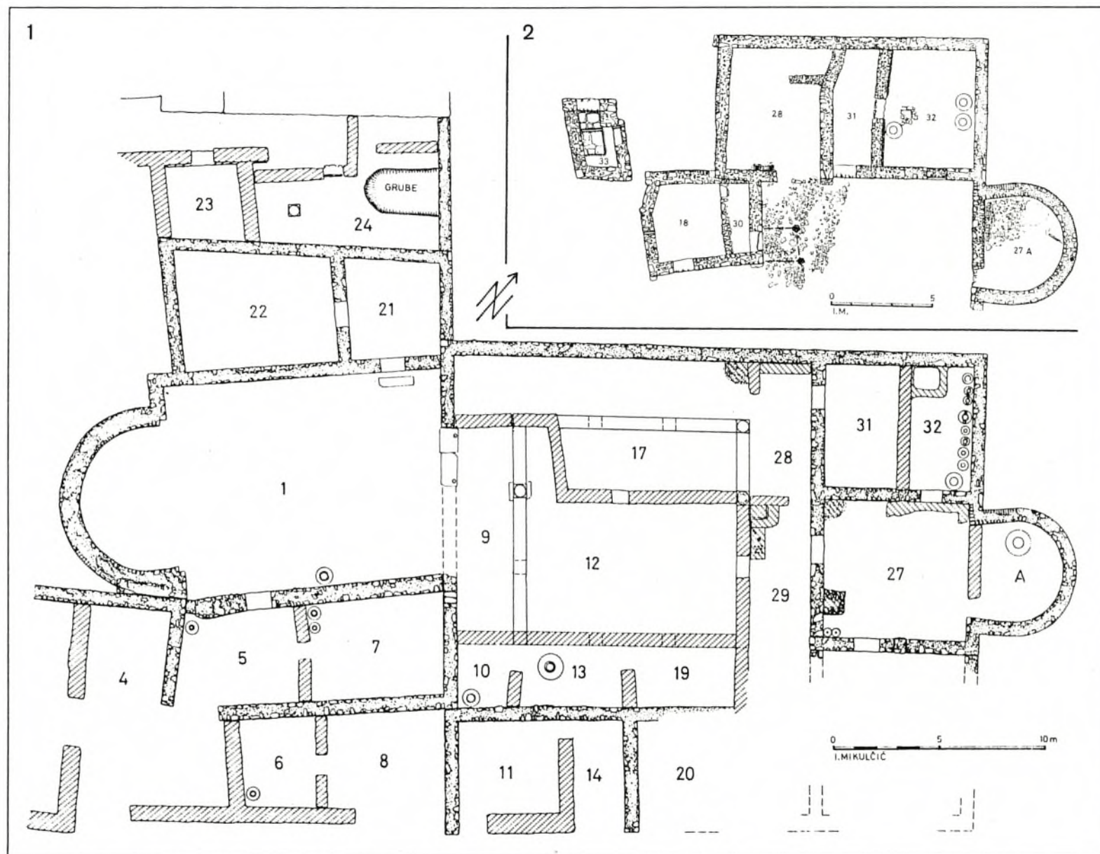
Abb. 57. Stobi (Makedonien), Domus fullonica: 1 Umbauphase vom Ende des 4. bis zur Mitte des 5. Jahrhunderts; 2 Wohnobjekt über dem Nordostflügel des zerstörten Palastes aus dem späten 5. und 6. Jahrhundert (nach Anm. 30). M. 1:250.
