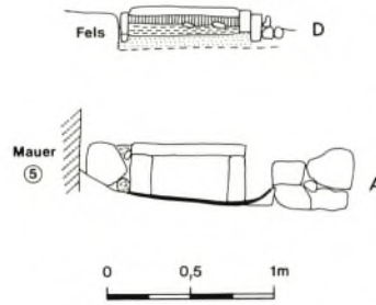
Abb. 12. Römischer Gebäudekomplex A: Querschnitte durch die Herdstellen A und D (Periode I). M. 1:50.
