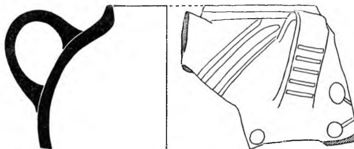
Abb. 1. Bruchstück von Wandung und Rand des Ausgußgefäßes K 7. [1:2]
