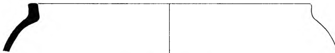
Abb. 11. Krater G 112 bis. [1:2]
