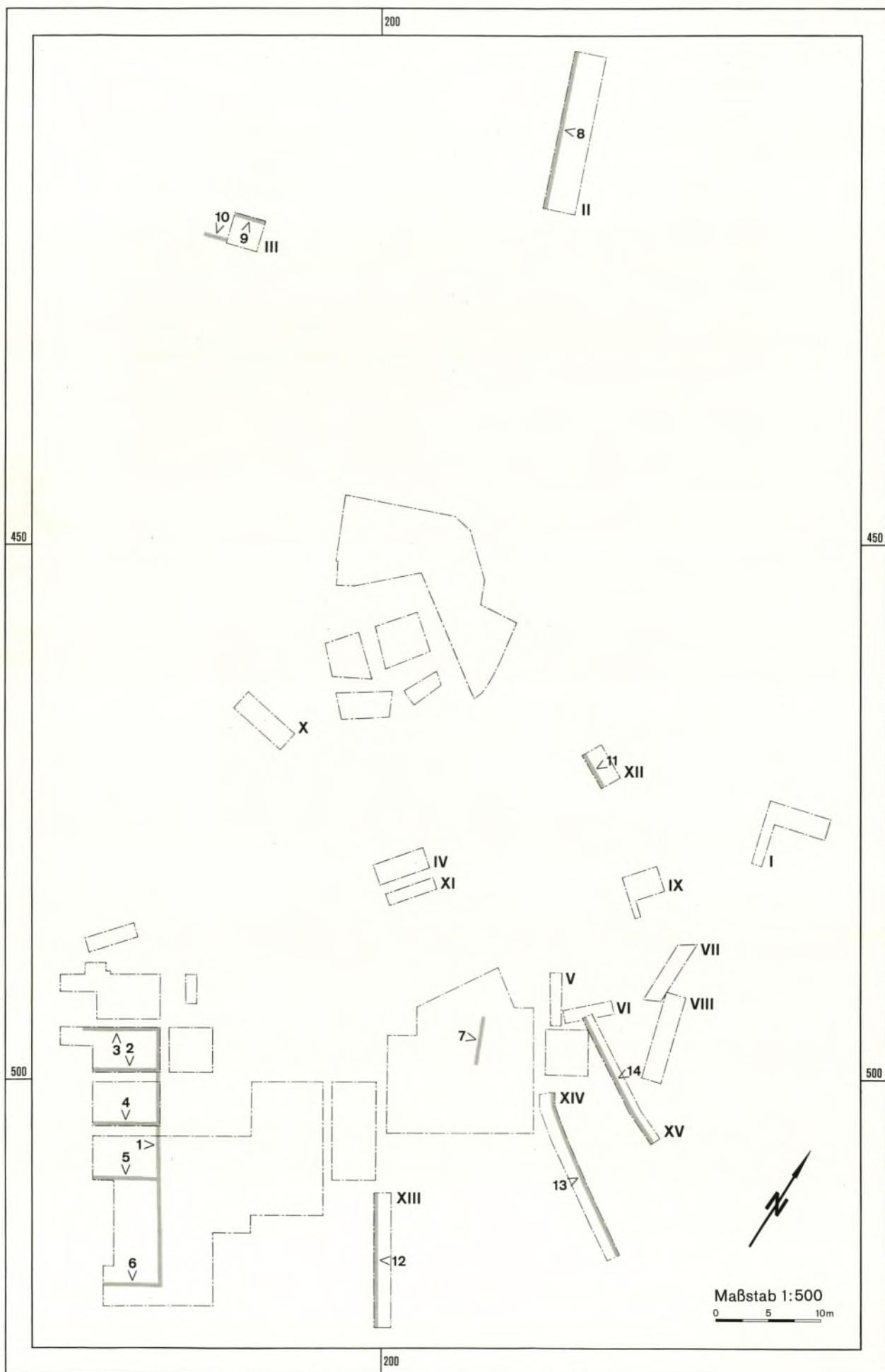
Abb. 31. Burg Sponeck. – Lageplan der Suchschnitte und Profile. M. 1:500.
