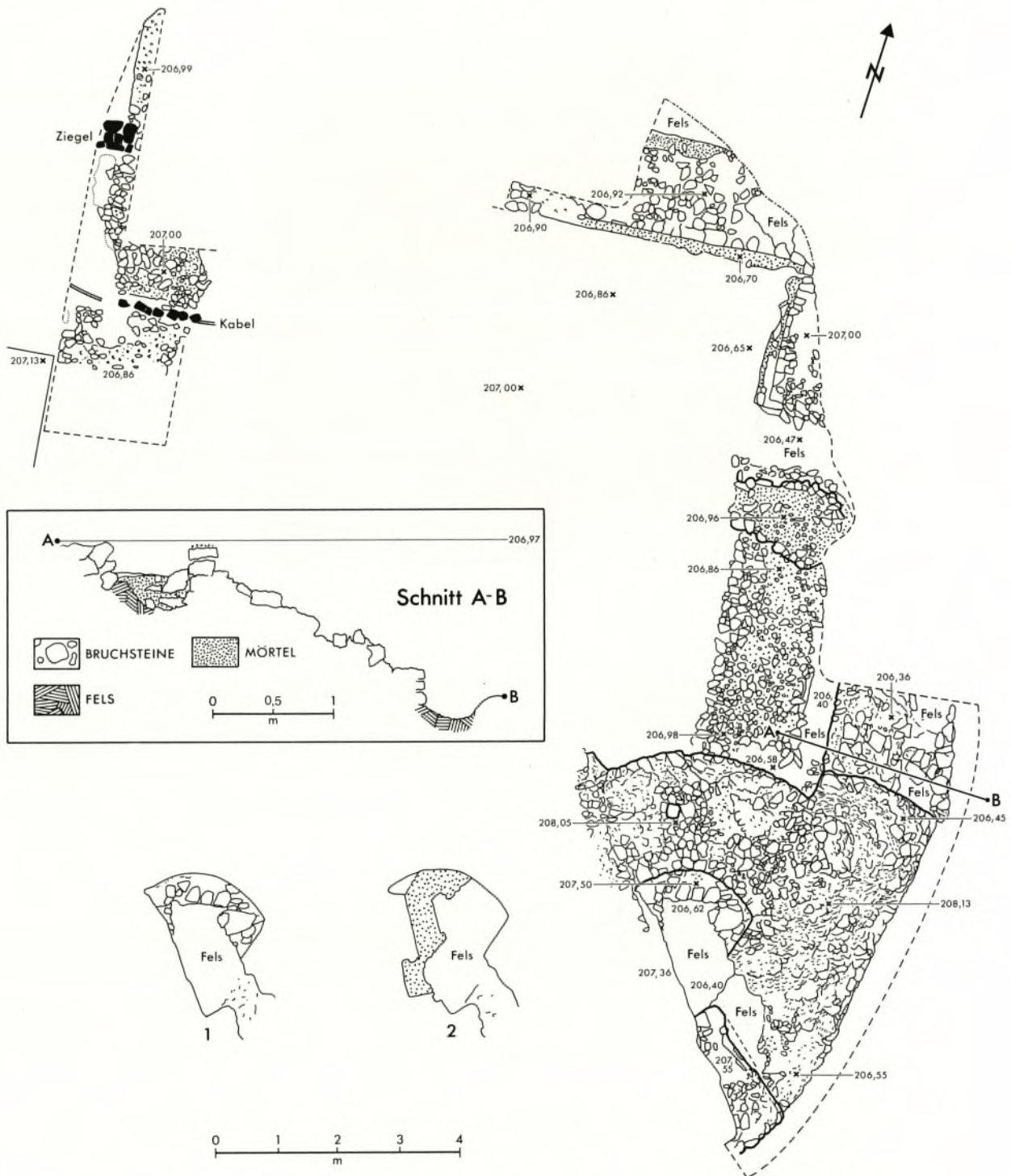
Abb. 39. Burg Sponeck. – Römische Mauerreste auf dem Burghügel. M. 1:100; Profil M. 1:50.
