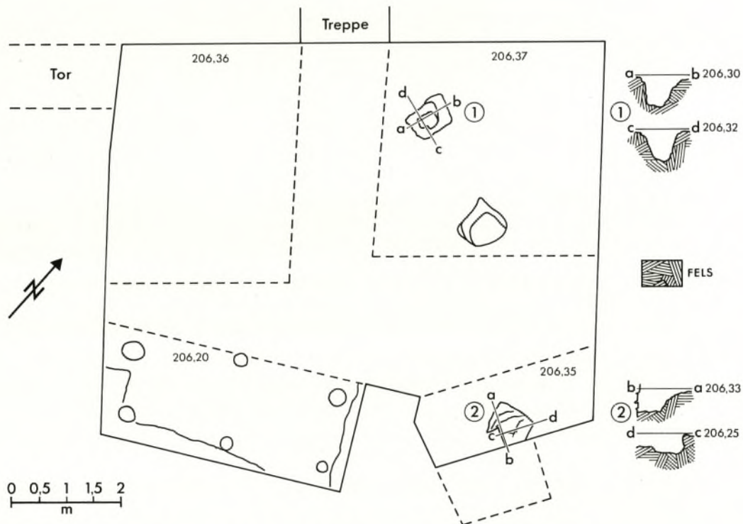
Abb. 42. Burg Sponeck. – Burginneres mit Gruben 1 und 2 sowie Grubenprofilen (Grabungsgrenzen gestrichelt). M. 1:100.
