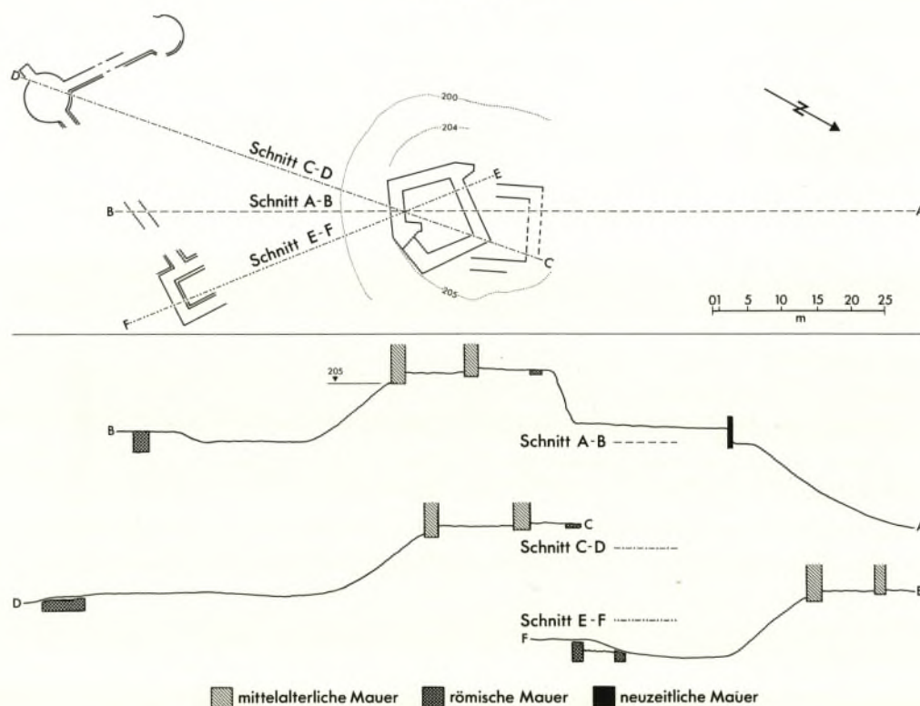
Abb. 48. Burg Sponeck. – Die Lage der Befestigung und der Mauern auf dem Burghügel anhand von Geländeprofilen. M. 1 : 1000.
