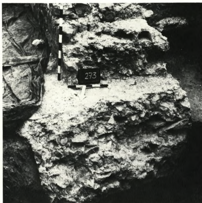
Abb. 24. Burg Sponeck. – Turm 3. Abgebrochene Südwestmauer. Oben rechts Balkenlöcher.
