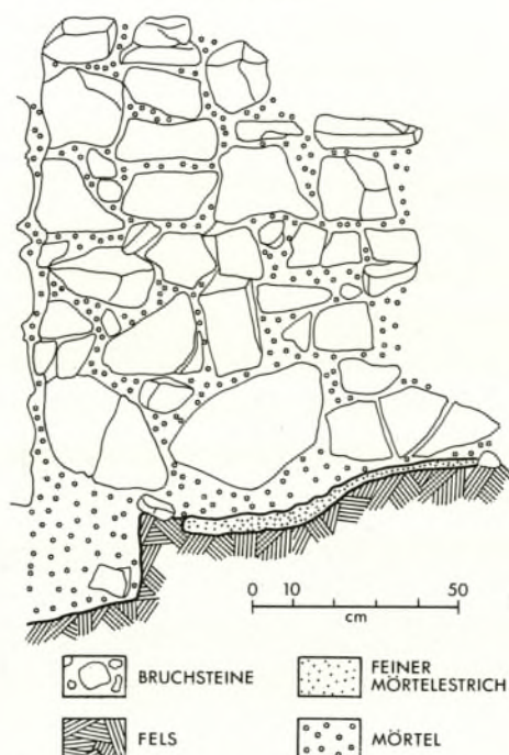
Abb. 47. Burg Sponeck. – Burghügel. Estrichbodenreste unter der mittelalterlichen Mauer von Nordwesten.
