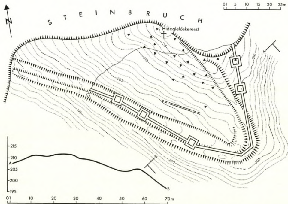
Abb. 52. Plan der spätrömischen Befestigung Esztergom-Hidegtelek-kereszt (Umzeichnung nach Vorlage S. Soproni). M. 1 : 1000.
