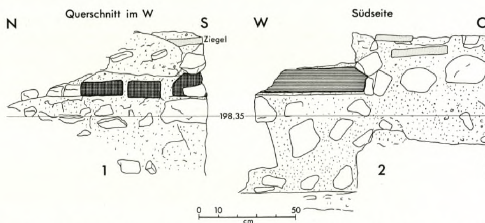
Abb. 25. Burg Sponeck. – Balkenhohlräume in der Südwestmauer von Turm 3. 1 Schnitt N-S von Westen; 2 Ansicht von Süden. M. 1:20.
