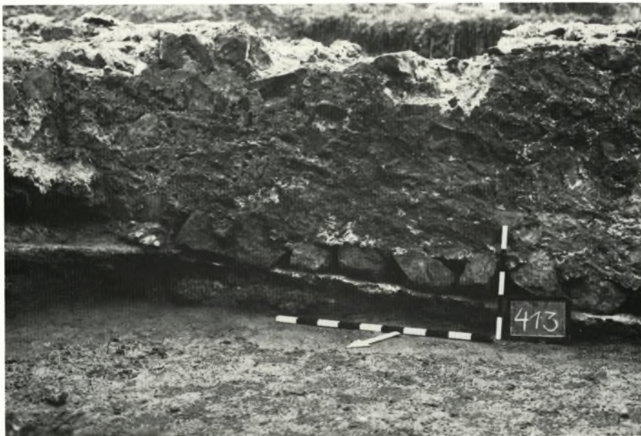
Abb. 17. Burg Sponeck. – Ostmauer. Die überkragende Fundamentdecke an der Mauerinnenseite.
