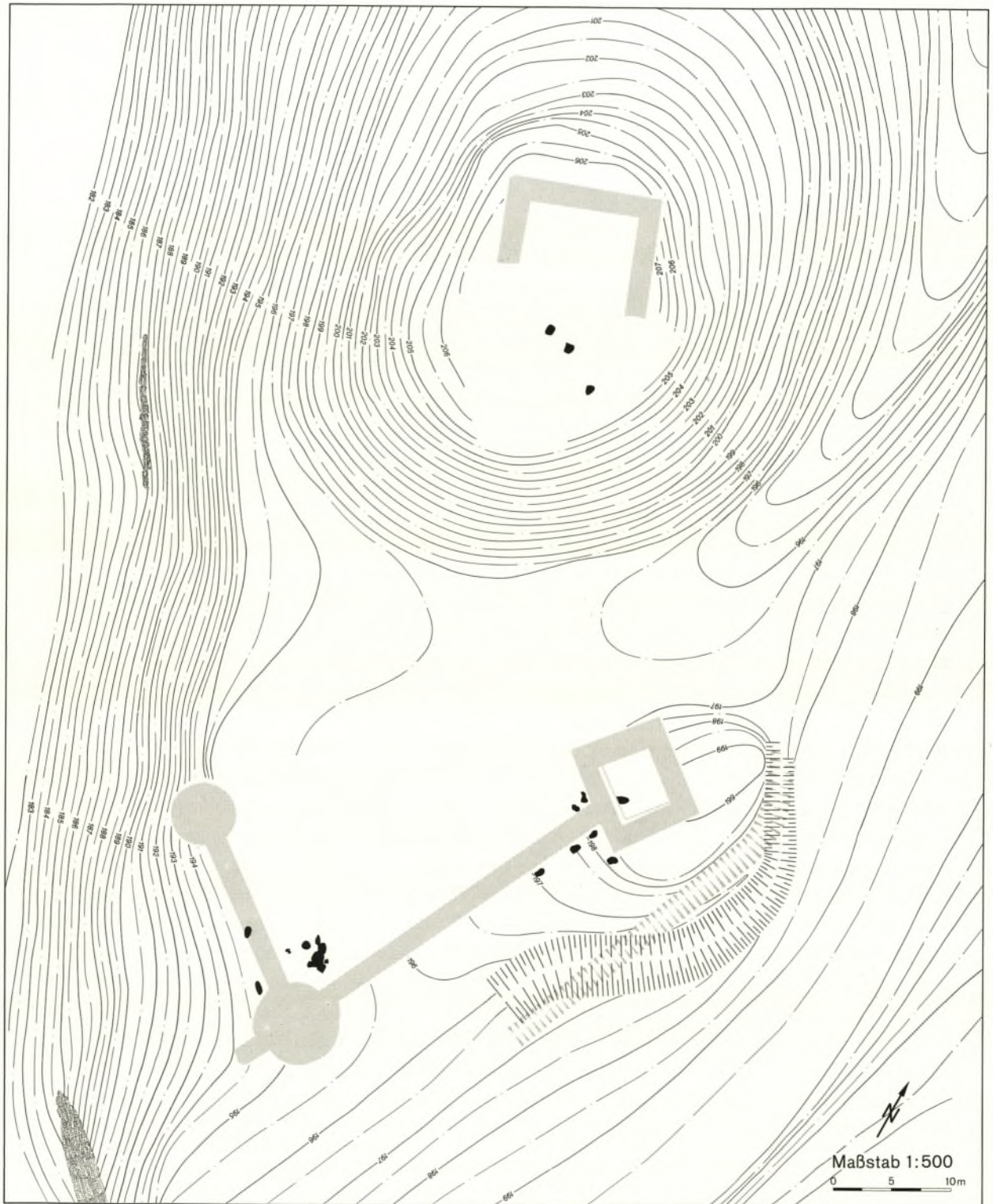
Abb. 5. Plan der Grabung mit den prähistorischen Befunden und dem älteren Wehrgraben (gerastert: spätrömische Befestigung). M. 1:500.
