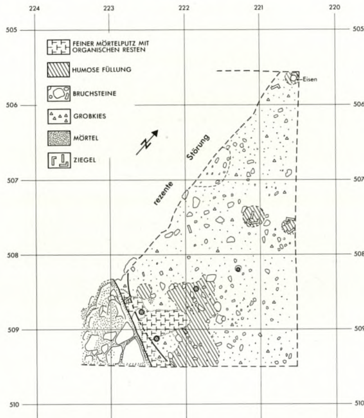
Abb. 34. Burg Sponeck. – Planum zwischen Südwestmauer und rezenten Störung. Mörtelboden mit kreisförmiger Schleifspur. M. 1:50.
