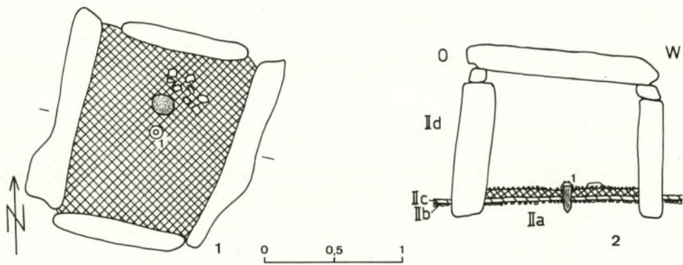
A Hügel 38: 1 Grundriß mit Planum, 2 NS-Schnitt. B Hügel 39: 1 Steinkiste, Grundriß mit Planum, 2 Steinkiste, OW-Schnitt. A: M. 1:100; B: M. 1:40.
