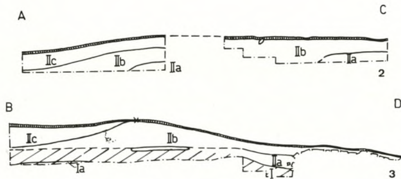
Hügel 47: 1 Grundriß, 2 NO-Profil, 3 SO-Profil. M. 1:100.
