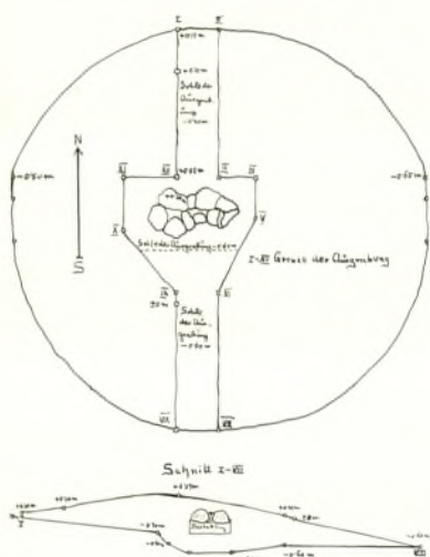
Abb. 112. Rappoltenkirchen (N 21 a), Hügel B 12, Grundriß und N-S-Schnitt. M. 1:200 (Caspert 1932, Beilage 22).
