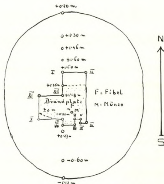
Abb. 85. Erla (N 16), Hügel D 22, Grundriß.
