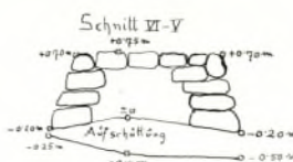
Abb. 100. Unteroberndorf (N 18 a), Hügel F 1, Grundrisse und Schnitte von Hügel und Grabkammer. M. 1:200 und 1:100 (Caspart 1932, Beilagen 54–56).
