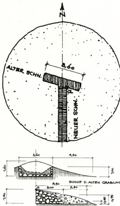
Abb. 75. Wiesfleck (B 76a), Hügel I, Grundriß und Profile. M. 1:200 (Barb 1972, Abb. 3).
