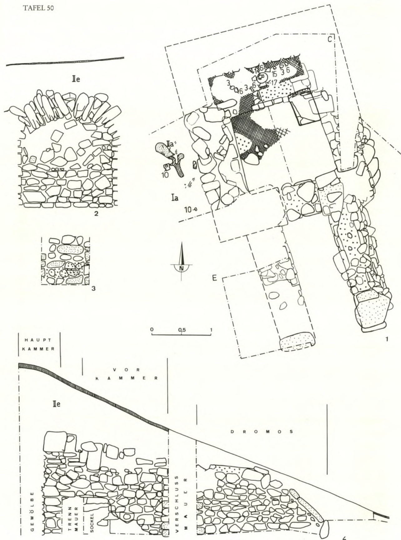
Hügel 53: 1 Mauerkammer mit Planum, 2 n Kammermauer, Innenseite, 3 Verschlussmauer, Außenseite, 4 ö Kammer- und Dromosmauer, Innenseite. M. 1:40.
