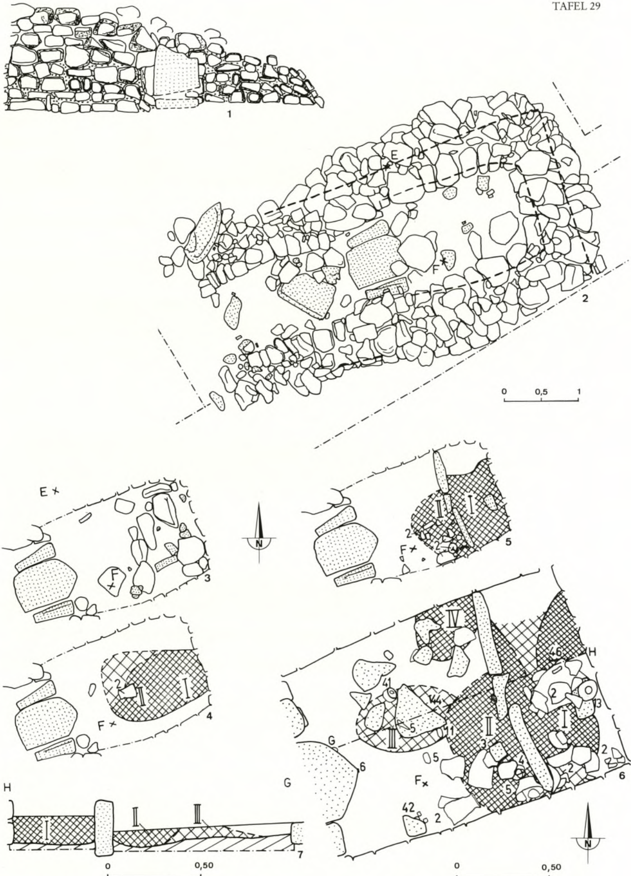
Hügel 37: 1 s Dromos- und Kammermauer, Innenseite, 2 Mauerkammer, Grundriß, Planum 1 (etwa 100–120 cm u. Fxpkt. F), 3 Planum 2 in der Grabkammer (190 cm), 4 Planum 3 (205 cm), 5 Planum 4 (215 cm), 6 Planum 5 (225 cm), 7 S-Profil u. Planum 5.
