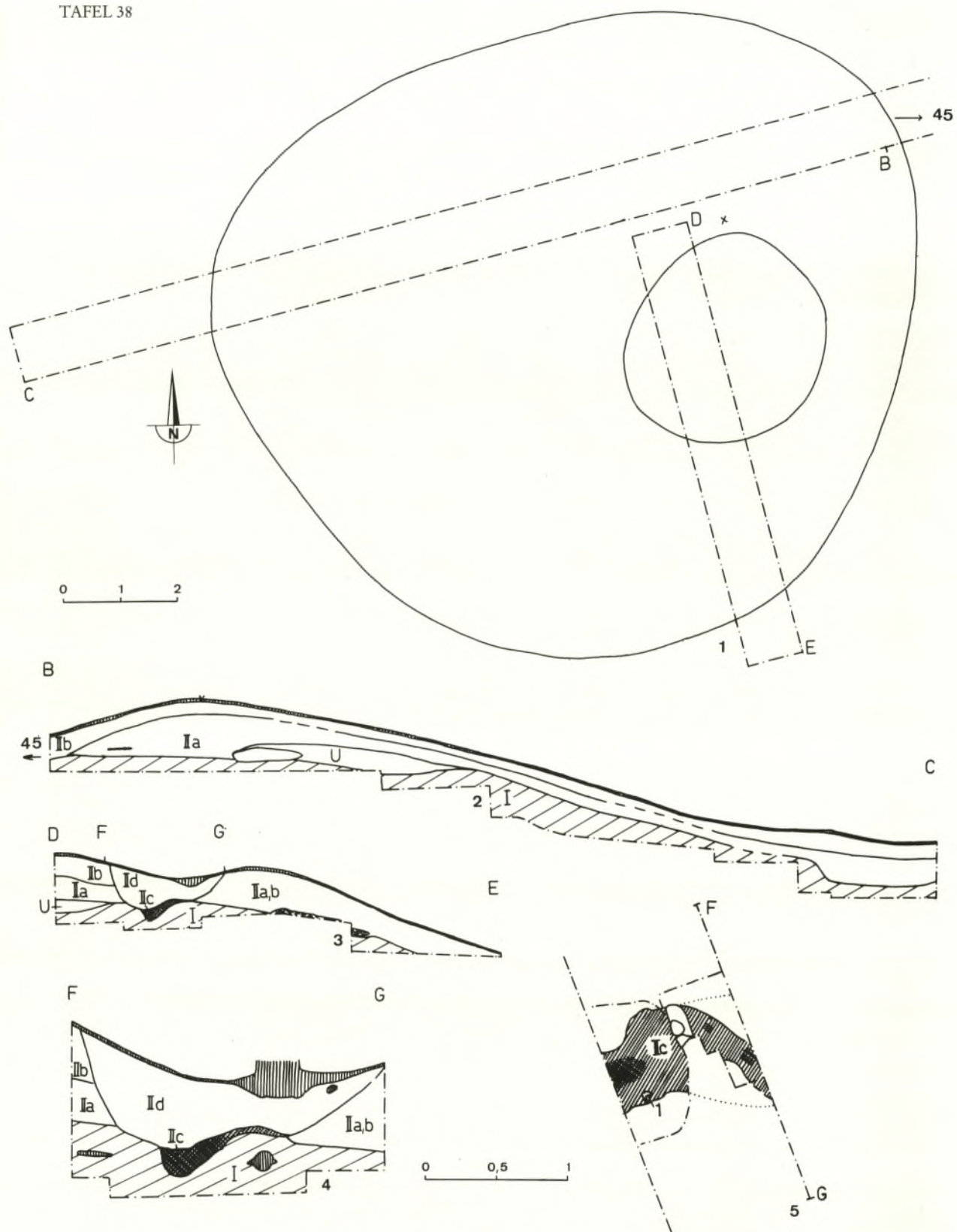
Hügel 46: 1 Grundriß, 2 S-Profil, 3 O-Profil, 4 O-Profil, 5 Planum I (40-60 cm u. HOK.). 1-3: M. 1:100; 4-5: M. 1:40.
