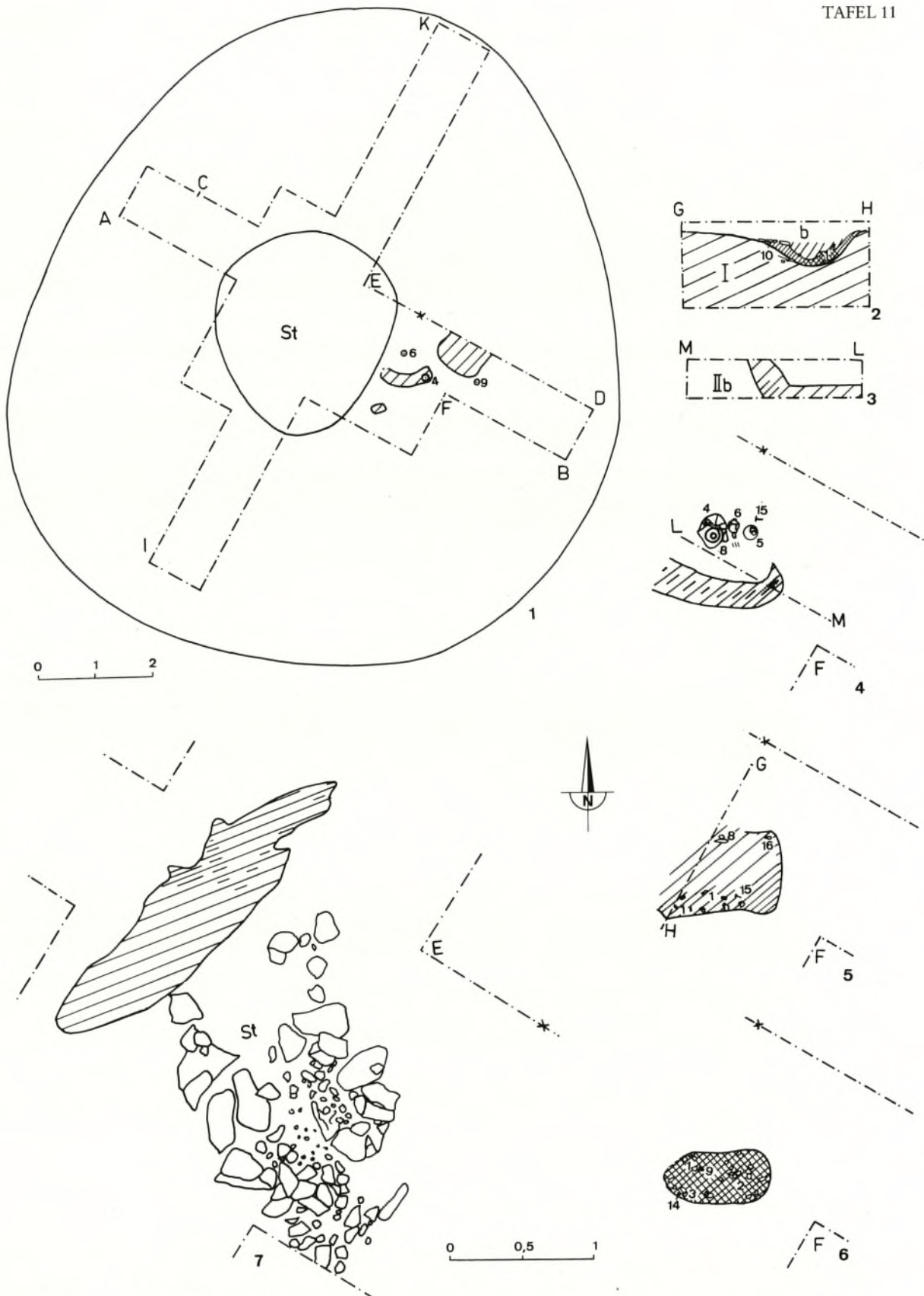
Hügel 16: 1 Grundriß mit Planum 1 (90 cm u. Fxpkt.), 2 SO-Profil u. Planum 2, 3 SW-Profil u. Planum 1, 4 Planum 1, 5 Planum 2 (115 cm), 6 Planum 3 (140 cm), 7 Planum 2 im Zentrum.
