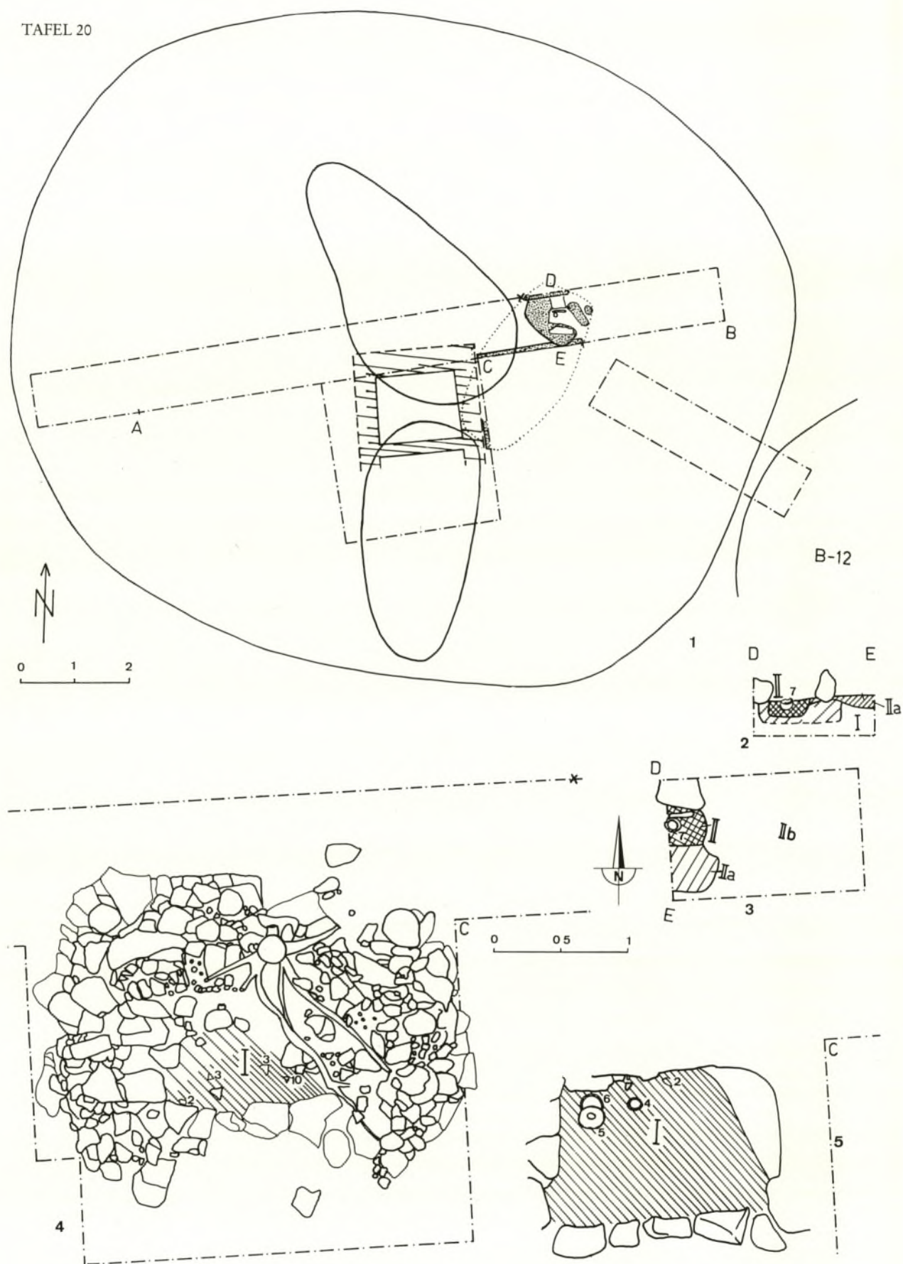
Hügel 26: 1 Grundriß mit Planum 1 im OW-Schnitt (120 cm u. Fxpkt.), 2 O-Profil u. Planum 2 im OW-Schnitt, 3 Planum 2 im OW-Schnitt (135 cm), 4 Planum 1 im Zentrum (140 cm), 5 Planum 2 im Zentrum (150 cm).
