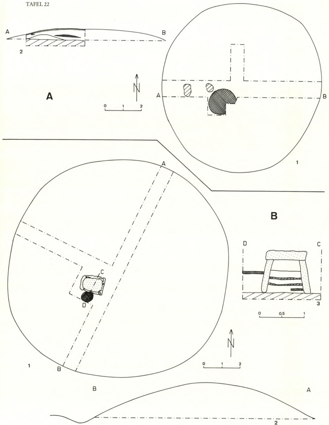
A Hügel 27: 1 Grundriß mit Planum (45 cm u. HOK.), 2 S-Profil. B Hügel 30: 1 Grundriß mit Planum, 2 W-Profil, 3 Steinkiste, NS-Schnitt. A, B 1-2: M. 1:100; B 3: M. 1:40.
