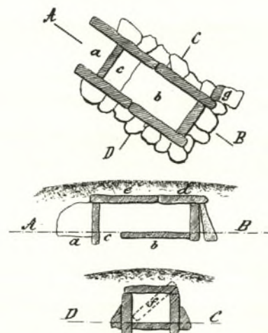
Abb. 137. Vordersdorf (St 36 d), Hügel 1, Steinkammer, Grundriß und Schnitte.
