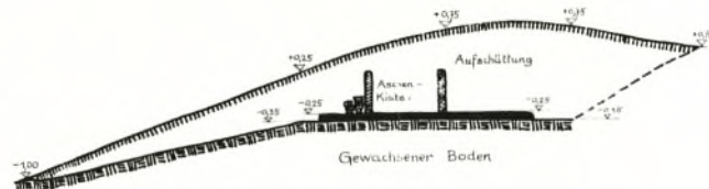
Abb. 110. Rappoltenkirchen (N 21 a), Hügel B 2, Grundriß und N-S-Schnitt. M. 1:200 und 1:100 (Caspert 1932, Beilagen 13 und 14).
