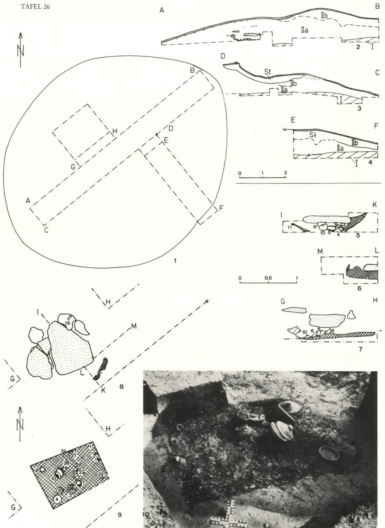
Hügel 33: 1 Grundriß, 2 NW-Profil, 3 SO-Profil, 4 NO-Profil u. Planum 1, 5 NO-Profil u. Planum 1, 6 SO-Profil u. Planum 1, 7 NW-Profil u. Planum 1, 8 Planum 1 (110 cm u. Fxpkt.), 9 Planum 2 (130 cm u. Fxpkt.), 10 Ansicht von N (Planum 2).
