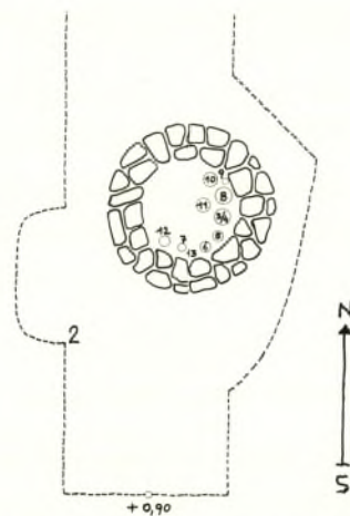
Abb. 103. Unterberndorf (N 18 b), Hügel E 2, Grundriß der Steinkammer. M. 1:100 (Caspert 1932, Beilage 53, Ausschnitt: „E 3“).
