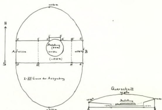
Abb. 113. Rappoltenkirchen (N 21 a), Hügel B 4, Grundriß und W-O-Schnitt. M. 1:200 (Caspert 1932, Beilage 16).
