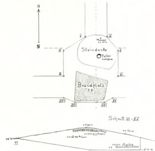
Abb. 109. Rappoltenkirchen (N 21 a), Hügel B 7, Ausschnitt aus dem Grundriß mit N-S-Schnitt. M. 1:100 (Caspert 1932, Beilagen 19, Ausschnitt, und 20, Teil).
