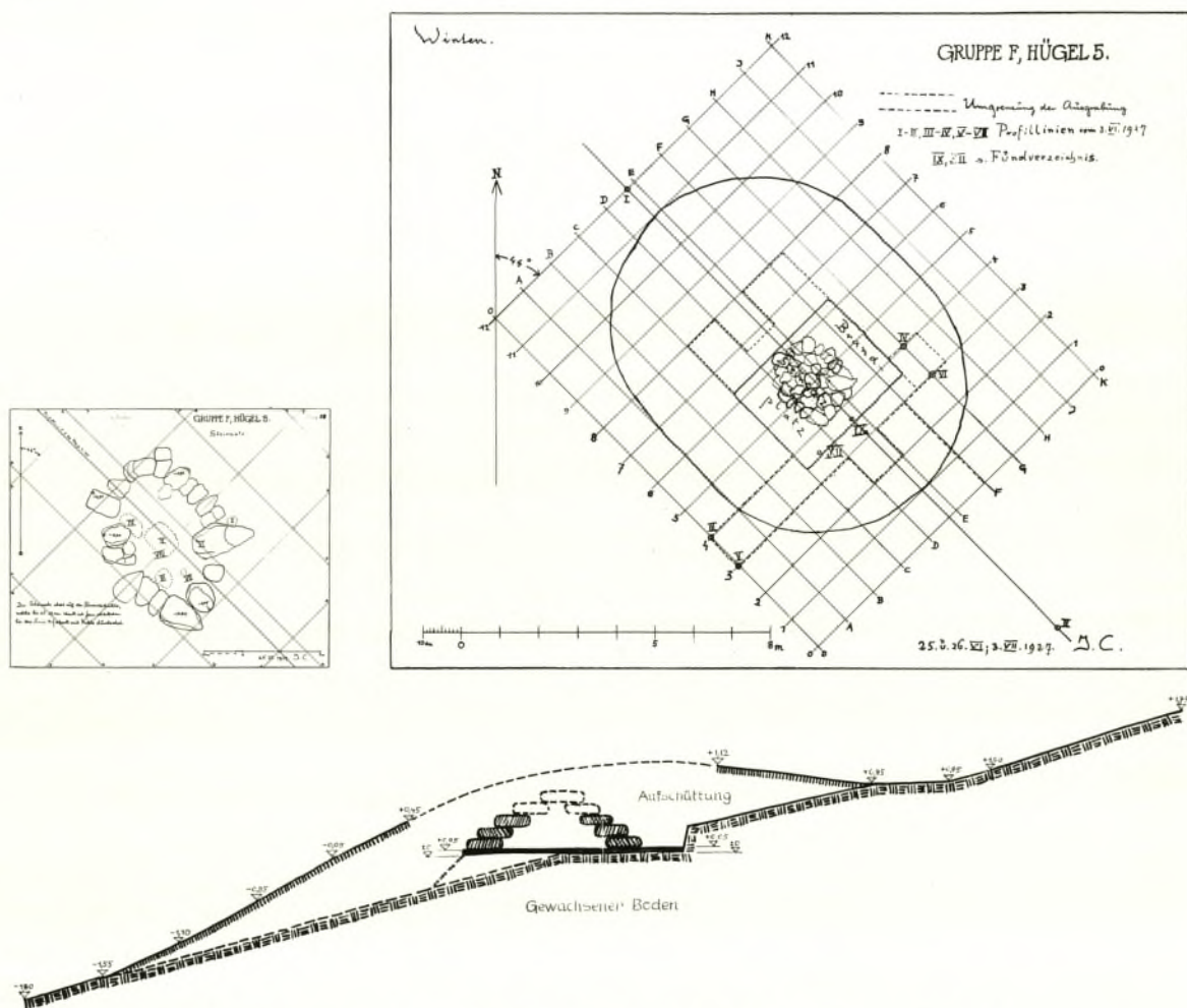
Abb. 101. Unterberndorf (N 18 a), Hügel F 5, Grundriß und NW-SO-Schnitt, Grundriß der Grabkammer. M. 1:200 und 1:100 (Caspert 1932, Beilagen 14, 57 und 58).
