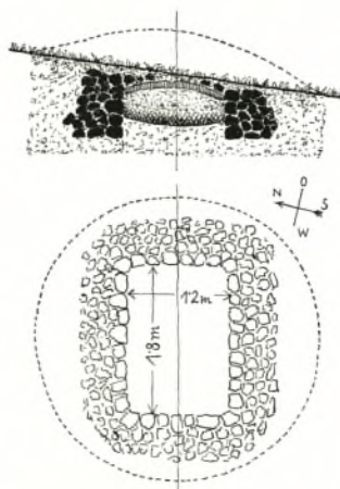
Abb. 127. Obernberg (S 4), Hügelgrundriß und N-S-Schnitt.
