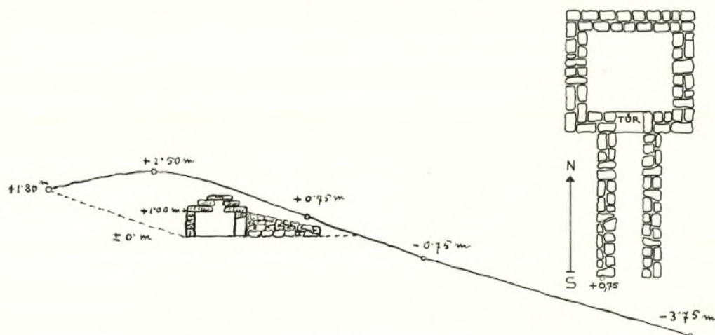
Abb. 99. Getzwiesen (N 17), Hügel K 1, Grundriß der Steinkammer und N-S-Schnitt. M. 1:100 und 1:200 (Caspart 1932, Beilagen 68, Ausschnitt, und 69).
