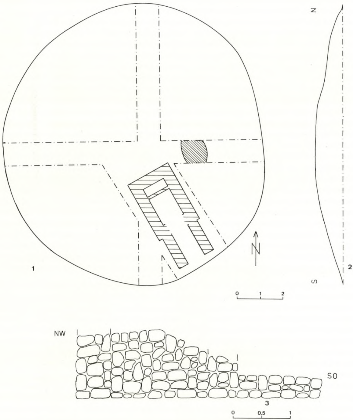
Hügel 52: 1 Grundriß mit Planum; 2 NS-Schnitt, 3 sw Kammer- und Dromosmauer, Außenseite. 1-2: M. 1:100; 3: M. 1:40.
