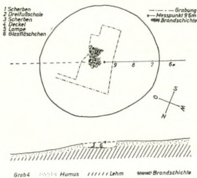
Abb. 155. Hütteldorf (W 1), Grab 4, Grundriß und O-W-Schnitt.
