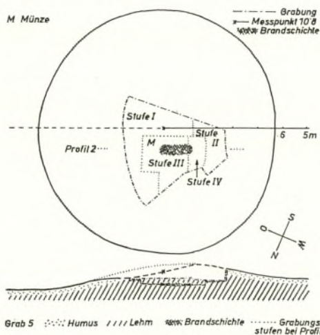
Abb. 156. Hütteldorf (W 1), Grab 5, Grundriß und O-W-Schnitt.
