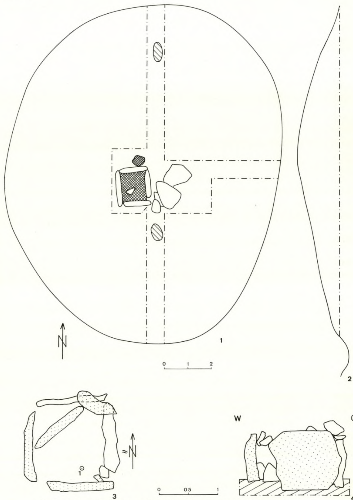
Hügel 17: 1 Grundriß mit Planum, 2 NS-Schnitt, 3 Steinkiste, Grundriß, 4 Steinkiste, Ansicht von S. 1-2: M. 1:100; 3-4: M. 1:40.
