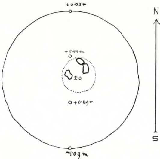
Abb. 88. Erla (N 16), Hügel D 18, Grundriß. M. 1:200 (Caspert 1932, Beilage 41).
