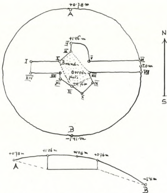
Abb. 108. Rappoltenkirchen (N 21 a), Hügel B 3, Grundriß und N-S-Schnitt. M. 1:200 (Caspert 1932, Beilage 15).
