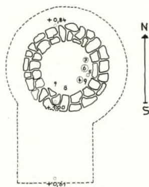
Abb. 102. Unterberndorf (N 18 b), Hügel E 1, Grundriß der Steinkammer. M. 1:100 (Caspert 1932, Beilage 52, Ausschnitt).
