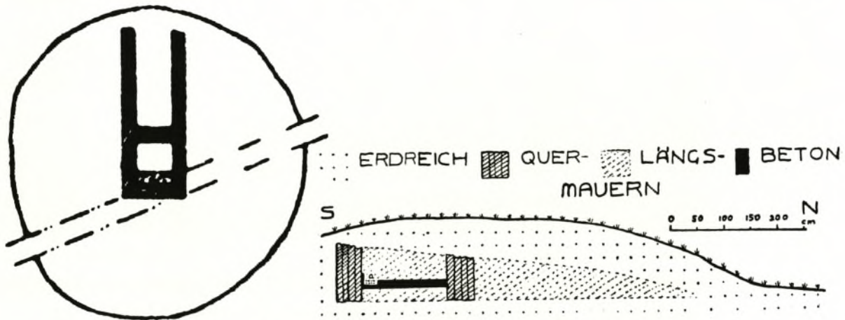
Abb. 68. Schandorf (B 66 d), Hügel X, Grundriß und SW-NO-Profil. M. 1:200 und 1:100 (Barb 1937, Abb. 3 und 4).
