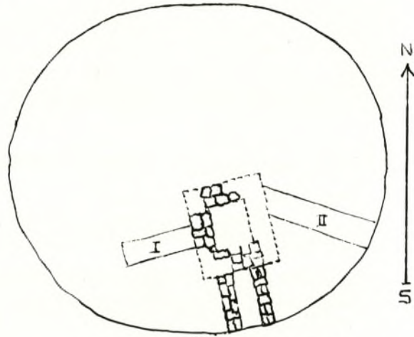
Abb. 82. Hart (N 15), Hügel J 9, Grundriß. M. 1:200 (Caspart 1932, Beilage 64).
