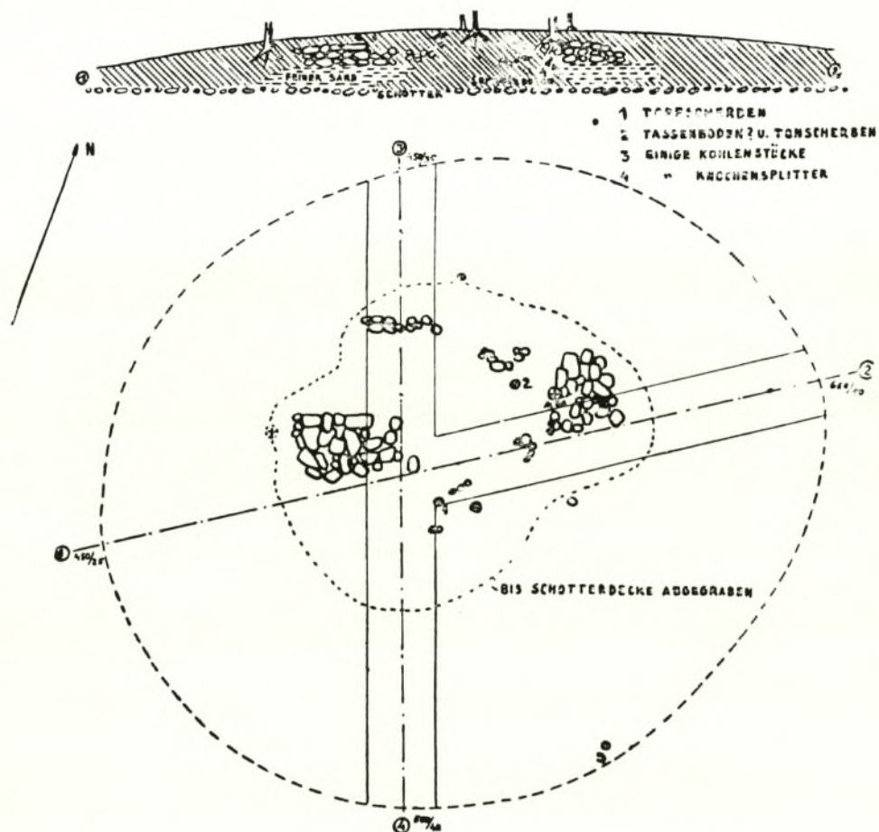
Abb. 105. Purgstall und Schauboden (N 19), Hügel 4, Grundriß und SW-NO-Profil. M. etwa 1:200 (Vetters 1954, Abb. 46).
