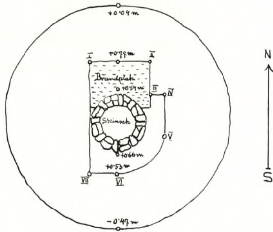
Abb. 91. Erla (N 16), Hügel D 13, Grundriß. M. 1:200 (Caspert 1932, Beilage 36).
