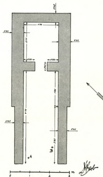
Abb. 57. Großpetersdorf (B 40b), Hügel I/5, Grundriß der Grabkammer.
