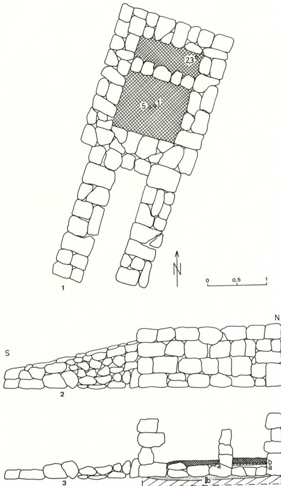
Hügel 32: 1 Mauerkammer, Grundriß, 2 ö Kammer- und Dromosmauer, Außenansicht, 3 NS-Schnitt durch Steinsetzung. M. 1:40.
