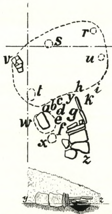
Abb. 129. Kerschbaum (St 19 a), Hügel 1, Ausschnitt aus Grundriß und N-S-Schnitt. M. 1:100 (Radimský u. Szombathy 1888, Abb. 28 und 30).
