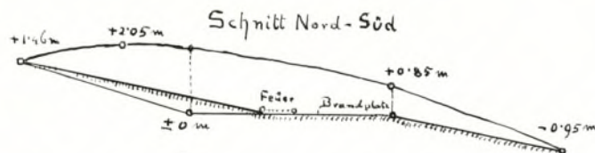
Abb. 98. Erla (N 16), Hügel D 21, Grundriß und N-S-Schnitt. M. 1:200 (Caspart 1932, Beilage 44).
