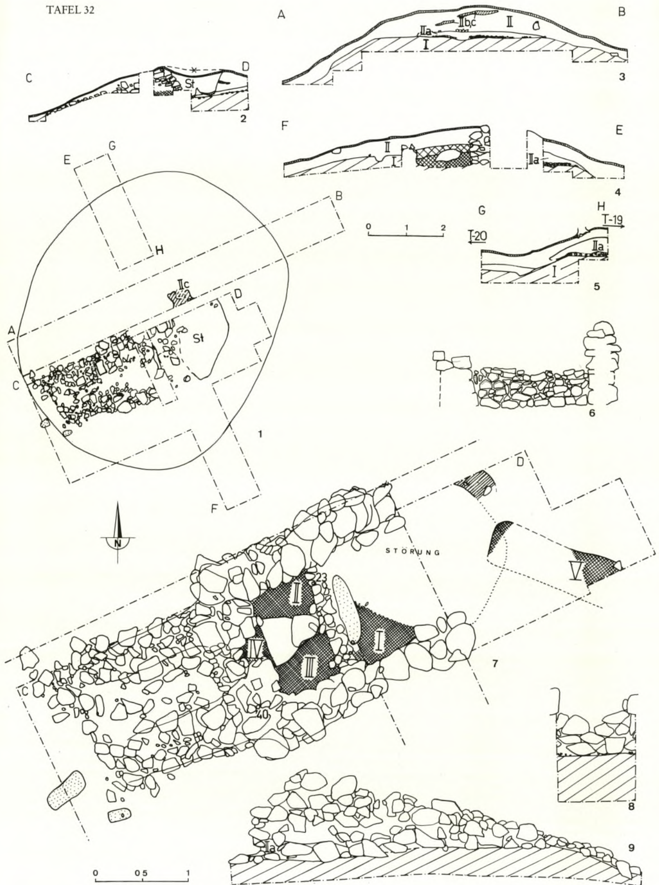
Hügel 40: 1 Grundriß mit Planum 1, 2 S-Profil, 3 N-Profil, 4 W-Profil, 5 O-Profil, 6 Trennmur von W, 7 Planum 2, 8 Verschlussmauer von W, 9 n Dromos- und Kammermauer, Außenseite.
