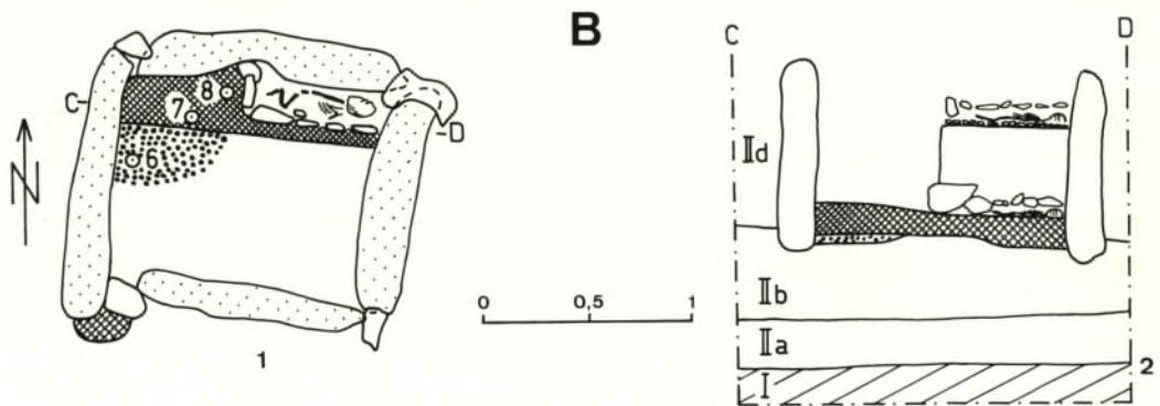
A Hügel 19: 1 Grundriß mit Planum, 2 NS-Schnitt, 3 Steinkiste, Grundriß, 4 Schnitt durch die nw Seite der Kiste.
