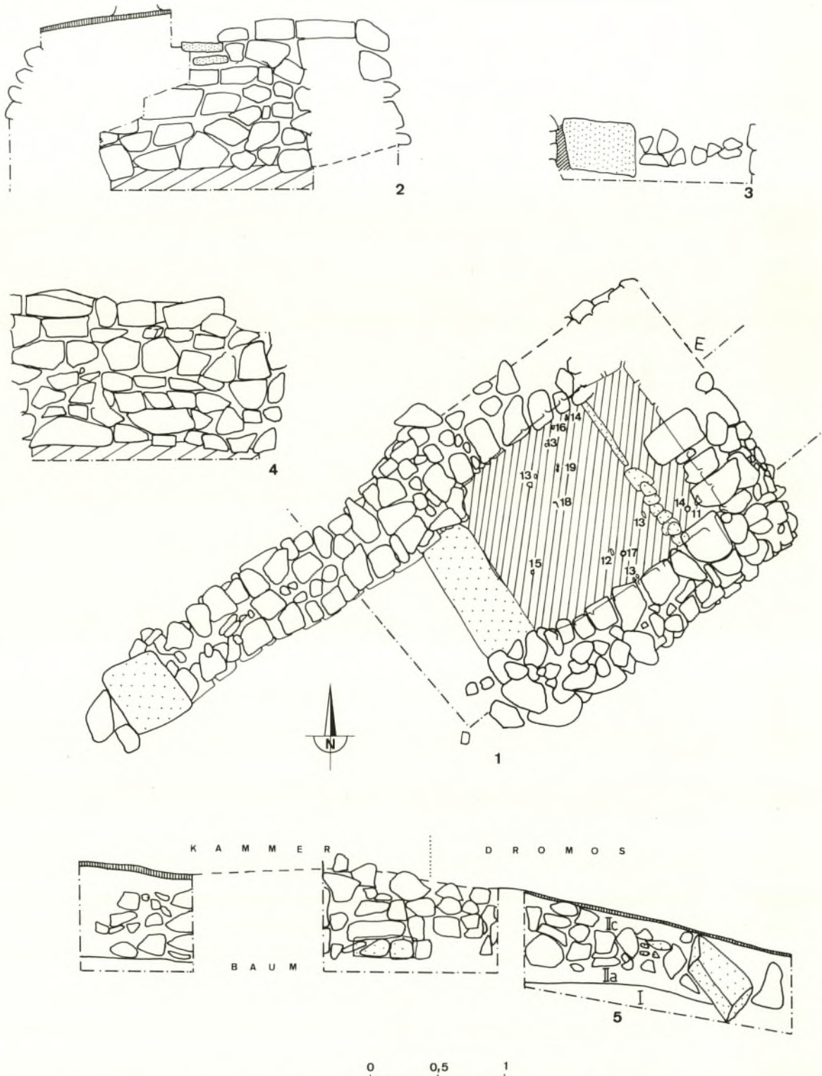
Hügel 47: 1 Mauerkammer, Grundriß mit Planum 1 und 2 (abgestufte Strichstärke), 2 nö Kammermauer, Innenseite, 3 Trennmauer von SW, 4 sö Kammermauer, Innenseite, 5 nw Dromos- und Kammermauer, Außenseite.
