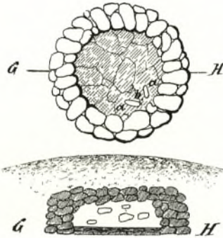
Abb. 133. Wieden (St 23 a), Hügel 1, Steinkammer, Grundriß und W-O-Schnitt.
