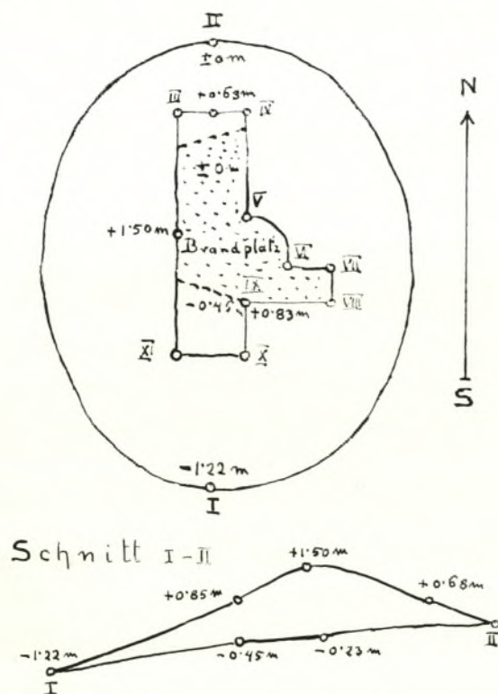
Abb. 120. Rekawinkel (N 24 a), Hügel G 2, Grundriß und S-N-Schnitt.
