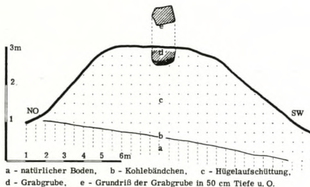
Abb. 50. Königsdorf (B 15 b), Hügel 1, NO-SW-Profil. M. 1:100 bzw. 1:200 (Kaus 1978, 92).
