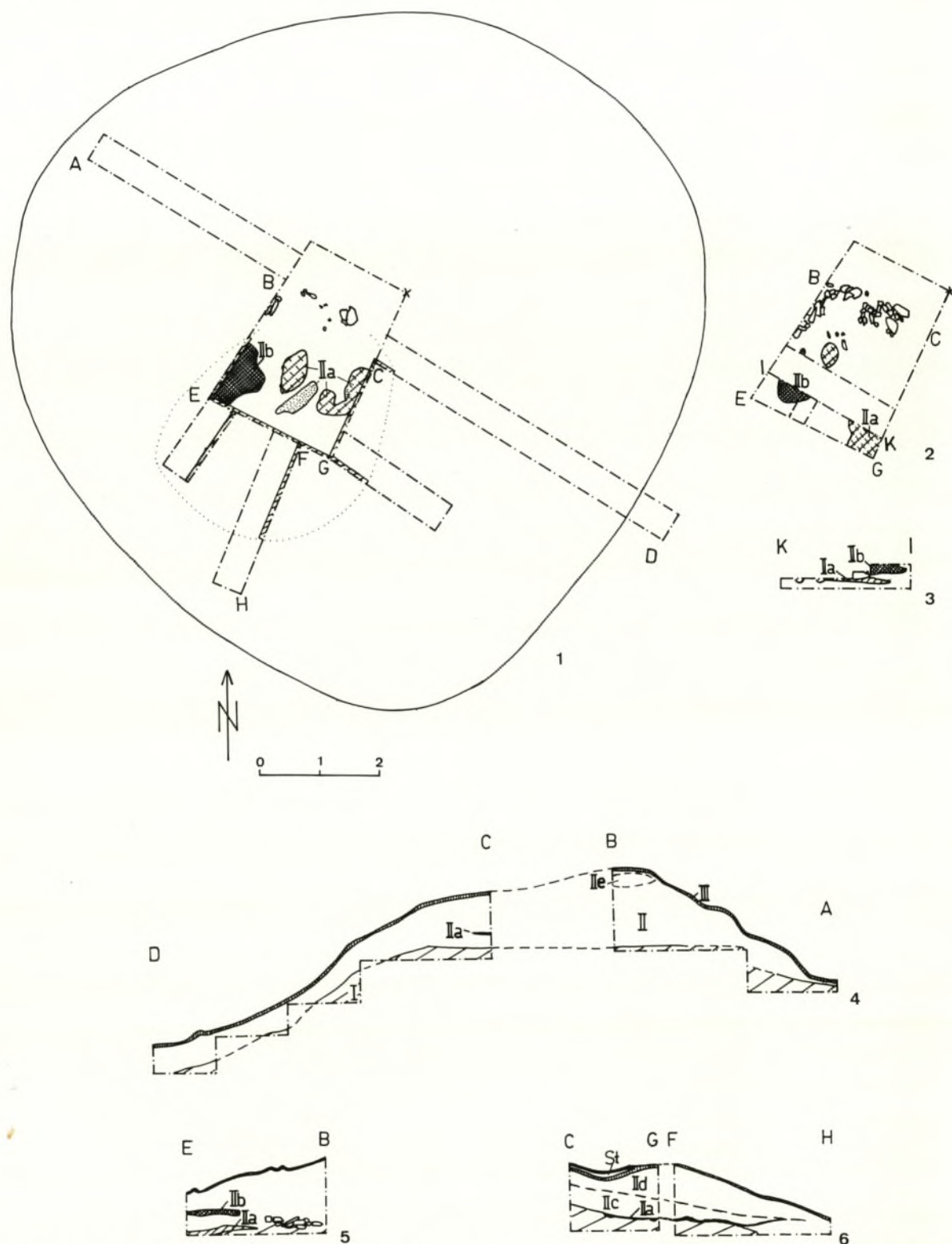
Hügel 11: 1 Grundriß mit Planum 1 (90 cm u. Pkt. B), 2 Planum 2 (110 cm), 3 S-Profil u. Planum 2, 4 S-Profil, 5 W-Profil, 6 versetztes O-Profil. M. 1:100.
