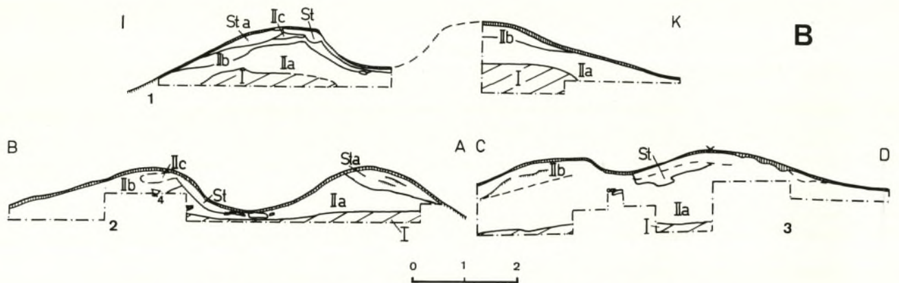
A Hügel 15: 1 Grundriß mit Planum 1 (55 cm u. HOK.), 2 SO-Profil, 3 Planum 1. B Hügel 16: 1 NW-Profil, 2 SW-Profil, 3 NO-Profil. A 1,3, B: M. 1:100; A 2: M. 1:40.
