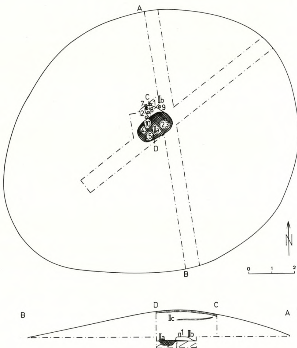
Hügel 23: 1 Grundriß mit Planum (130 cm u. HOK.), 2 W-Profil. M. 1:100.
