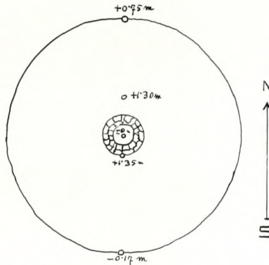
Abb. 90. Erla (N 16), Hügel D 11, Grundriß. M. 1:200 (Caspert 1932, Beilage 34).
