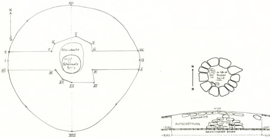
Abb. 118. Au a. K. (N 23b), Hügel C 2, Grundriß, Grabkammer und N-S-Schnitt. M. 1:200 und 1:100 (Caspert 1932, Beilagen 27–29).
