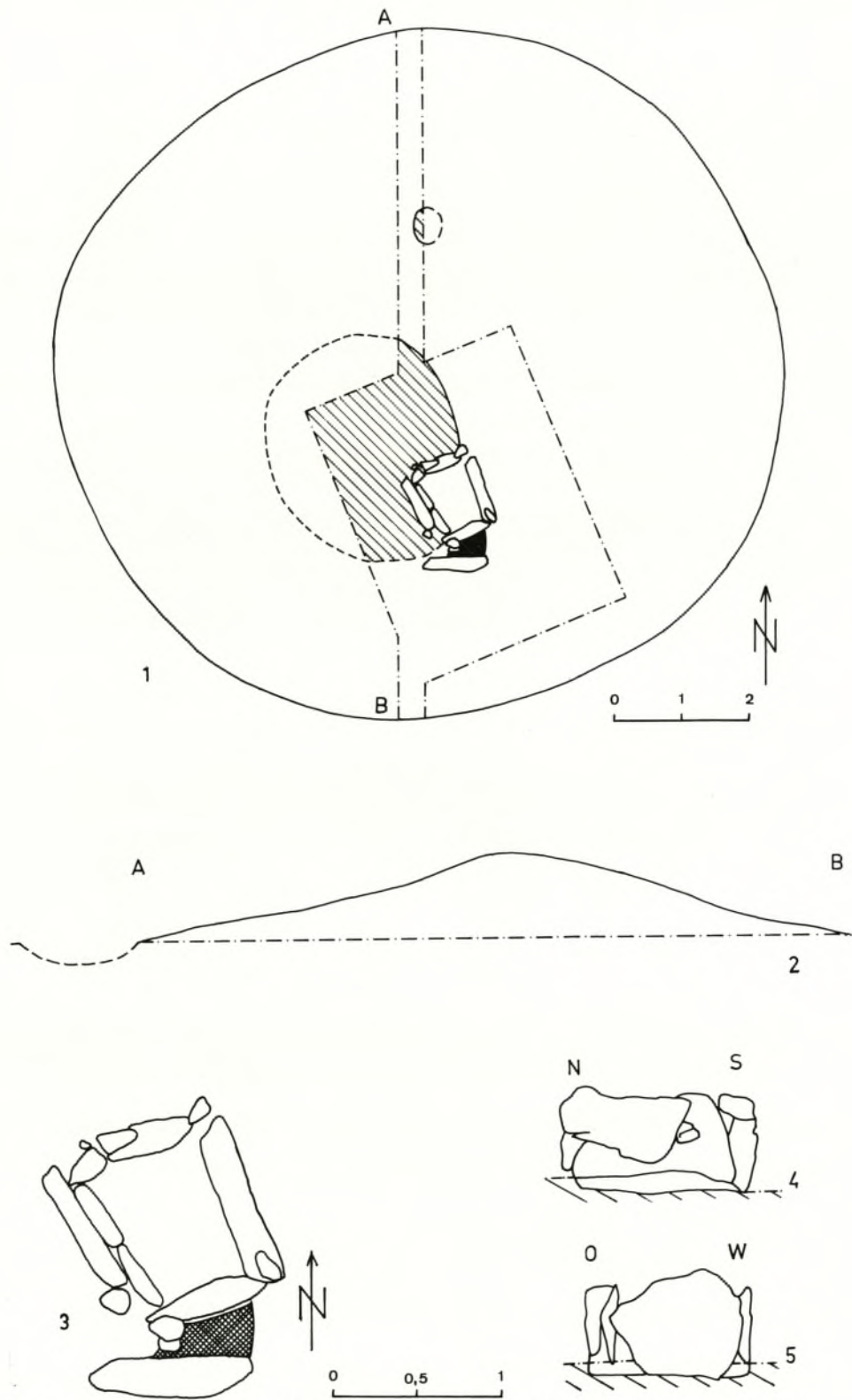
Hügel 28: 1 Grundriß mit Planum, 2 NS-Schnitt, 3 Steinkiste, Grundriß, 4 Steinkiste von W, 5 Steinkiste von N. 1-2: M. 1:100; 3-5: M. 1:40.
