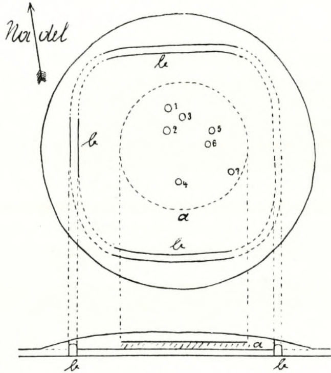
Abb. 54. Neusiedl a. S. (B 23), Hügel 3, Grundriß: 1-7 Pfahllöcher, a Brandschicht, b Mauer aus steilgestellten Bruchsteinen. M. 1:200 (Mühlhofer 1927, Abb. 12).
