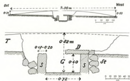
Abb. 142. Grafendorf (St 133), Ellison-Hügel, O-W-Schnitte.
