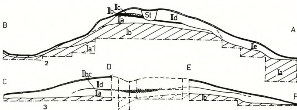
Hügel 6: 1 Grundriß mit Planum 1 (60 cm u. Fxpkt.), 2 S-Profil, 3 O-Profil. M. 1:100.
