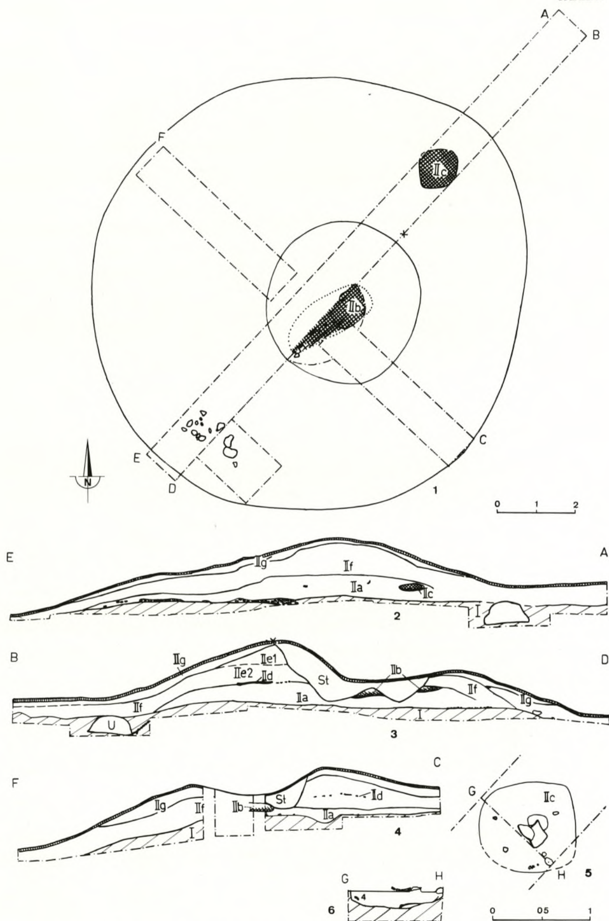
Hügel 42: 1 Grundriß mit Planum 1, 2 NW-Profil, 3 SO-Profil, 4 NO-Profil, 5 Planum 1 im nö Teil des SW-NO-Schnitts (75 cm u. Fxpkt.), 6 NO-Profil u. Planum 1.
