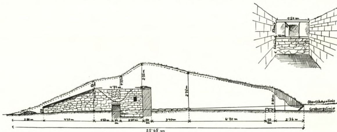
Abb. 140. Oberwaldbauern (St 132), Hügel AI, NO-SW-Schnitt und Blick in die Grabkammer. M. 1:200 und 1:100 (Barb 1937, Abb. 11).
