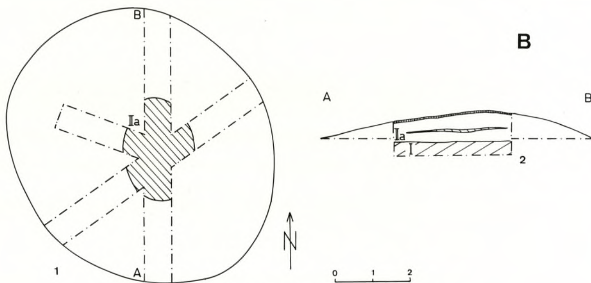
A Hügel 12: 1 Grundriß mit Planum, 2 S-Profil. B Hügel 13: 1 Grundriß mit Planum I (50 cm u. HOK.), 2 W-Profil. M. 1:100.
