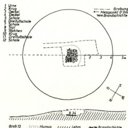
Abb. 163. Hütteldorf (W 1), Grab 13, Grundriß und O-W-Schnitt.
