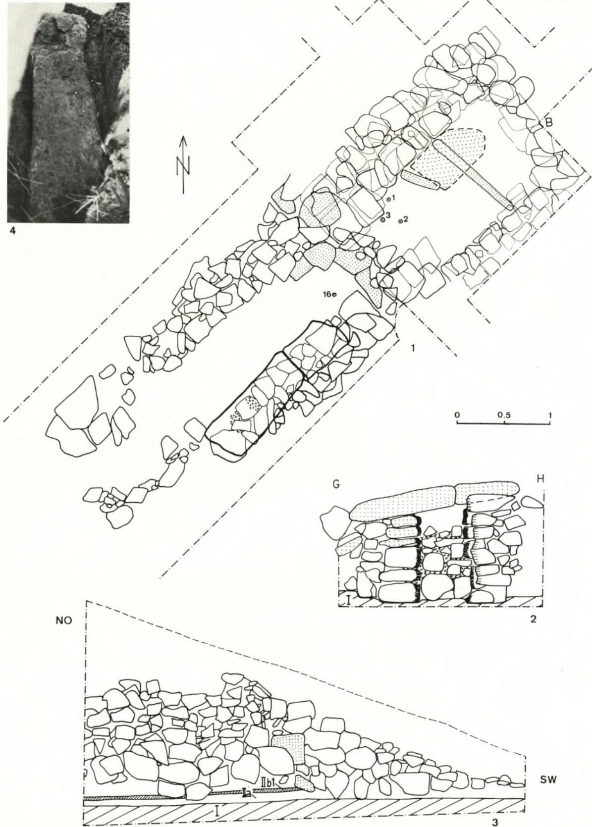
Hügel 43: 1 Mauerkammer, Grundriß mit Planum 1-3 (abgestufte Strichstärken), 2 Verschußmauer von SW, 3 nw Dromos- und Kammermauer, Außenseite, 4 Steinstele.
