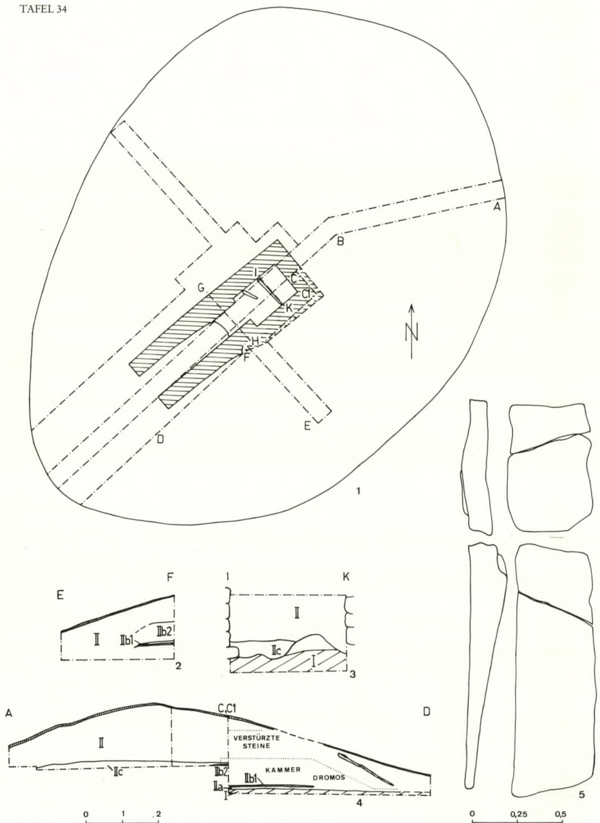
Hügel 43: 1 Grundriß, 2 SW-Profil, 3 NO-Profil in Hauptkammer, 4 versetztes SO-Profil, 5 Steinstele, Umriß und Schnitt. 1.2.4: M. 1:100; 3: M. 1:40; 5: M. 1:20.
