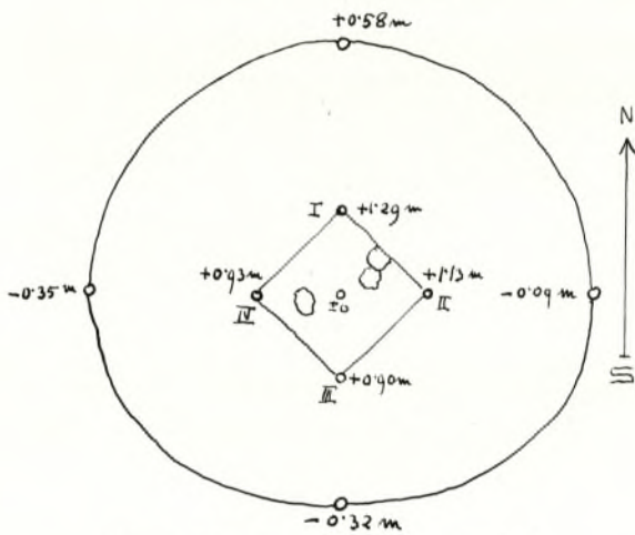
Abb. 87. Erla (N 16), Hügel D 6, Grundriß. M. 1:200 (Caspert 1932, Beilage 33).
