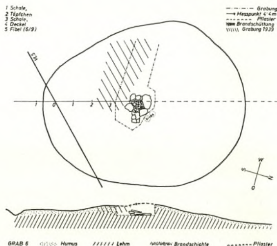
Abb. 157. Hütteldorf (W 1), Grab 6, Grundriß und O-W-Schnitt.
