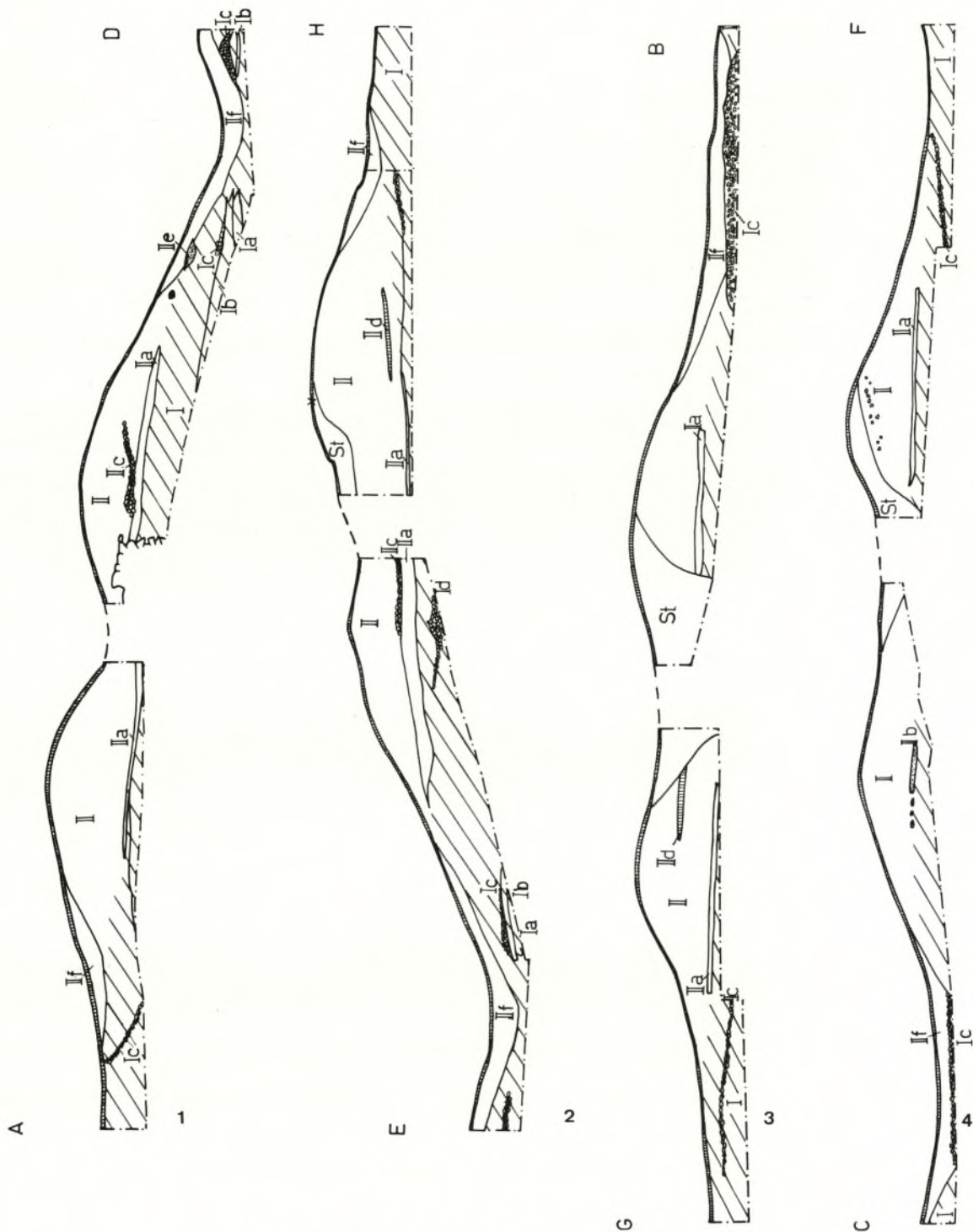
Hügel 50: 1 SO-Profil; 2 NW-Profil, 3 NO-Profil, 4 SW-Profil. M. 1:100.
