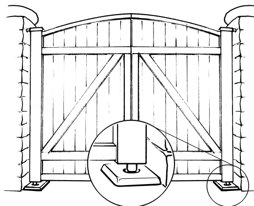
Abb. 14: Tor mit Kegeltrum (Traunstein).
